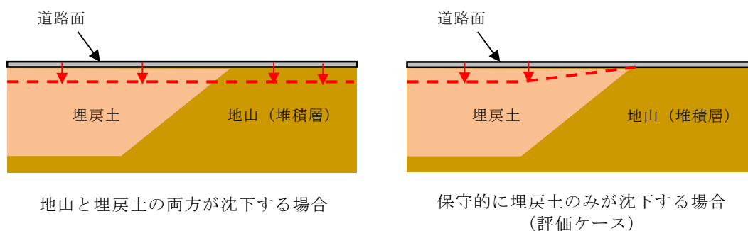
第 5. 4. 3-4 図 揺すり込みや液状化による沈下のイメージ図
