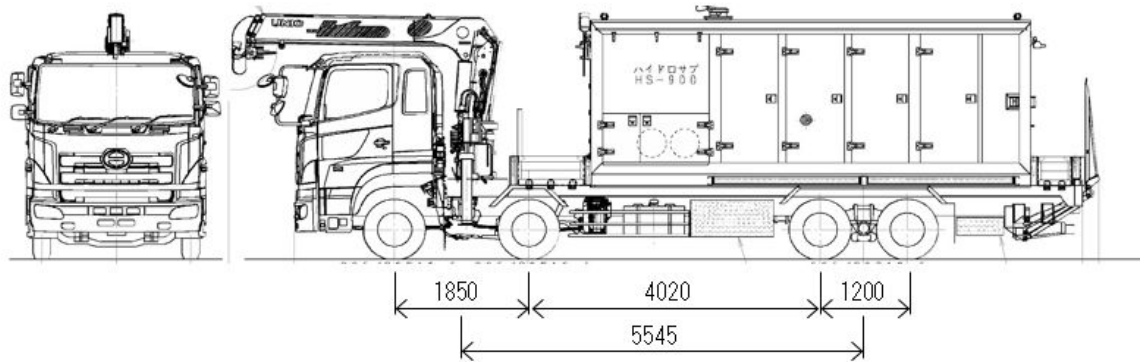
第2図 大型ポンプ車
