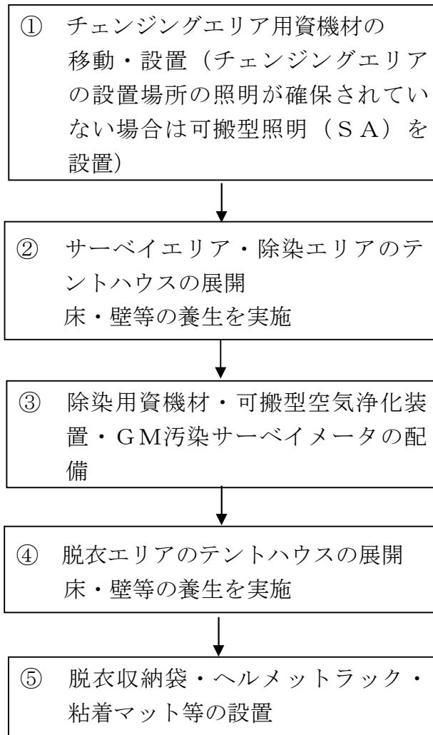
第4図 チェンジングエリアの設営フロー
