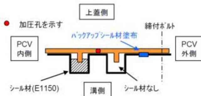
第 10 図 内シール材+PCV 外側バックアップシール材塗布条件
