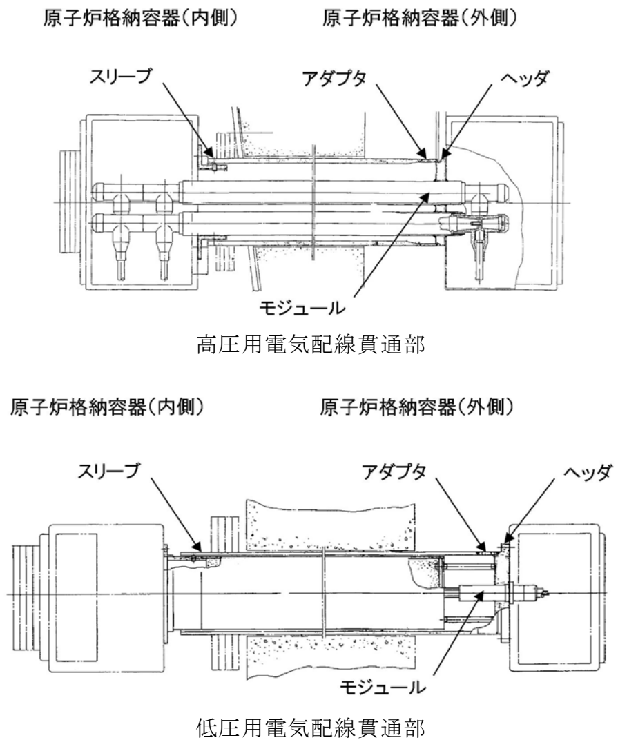
第 14 図 ヘッダの評価対象
