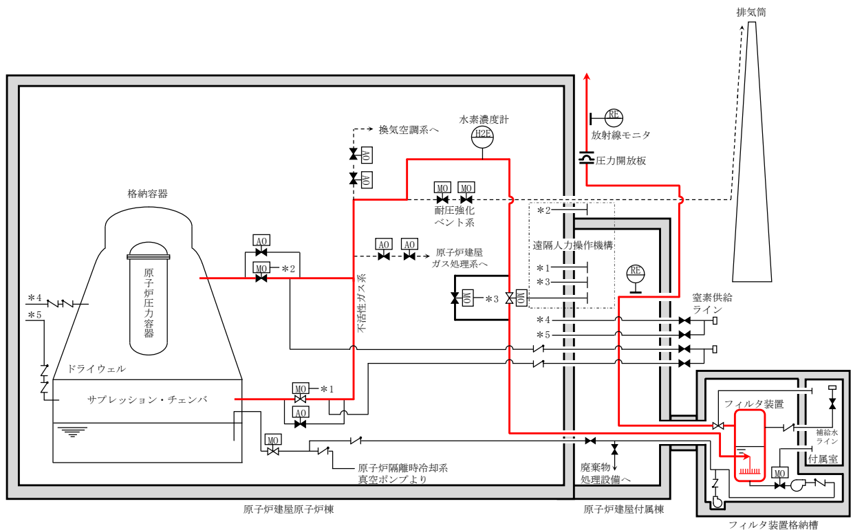
第 1 図 格納容器圧力逃がし装置 概要図
