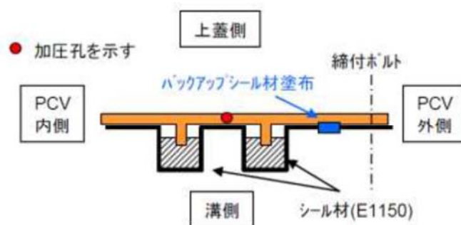
第 9 図 内外シール材+PCV 外側バックアップシール材塗布条件
