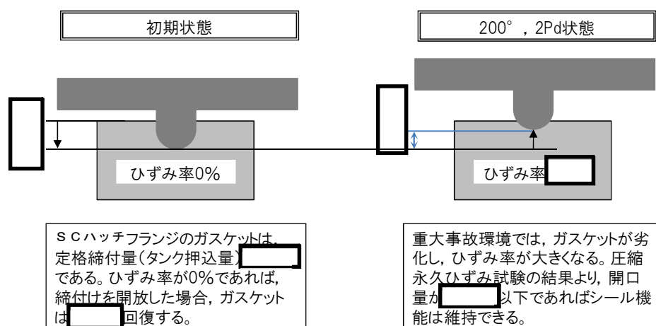
第 4-9 図 ひずみ率と許容開口量関係図
