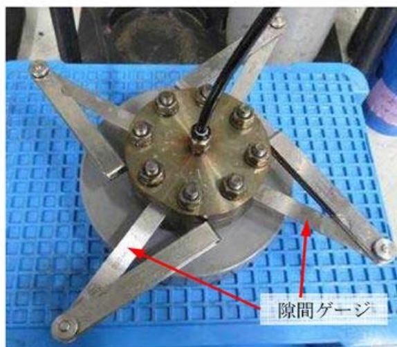
第6図 He 気密試験時開口模擬 (隙間ゲージ使用)
