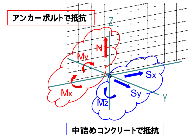
接合部の荷重分担(本震時の例)
