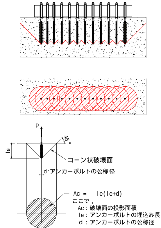
定着部コーン破壊照査における 有効水平投影面積
