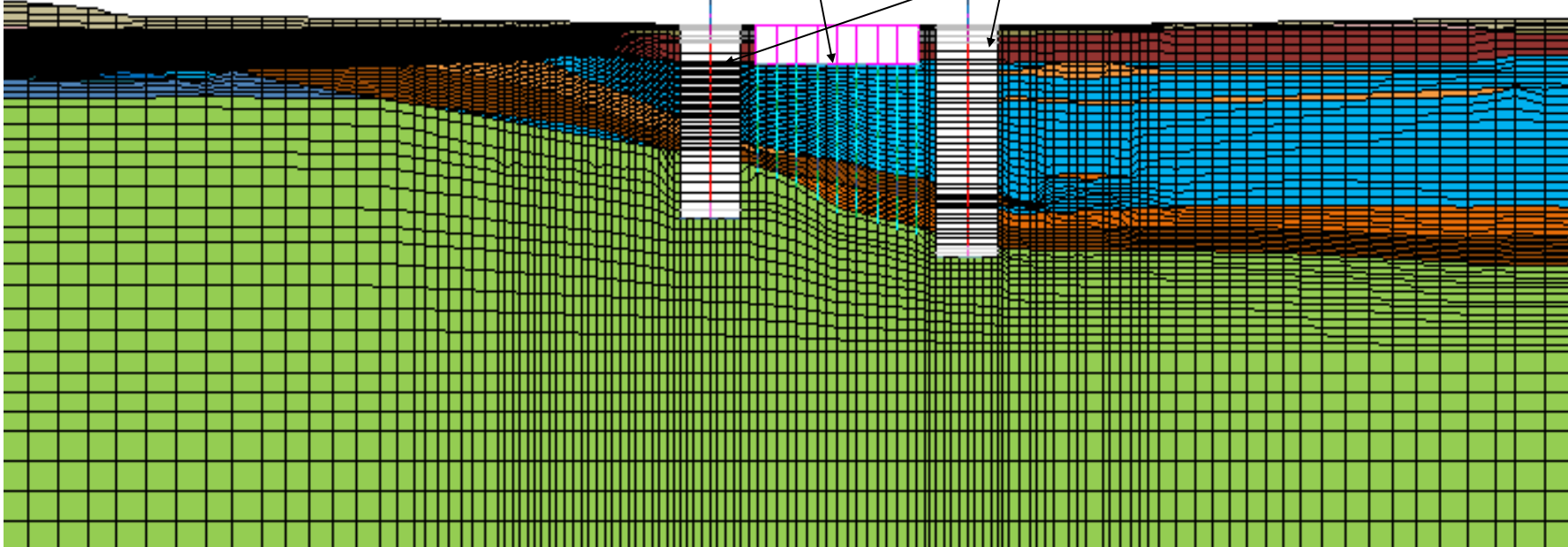
【解析モデル】 (A-A 断面)
