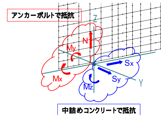
接合部の荷重分担(本震時の例)
