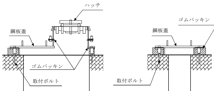
(A-A断面：ハッチ部)
