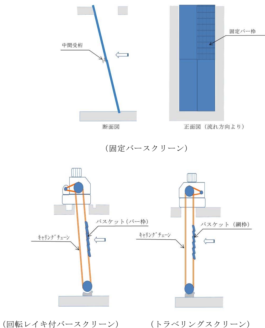
図 2.5-33 図 除塵装置概略構造
