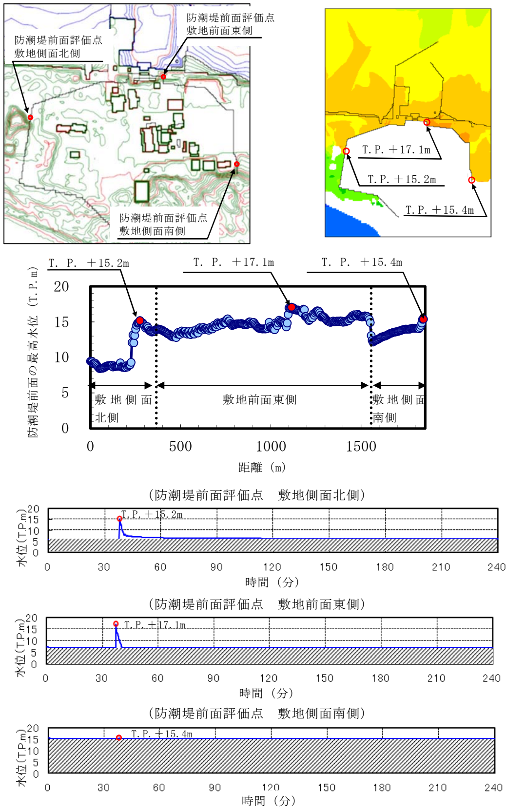
第1.4-2図 基準津波による防潮堤前面における上昇側水位の評価結果 (防波堤の有無による影響) (1/2)
