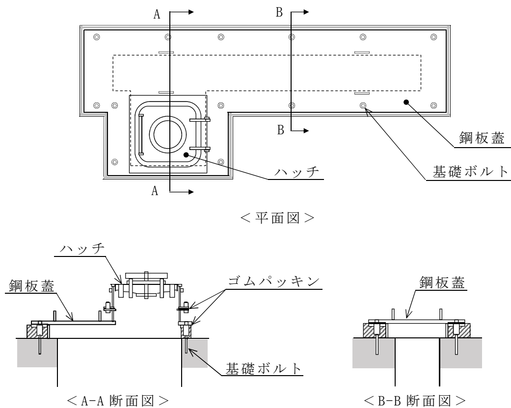
第 10.6-9 図 放水路ゲート点検用開口部浸水防止蓋概念図
