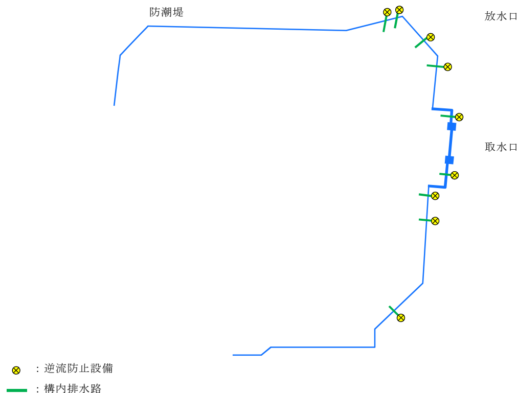
第1.4-11図 構内排水路逆流防止設備の配置
