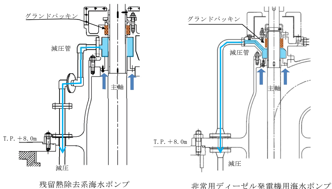
図 2.3-8 非常用海水ポンプグラント減圧配管の概要
