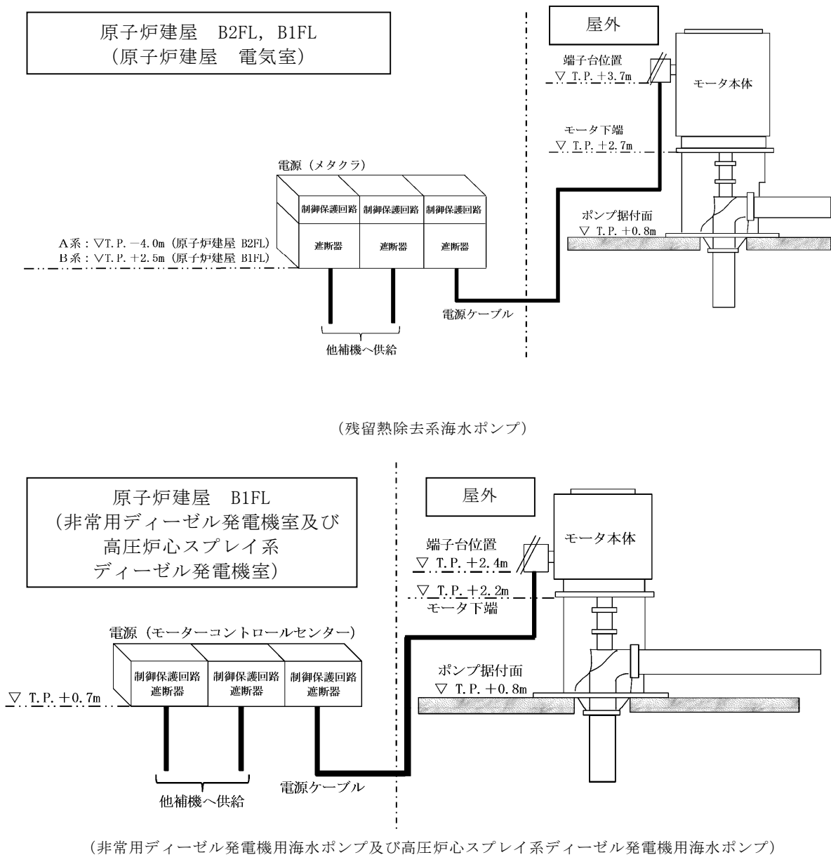
第 2.3-4 図 非常用海水ポンプの位置関係図
