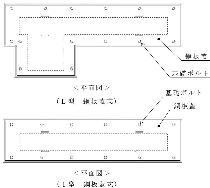
第 10.6-6 図 取水路点検用開口部浸水防止蓋概念図
