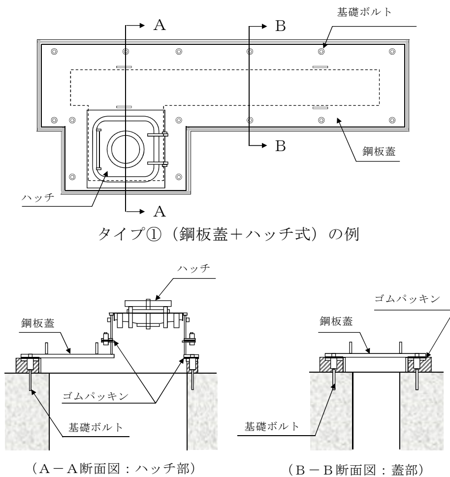
第 2.2-13 図 取水路点検用開口部浸水防止蓋構造図
