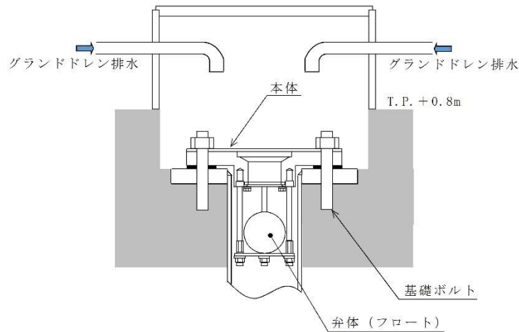
第 2.3-5 図 海水ポンプグランドドレン排出口逆止弁構造図
