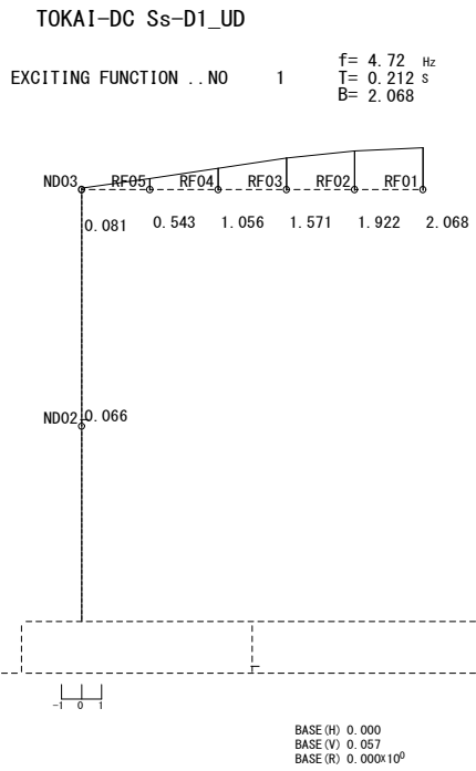
図4-1 (3/3) 刺激関数 (S s -D1, UD方向)
