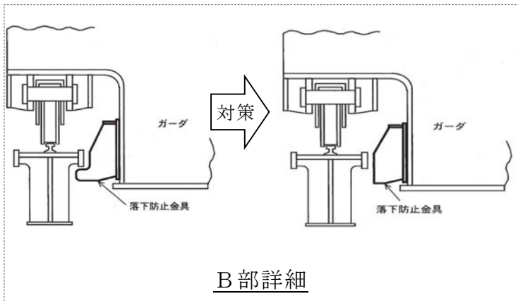
第3図 原子炉建屋クレーンの耐震補強概要図
