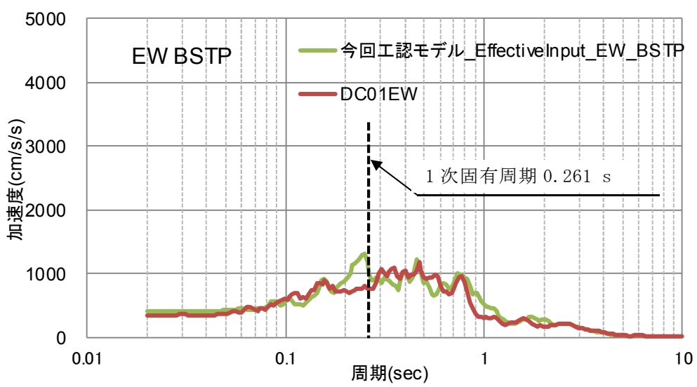
第2-1図 (2/3) 床応答スペクトルの比較 (EW方向, フレーム部, h = 5%)
