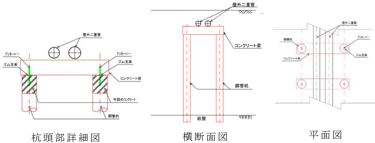
第 3-3-34 図 屋外二重管概念図 4条-別紙7-74
