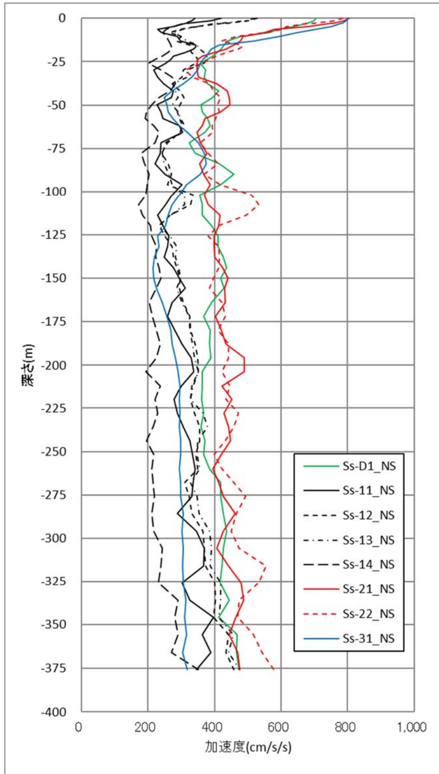
図 3-9 (1/3) 地盤応答解析結果 (N S 方向)
