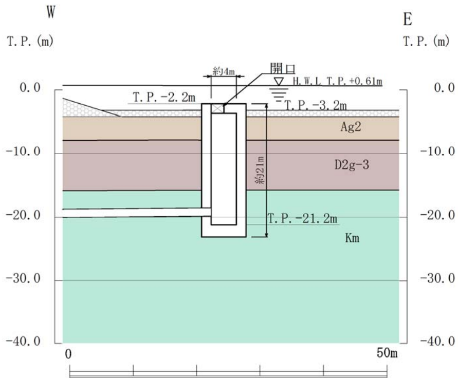
第 2.12-2 (1) 図 SA用海水ピット取水塔 断面図 (①-①断面)
