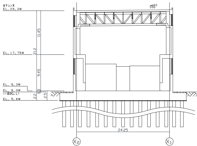
(EW方向, B-B断面)
