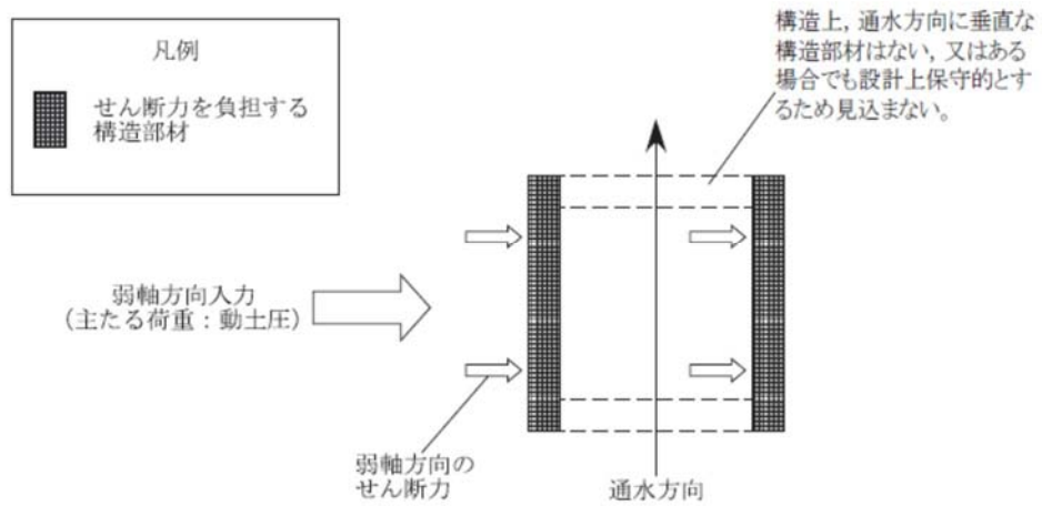
第3-4-2図 従来設計手法の考え方
