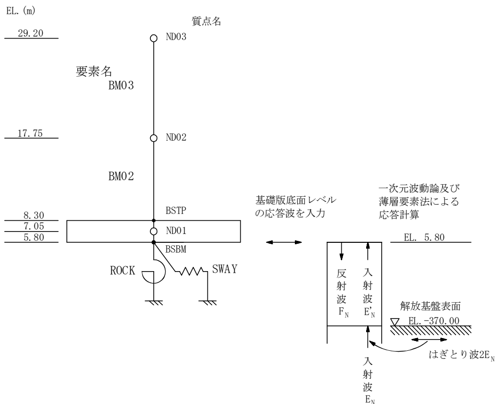
図 3-1 地震応答解析モデル (NS 方向)
