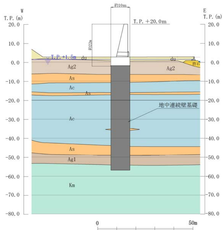
第 1.5-10 (3) 図 鉄筋コンクリート防潮壁 断面図(F-F 断面)
