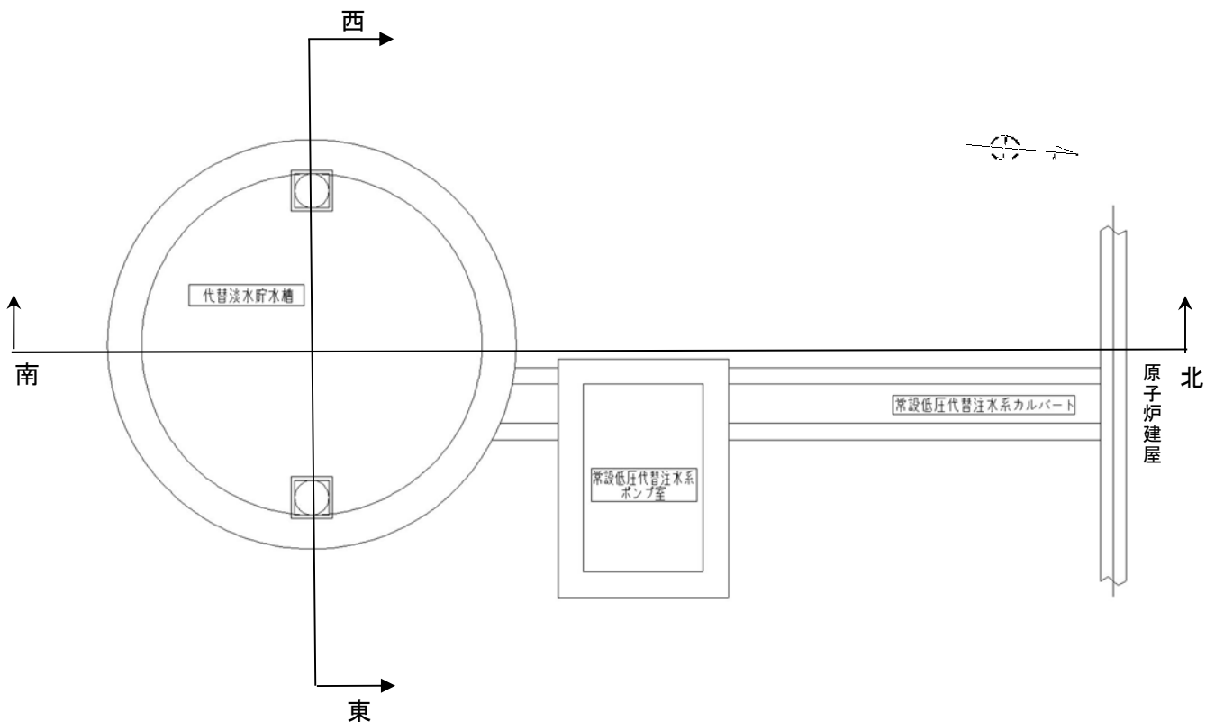
第 2.4-1 図 代替淡水貯槽 平面図
