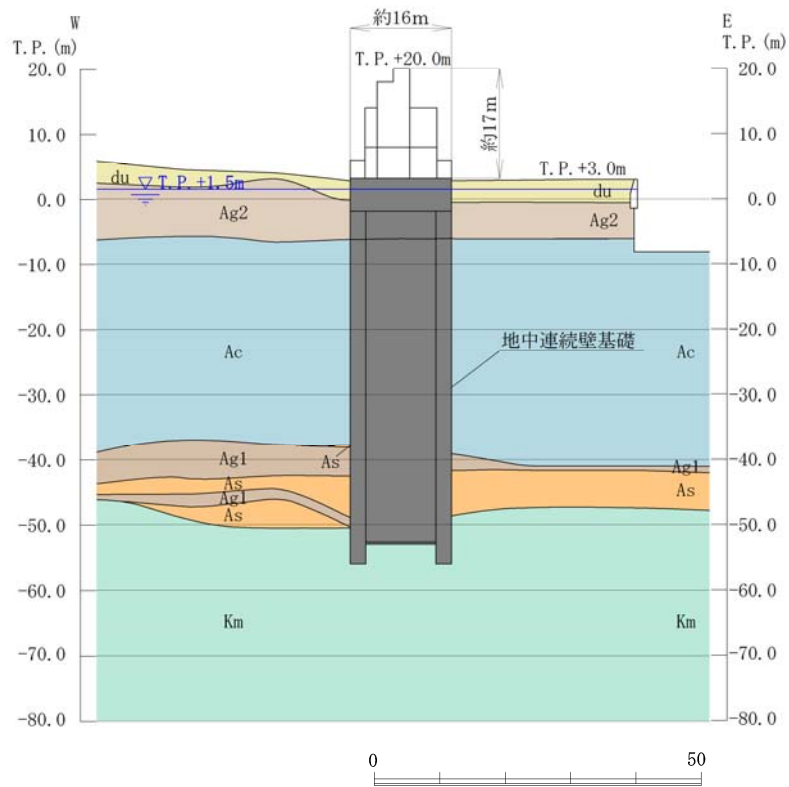
第 1.5-8 (2) 図 鋼製防護壁 断面図 (B-B 断面)
