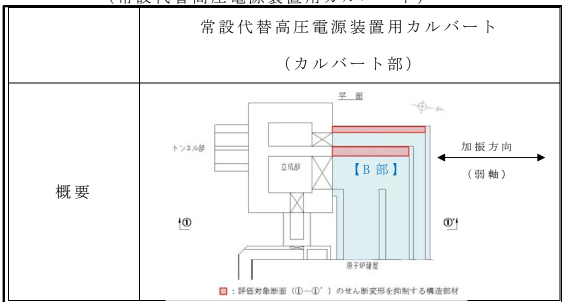
第3-3-4表 屈曲部における3次元的な拘束効果 （常設代替高圧電源装置用カルバート）
