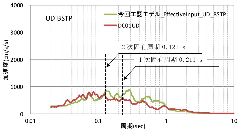
第2-1図 (3/3) 床応答スペクトルの比較 (上下方向, h = 5\% )
