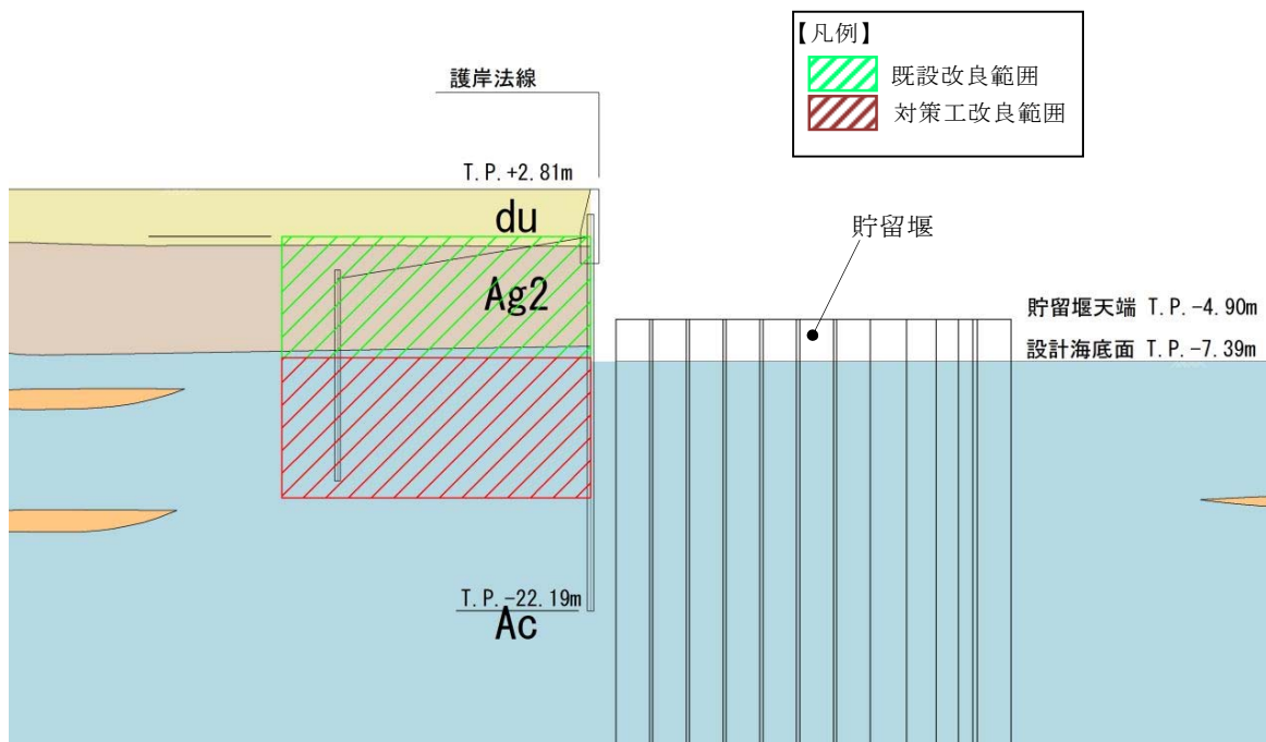
第9図 貯留堰取付護岸の耐震補強概要図
