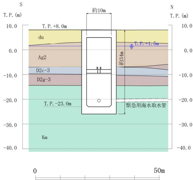
第 2.10-2 (2) 図 SA用海水ピット 断面図 (②-②断面)
