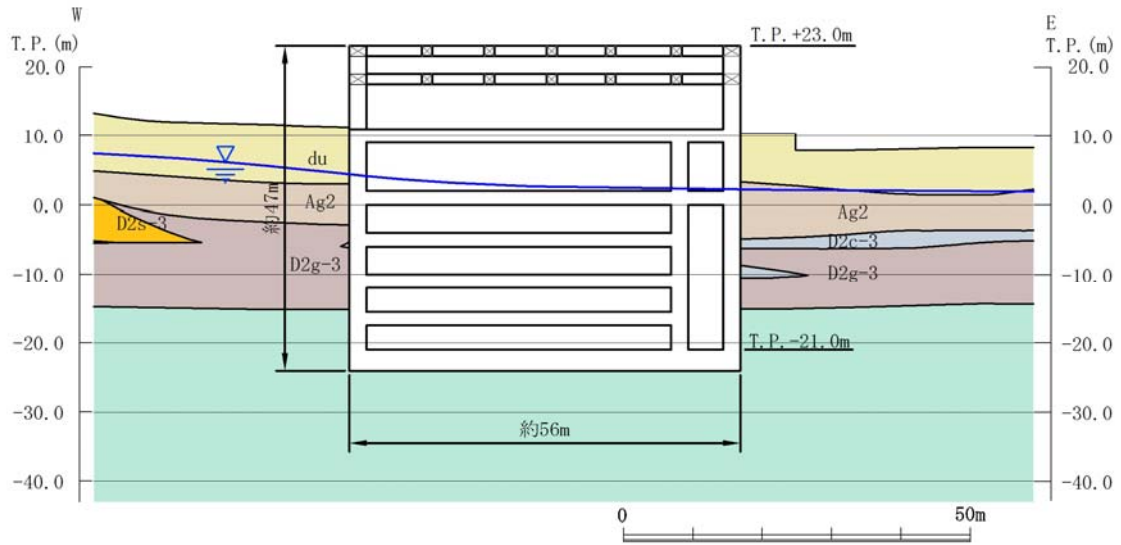
第 2.2-2 (1) 図 常設代替高压電源装置置場 断面図 (東西断面)
