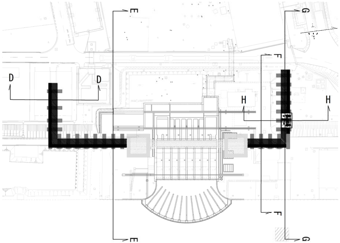
第 1.5-9 図 鉄筋コンクリート防潮壁 平面図
