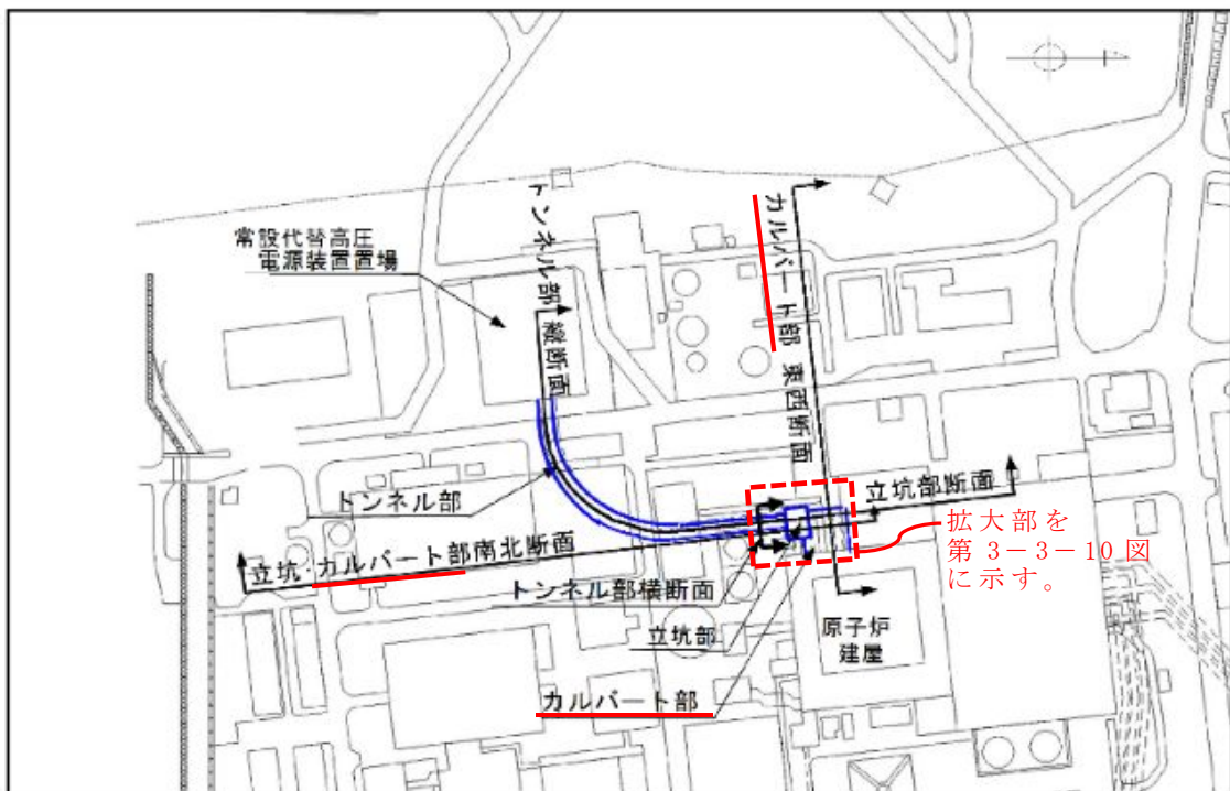
第 3-3-9 図 常設代替高圧電源装置用カルバート配置図
