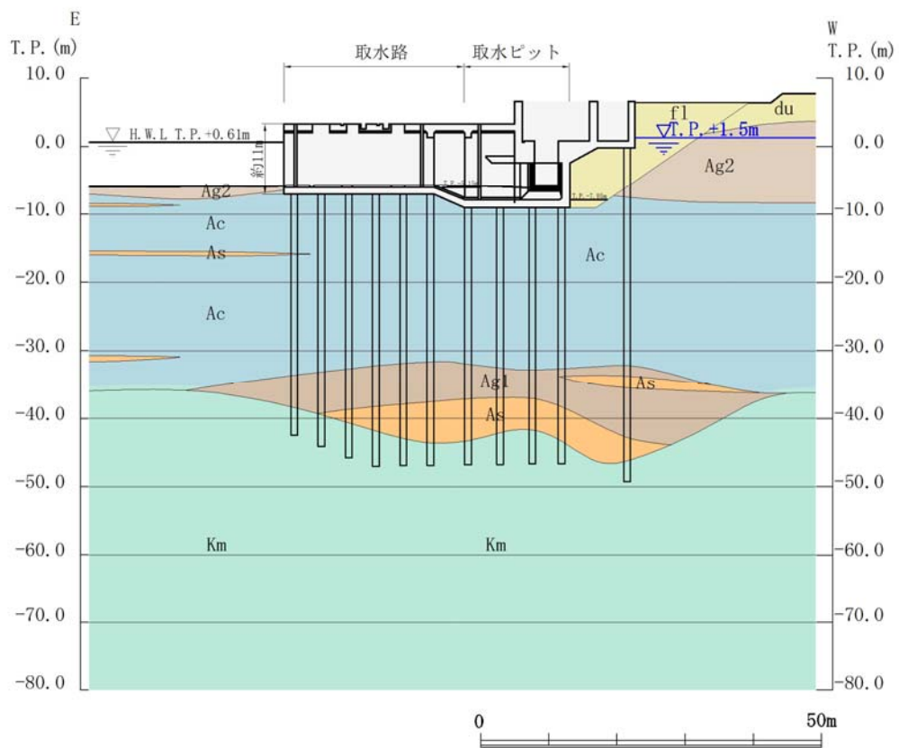
第 1.2-2 図 取水構造物 縦断面図 (A-A 断面)
