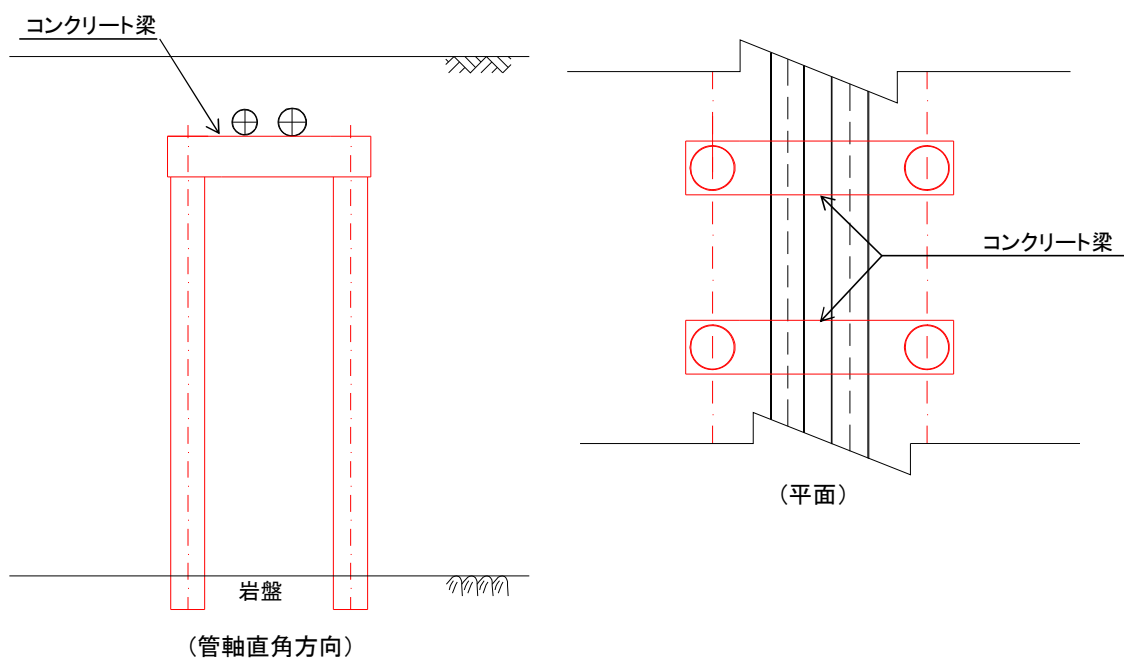
第 8 図 コンクリート梁イメージ図
