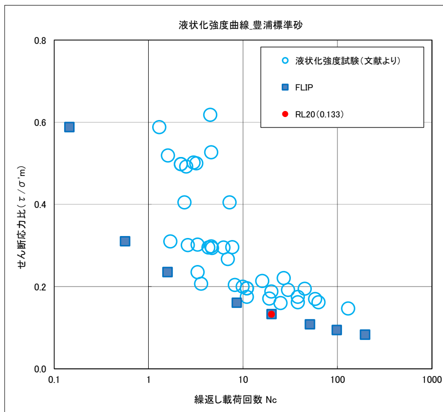
第 7.1.2 図 FLIP による十分に豊浦標準砂の保守的な液状化強度特性 ( -1\sigma )
