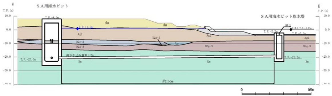
第 2.11-2 図 海水引込み管 縦断面図
