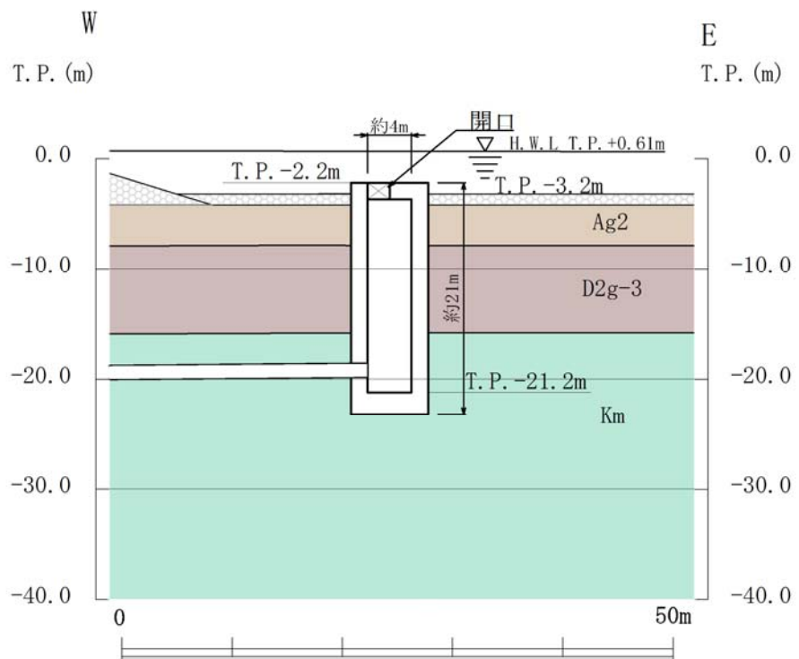
第 2.12-2 (2) 図 SA用海水ピット取水塔 断面図 (②-②断面)
