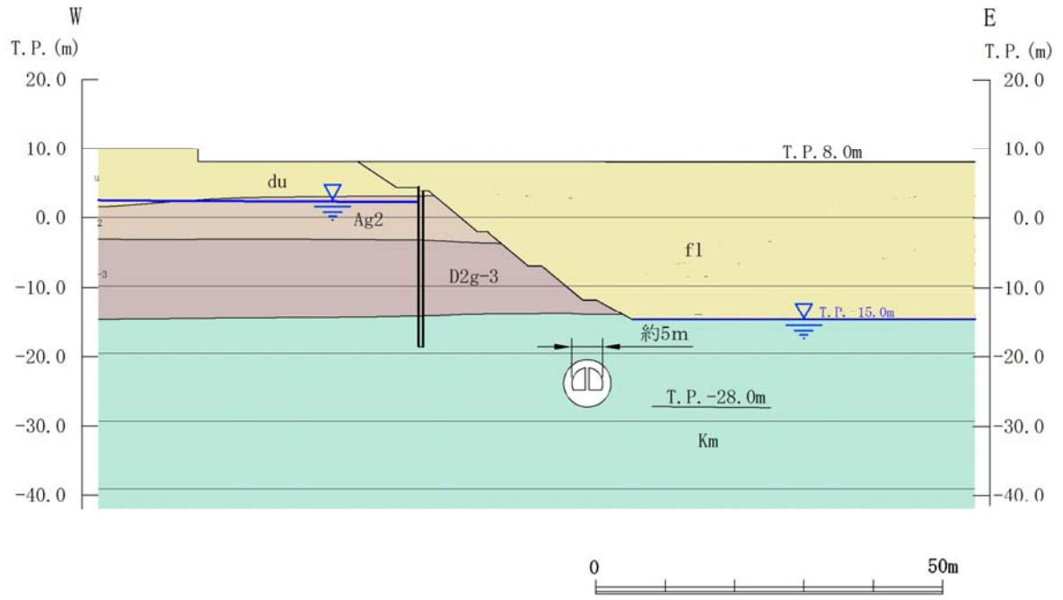
第 2.3-3 図 常設代替高圧電源装置用カルバート（トンネル部） 横断面図
