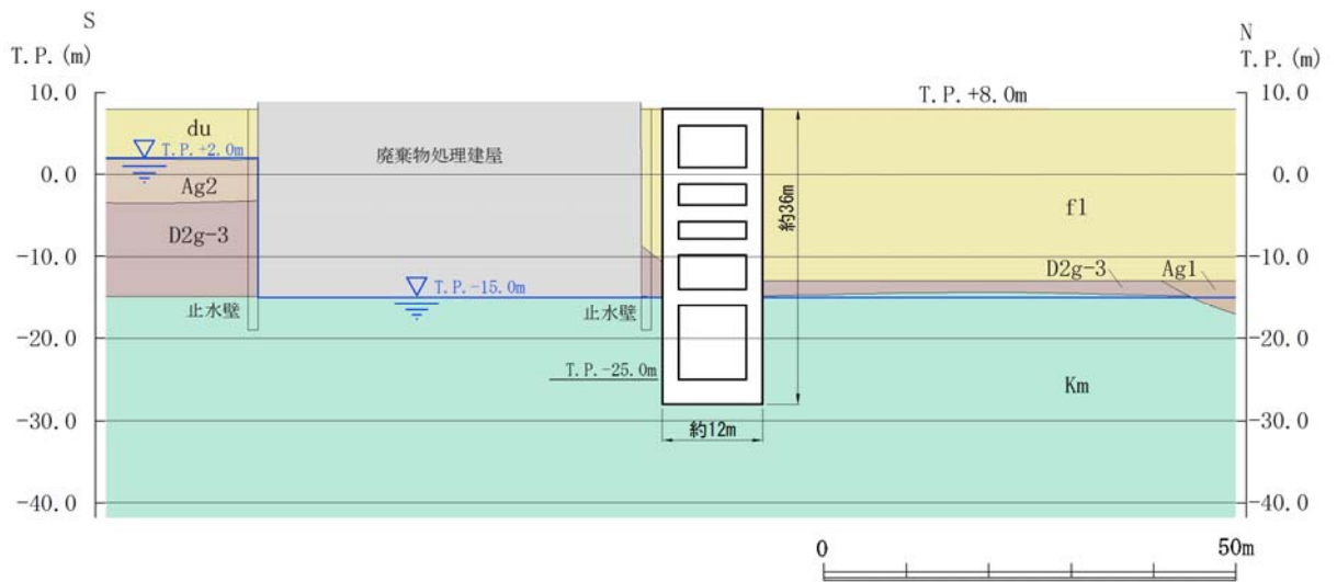
第 2.7-2 (2) 図 緊急用海水ポンプピット 断面図 (南北断面)
