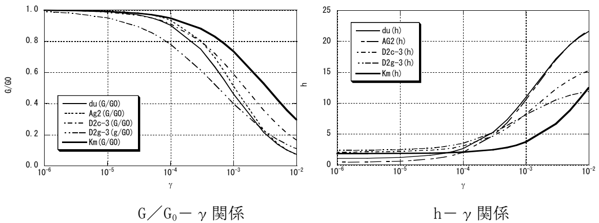
図 3-8 使用済燃料乾式貯蔵建屋 地盤の非線形特性
