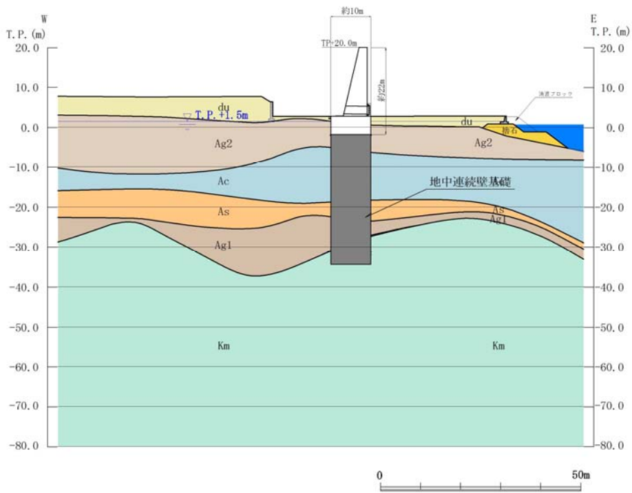
第 1.5-10 (2) 図 鉄筋コンクリート防潮壁 断面図(E-E 断面)
