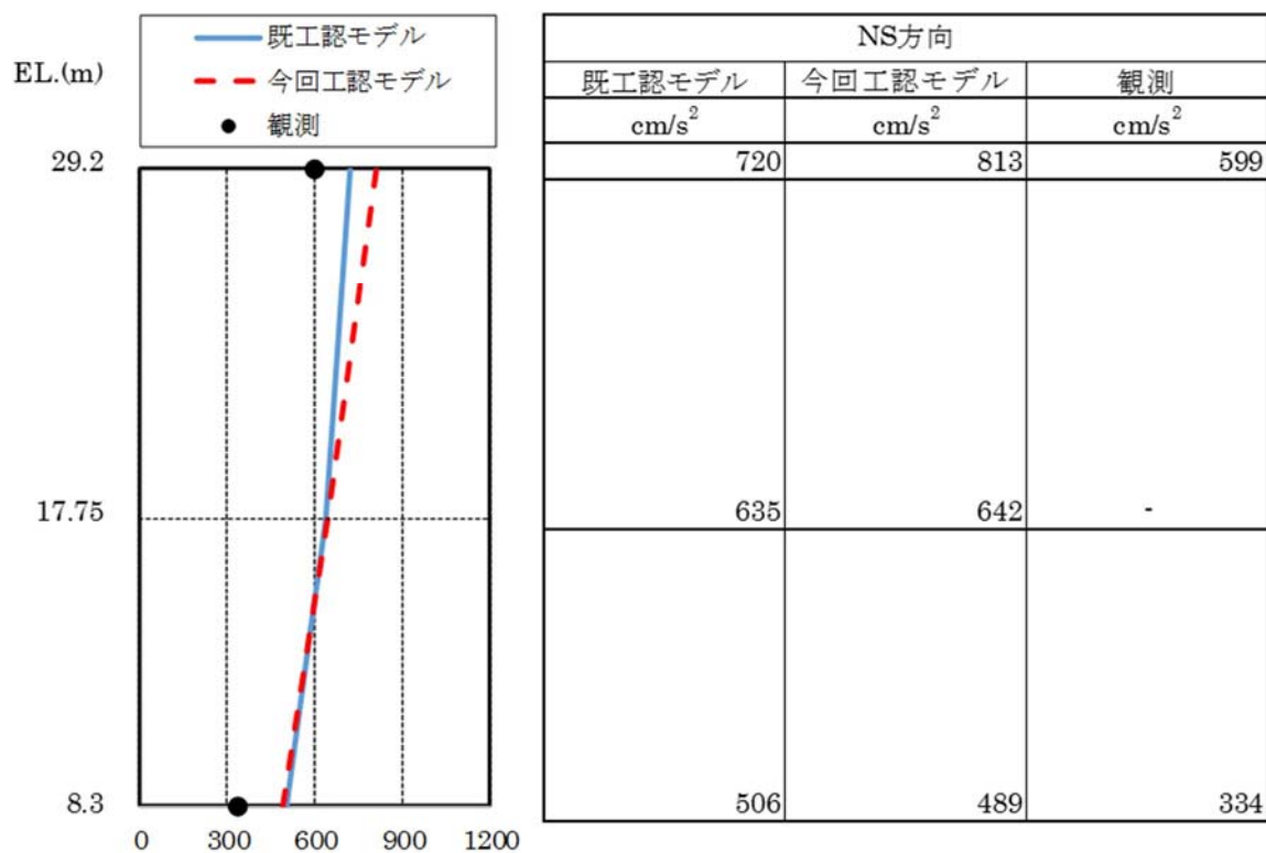
第2-3図 (1/3) 最大応答加速度分布の比較 (NS方向)
