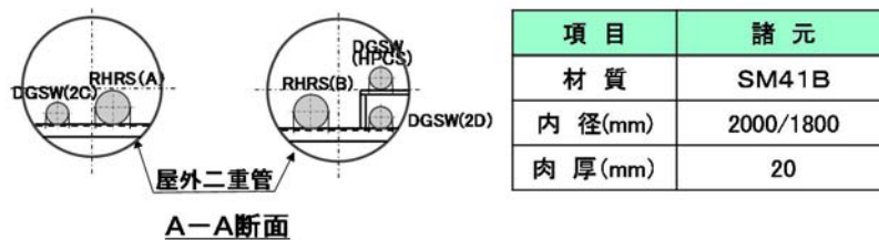
第 2 図 屋外二重管の平面位置図及び断面図
