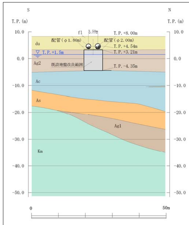
第 1.3-3 図 (2) 屋外二重管 横断面図 (C-C 断面)
