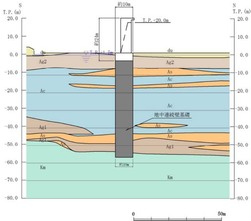
第 1.5-10 (5) 図 鉄筋コンクリート防潮壁 断面図(H-H 断面)
