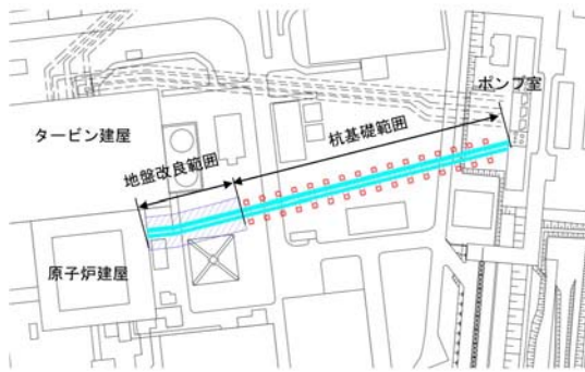
基礎平面配置図
