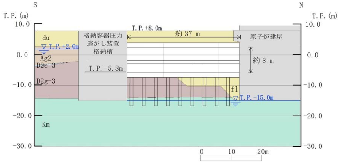
第 2.8-2 図 格納容器圧力逃がし装置用配管カルバート 縦断面図 (A-A断面)
