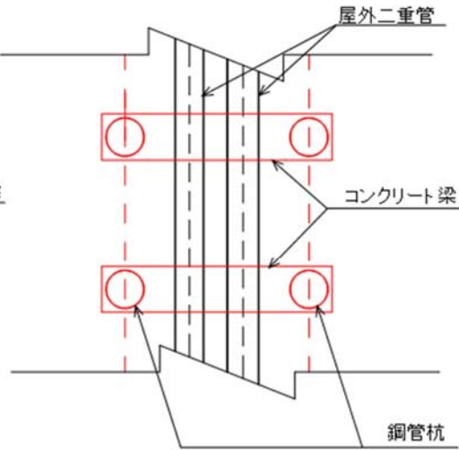
基礎縦断配置図
