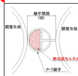
第3-4-8図 貯留堰
