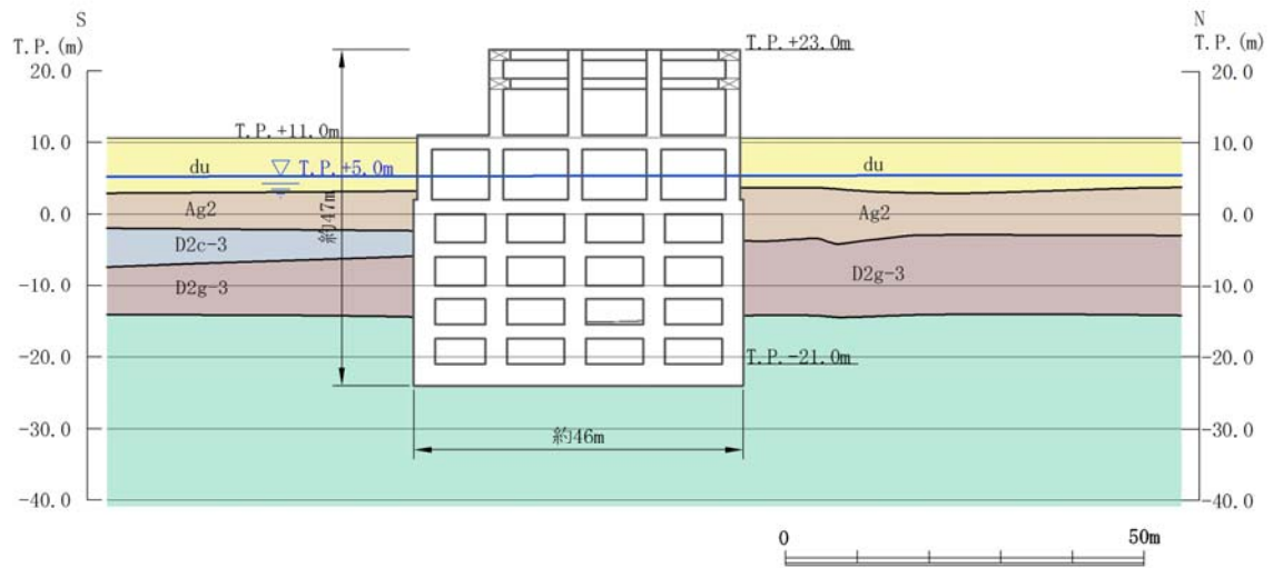
第 2.2-2 (2) 図 常設代替高压電源装置置場 断面図 (南北断面)
