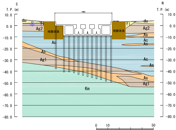
横断面図 (B-B断面：取水ピット)
