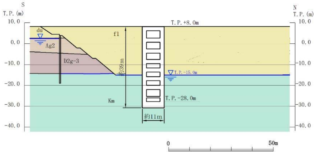
第 3-3-23 図 常設代替高压電源装置用カルバート（立坑部）断面図
