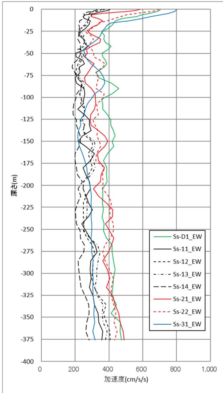
図 3-9 (2/3) 地盤応答解析結果 (EW方向)
