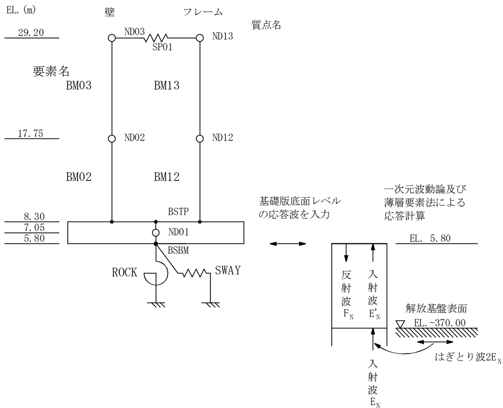
図3-2 地震応答解析モデル (E W方向)
