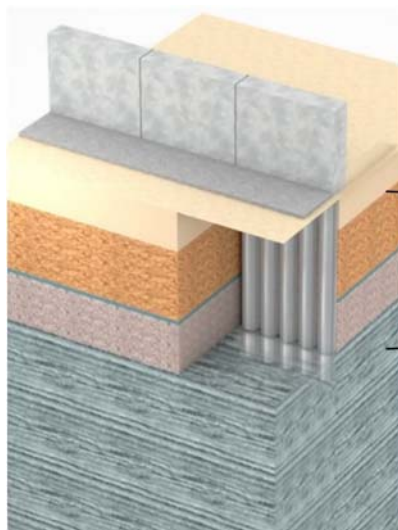
第3-4-12 図 鋼管杭鉄筋コンクリート防潮壁の下部工
