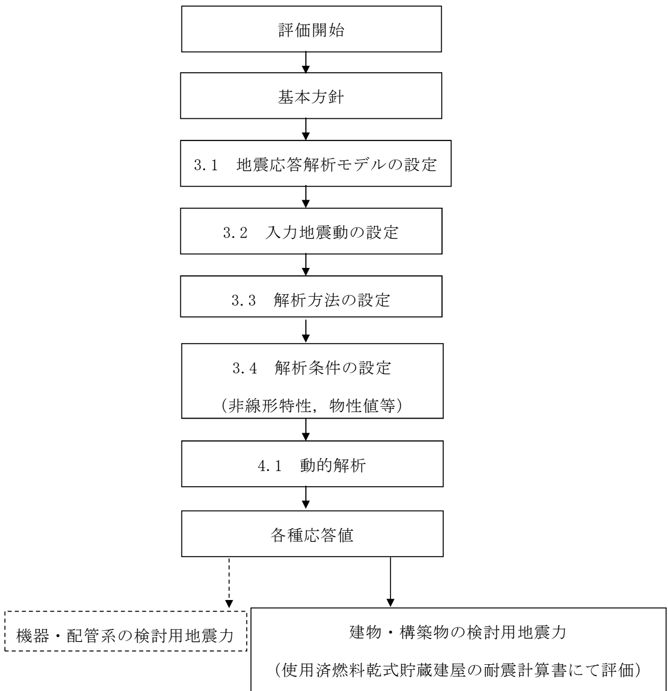
図 2-4 使用済燃料乾式貯蔵建屋の地震応答解析フロー
