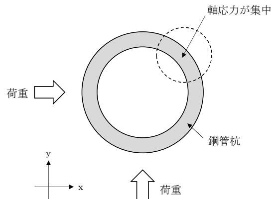
第3-4-13 図 鋼管杭基礎に係る応答特性
