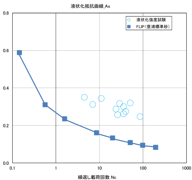
(b) 全ての試験データを保守側に包含する
