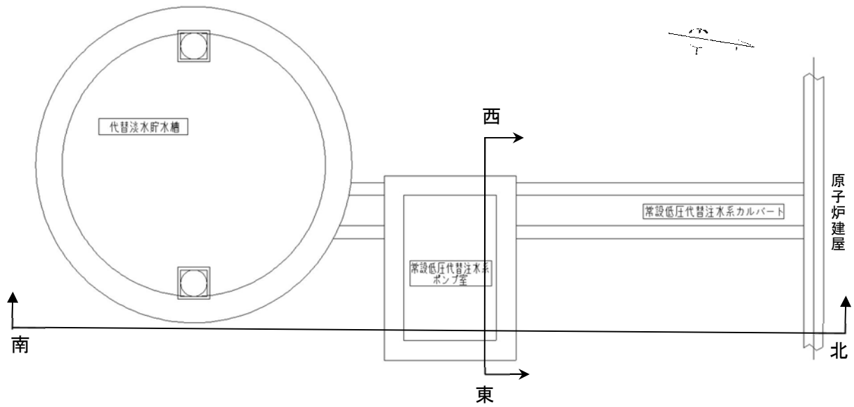
第 2.5-1 図 常設低圧代替注水系ポンプ室 平面図
