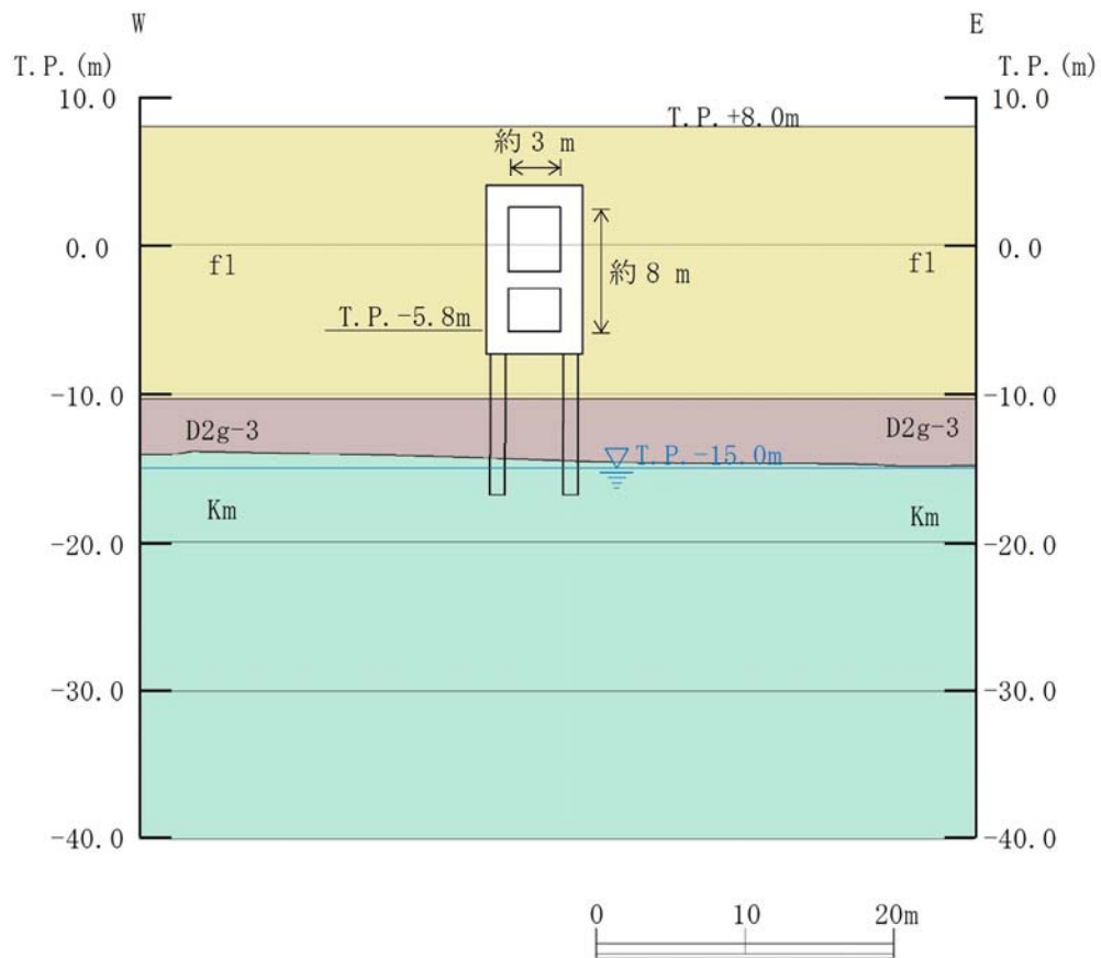
第 2.8-3 (1) 図 格納容器圧力逃がし装置用配管カルバート 断面図 (B-B断面)
