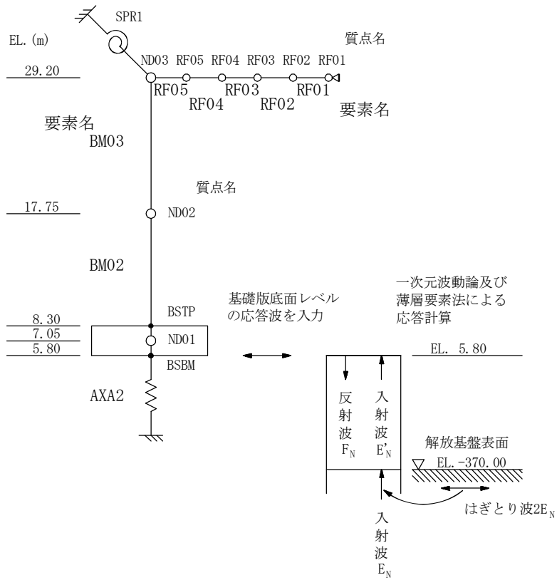
図3-3 地震応答解析モデル (鉛直方向)
