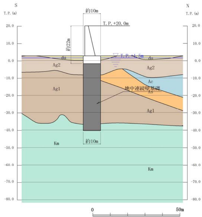
第 1.5-10 (1) 図 鉄筋コンクリート防潮壁 断面図(D-D 断面)
