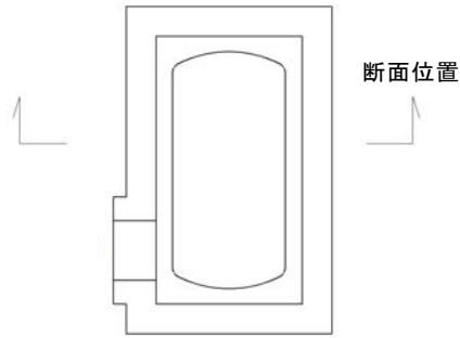
第 2.13-1 図 緊急時対策所用発電機燃料油貯蔵タンク基礎 平面図
