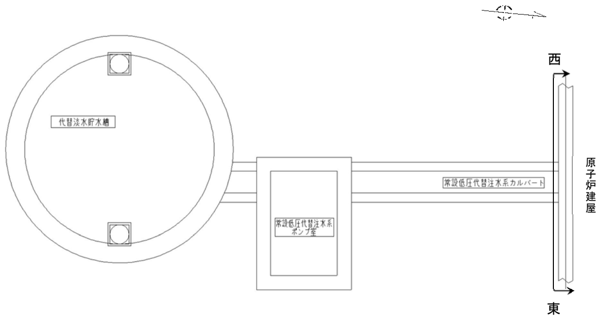
第 2.6-1 図 常設低圧代替注水系配管カルバート 平面図
