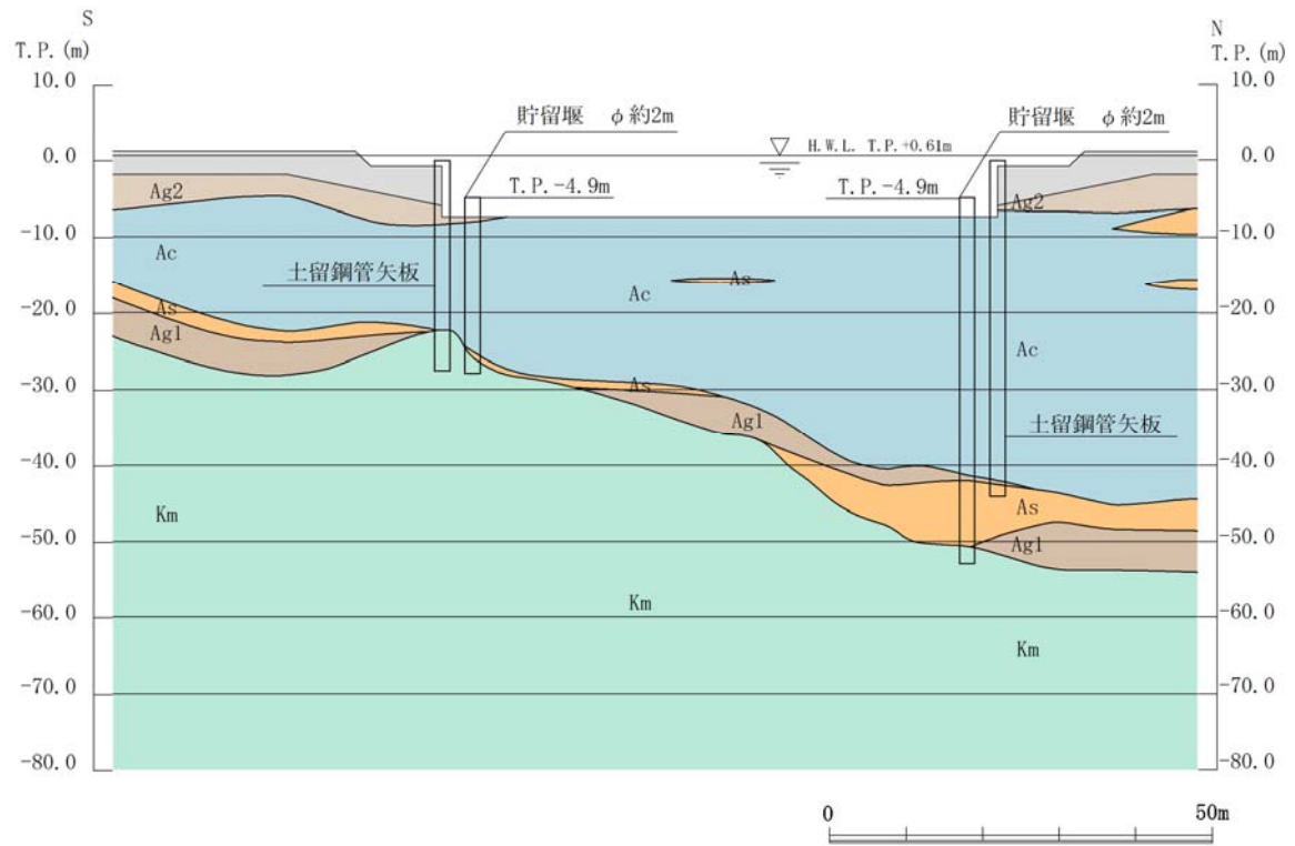
第 1.4-2 (3) 図 貯留堰 断面図 (NS-1 断面)
