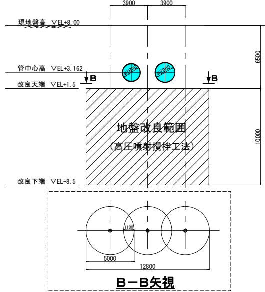
第 3 図 地盤改良範囲（既施工）説明図
