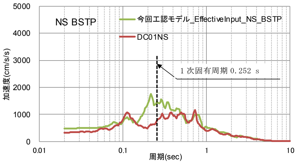
第2-1図 (1/3) 床応答スペクトルの比較
