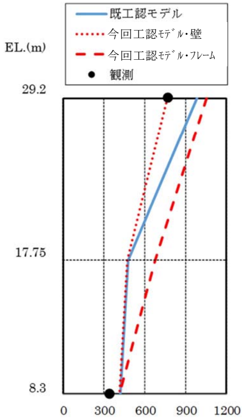
第2-3図 (2/3) 最大応答加速度分布の比較 (EW方向)
