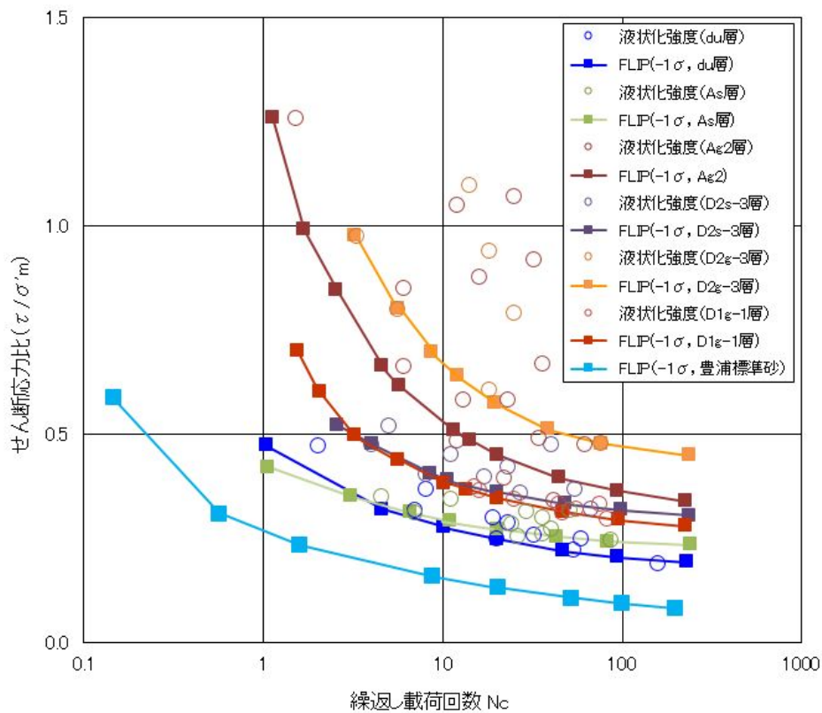
第 4.3.3 図 東海第二発電所の原地盤に基づく液状化強度試験データとその全てを保守側で包含する F L I P の液状化強度特性（豊浦標準砂）
