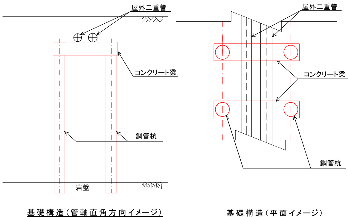
第5図 屋外二重管の基礎構造概要図
