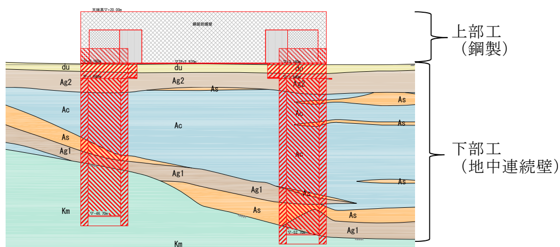
第 3-4-9 図 鋼製防護壁の下部工
