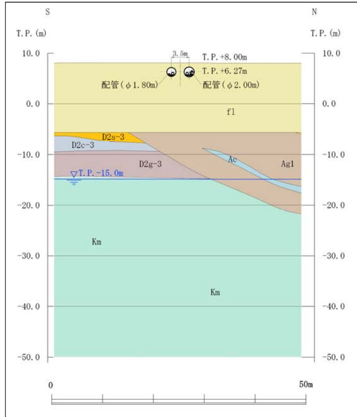
第 1.3-3 図 (1) 屋外二重管 横断面図 (B-B 断面)
