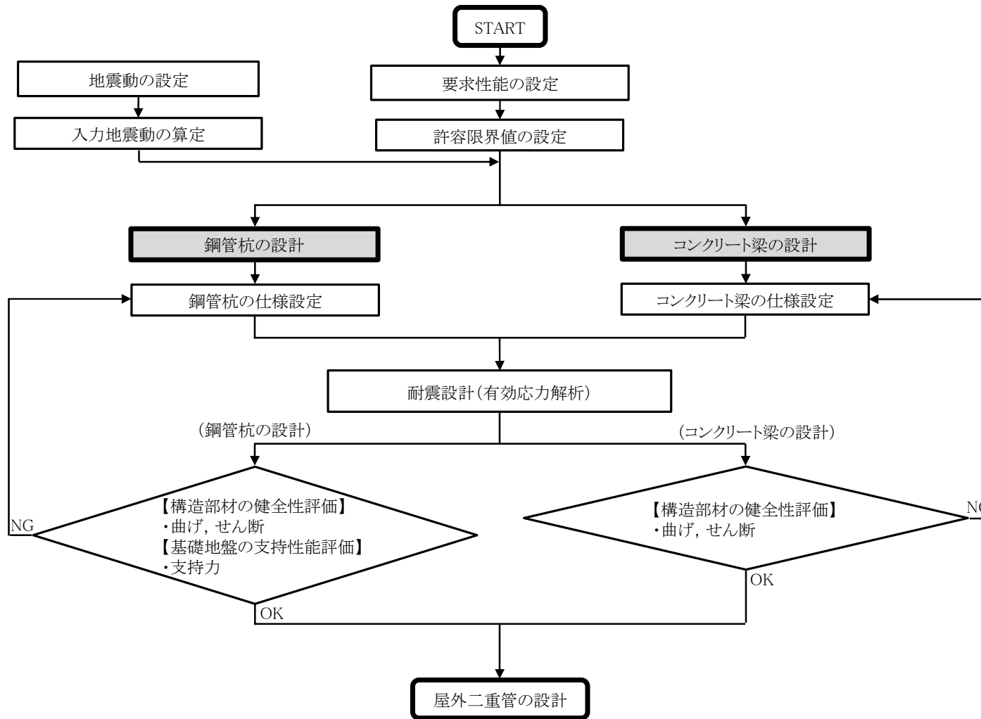
第6図 屋外二重管の基礎構造の構造健全性及び支持性能評価の検討フロー
