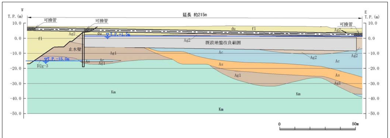
第 1.3-2 図 屋外二重管 縦断面図 (A-A断面)
