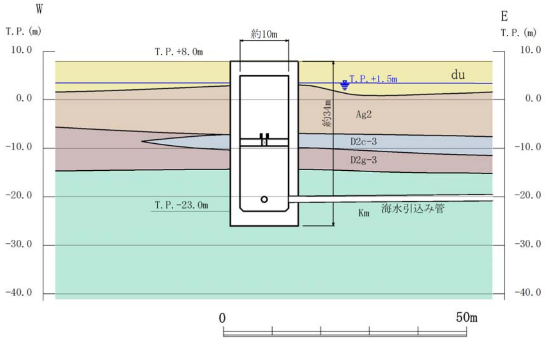
第 2.10-2 (1) 図 SA用海水ピット 断面図 (①-①断面)
