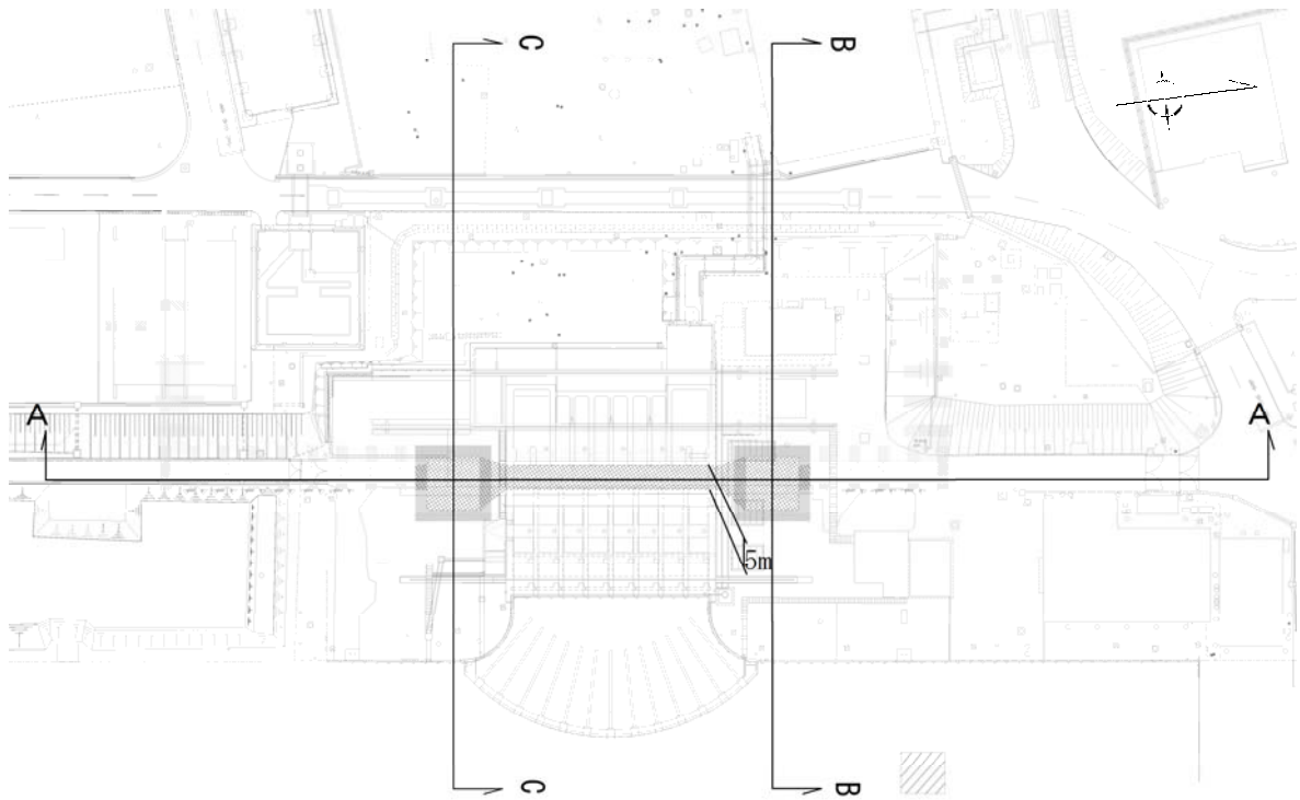
第 1.5-6 図 鋼製防護壁 平面図
