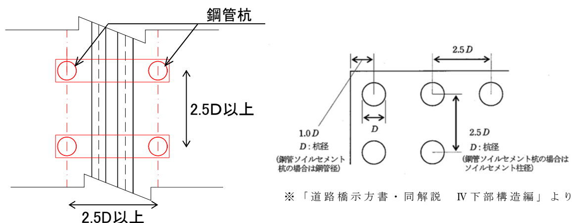
第 7 図 杭の最小中心間隔
