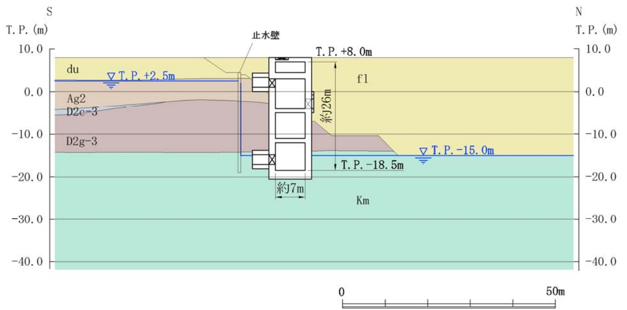
第 2.5-2 (2) 図 常設低圧代替注水系ポンプ室 断面図 (南北断面)
