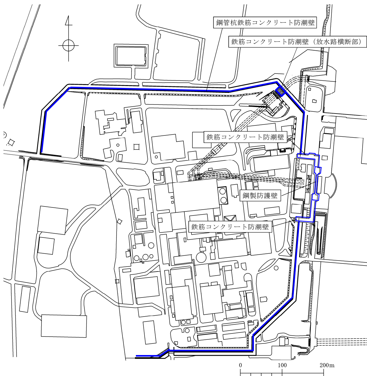
第 1.5-1 図 防潮堤 平面図
