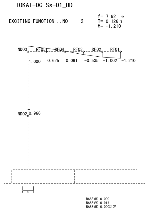
図4-1 (3/3) 刺激関数 (S s -D1, UD方向)
