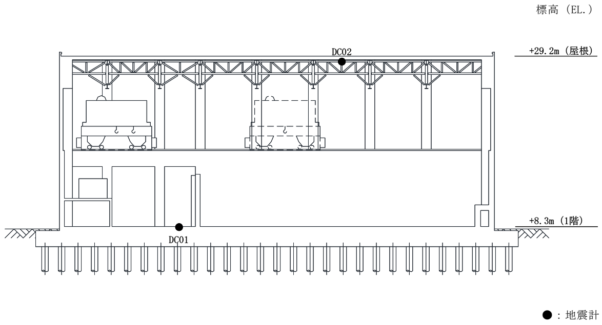
(a) 断面図
