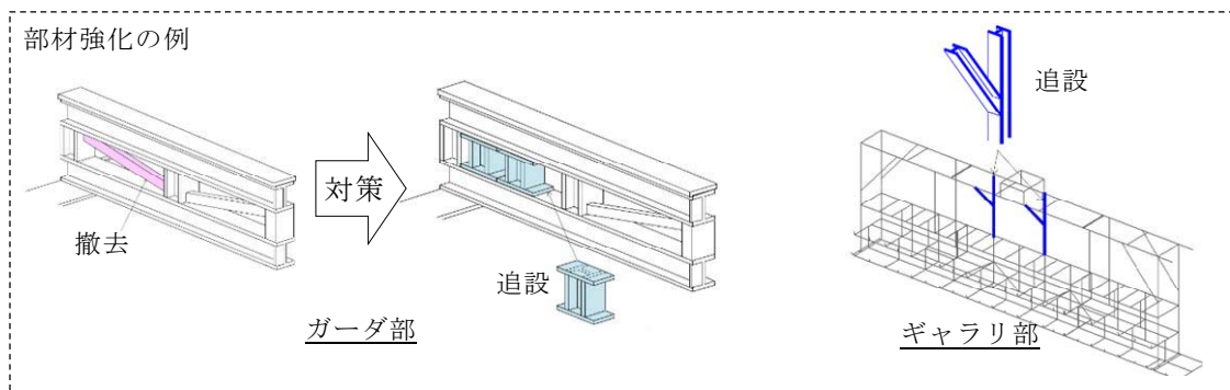
第3図 原子炉建屋クレーンの耐震補強概要図
