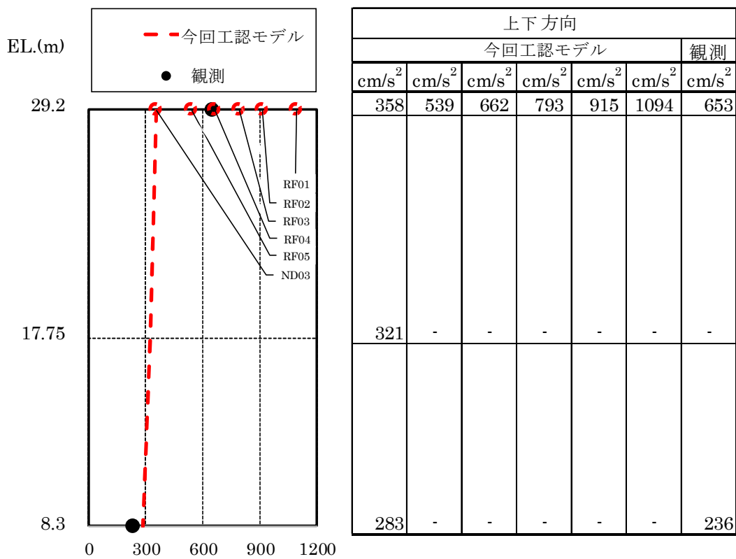
第2-3図 (3/3) 最大応答加速度分布の比較 (上下方向)
