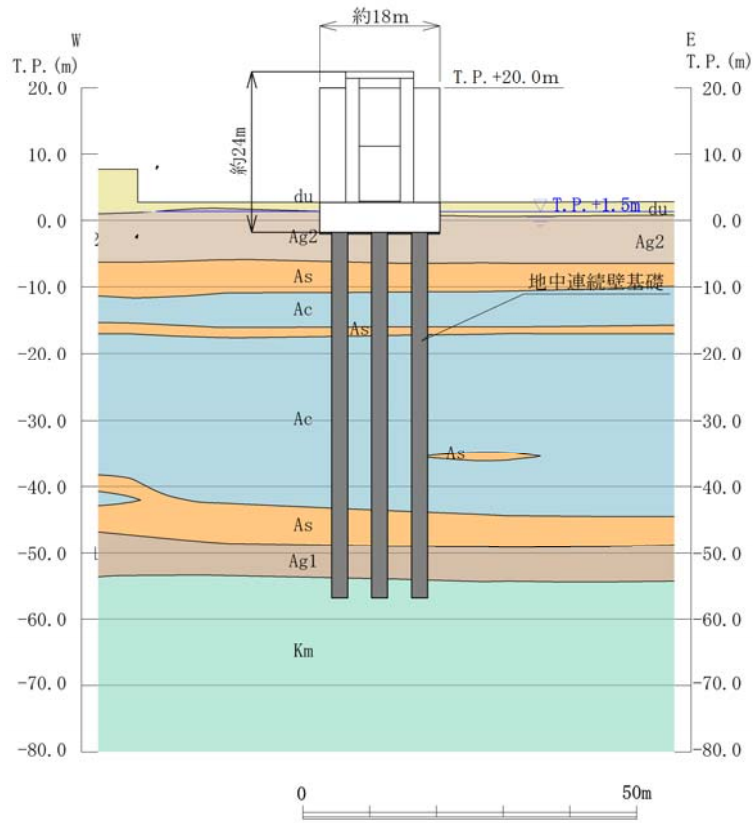
第 1.5-10 (4) 図 鉄筋コンクリート防潮壁 断面図(G-G 断面)
