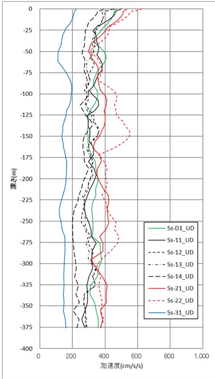
図 3-9 (3/3) 地盤応答解析結果 (UD方向)
