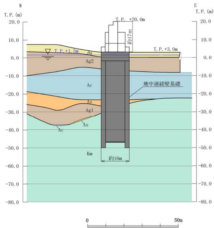
第 1.5-8 (2) 図 鋼製防護壁 断面図 (C-C 断面)
