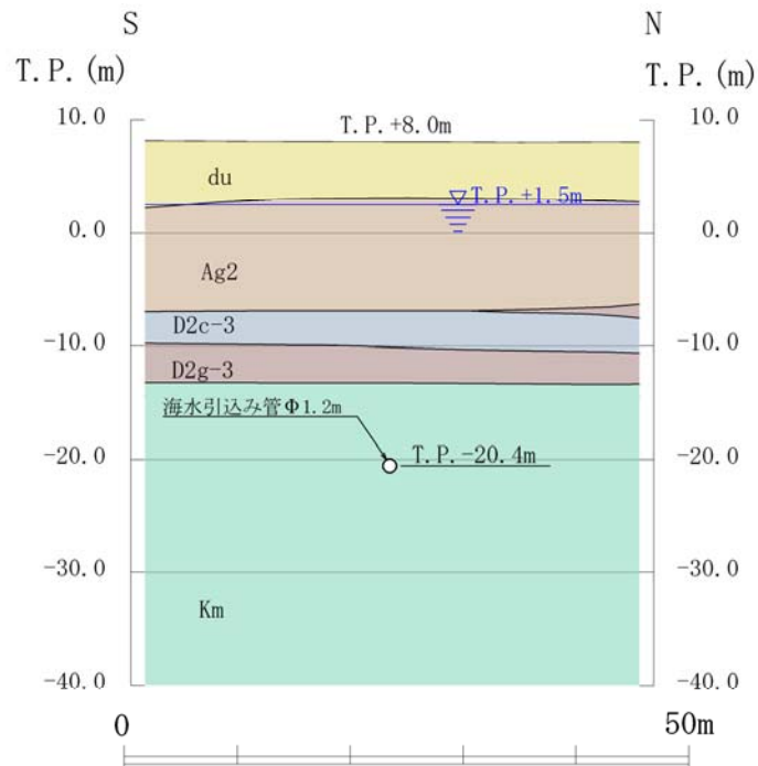
第 2.11-3 図 海水引込み管 横断面図 (A-A断面)
