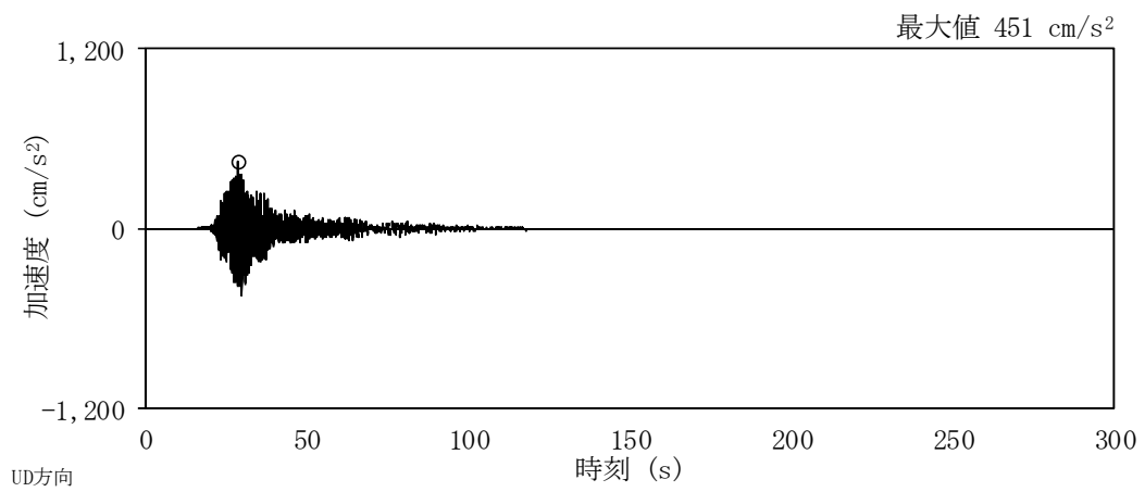
(c) UD方向
