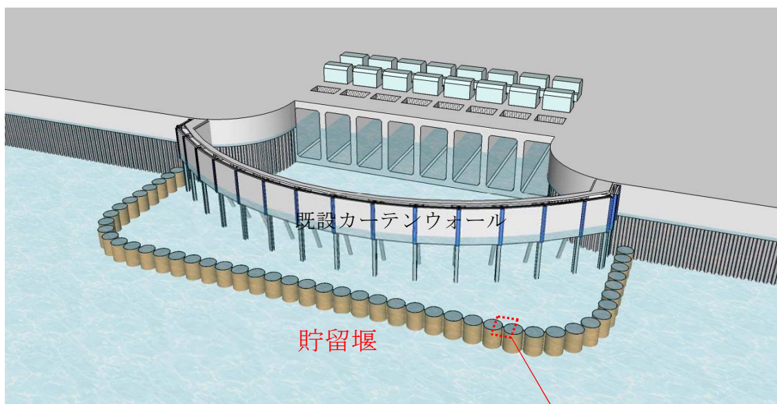
第3-4-8図 貯留堰
