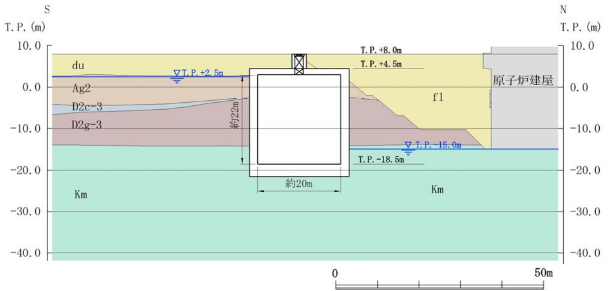
第 2.4-2 (1) 図 代替淡水貯槽 断面図 (東西断面)
