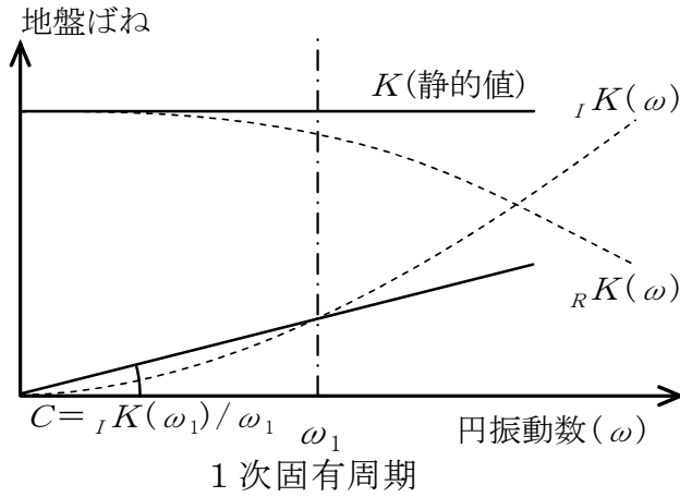
図3-4 底面地盤ばねの近似法
