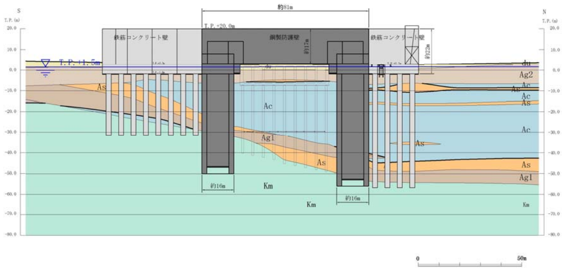
第 1.5-7 図 鋼製防護壁 正面図 (A-A 断面)
