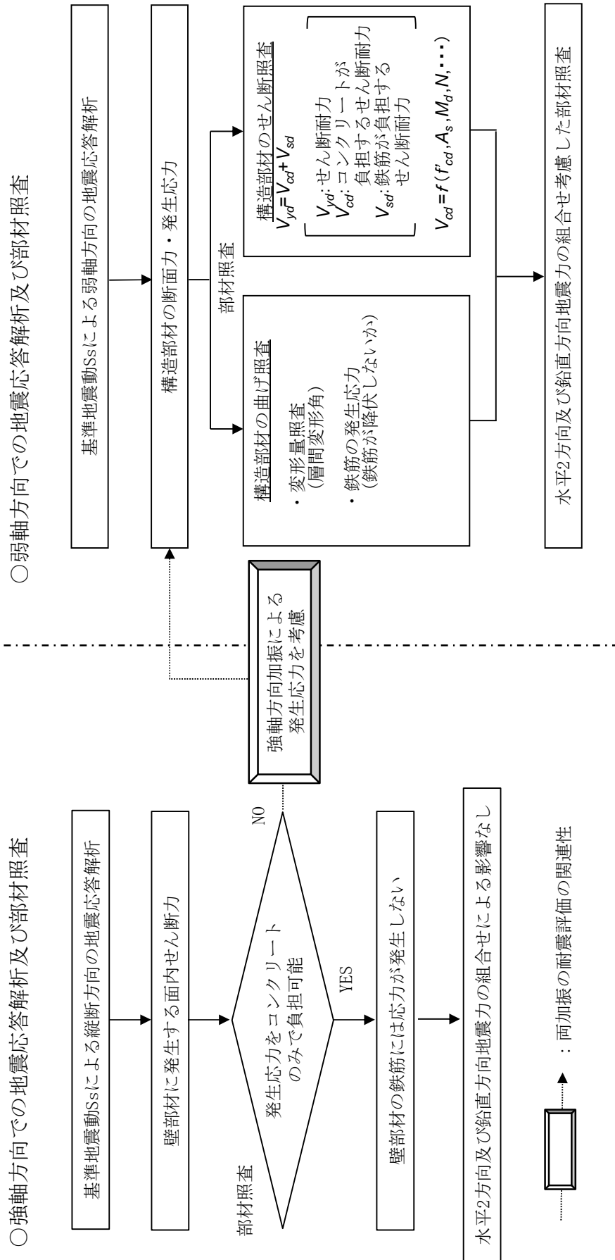
第 3-4-23 図 水平 2 方向及び鉛直方向地震力の組合せの評価フロー 4 条-別紙 7-113
