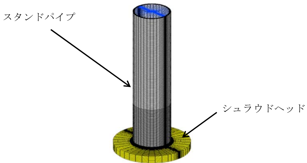
第 8-5 図 極限解析に用いる解析モデル概要図（中央位置）
