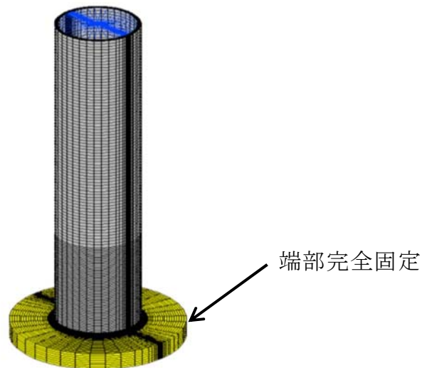
第 8-6 図 解析モデルの境界条件
