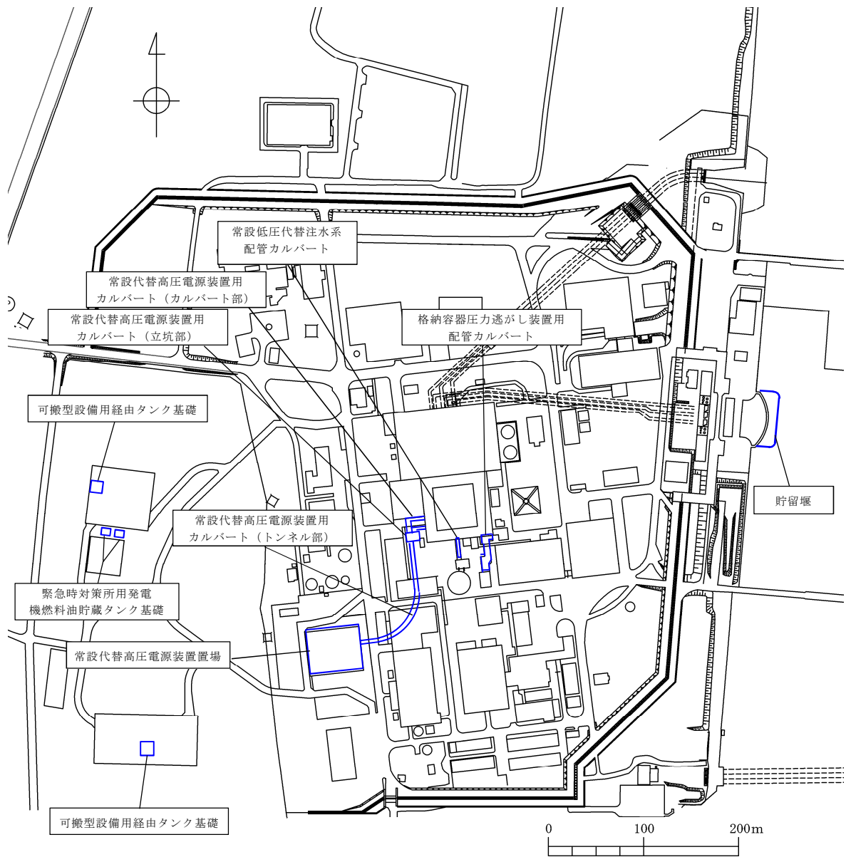
第6-1-1図 平面配置図
