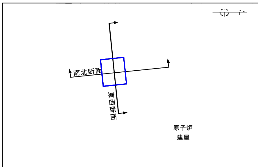
第6-3-1図 常設代替高圧電源装置置場 平面図
