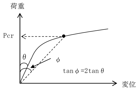
第 8-9 図 崩壊荷重の下限 (Pcr) の定義
