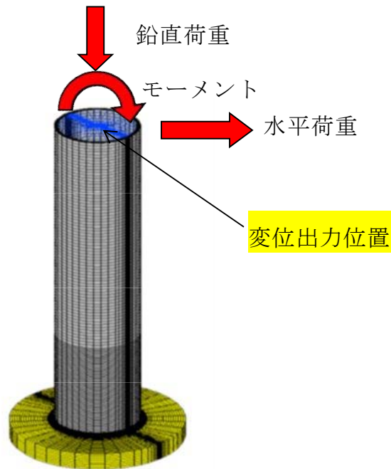
第 8-8 図 荷重の負荷
