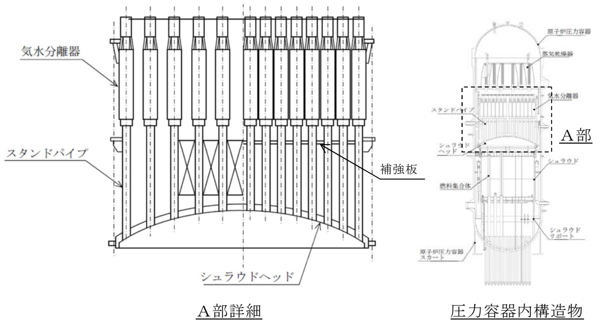
第 8-4 図 炉内構造物（気水分離器及びスタンドパイプ）構造概要図
