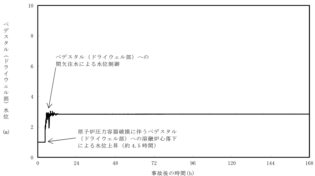
第10図 ペデスタル（ドライウエル部）の水位の推移（基本ケース）
