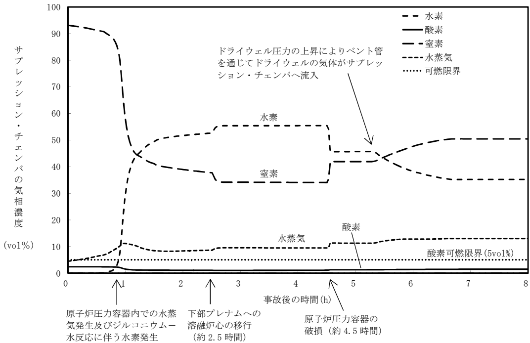
第 3.2-23 図 サブプレッション・チェンバの気相濃度の推移 (ウェット条件) (～8 時間)
