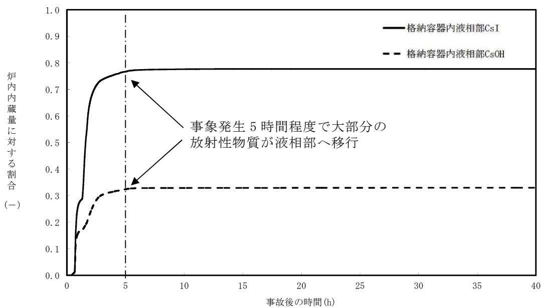
第 2 図 格納容器内液相部中の存在割合
