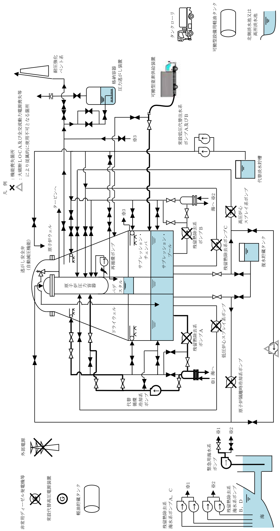
第 3.1.2-1 図 「雰囲気圧力・温度による静的負荷（格納容器過圧・過温破損）」の重大事故等対策の概略系統図（代替循環冷却系を使用する場合）（3/3）
