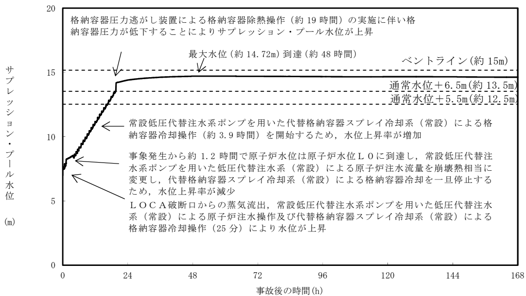
第 1 図 サプレッション・チェンバプール水位の推移
