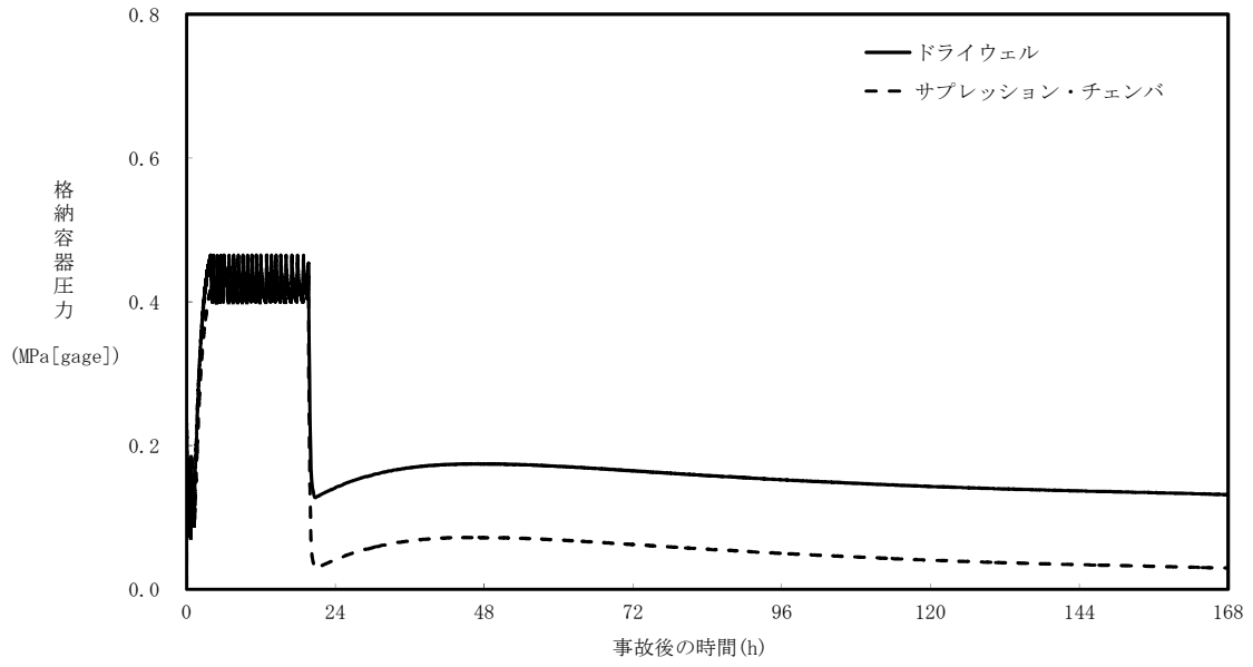
大破断LOCA解析（ベースケース：空隙率 0.1 以下で完全閉塞）
