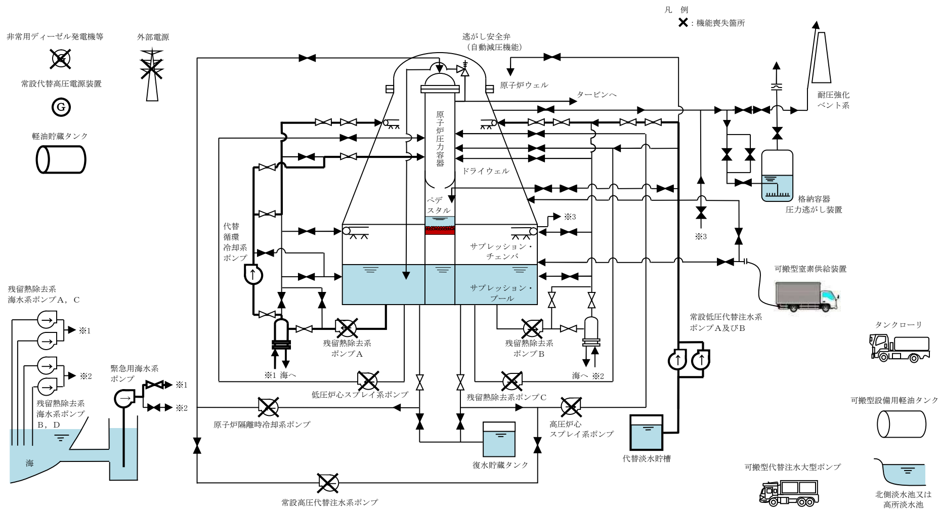
第 3.2-1 図 高压溶融物放出／格納容器雰囲気直接加熱時の重大事故等対処設備の概略系統図(4/5) (原子炉圧力容器破損後の代替循環冷却系による原子炉注水及び格納容器除熱、 代替格納容器スプレイ冷却系(常設)による格納容器压力制御段階)
