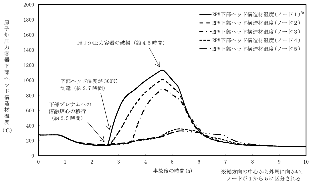
第 3. 2-6 図 原子炉压力容器下部ヘッド温度の推移
