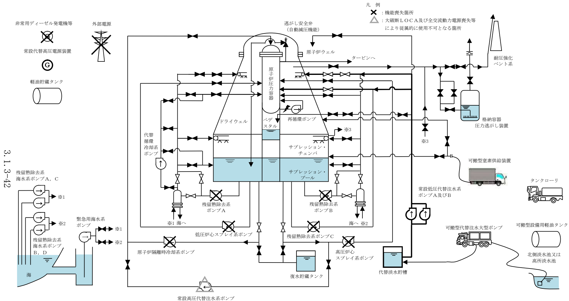
第 3.1.3-1 図 「雰囲気圧力・温度による静的負荷（格納容器過圧・過温破損）」の重大事故等対策の概略系統図（代替循環冷却系を使用しない場合）（1/2） （低圧代替注水系（常設）による原子炉注水，代替格納容器スプレイ冷却系（常設）による格納容器冷却段階）
