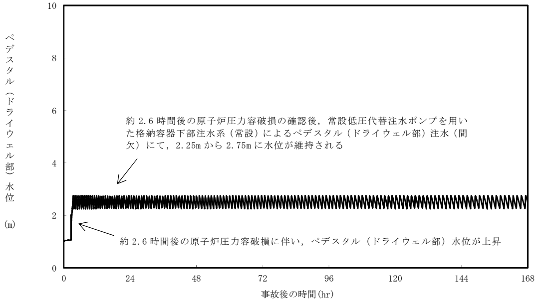
第4図 ペDESTAL水位の推移
