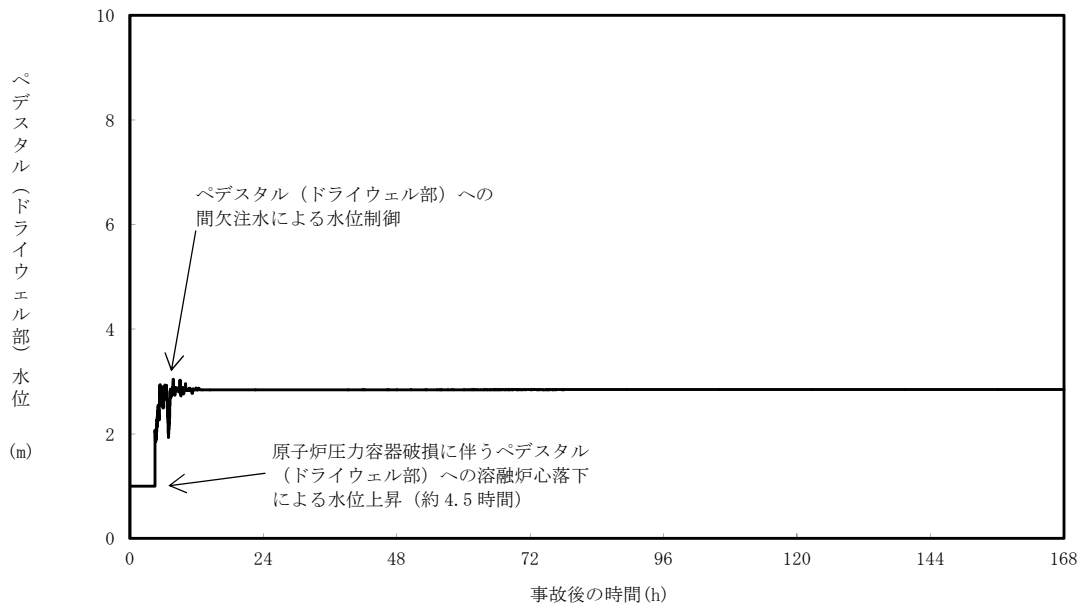
第 3.2-15 図 ペデスタル（ドライウエル部）の水位の推移
