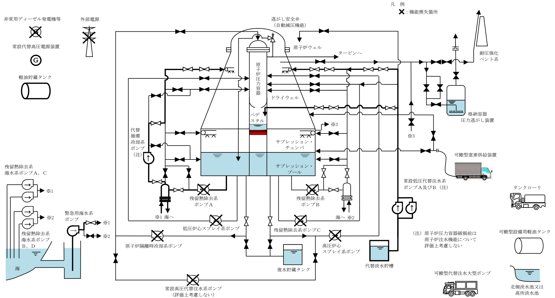
第 3.2-1 図 高圧溶融物放出／格納容器雰囲気直接加熱時の重大事故等対処設備の概略系統図 (3/5) (原子炉圧力容器破損後の代替循環冷却系による格納容器除熱，代替格納容器スプレイ冷却系 (常設) による格納容器冷却及び格納容器下部注水系 (常設) による溶融炉心への注水段階)
