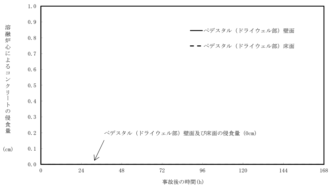
第 3.2-17 図 ペDESTAL (ドライウエル部) の 壁面及び床面のコンクリート侵食量の推移
