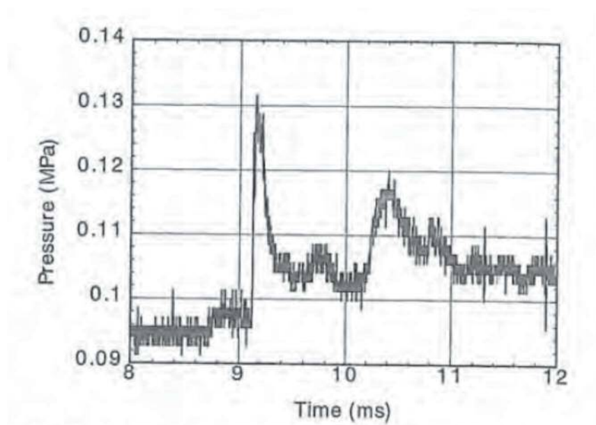
第 2 図 ALPHA 試験の圧力評価の例 (STX016)
