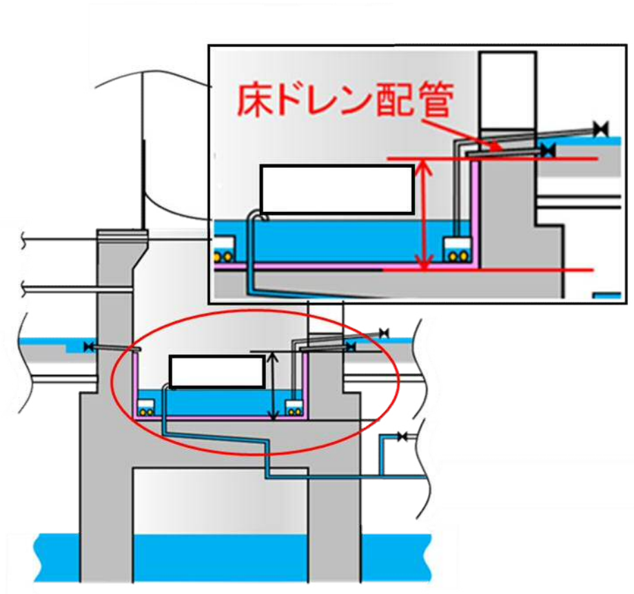
第1図 デブリがペDESTAL外へ流出する可能性のある経路
