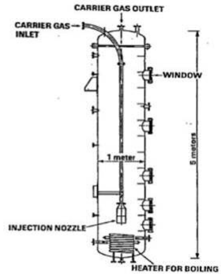
第4図 試験装置の概要
