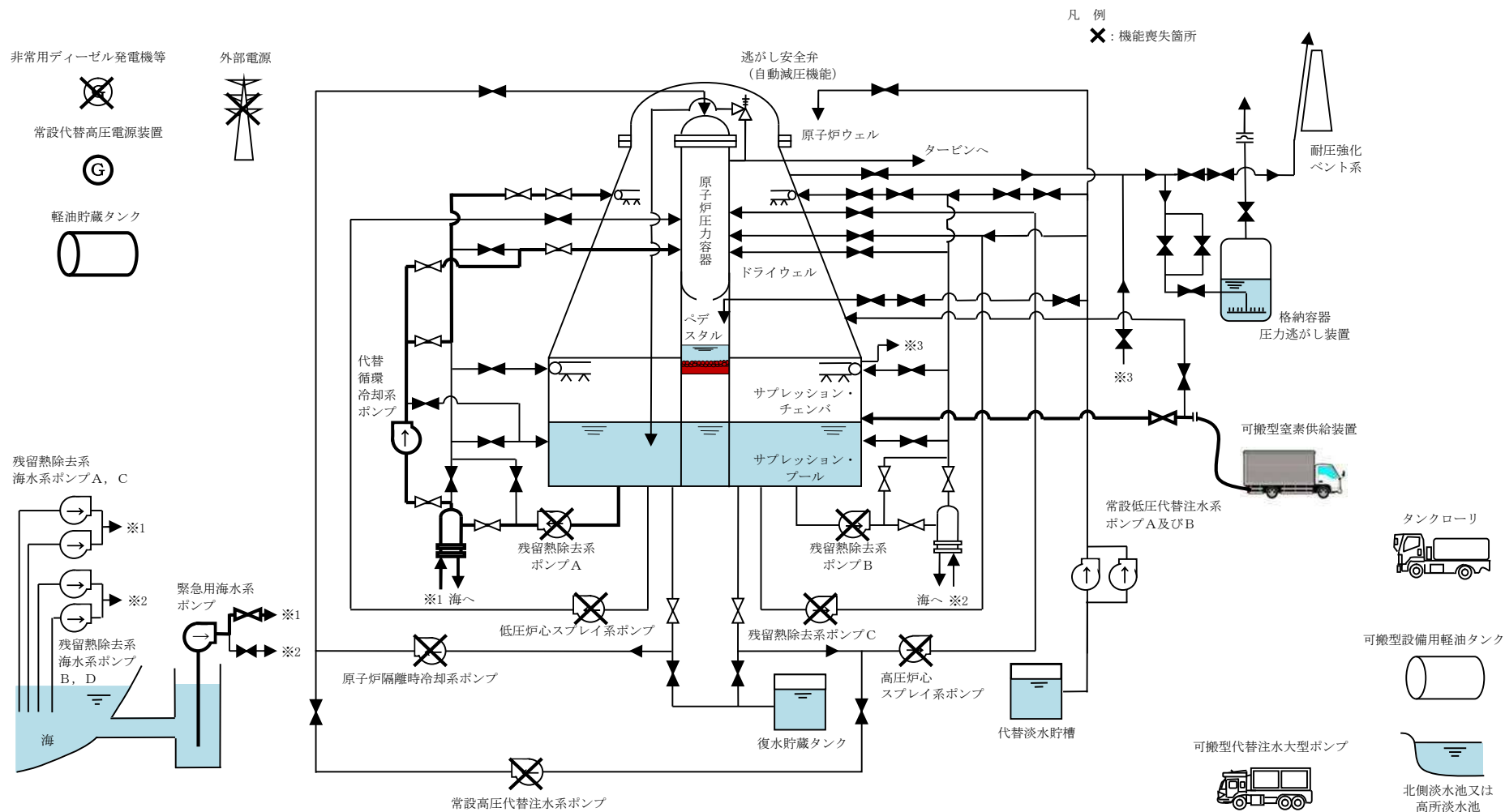
第 3.2-1 図 高圧溶融物放出／格納容器雰囲気直接加熱時の重大事故等対処設備の概略系統図 (5/5) (原子炉圧力容器破損後の代替循環冷却系による原子炉注水及び格納容器除熱、 可搬型窒素供給装置を用いた格納容器内窒素供給段階)
