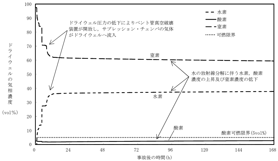
第 3.2-20 図 ドライウエルの気相濃度の推移（ドライ条件）
