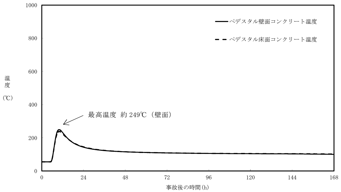
第 5 図 ペデスタル（ドライウェル部）コンクリート表面温度の推移 (ベースケース)
