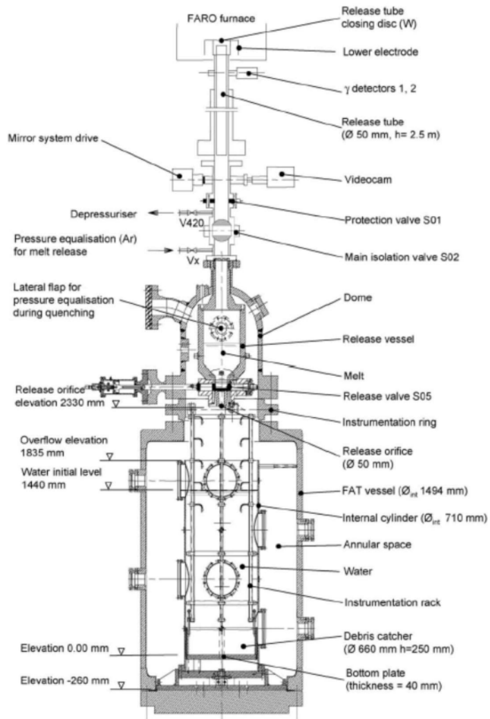
第 5 図 FARO 試験装置の概要
