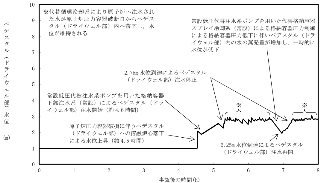
第 3.2-16 図 ペデスタル（ドライウエル部）の水位の推移（～8 時間）
