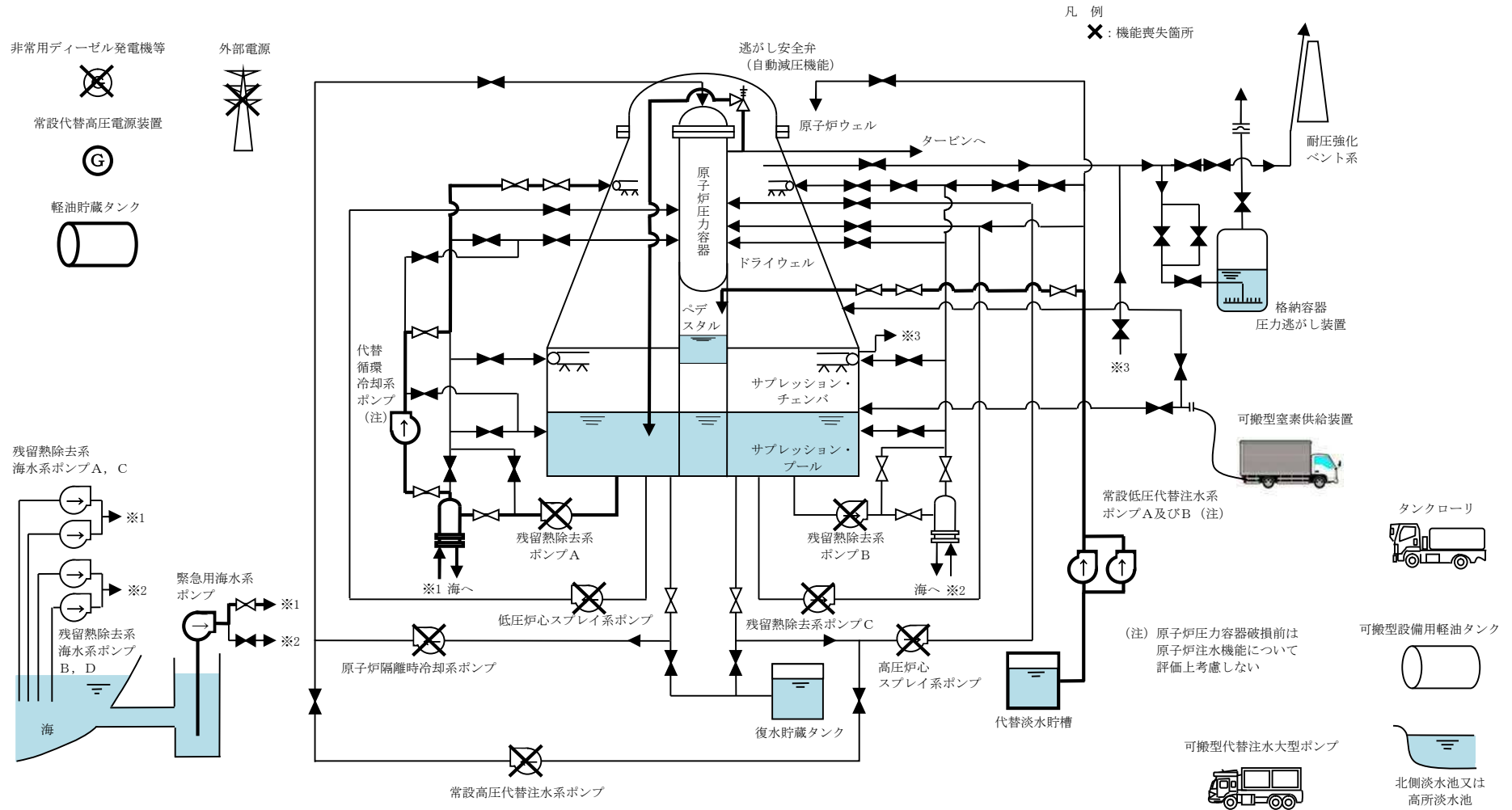
第 3.2-1 図 高压熔融物放出／格納容器雰囲気直接加熱時の重大事故等対処設備の概略系統図 (2/5) (原子炉压力容器破損前の代替循環冷却系による格納容器除熱及び格納容器下部注水系 (常設) による格納容器下部水位確保段階)
