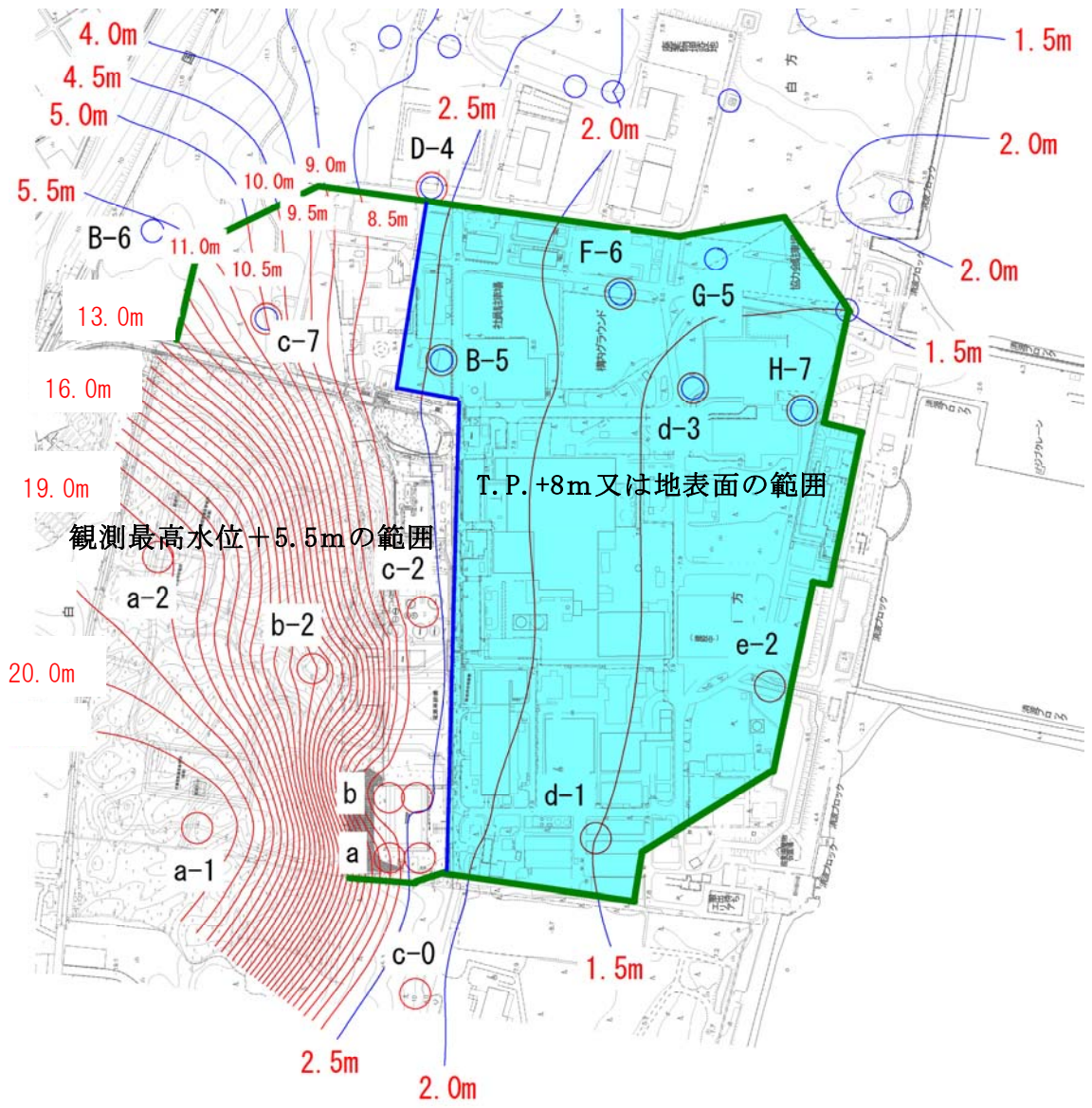
第 2 図 検討用地下水位コンター図
