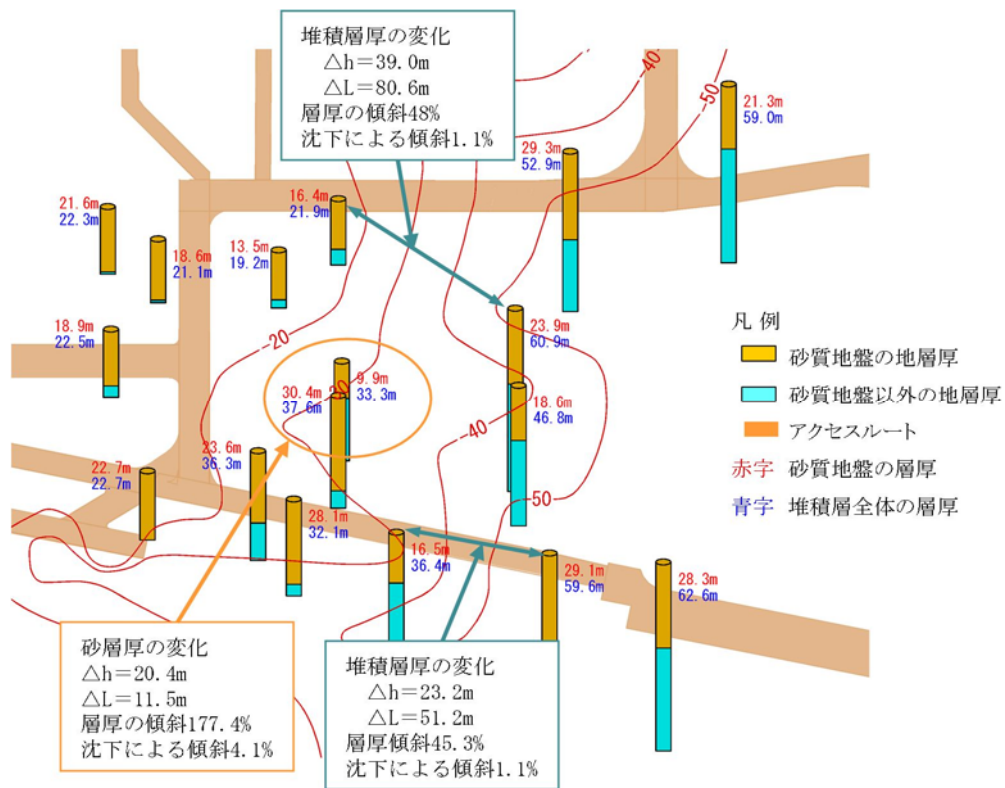
第4図 堆積層厚及び砂質地盤厚さの分布 (I部)
