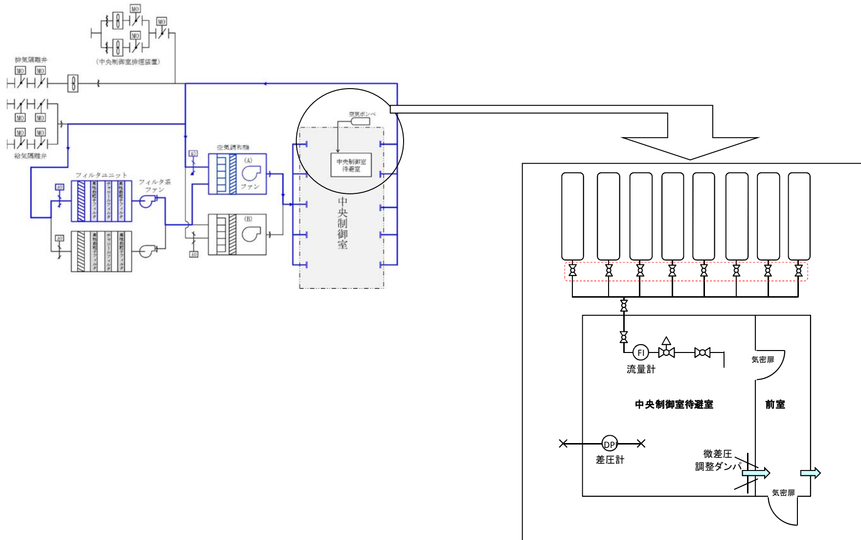
第59-4-2図 中央制御室待避室空気ポンベユニット 系統概要図
