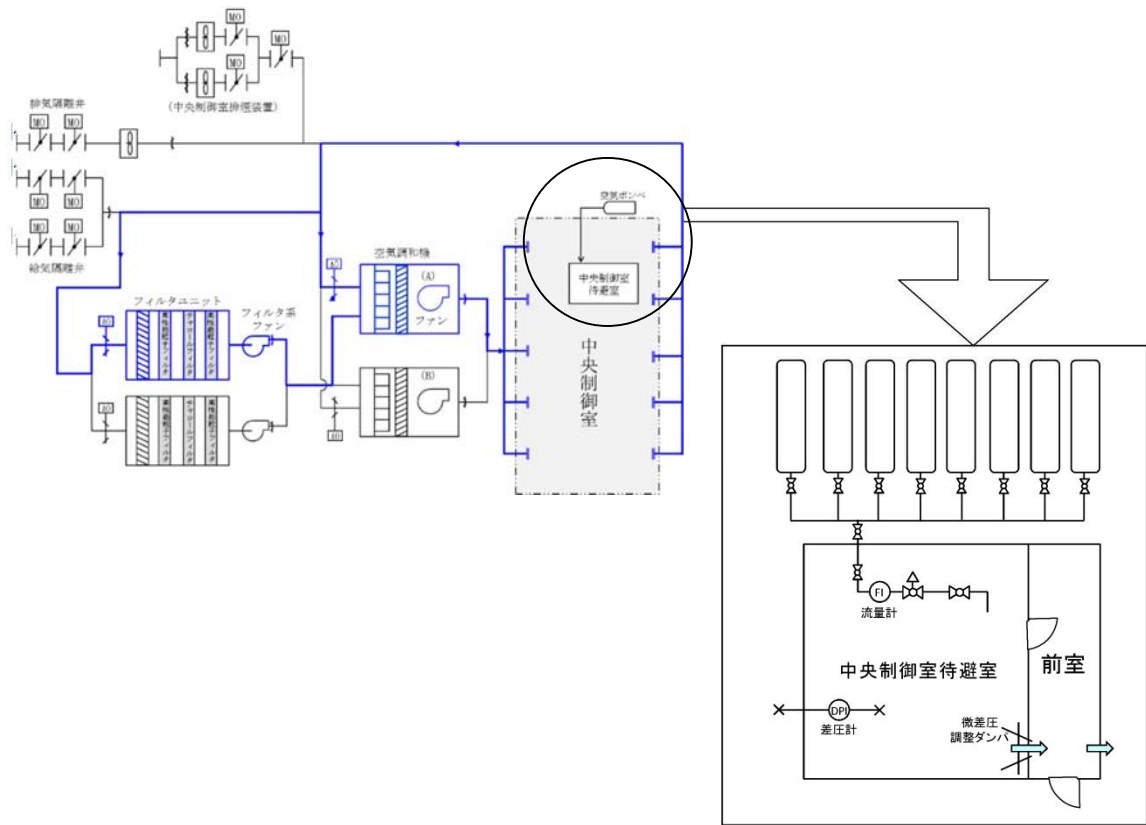
第59-5-2図 中央制御室待避室の正圧化試験におけるバウンダリ構成図
