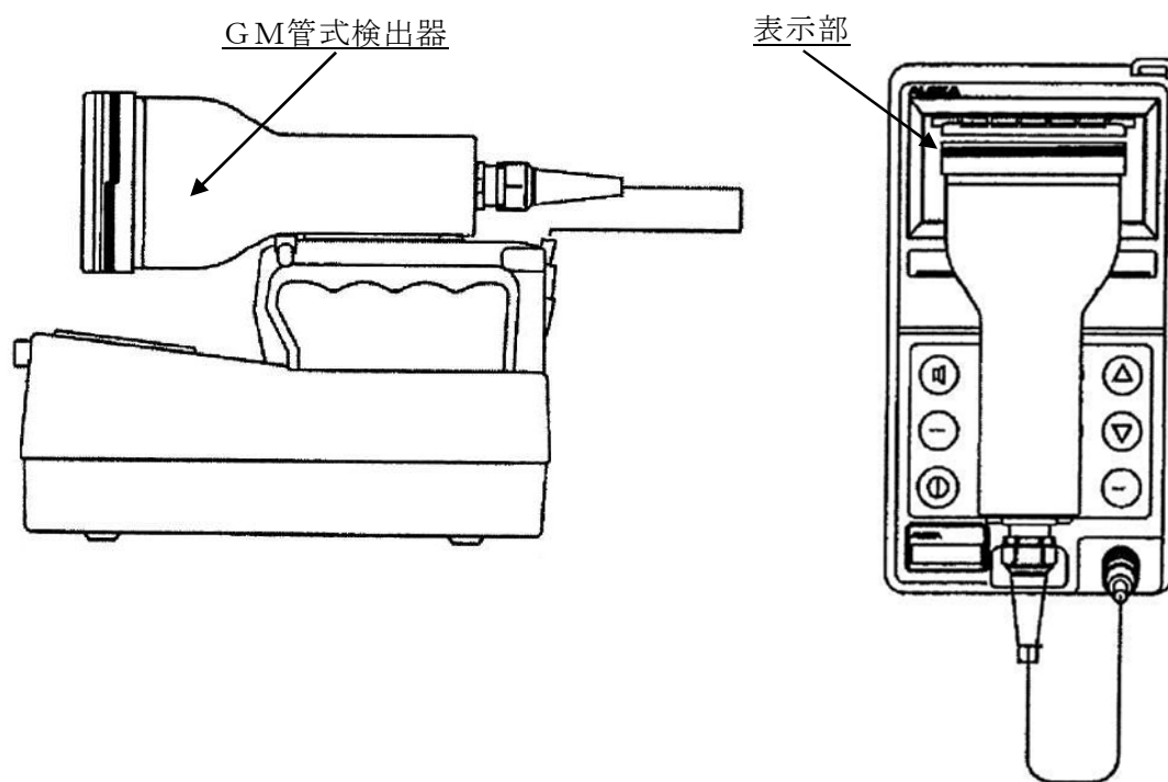
第 60-4-4 図 \beta 線サーベイ・メータ
