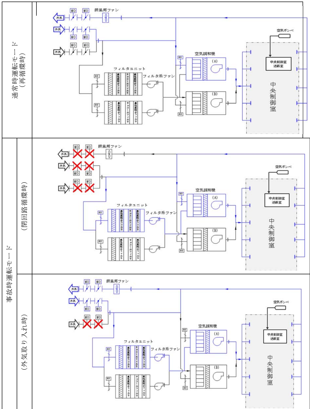
第5.1.3-2図 中央制御室換気系系統構成
