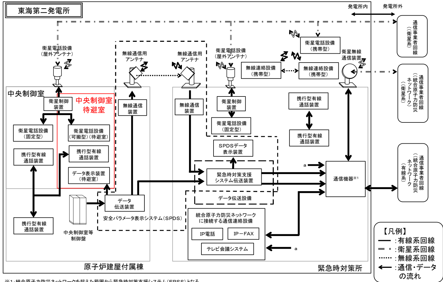
図59-4-5 データ表示装置 系統概要図
