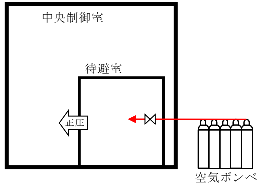
重大事故時【格納容器ベント実施中】 (空気ポンペ加圧)
