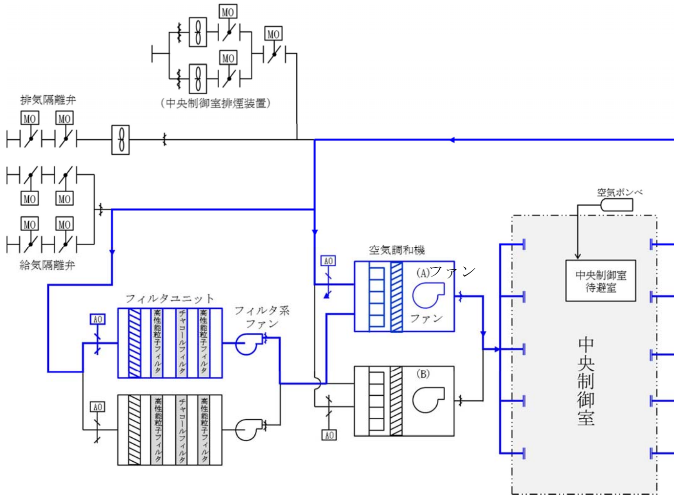
第59-4-1図 中央制御室換気系 系統概要図
