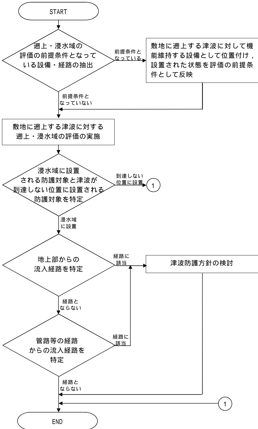
第 2.2-1 図 敷地に遡上する津波に対する津波防護の検討フロー
