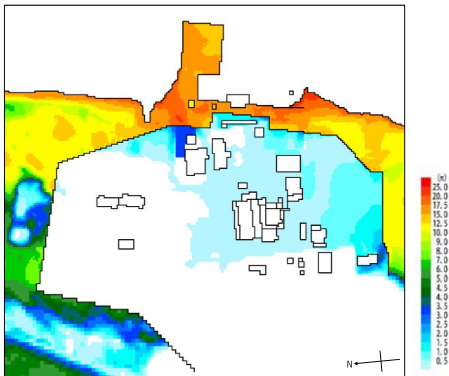
11m 盤周辺拡大
