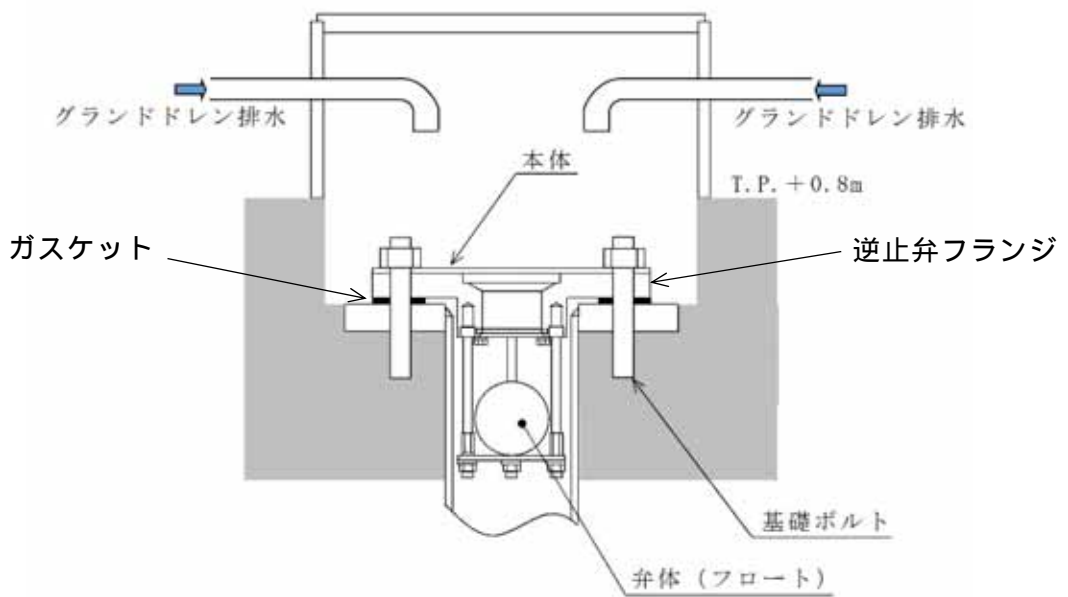
第 2.3.1 - 4 図 緊急用海水ポンプグランド dren 排出口逆止弁構造図
