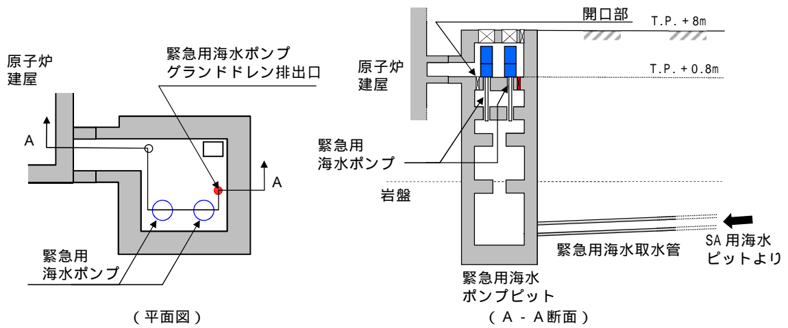
第 2.2.3-3 図 緊急用海水ポンプグランドドレン排出口及び 緊急用海水ポンプ配置図
