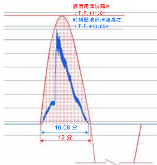
第2.3.2 - 3図 時刻歴波形の正弦波モデル例 (津波 (類型化 a) の場合)
