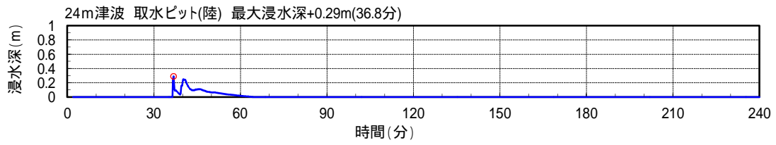
( 取水ピット )
