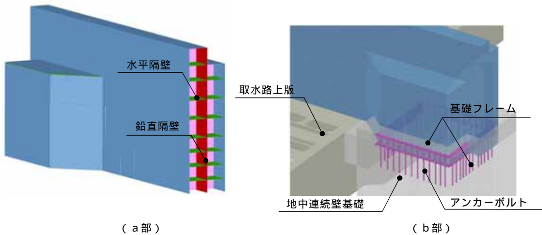
第 3.1 - 3 図 構造形式毎の防潮提構造図 ( 1 / 4 ) [ ( a ) 鋼製防護壁 ]
