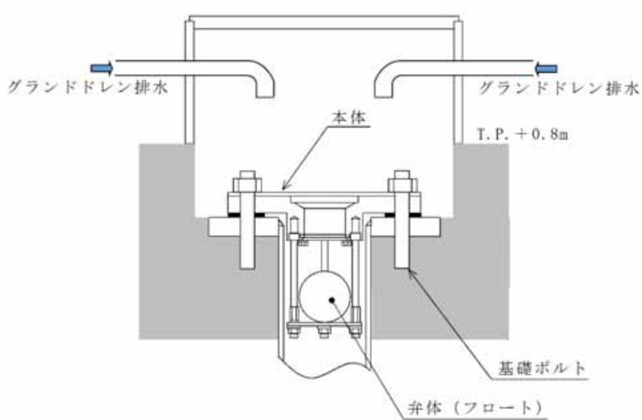
第 2.2.3-4 図 緊急用海水ポンプピット点検用開口部浸水防止蓋概略構造
