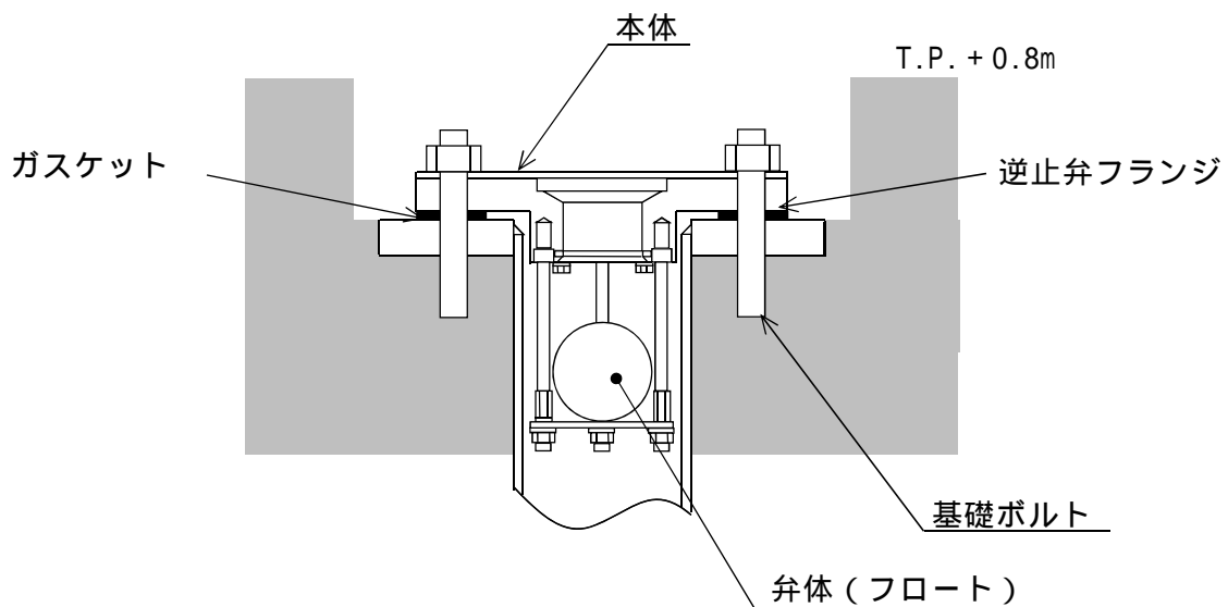
第 3.2 - 7 図 緊急用海水ポンプ室床 dren 排出口逆止弁構造図
