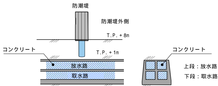
第 2.2.1-27 図 東海発電所取水路及び放水路の閉鎖概要図
