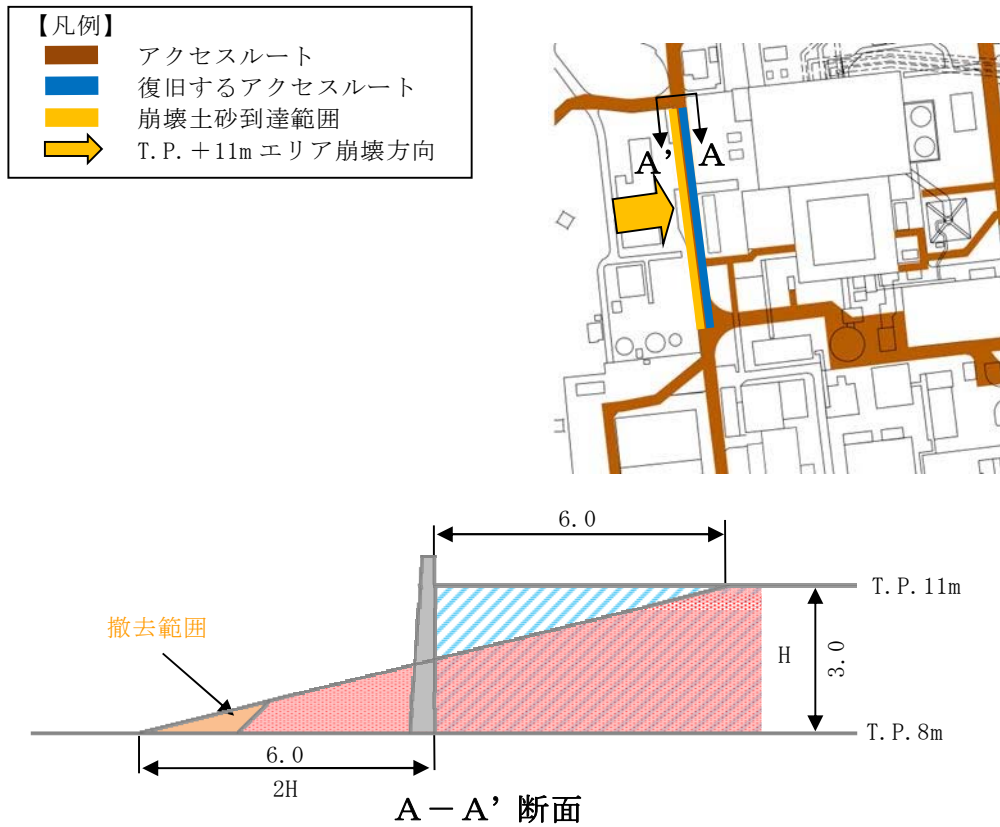
第5.5.1-5図 崩壊土砂撤去の考え方
