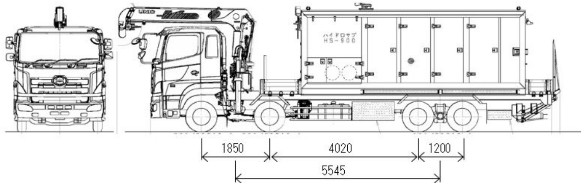
第2図 可搬型代替注水大型ポンプ
