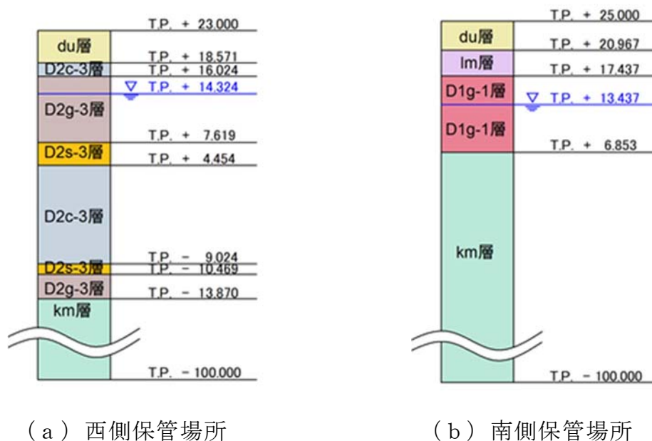
第4.3.3-4図 一次元有効応力解析モデル 1.0.2-64
