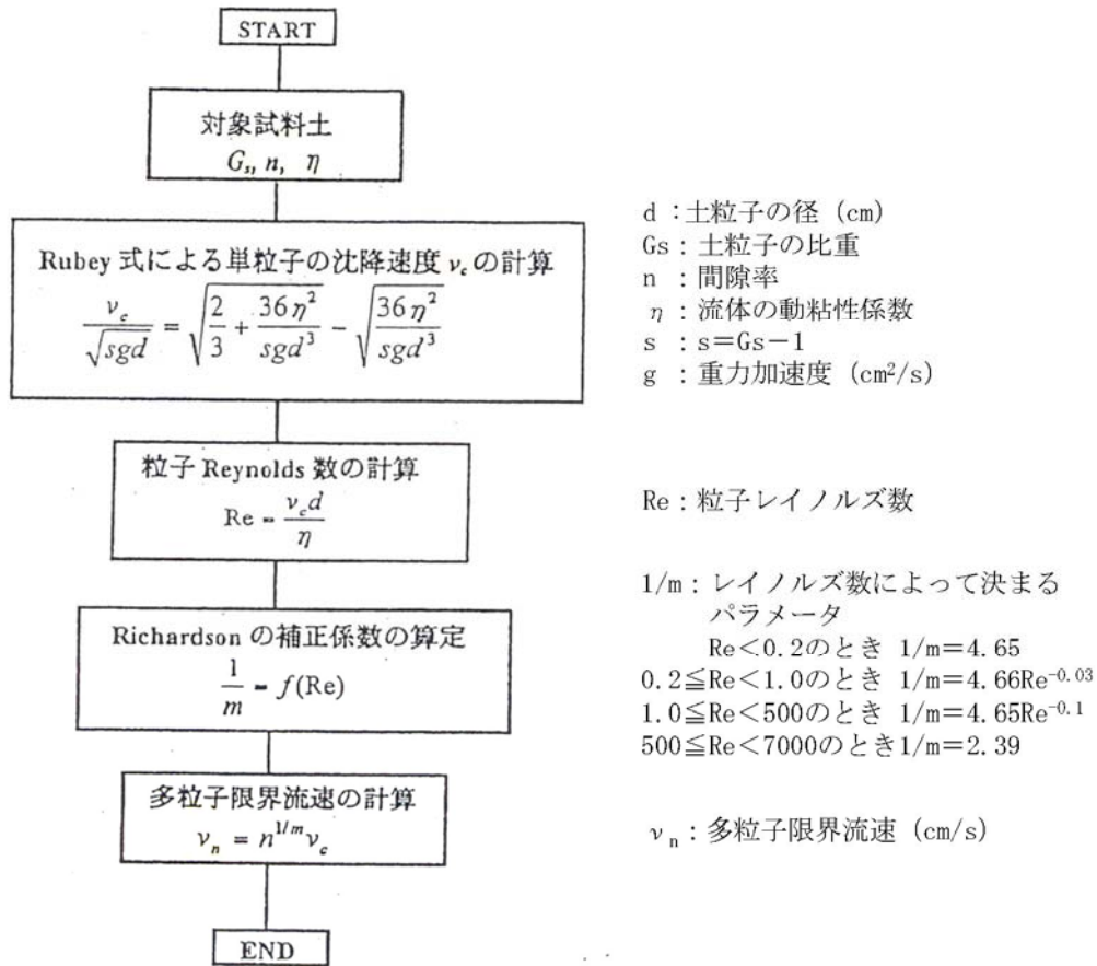
第6図 多粒子限界流速の検討フロー
