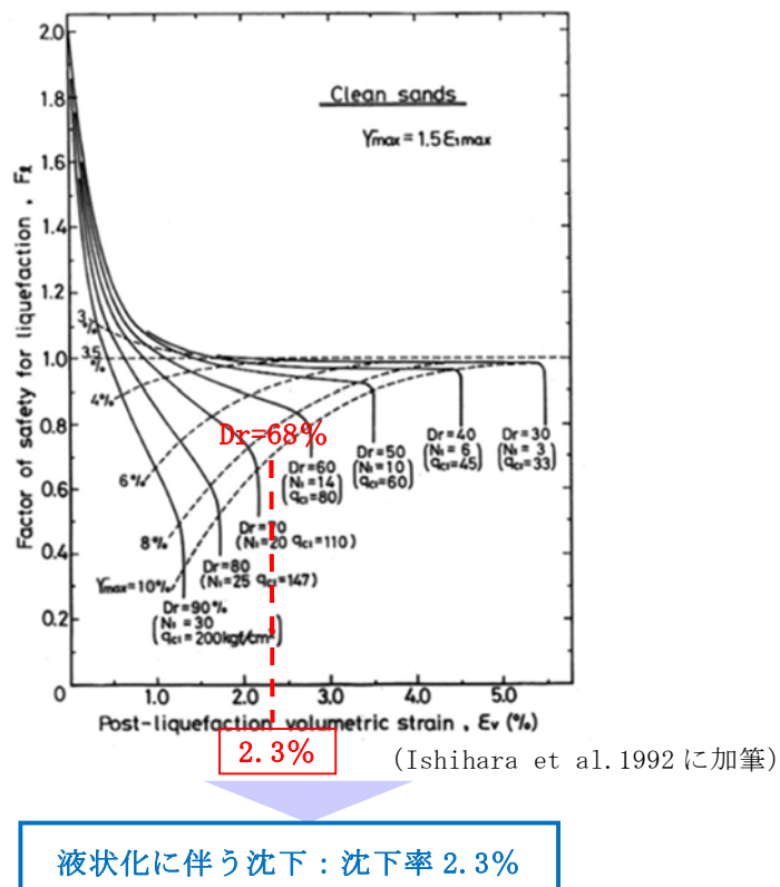
第5.4.3-2図 体積ひずみと液状化抵抗の関係及び想定する沈下率
