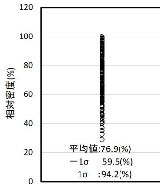
第 3 図 du 層（砂層）の相対密度
