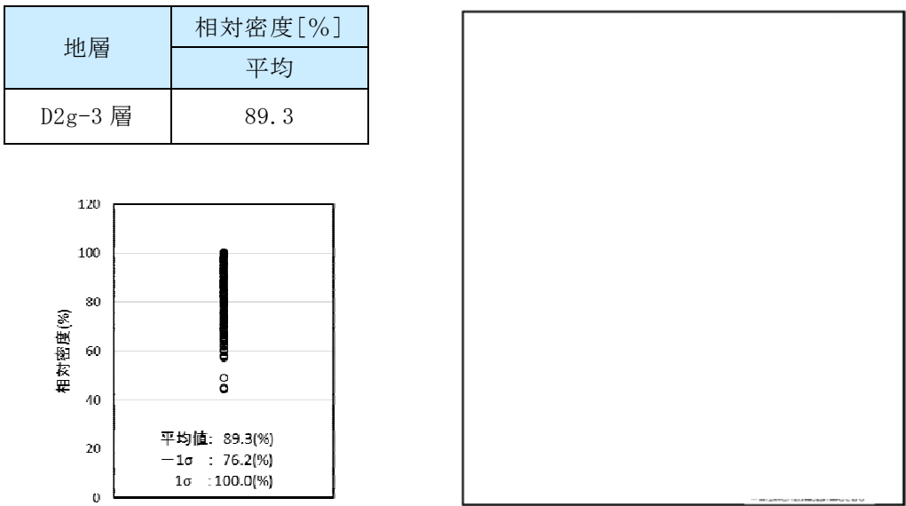
第 8 図 D2g-3 層（砂礫層）の相対密度
