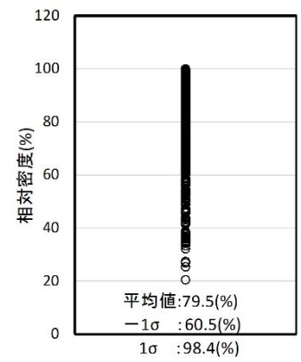
第 4 図 Ag2 層（砂礫層）の相対密度
