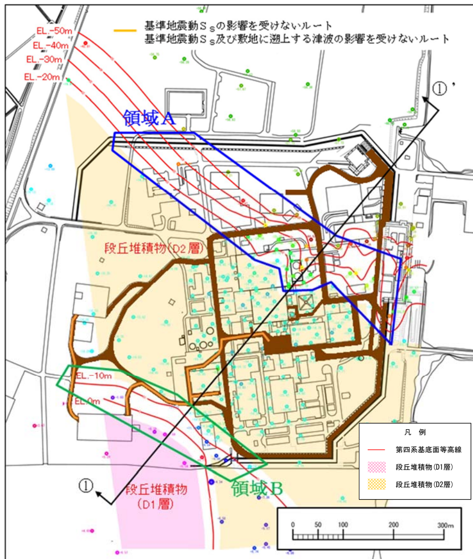
第 1 図 第四系基底の標高分布及び段丘面区分図
