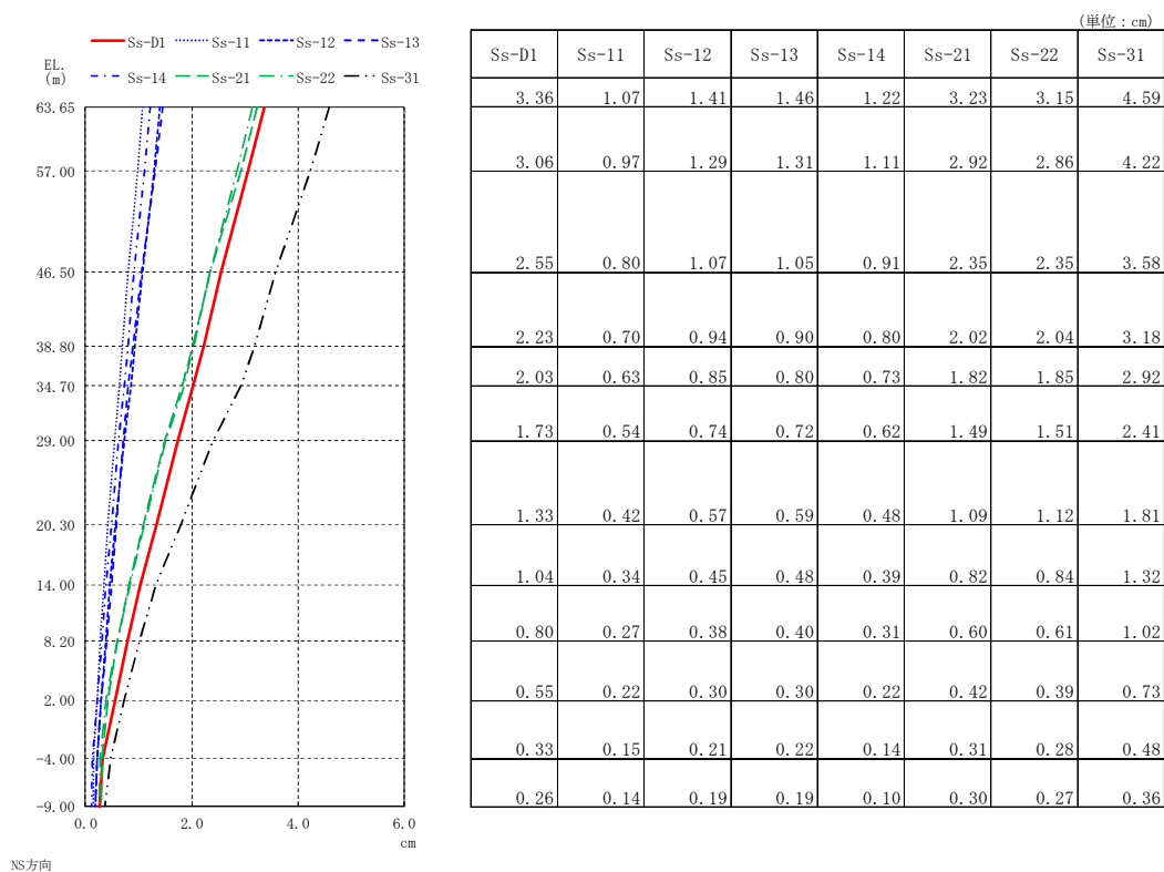
第 5-23 図 最大応答水平変位（N S 方向）
