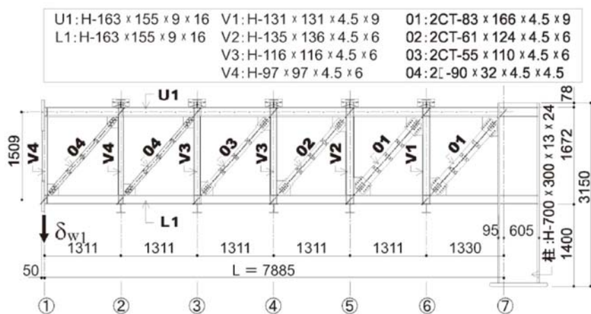
(a) プラット形試験体
