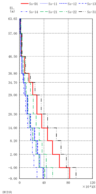
第 5-28 図 最大応答せん断力 (E W 方向)
