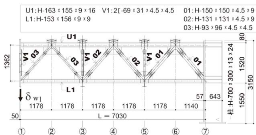
(b) ワーレン形試験体
