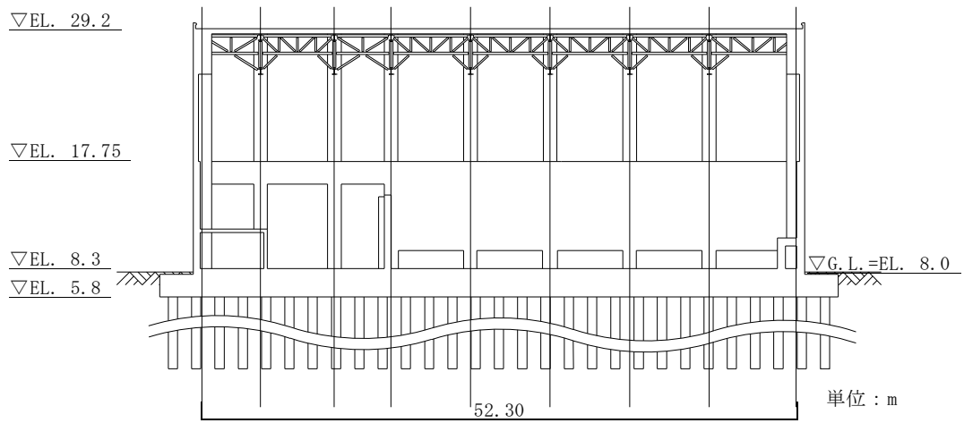
(N S 方向，A—A 断面)
