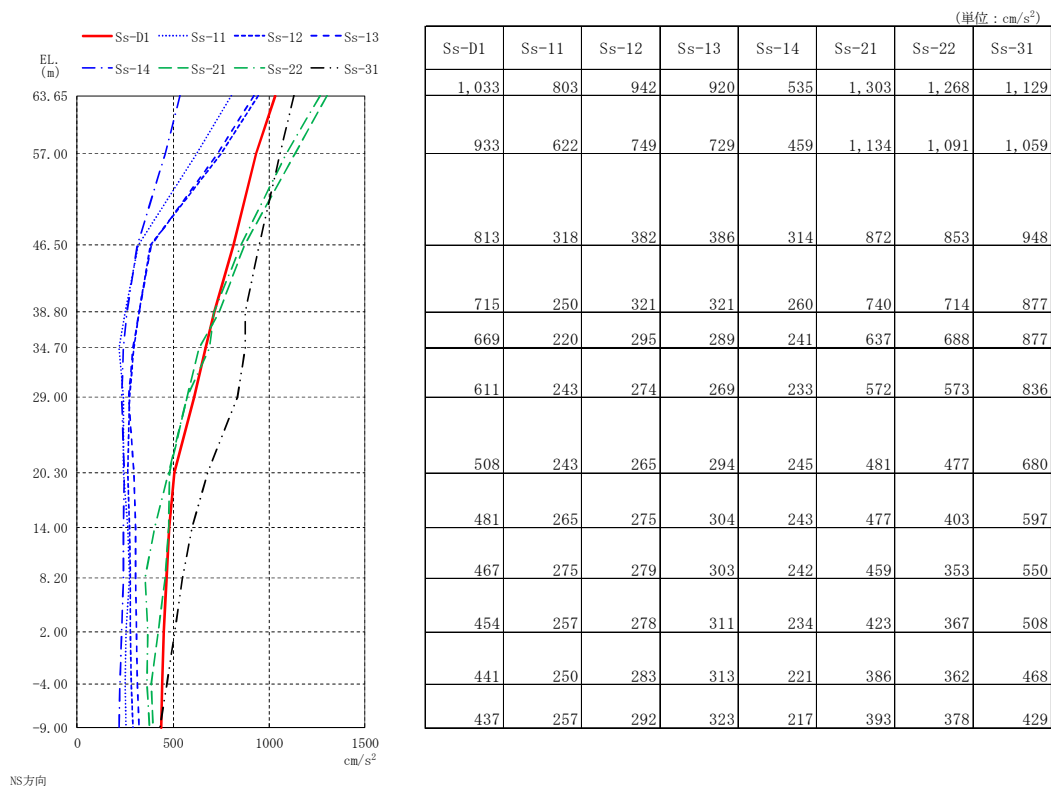
第 5-22 図 最大応答加速度（N S 方向）
