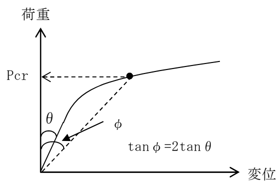
第 8-12 図 崩壊荷重の下限 ( P_{cr} ) の定義
