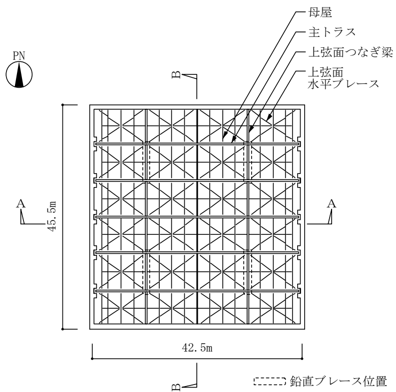
(屋根伏図)
