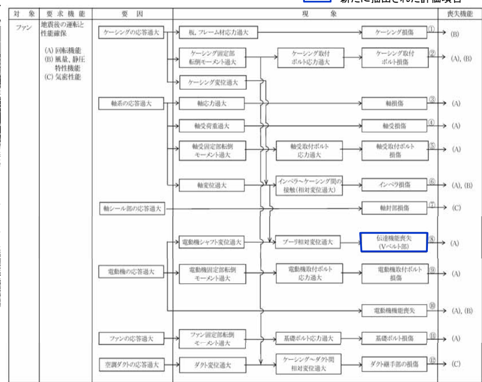
図6 遠心Vベルト式ファン地震時異常要因分析図【東海第二】
