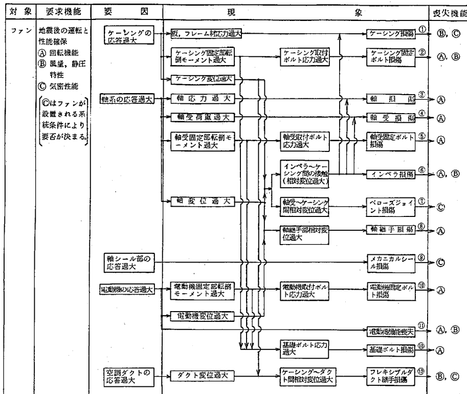
図5 遠心直結式ファン地震時異常要因分析図【耐特委における検討】
