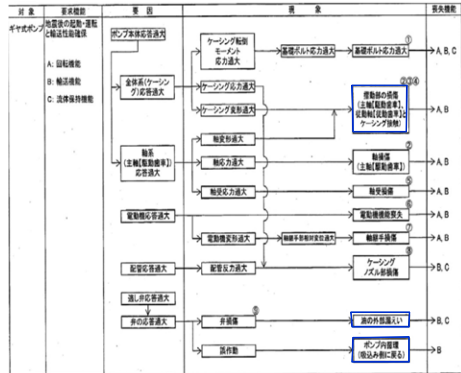
図8 ギヤ式ポンプ地震時異常要因分析図【東海第二】
