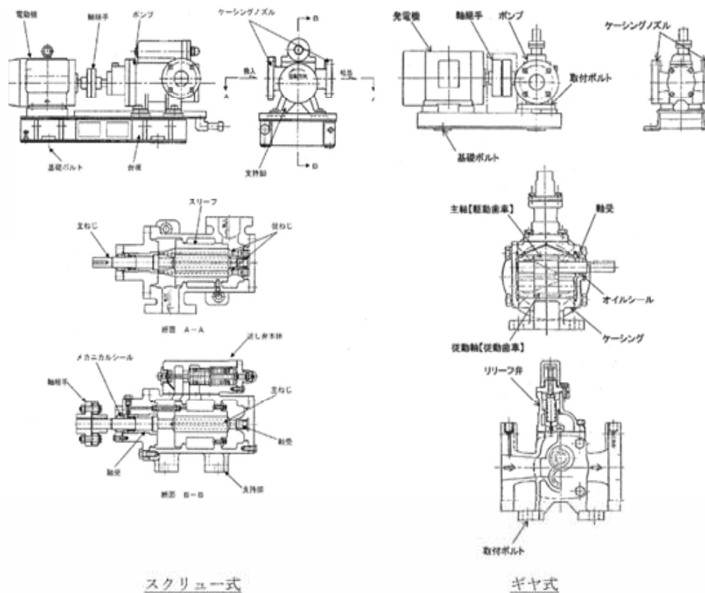
図4 スクリュー式及びギヤ式ポンプ構造図
