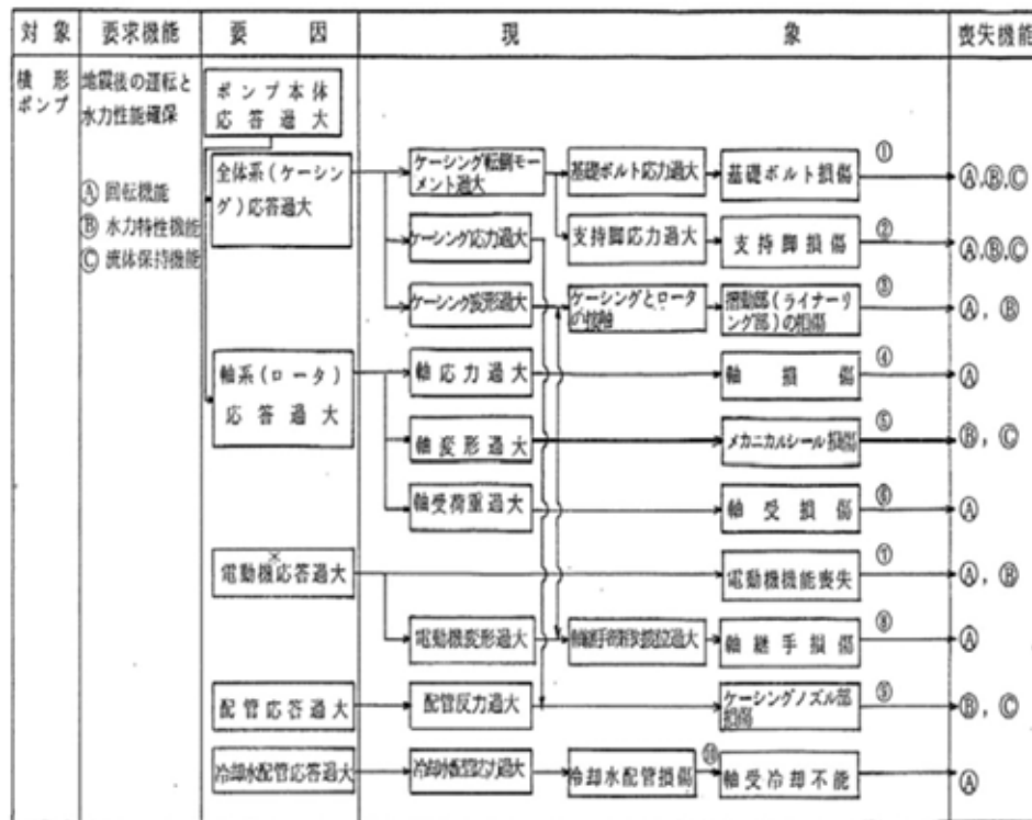
図7 遠心式横形ポンプ地震時異常要因分析図【耐特委における検討】
