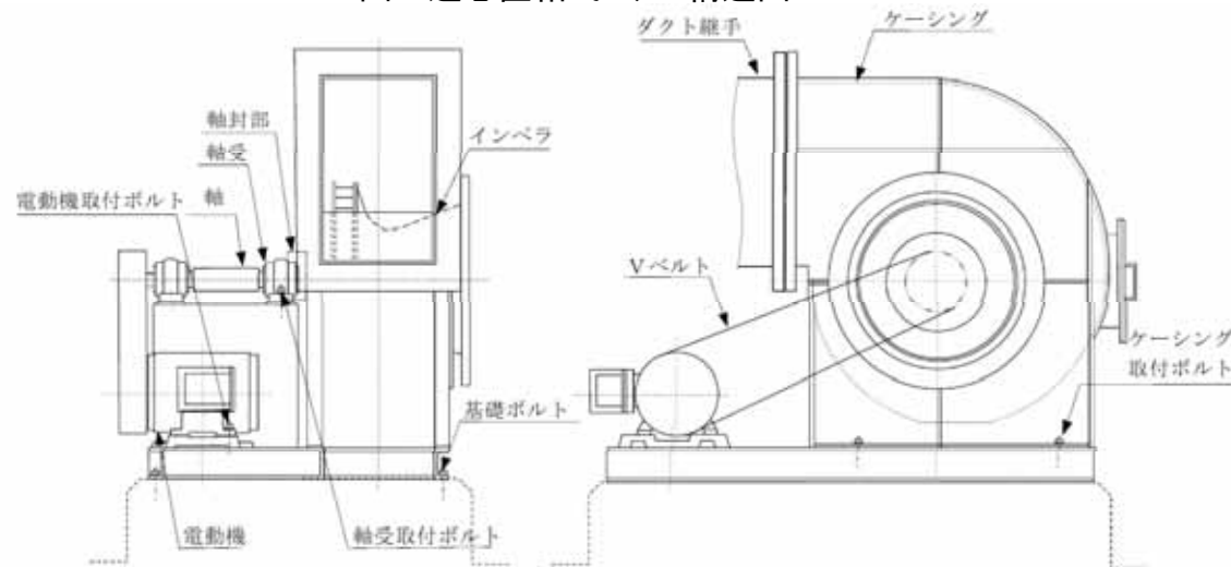
図2 遠心Vベルト式ファン構造図
