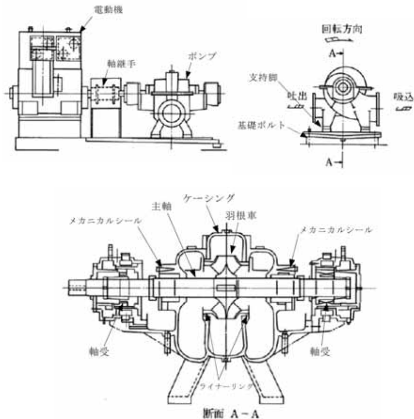
図3 遠心式横形ポンプ構造図
