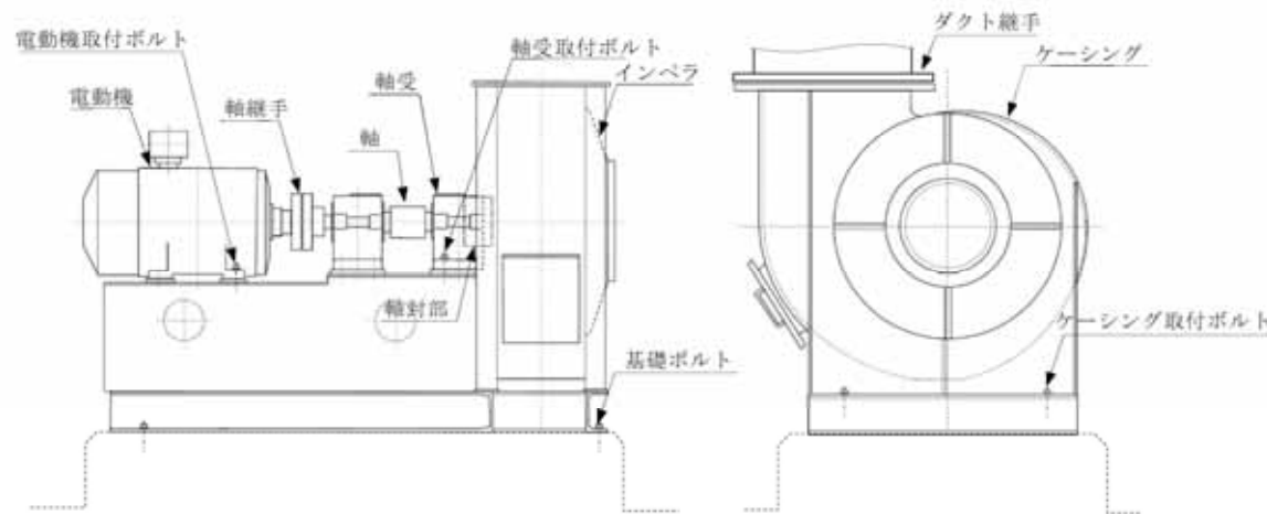
図1 遠心直結式ファン構造図
