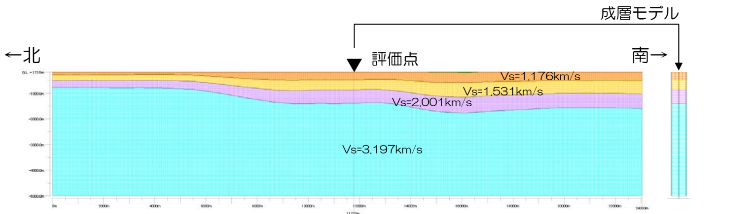
2次元FEMモデル（南北断面）
