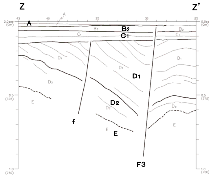
Z-Z' 断面
