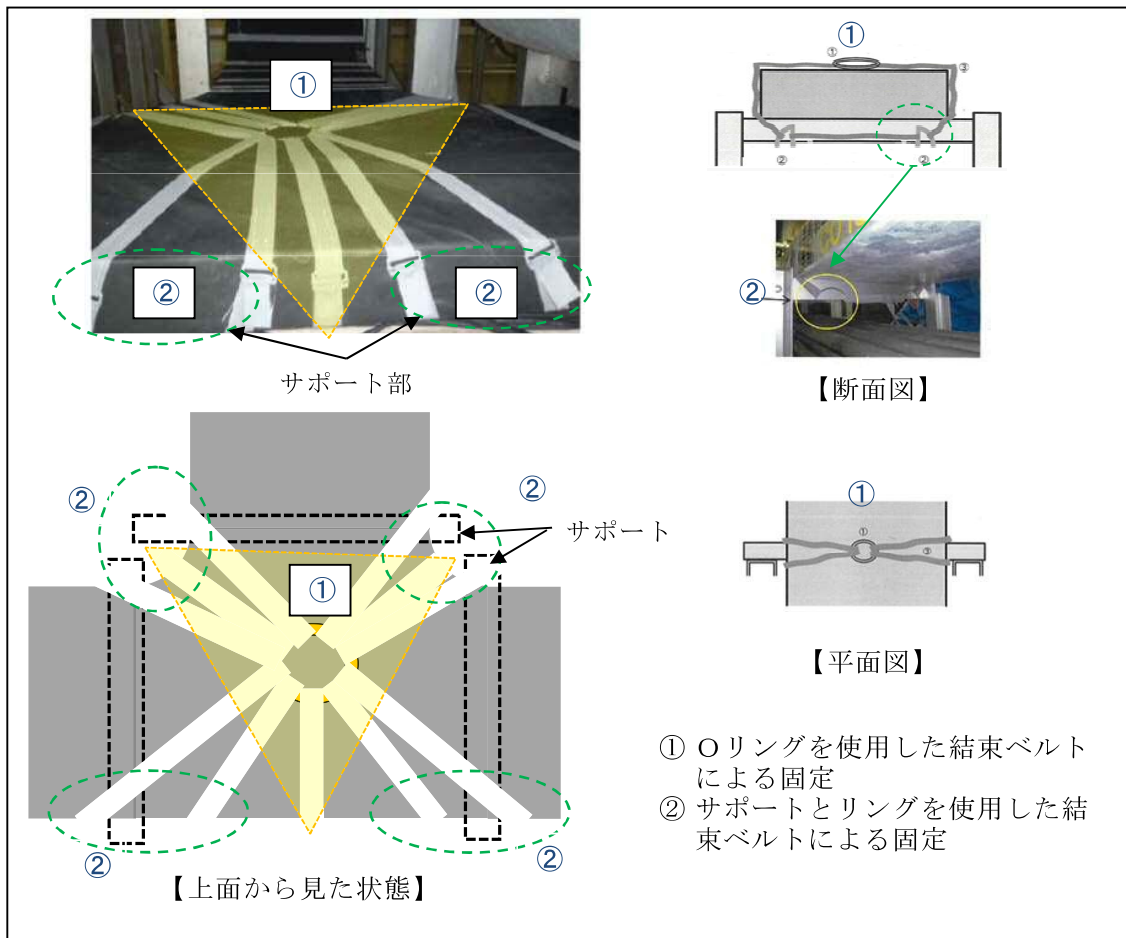
第 6-1-6 図 T字分岐ケーブルトレイの結束ベルト施工例
