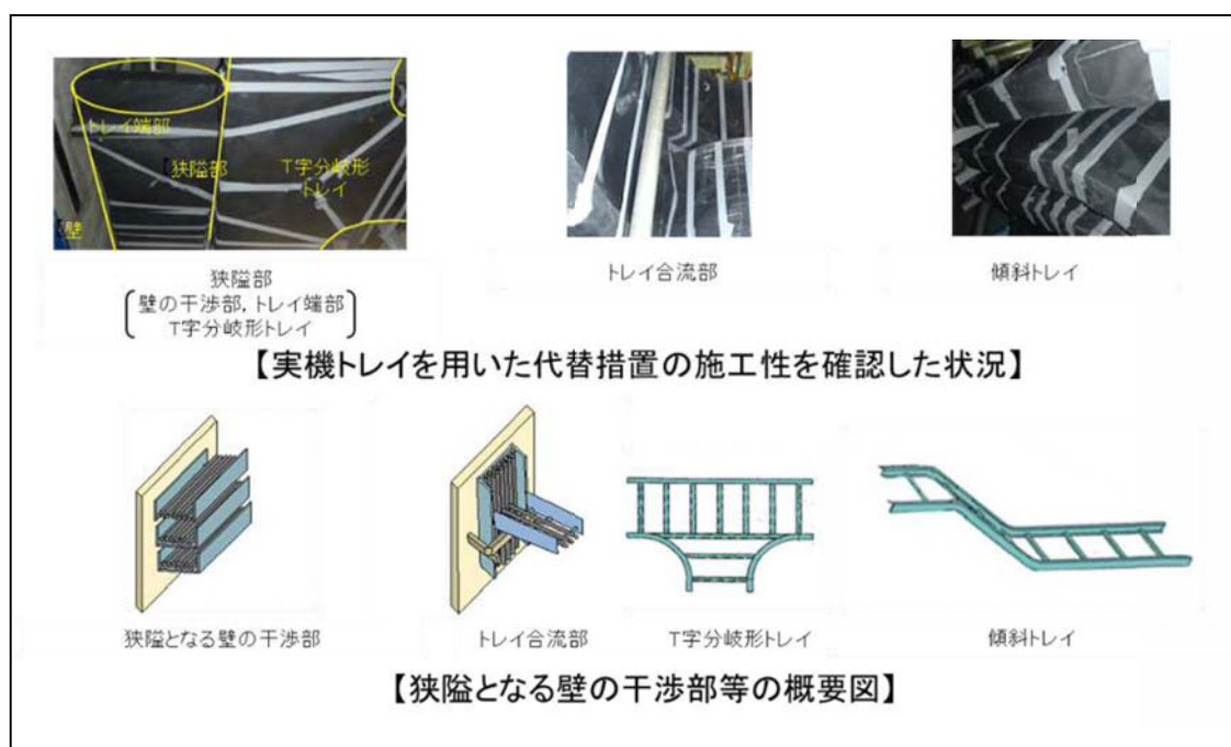
第6-1-3図 狭隘部等への施工例
