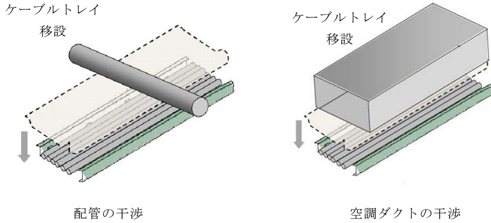
第 6.1-3 図 ケーブルトレイの移設
