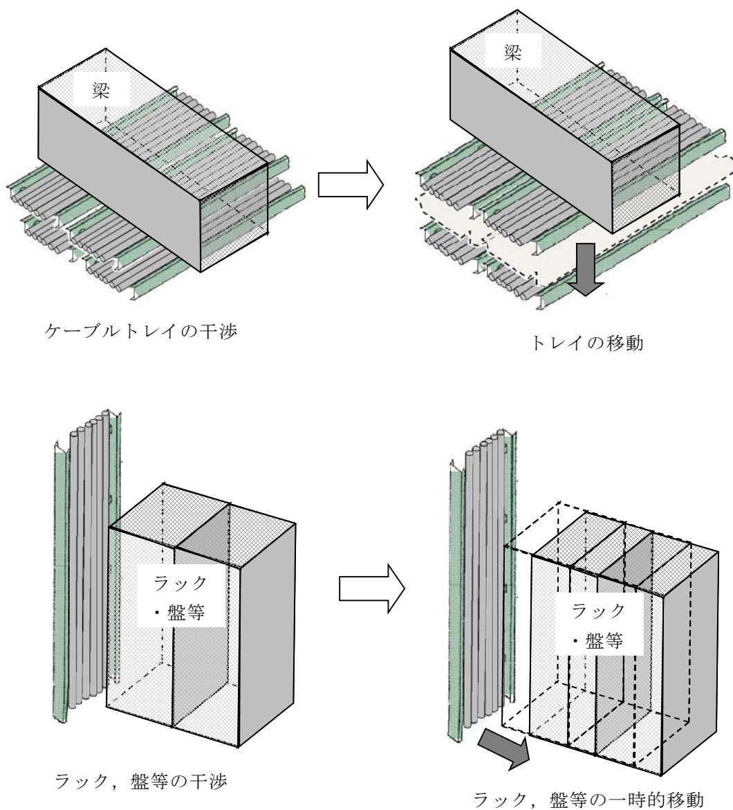
第 6.1-5 図 干渉物移動による作業
