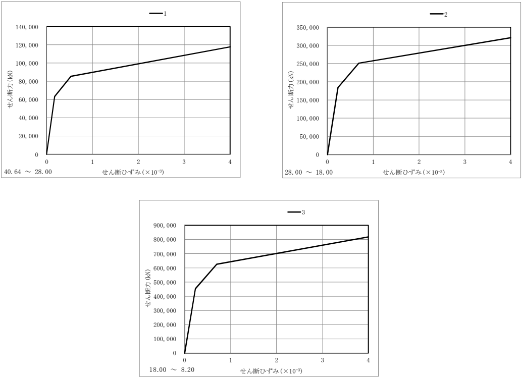
補図 1-2 タービン建屋各層の代表せん断ひずみーせん断力図
