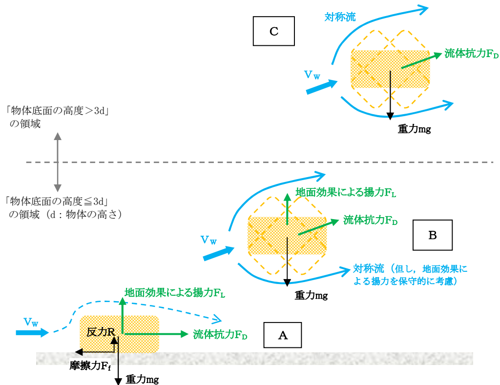
第 5.1-3 図 物体の運動モデルの模式図
