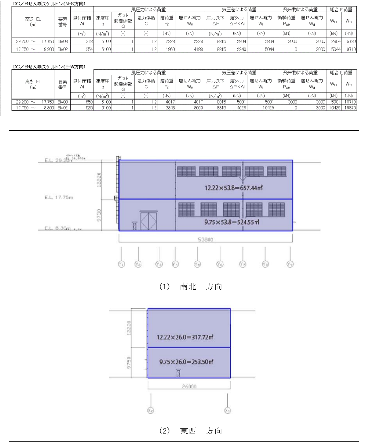
補図 1-1 使用済燃料乾式貯蔵建屋の受圧面の面積図
