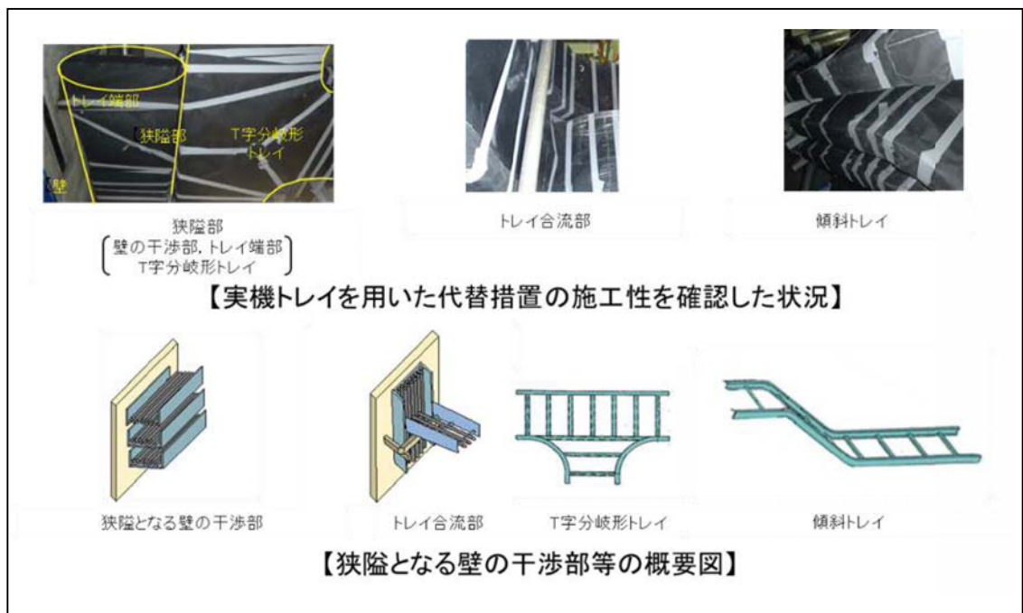
第 6-1-3 図 狭隘部等への施工例
