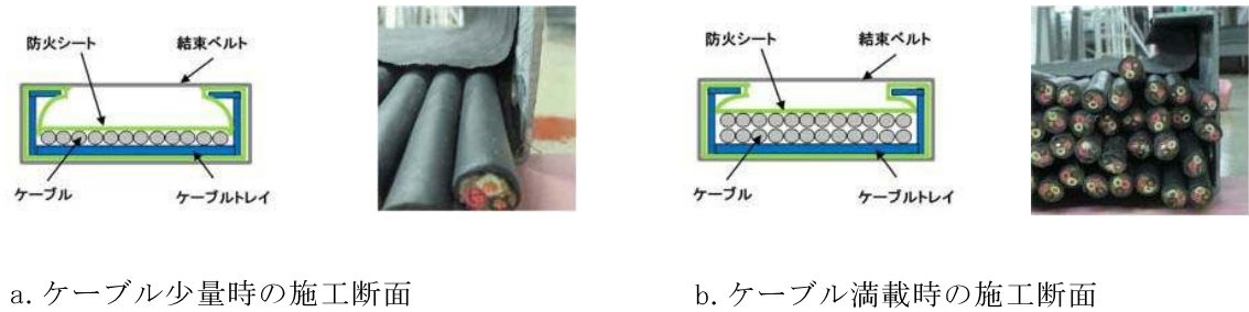
第 6-1-1 図 標準施工の概要
