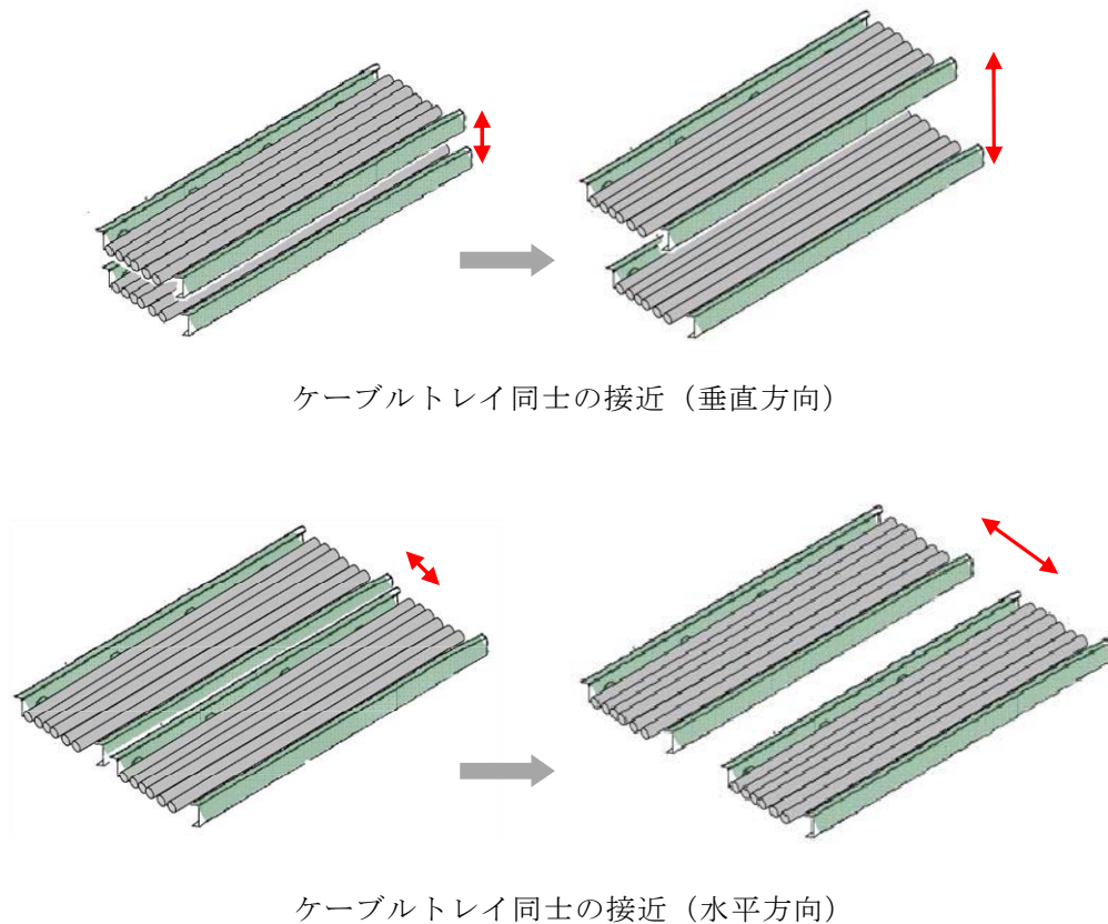
第 6.1-4 図 ケーブルトレイの干渉緩和
