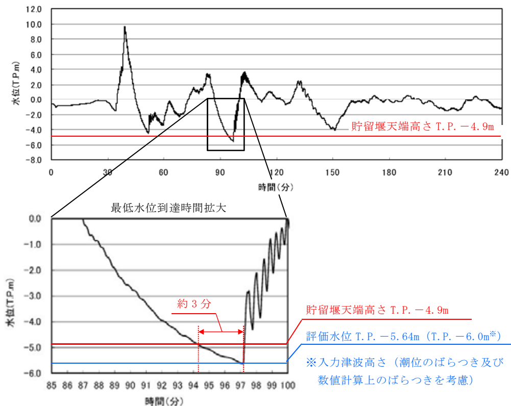
第 2.5-2 図 引き波の継続時間
