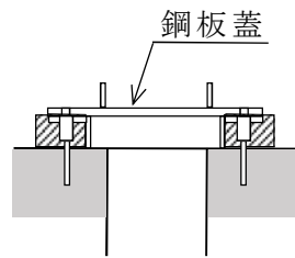
< A-A 断面図 >
