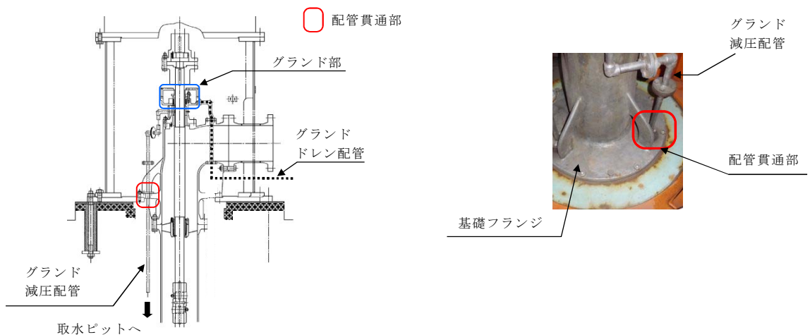
第 2.2-17 図 グランド減圧配管基礎フランジ貫通部 (残留熱除去系海水ポンプの例) 構造図
