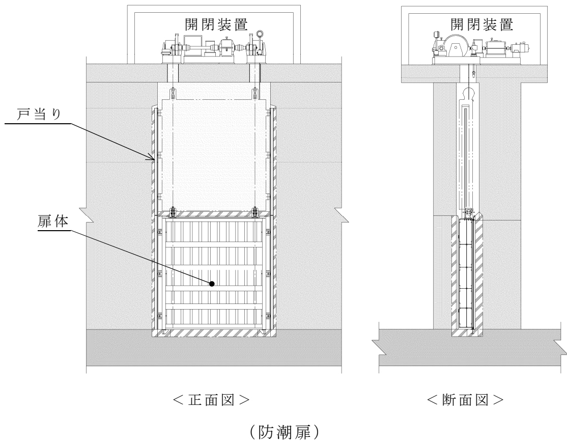
第 10.6-2 図 防潮堤及び防潮扉概念図 (5 / 5)
