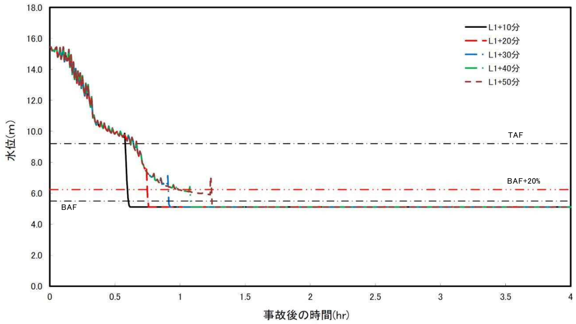
第 1 図 原子炉水位の時間変化（逃がし安全弁（自動減圧機能）7 弁）
