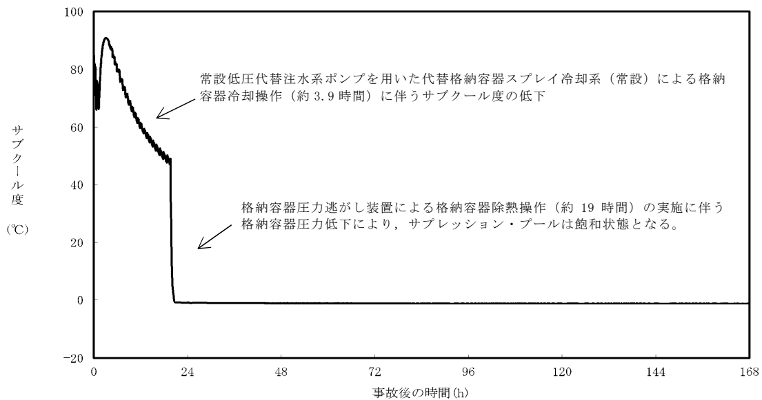
第9図 サブレーション・プールのサブクール度の推移
