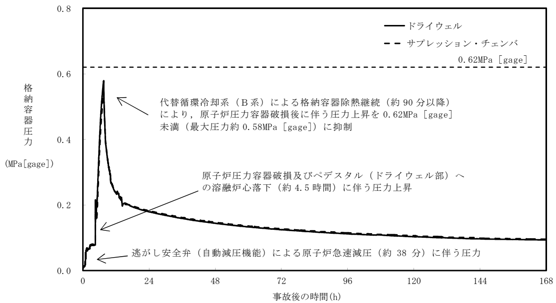
第 7 図 「DCH, FCI, MCCI」における 代替循環冷却系 (B系) を使用した場合の格納容器圧力の推移
