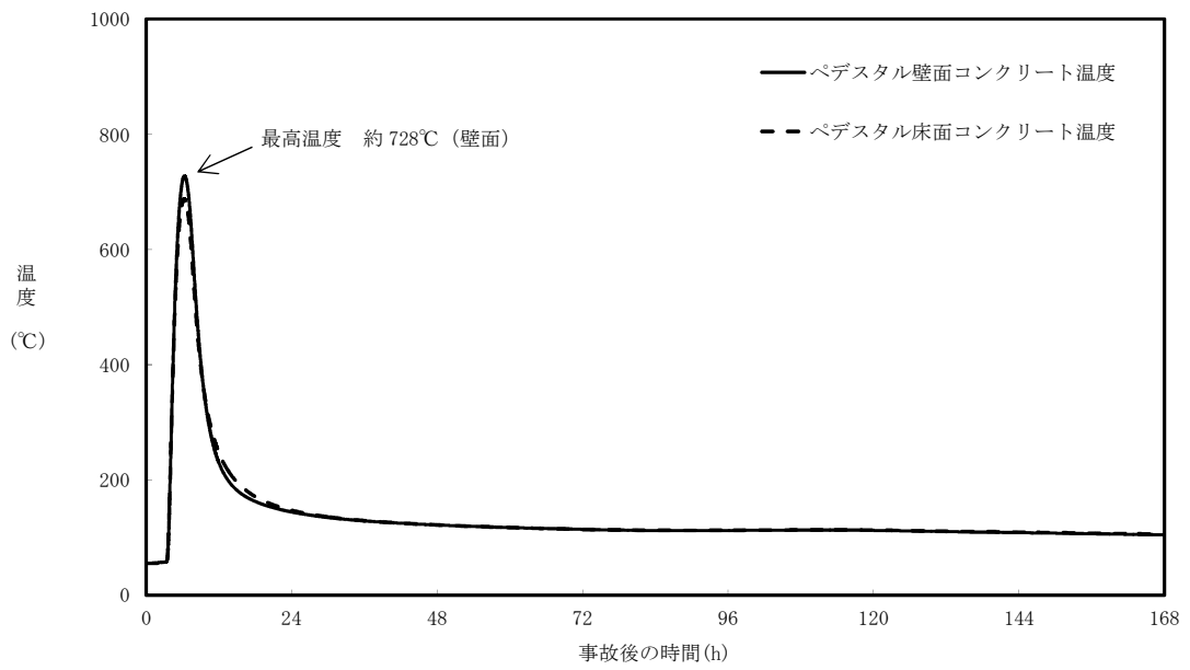
第 7.2.5-3 図 コリウムシールドの侵食及び伝熱物性値の温度依存性を考慮した場合のペDESTAL（ドライウェル部）の壁面及び床面のコンクリート温度の推移
