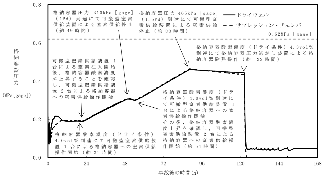
第 3.4-15 図 G 値を設計基準事故ベースとした場合の
