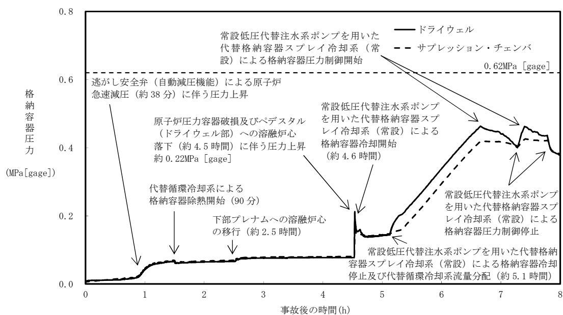
第 3.3-1 図 格納容器圧力の推移
