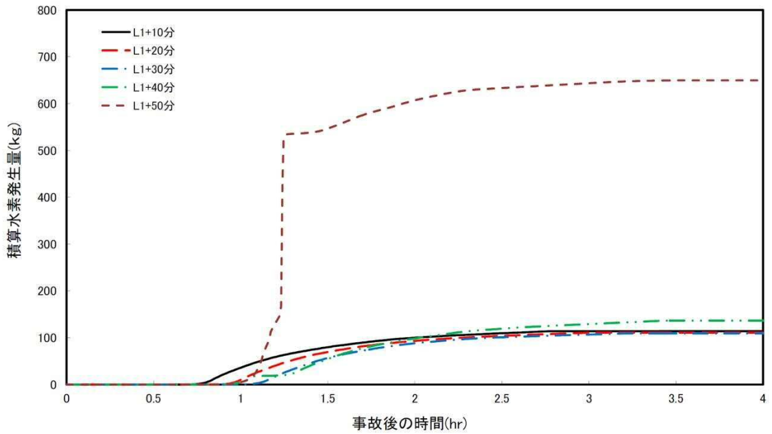
第 2 図 積算水素発生量の時間変化（逃がし安全弁（自動減圧機能）7 弁）
