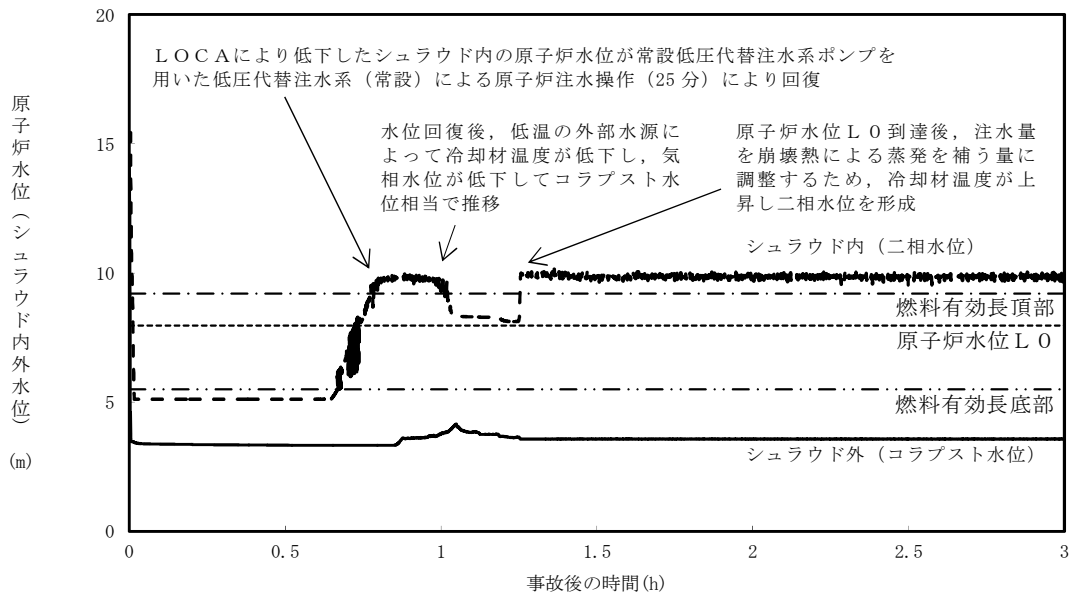
第 3.1.3-6 図 原子炉水位 (シユラウド内外水位) の推移 (~3 時間)
