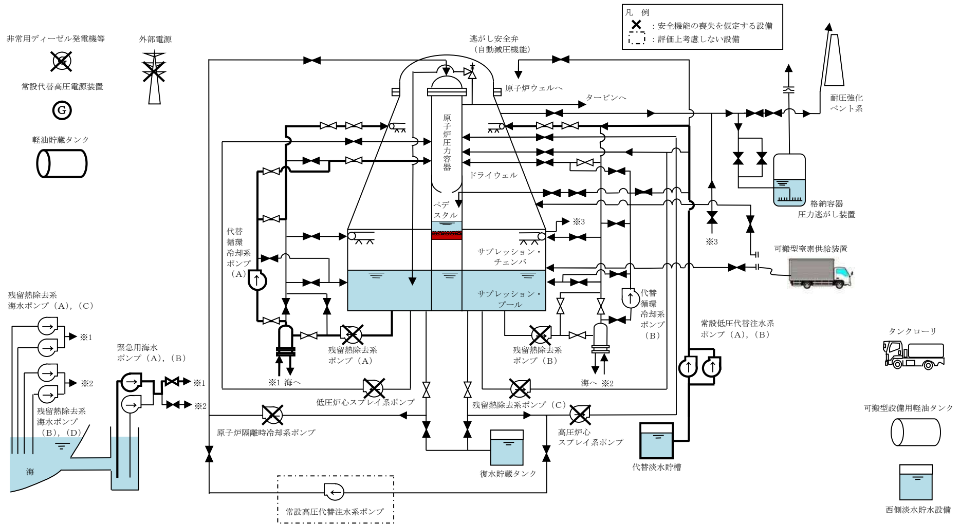
第 3.2-1 図 高圧溶融物放出／格納容器雰囲気直接加熱時の重大事故等対処設備の概略系統図(4/5) (原子炉压力容器破損後の代替循環冷却系による原子炉注水及び格納容器除熱、 代替格納容器スプレー冷却系(常設)による格納容器圧力制御段階)
