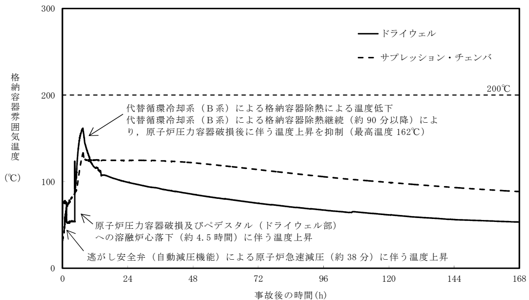
第 8 図 「DCH, FCI, MCCI」における 代替循環冷却系 (B系) を使用した場合の格納容器雰囲気温度の推移
