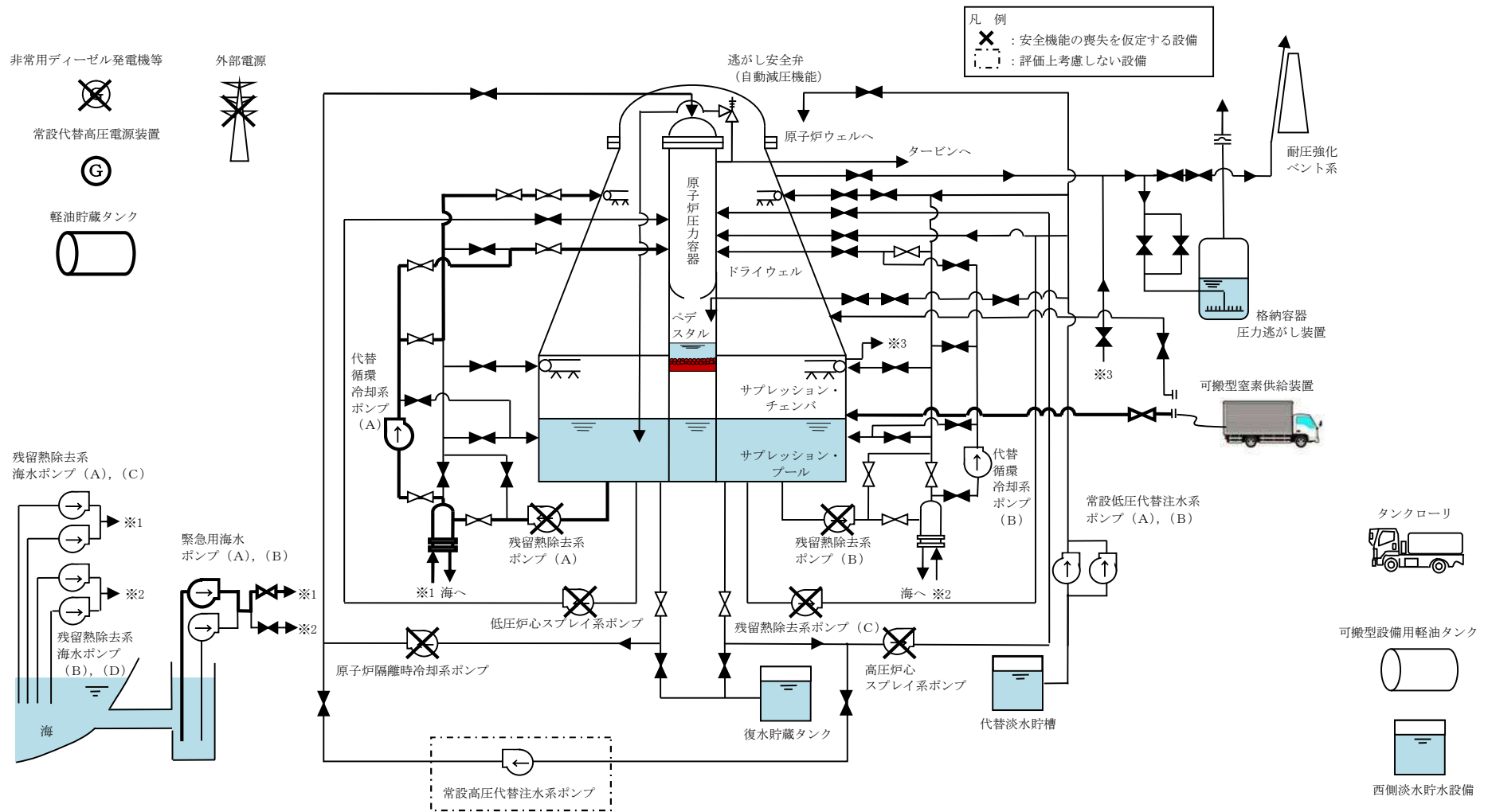
第 3.2-1 図 高压溶融物放出／格納容器雰囲気直接加熱時の重大事故等対処設備の概略系統図(5/5) (原子炉压力容器破損後の代替循環冷却系による原子炉注水及び格納容器除熱、 可搬型窒素供給装置を用いた格納容器内窒素供給段階)
