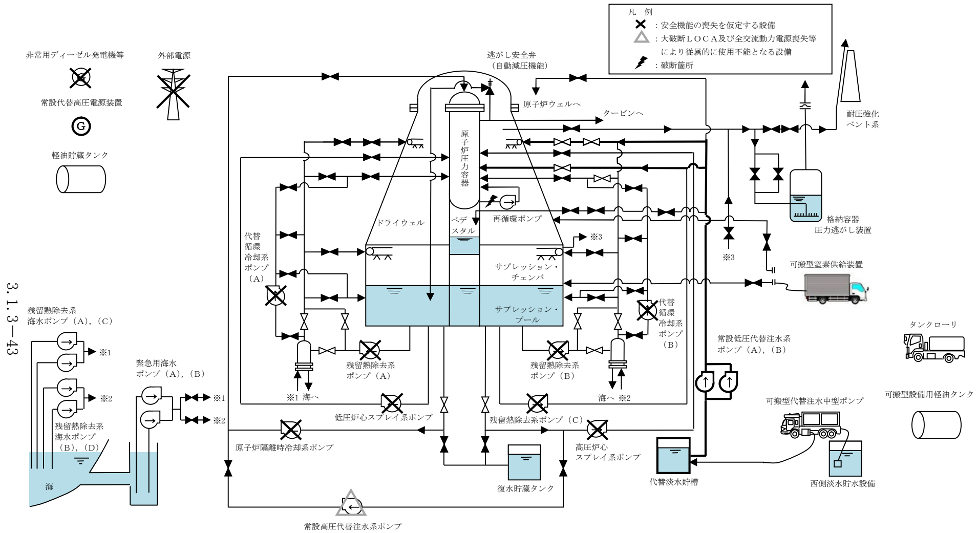
第 3.1.3-1 図 「雰囲気圧力・温度による静的負荷（格納容器過圧・過温破損）」の 重大事故等対策の概略系統図（代替循環冷却系を使用できない場合）（1/2） （低压代替注水系（常設）による原子炉注水，代替格納容器スプレイ冷却系（常設）による格納容器冷却段階）
