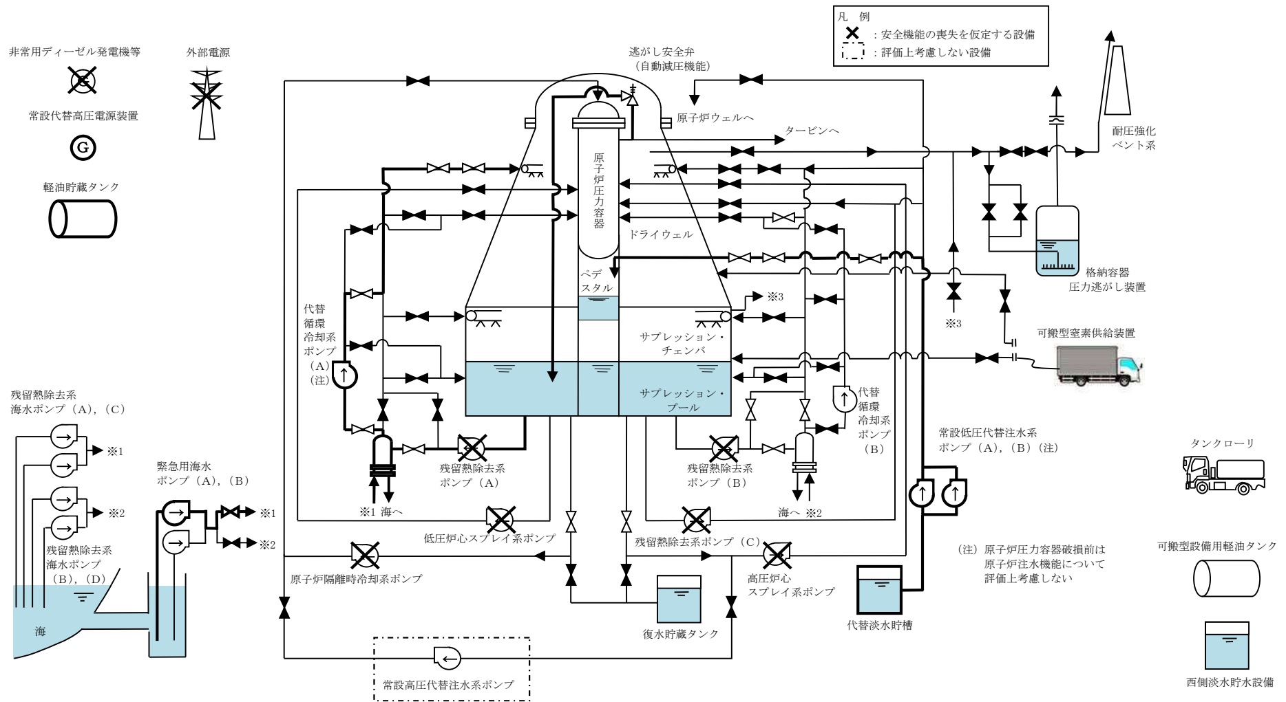
第 3.2-1 図 高圧溶融物放出／格納容器雰囲気直接加熱時の重大事故等対処設備の概略系統図 (2/5) (原子炉圧力容器破損前の代替循環冷却系による格納容器除熱及び格納容器下部注水系 (常設) による格納容器下部水位確保段階)
