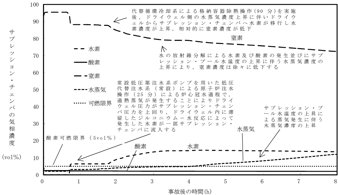
第 7.2.4-6 図 サプレッション・チェンバの気相濃度の推移 (ウェット条件) (~8 時間)
