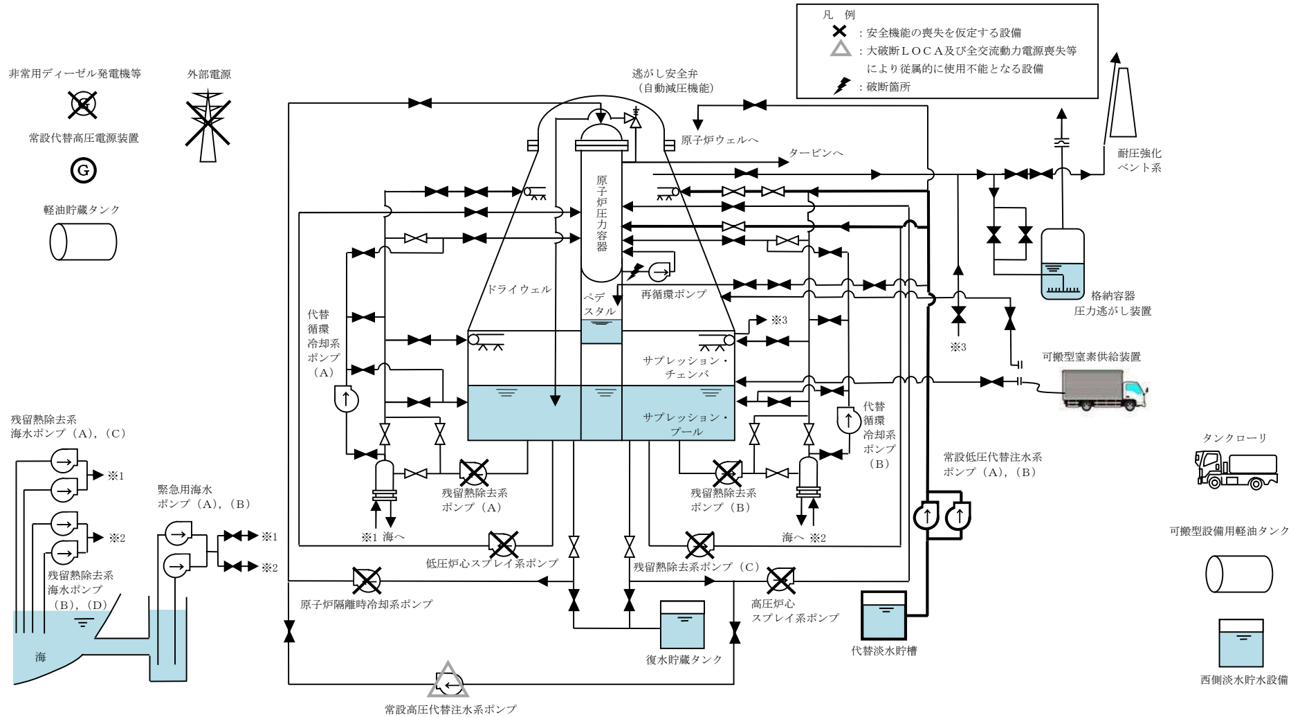
第3.1.2-1図 「雰囲気圧力・温度による静的負荷（格納容器過圧・過温破損）」の重大事故等対策の概略系統図（代替循環冷却系を使用する場合）（1/3） （低压代替注水系（常設）による原子炉注水，代替格納容器スプレー冷却系（常設）による格納容器冷却段階）
