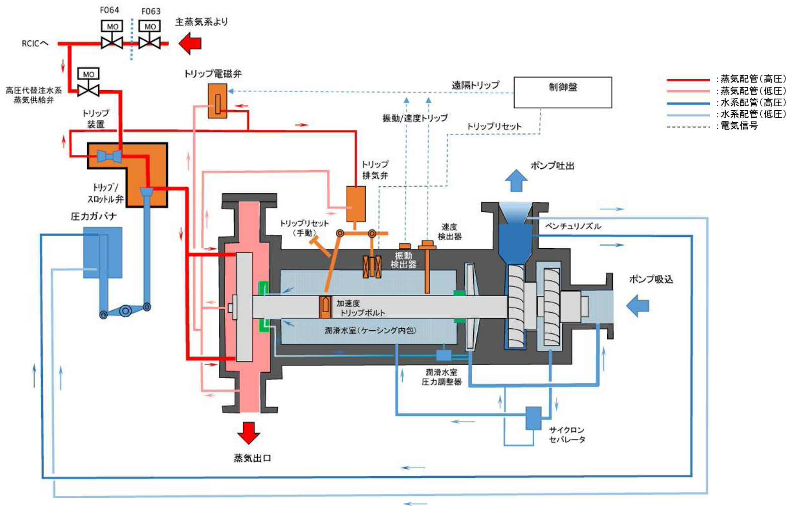
第2図 高圧代替注水系ポンプ周り系統図
