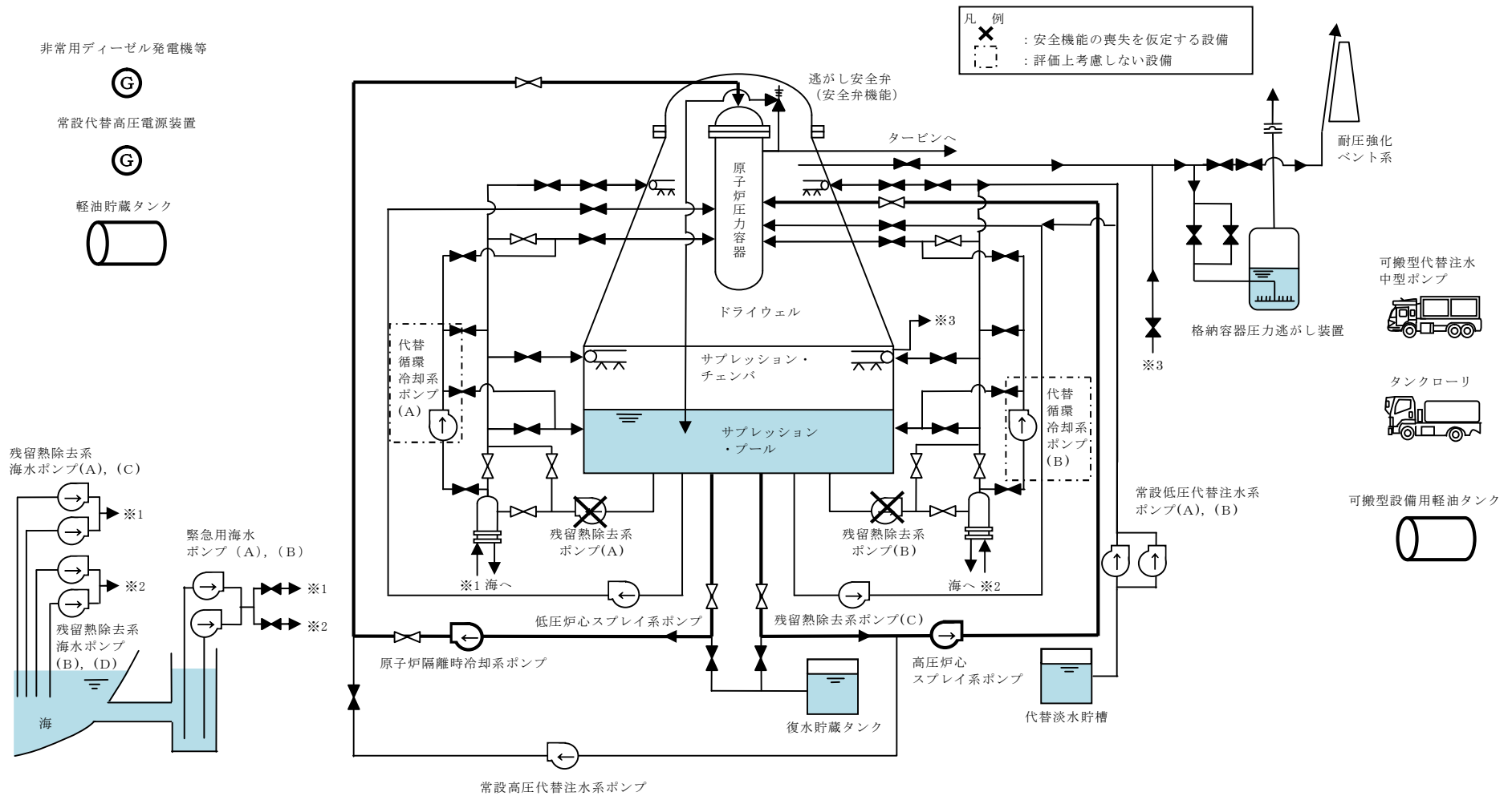
第 2.4.2-1 図 崩壊熱除去機能喪失（残留熱除去系が故障した場合）時の重大事故等対策の概略系統図（1/4） （高压炉心スプレー系及び原子炉隔離時冷却系による原子炉注水段階）
