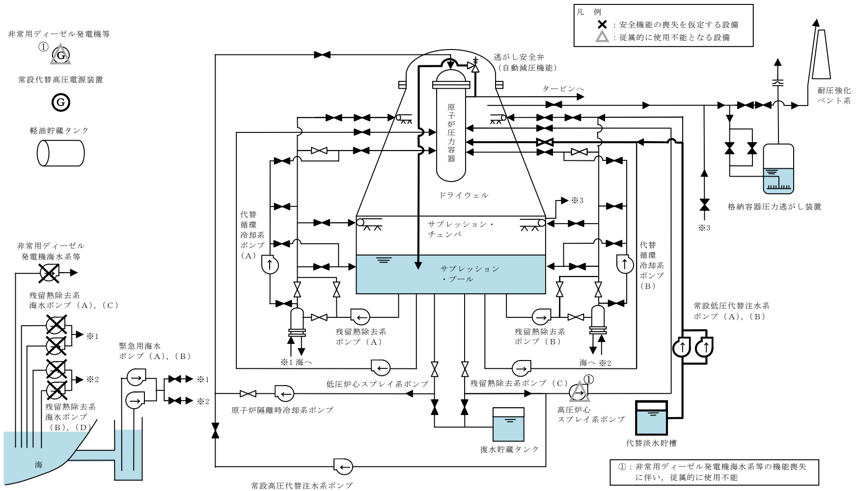
第 2.4.1-1 図 崩壊熱除去機能喪失（取水機能が喪失した場合）時の重大事故等対策の概略系統図（2/3） （常設低圧代替注水系ポンプを用いた低圧代替注水系（常設）による原子炉注水段階）
