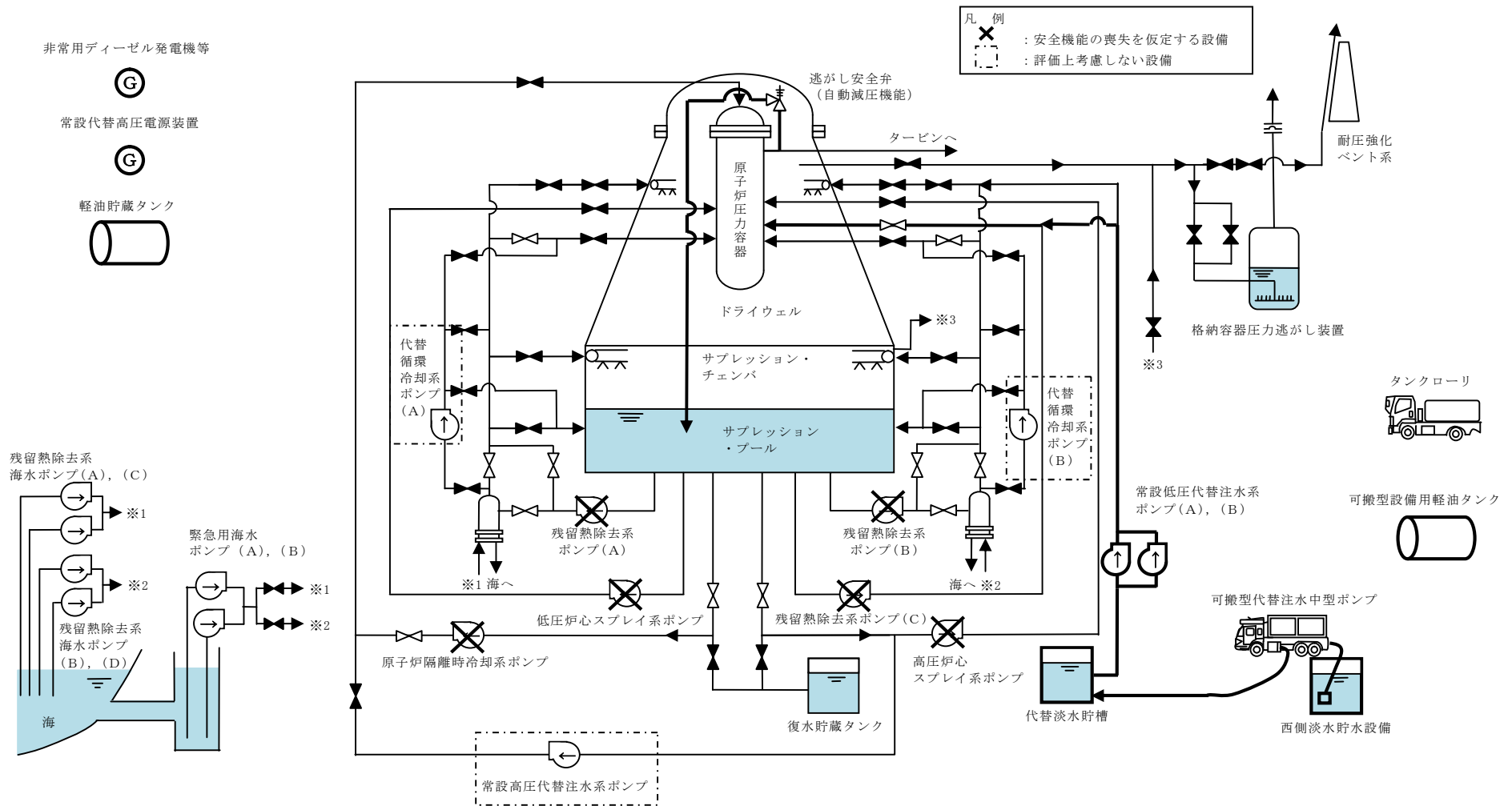
第 2.1-1 図 高压・低圧注水機能喪失時の重大事故等対策の概略系統図 (1/3) (常設低圧代替注水系ポンプを用いた低圧代替注水系 (常設) による原子炉注水段階)
