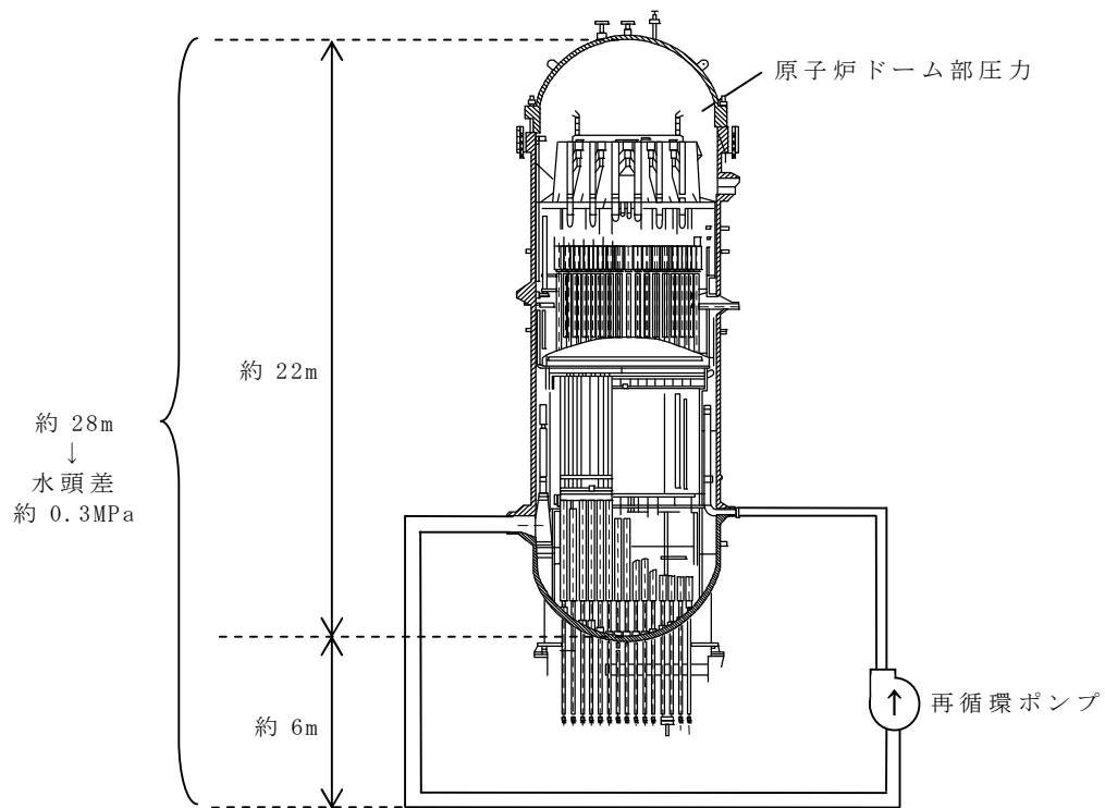
第1図 原子炉冷却材圧力バウンダリにかかる圧力の概要図
