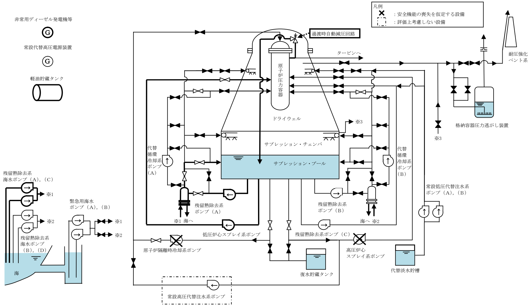
第 2.2-1 図 高压注水・減圧機能喪失時の重大事故等対策の概略系統図 (2/2) (低圧炉心スプレイ系による原子炉注水及び残留熱除去系による格納容器除熱段階)
