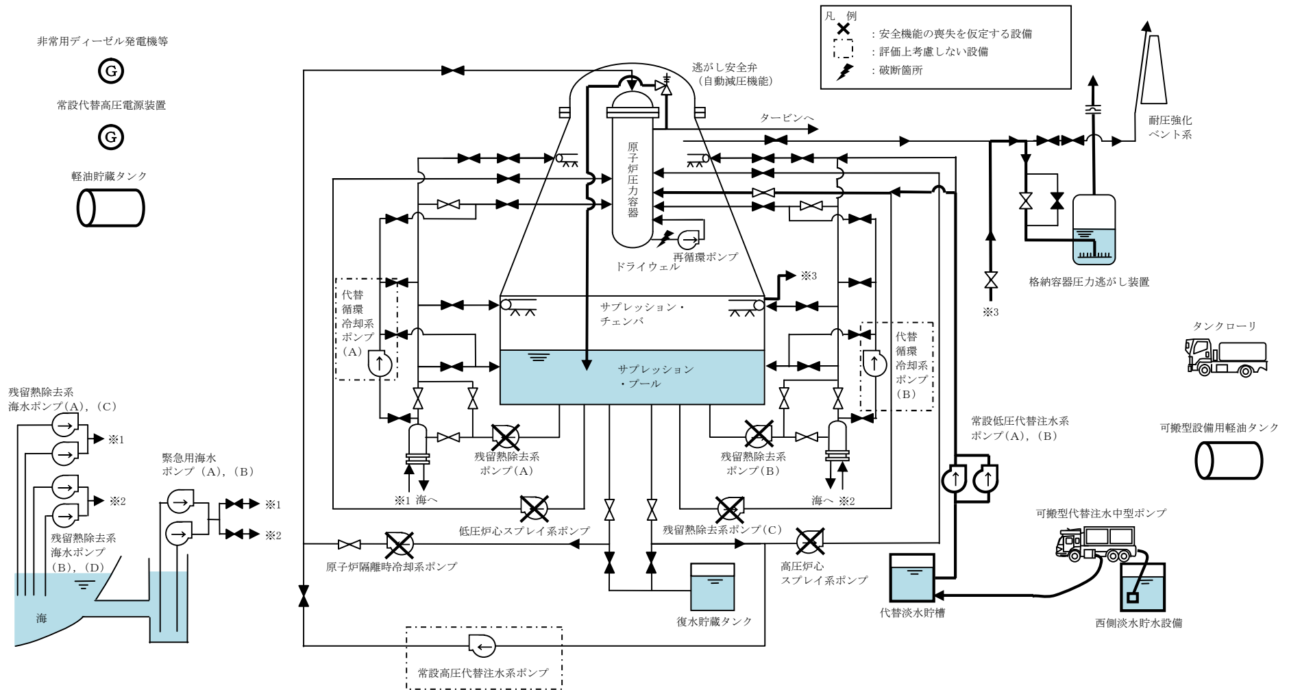
第 2.6-1 図 LOCA時注水機能喪失時の重大事故等対策の概略系統図 (3/3) (常設低圧代替注水系ポンプを用いた低圧代替注水系 (常設) による原子炉注水及び 格納容器圧力逃がし装置による格納容器除熱段階)
