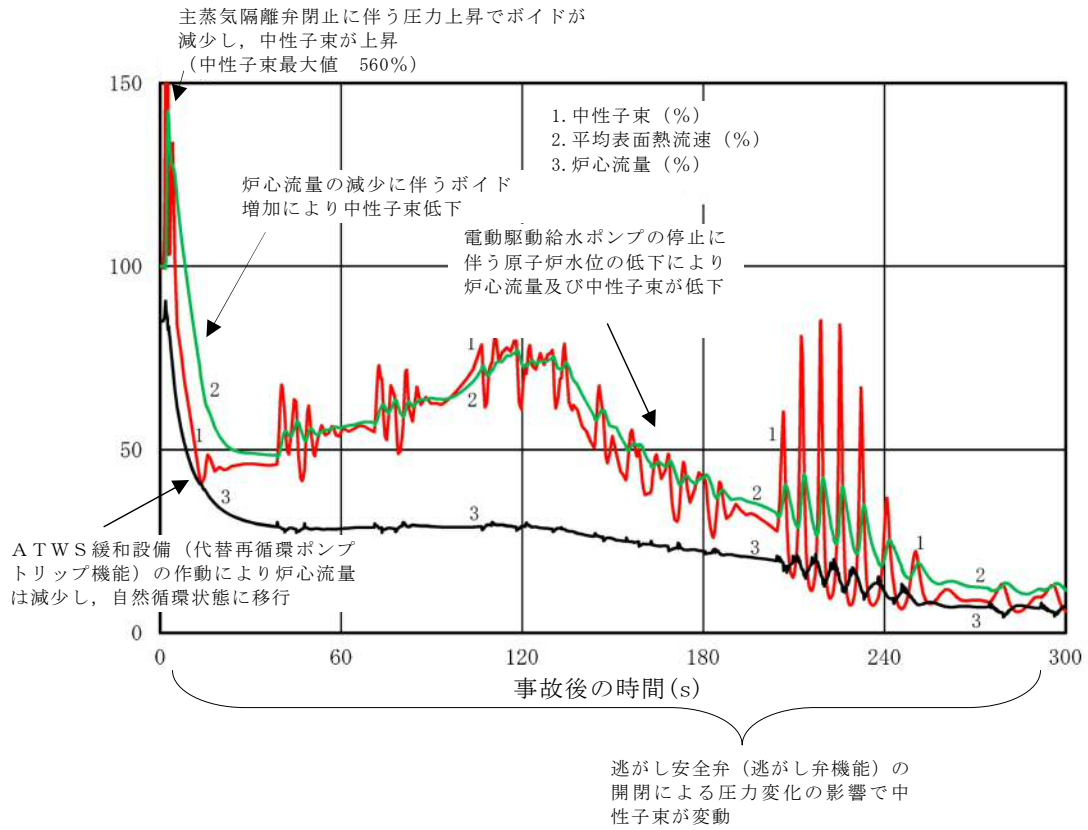
第 2.5-4 図 中性子束、平均表面熱流束及び炉心流量の推移 (短期)
