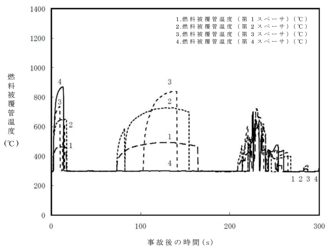
第 2 図 燃料被覆管温度の推移 (ベースケース (相関式 2))
