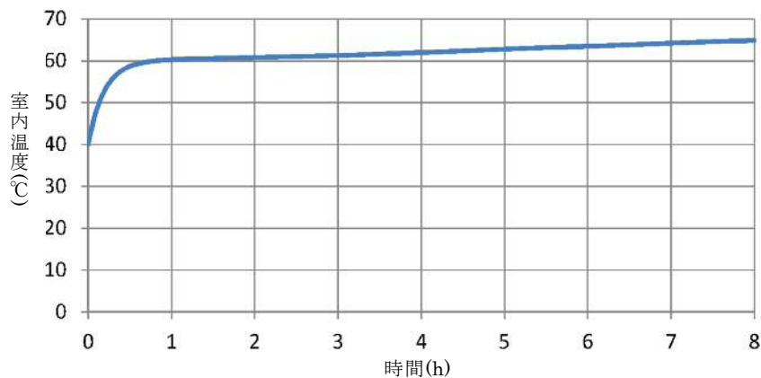
第 6 図 高圧代替注水系ポンプ室温の推移
