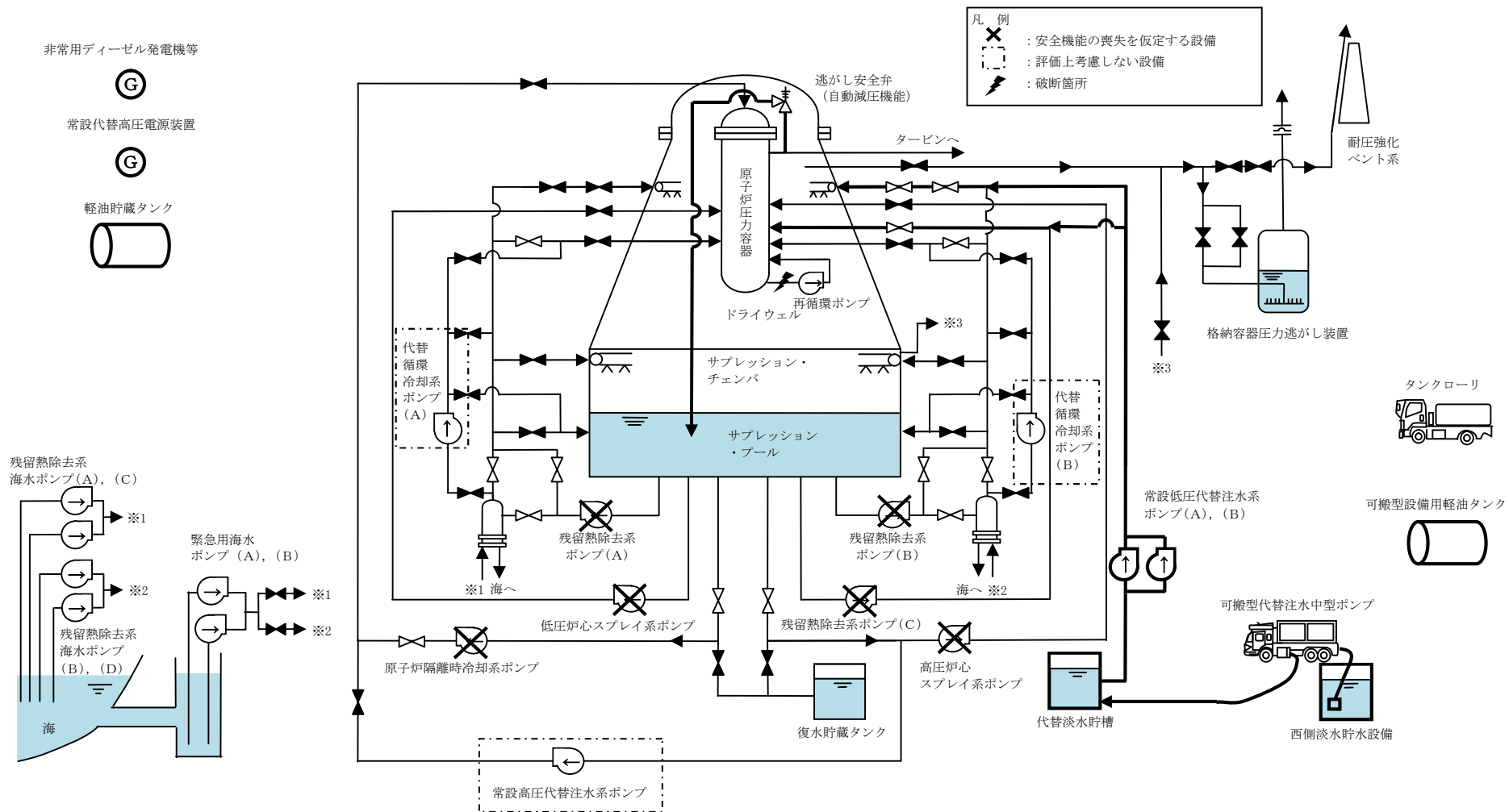
第 2.6-1 図 LOCA時注水機能喪失時の重大事故等対策の概略系統図 (2/3) (常設低圧代替注水系ポンプを用いた低圧代替注水系 (常設) による原子炉注水及び代替格納容器スプレイ冷却系 (常設) による格納容器冷却段階)
