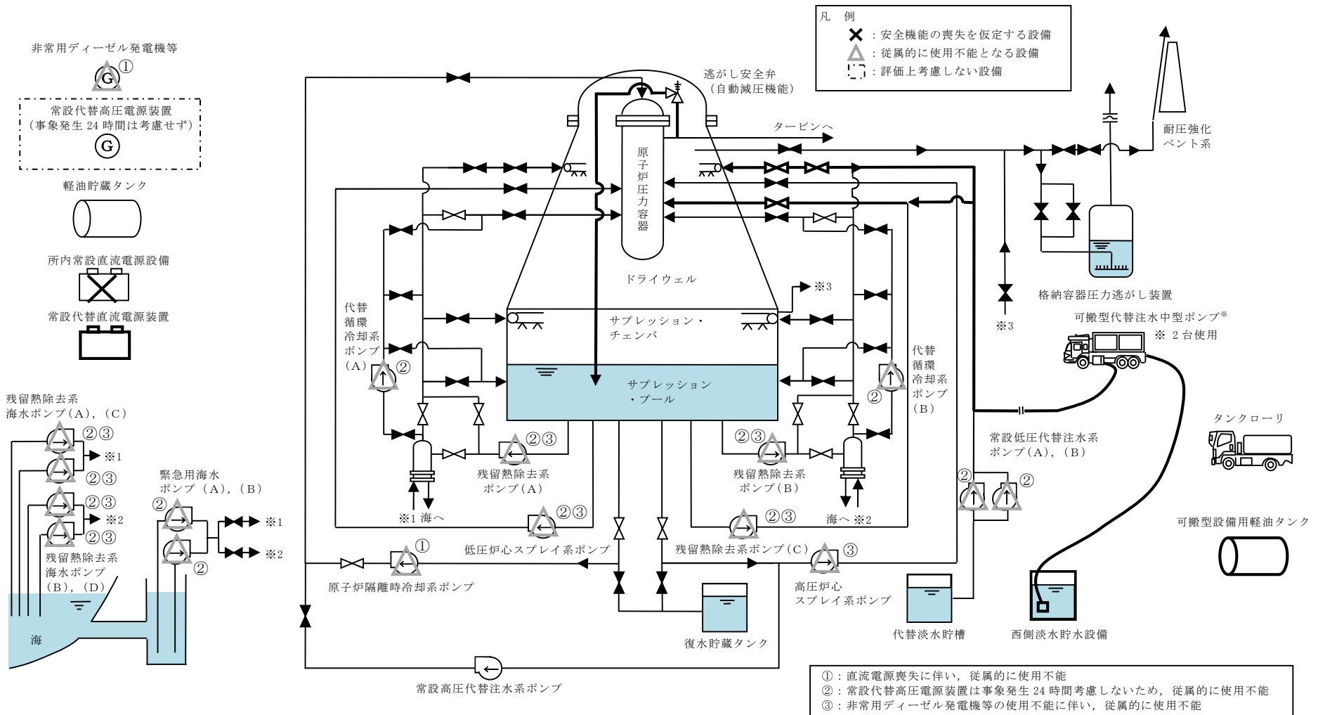
第 2.3.2-1 図 全交流動力電源喪失 (TBD, TBU) 時の重大事故等対策の概略系統図 (2/3) (可搬型代替注水中型ポンプを用いた低压代替注水系 (可搬型) による原子炉注水及び 代替格納容器スプレイ冷却系 (可搬型) による格納容器冷却段階)
