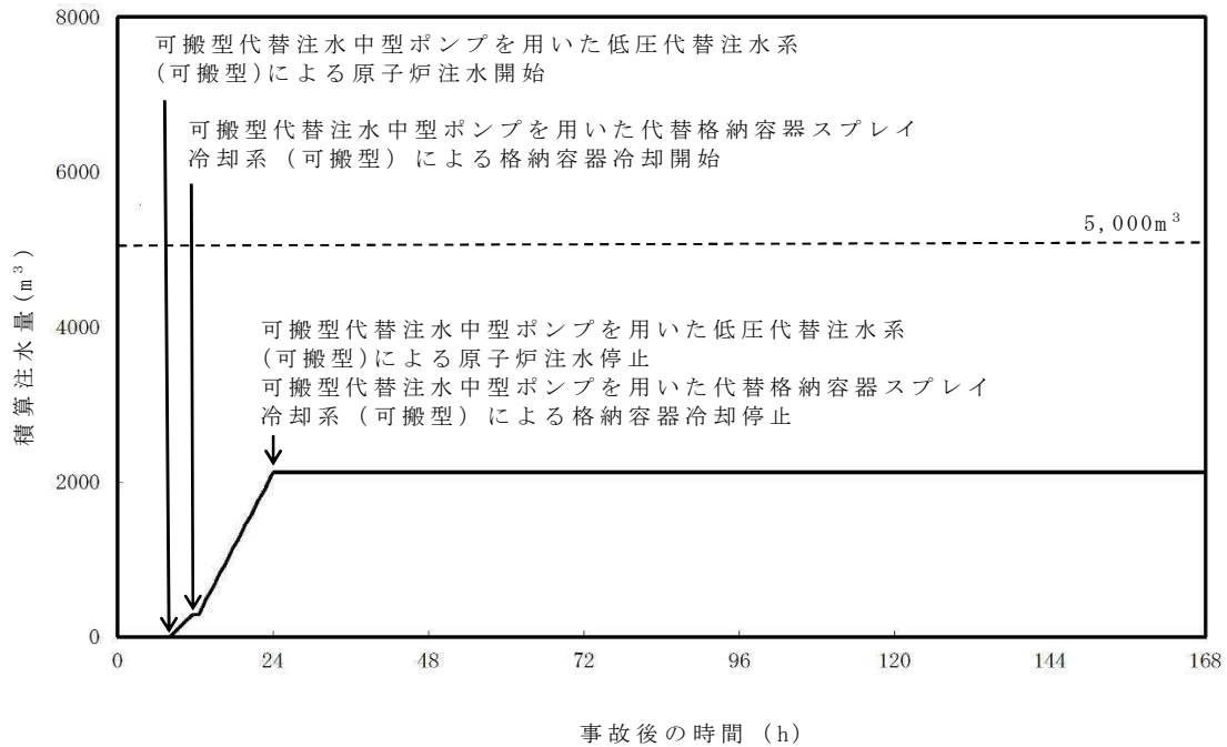
第 1 図 外部水源による積算注水量 (全交流動力電源喪失 (T B D , T B U))
