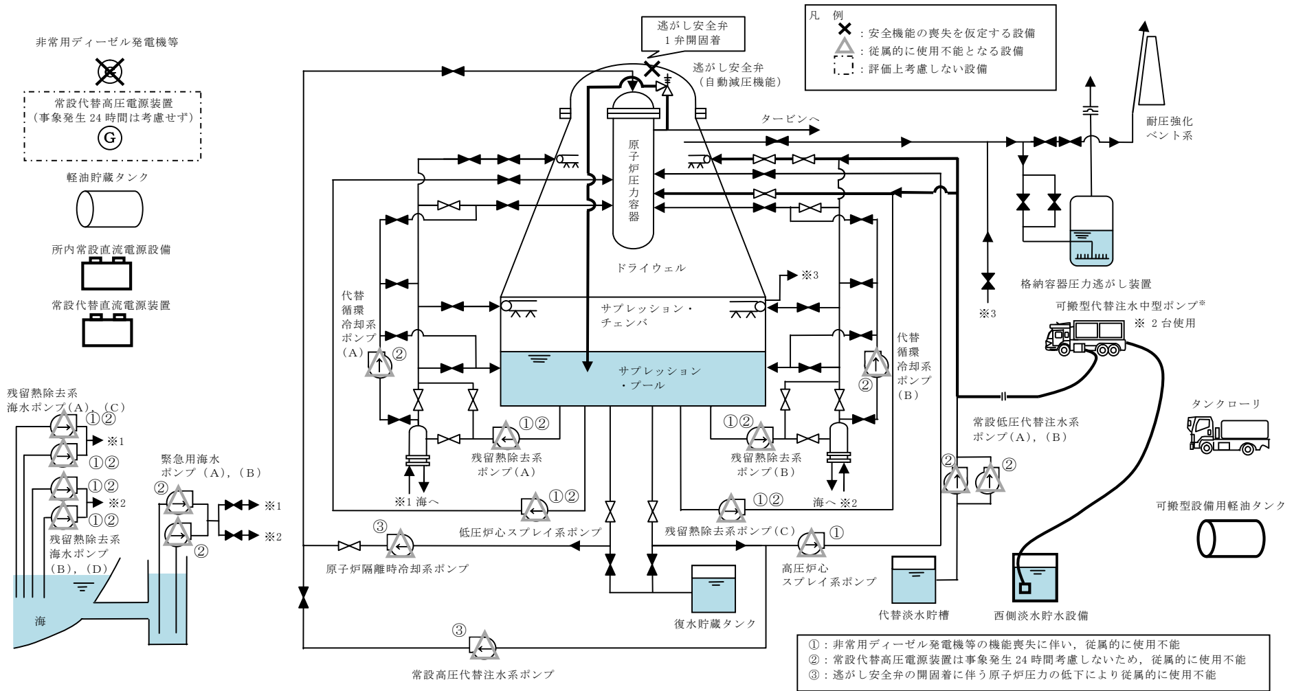
第 2.3.3-1 図 全交流動力電源喪失 (TBP) 時の重大事故等対策の概略系統図 (2/3) (可搬型代替注水中型ポンプを用いた低圧代替注水系 (可搬型) による原子炉注水及び 代替格納容器スプレー冷却系 (可搬型) による格納容器冷却段階)
