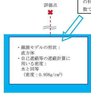
制御棒の線源モデル (冠水時)
