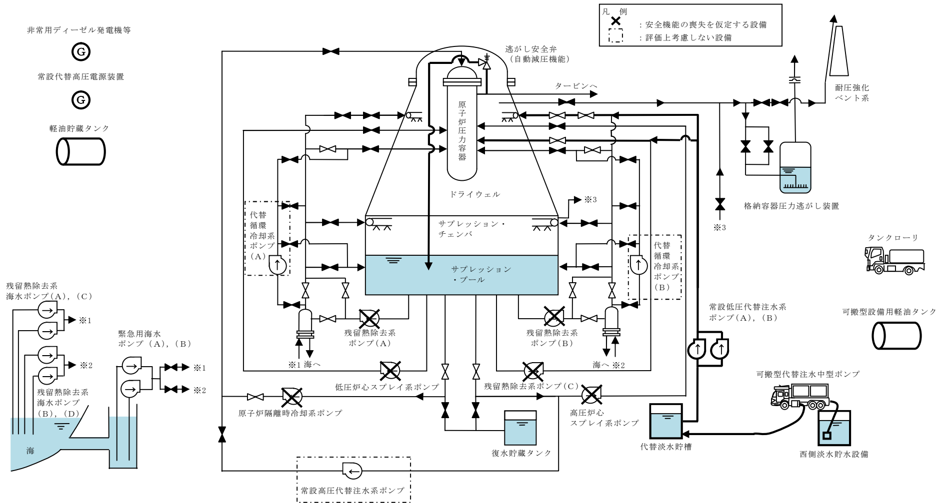
第 2.1-1 図 高压・低圧注水機能喪失時の重大事故等対策の概略系統図 (2/3)
