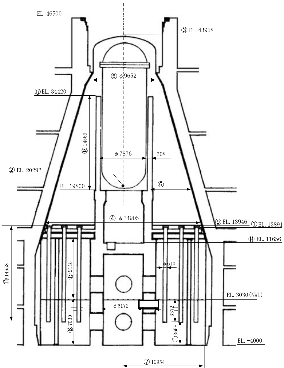
図 2.2 原子炉格納容器形状に関するデータ
