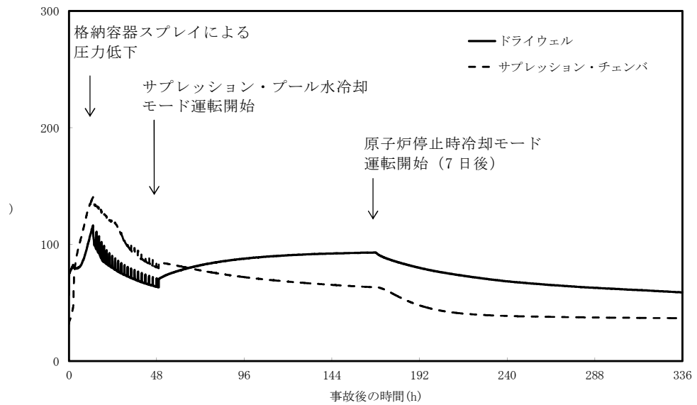
第5図 格納容器雰囲気温度の推移
