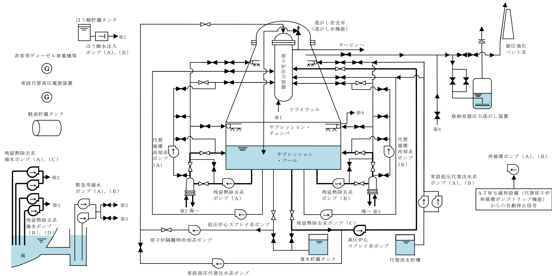
第 2.5-1 図 原子炉停止機能喪失時の重大事故等対策の概略系統図 (3/3) (高压炉心スプレイ系による原子炉注水及び 残留熱除去系 (サブプレッション・プール水冷却系) による格納容器除熱段階)
