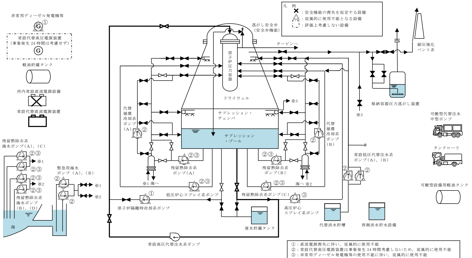
第 2.3.2-1 図 全交流動力電源喪失 (TBD, TBU) 時の重大事故等対策の概略系統図 (1/3) (高压代替注水系による原子炉注水段階)
