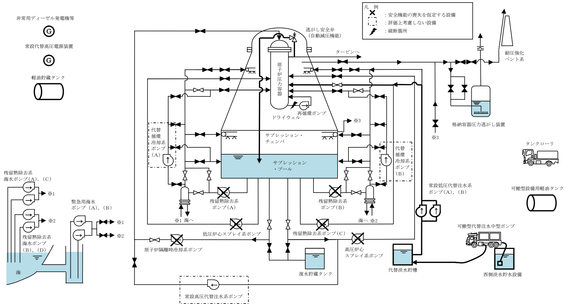
第 2.6-1 図 LOCA時注水機能喪失時の重大事故等対策の概略系統図 (1/3) (常設低压代替注水系ポンプを用いた低压代替注水系(常設)による原子炉注水段階)
