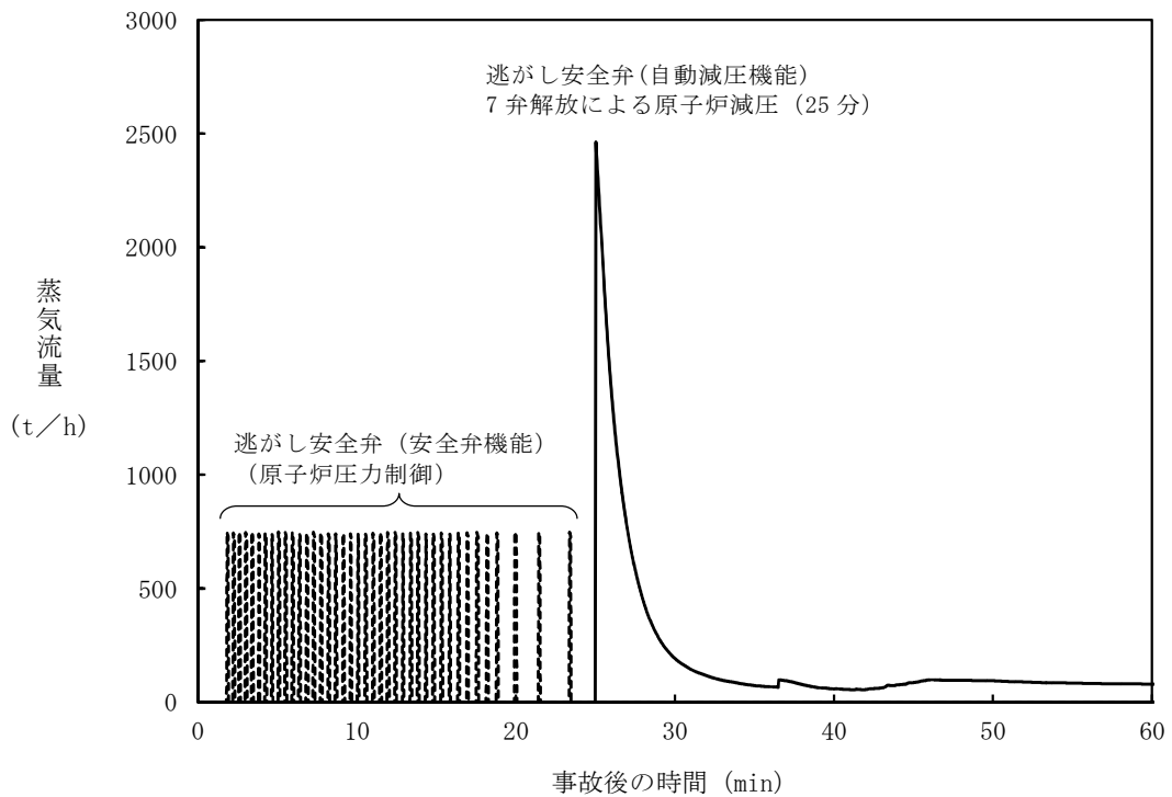
第 2.6-23 図 逃がし安全弁からの蒸気流量の推移 (約 9.5cm 2 の破断)
