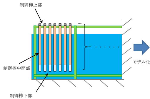
使用済制御棒の側面図
