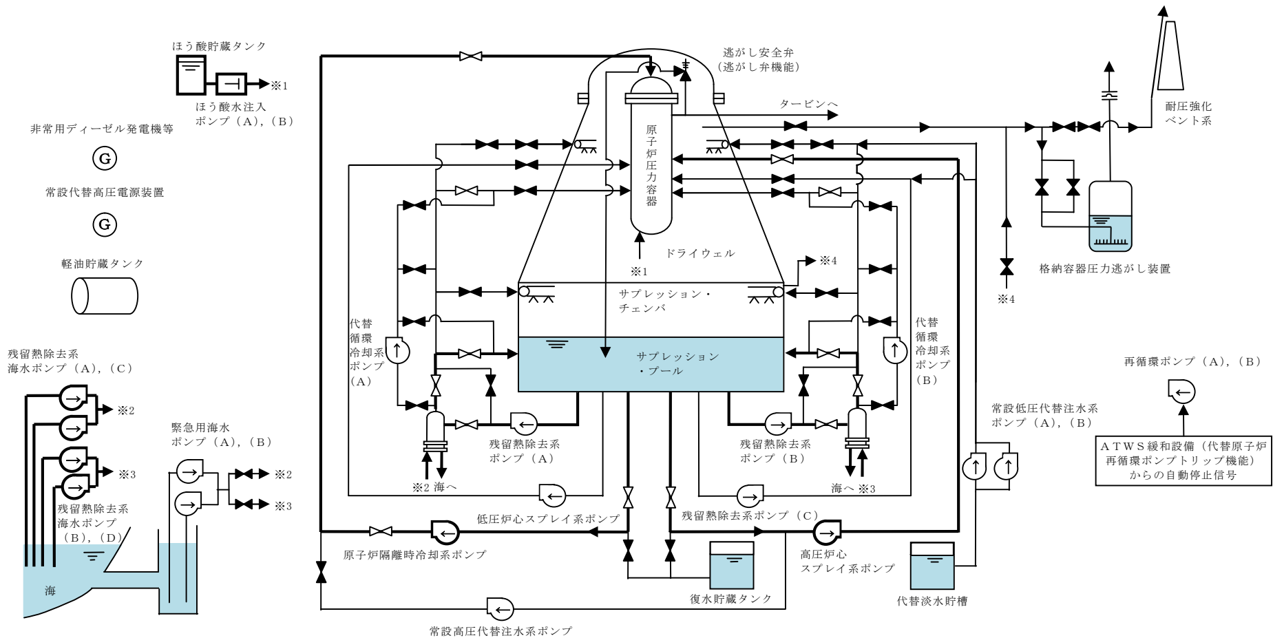
第 2.5-1 図 原子炉停止機能喪失時の重大事故等対策の概略系統図 (2/3) (高圧炉心スプレー系及び原子炉隔離時冷却系による原子炉注水, ほう酸注入系による原子炉停止並びに 残留熱除去系 (サブプレッション・プール水冷却系) による格納容器除熱段階)
