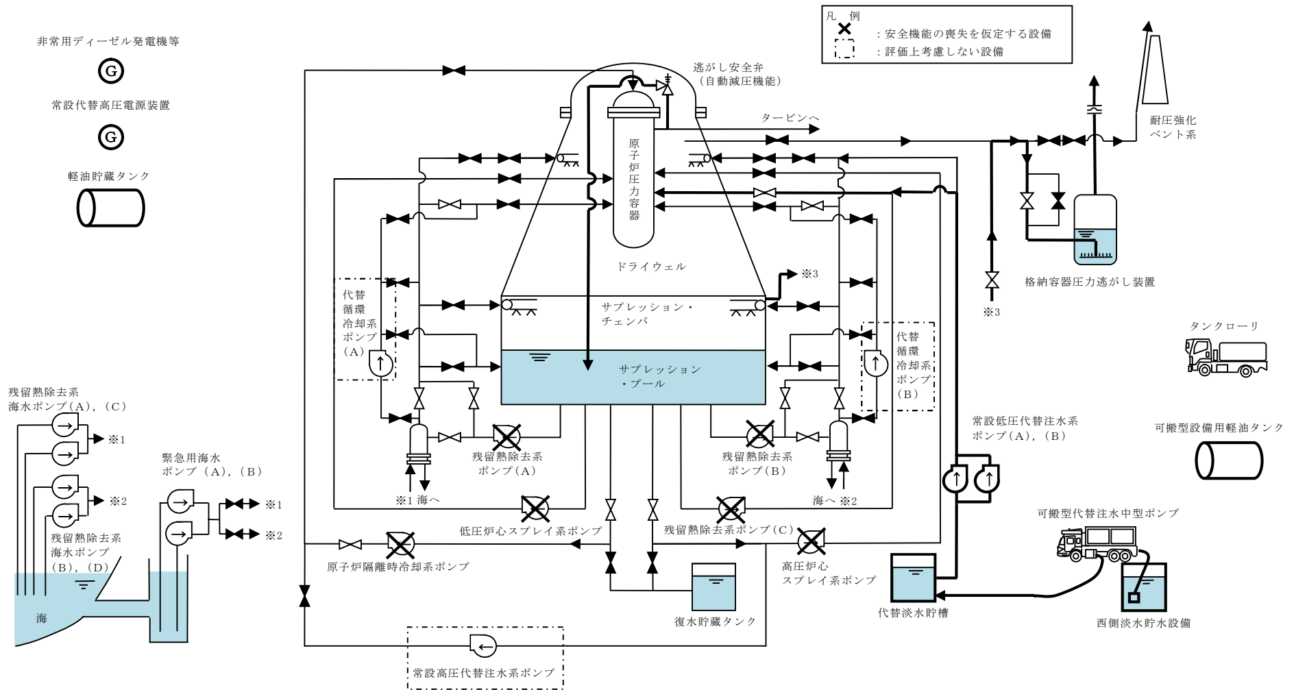
第 2.1-1 図 高压・低圧注水機能喪失時の重大事故等対策の概略系統図 (3/3)
