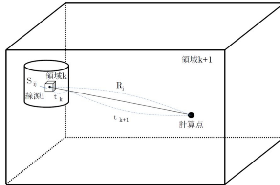
第9図 QAD-CGGP2Rコードの計算体
