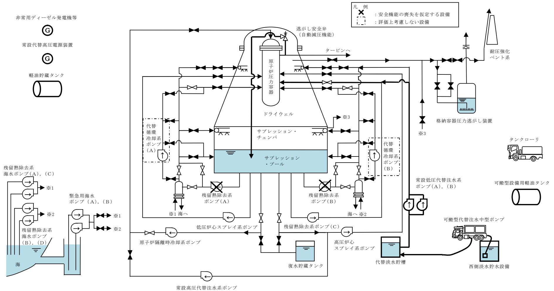
第 2.4.2-1 図 崩壊熱除去機能喪失（残留熱除去系が故障した場合）時の重大事故等対策の概略系統図（2/4） （常設低压代替注水系ポンプを用いた低压代替注水系（常設）による原子炉注水段階）
