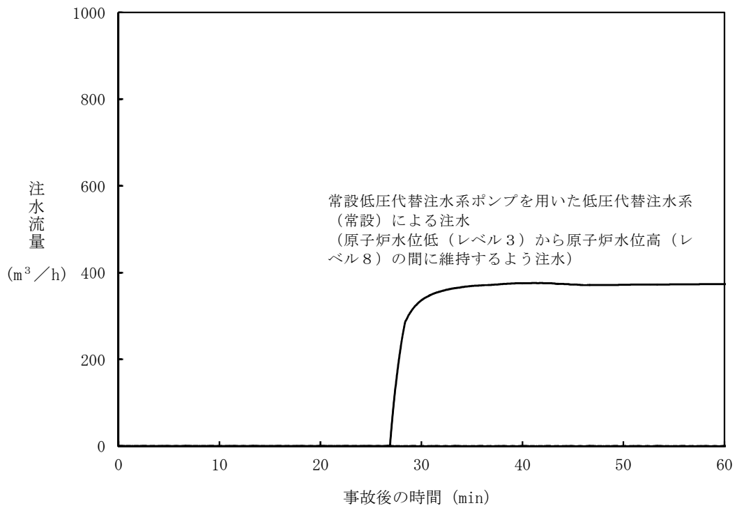
第 2.6-22 図 注水流量の推移 (約 9.5cm 2 の破断)
