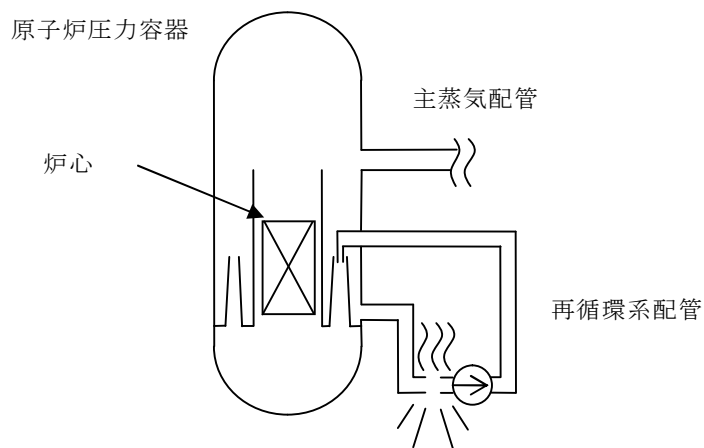
第1図 再循環ポンプ吸込み側配管破断の概要
