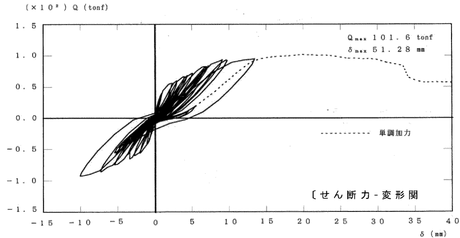
図 1 I 型耐震壁の仮動的試験例
