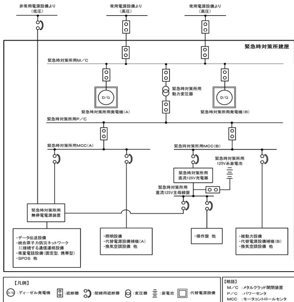
第 2.2-1 図 緊急時対策所 単線結線図
