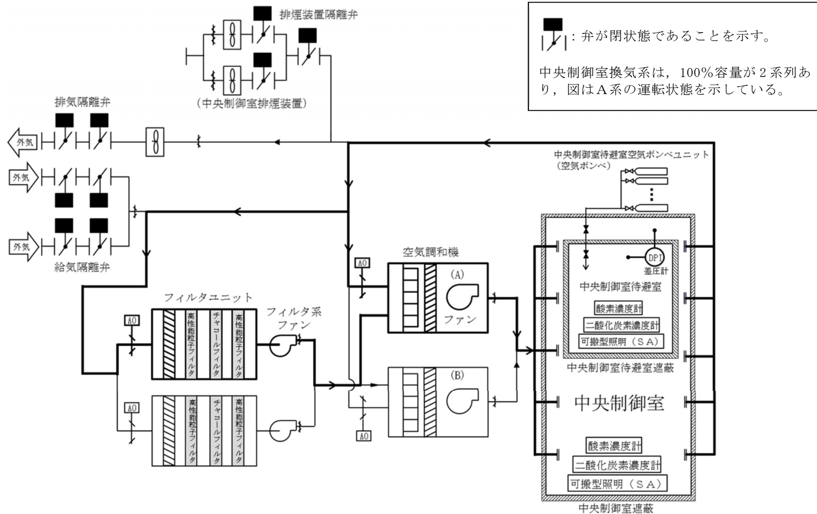
第59-4-1図 中央制御室換気系 系統概要図
