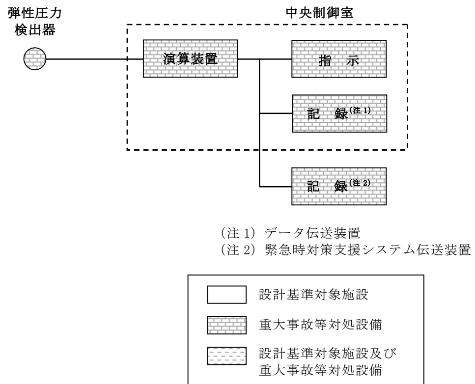
第 58-6-3 図 常設高圧代替注水系ポンプ吐出圧力の概略構成図
