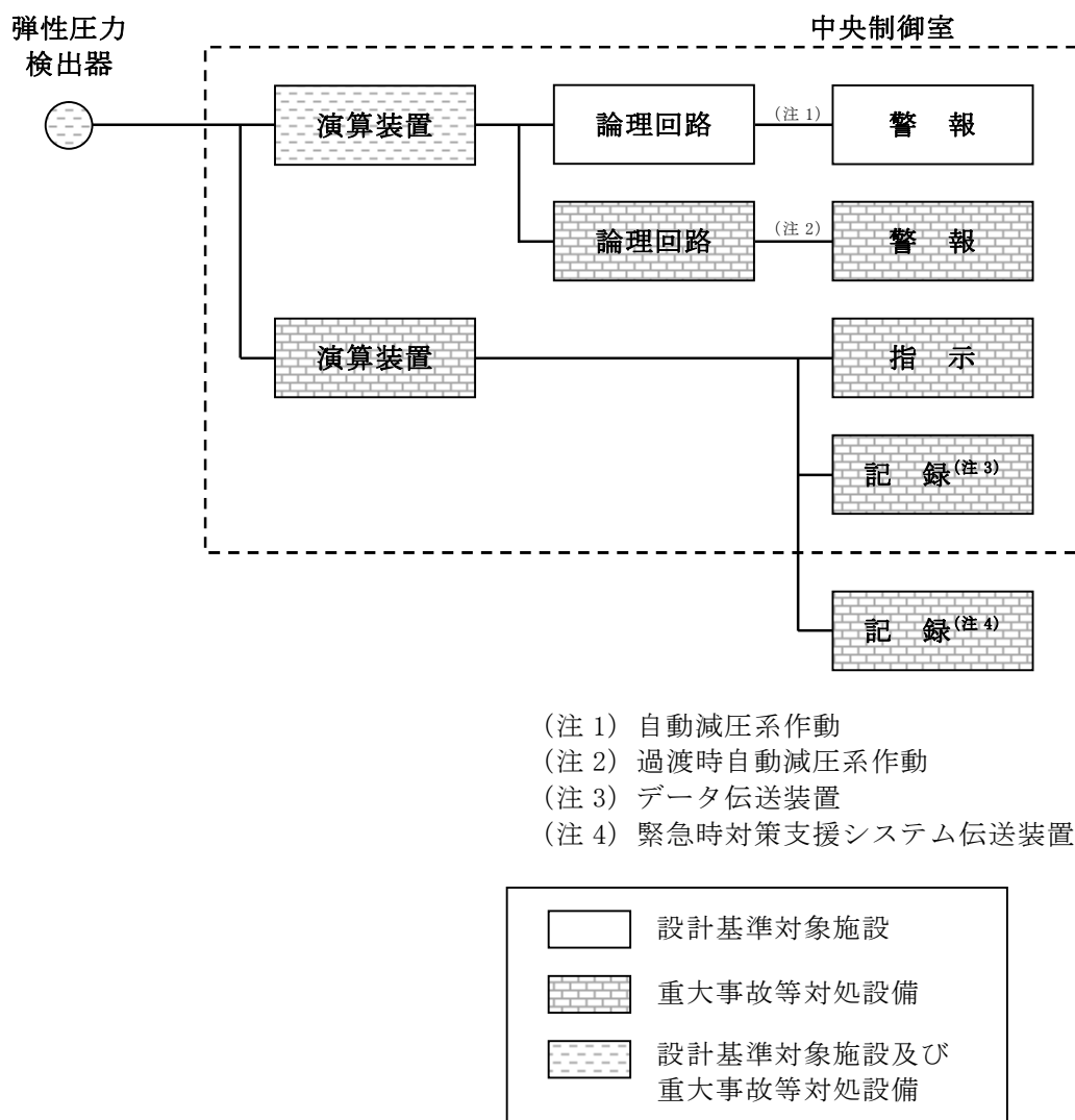
第 58-6-8 図 残留熱除去系ポンプ吐出圧力の概略構成図
