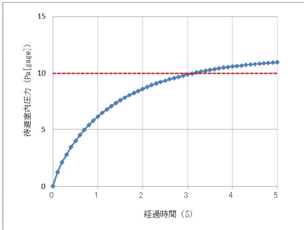
第 2.4-7 図 中央制御室待避室内圧力の時間変化
