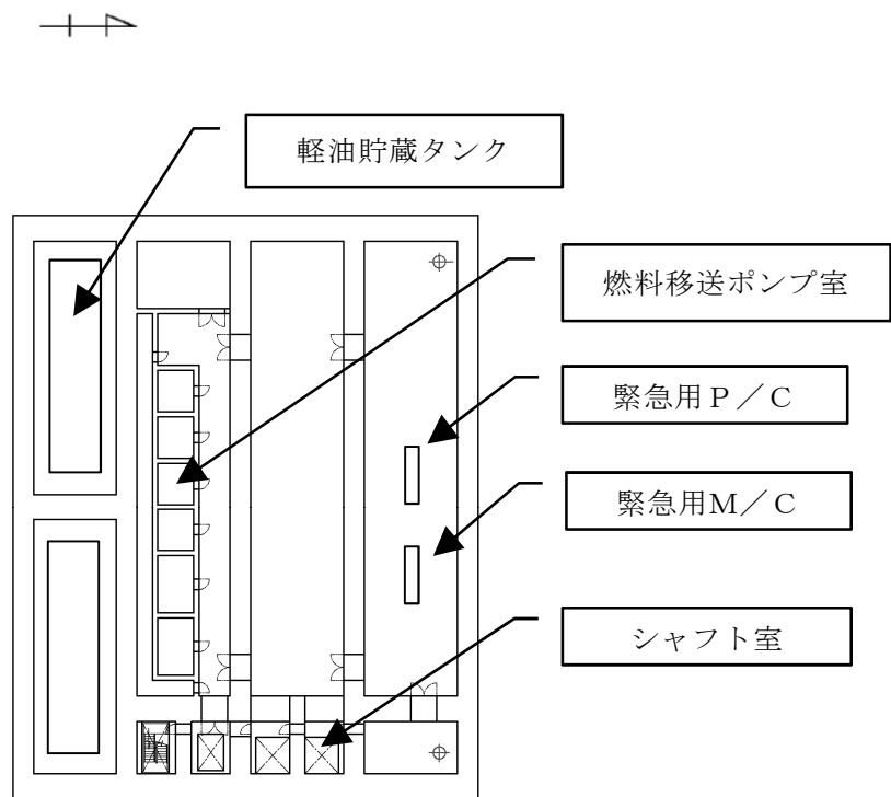
第57-11-7図 常設代替高圧電源装置置場の配置 (T.P. +2.0m) (2/5)
