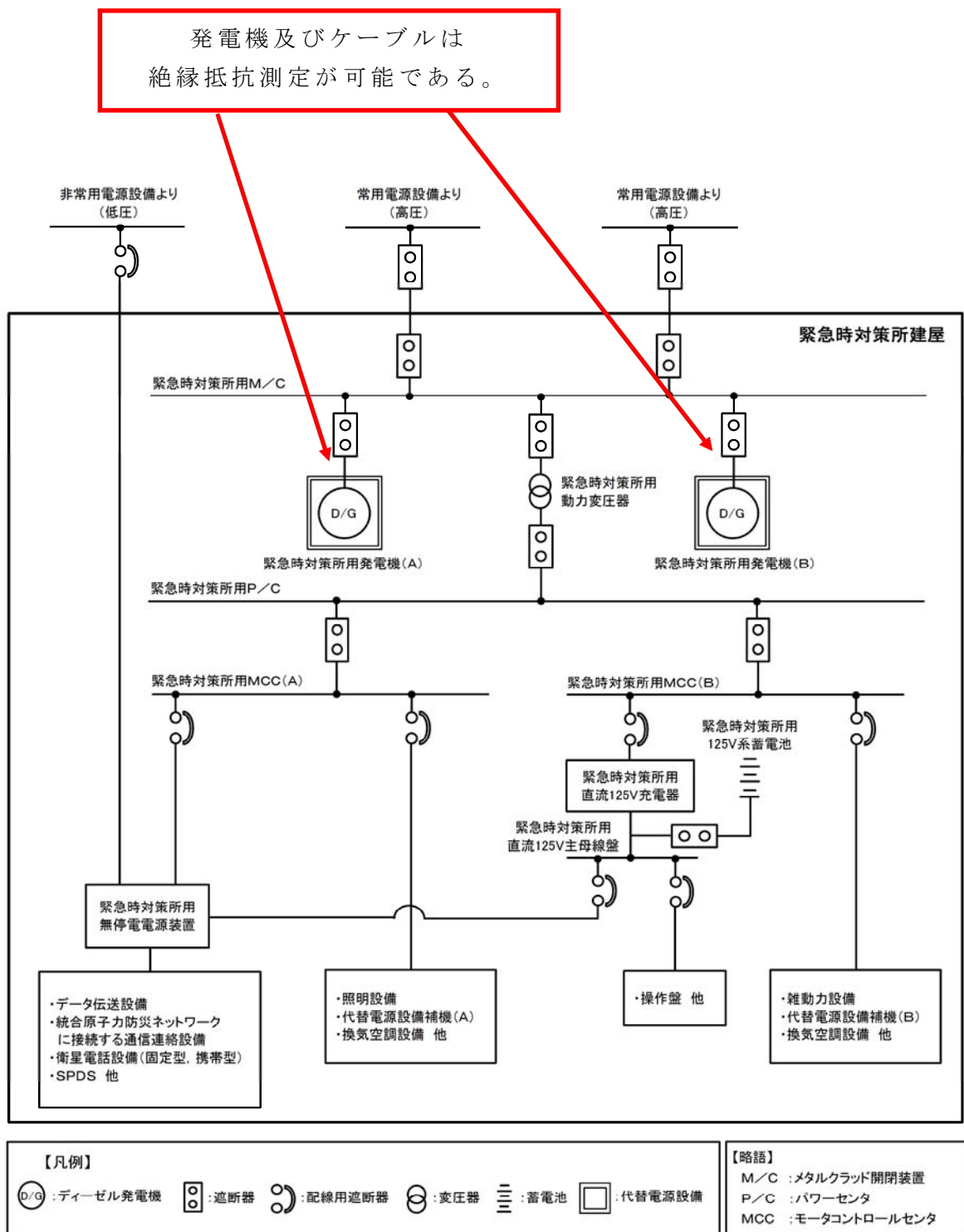
第61-5-4図 緊急時対策所用発電機 検査系統図
