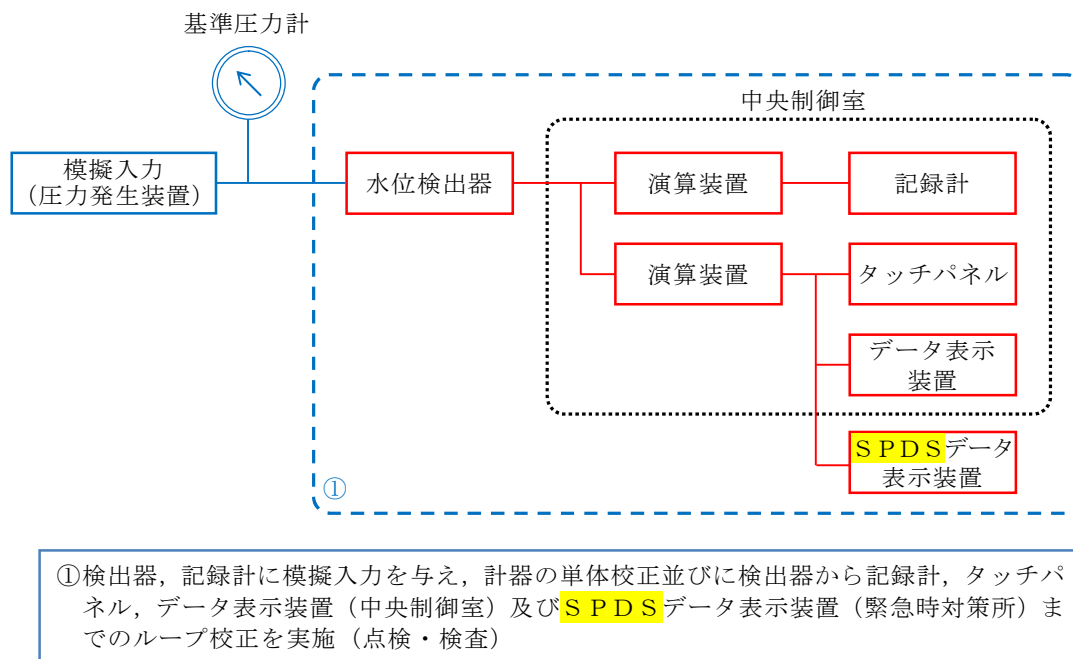
第 58-5-1 図 水位計の試験及び検査
