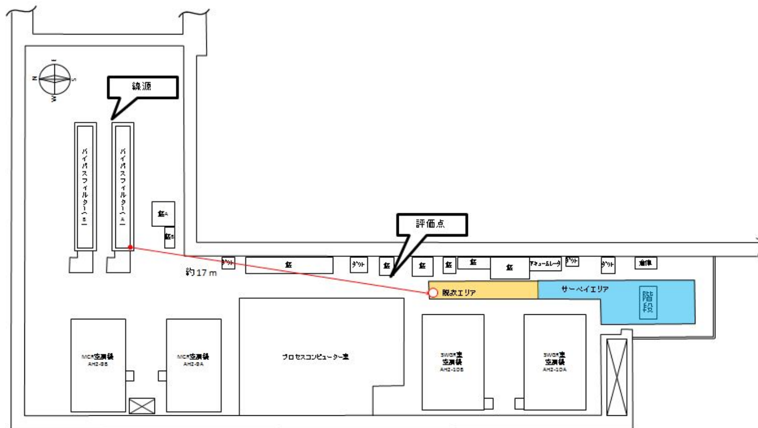
第 10-1 図 線源，チェンジングエリア及び評価点の位置関係
