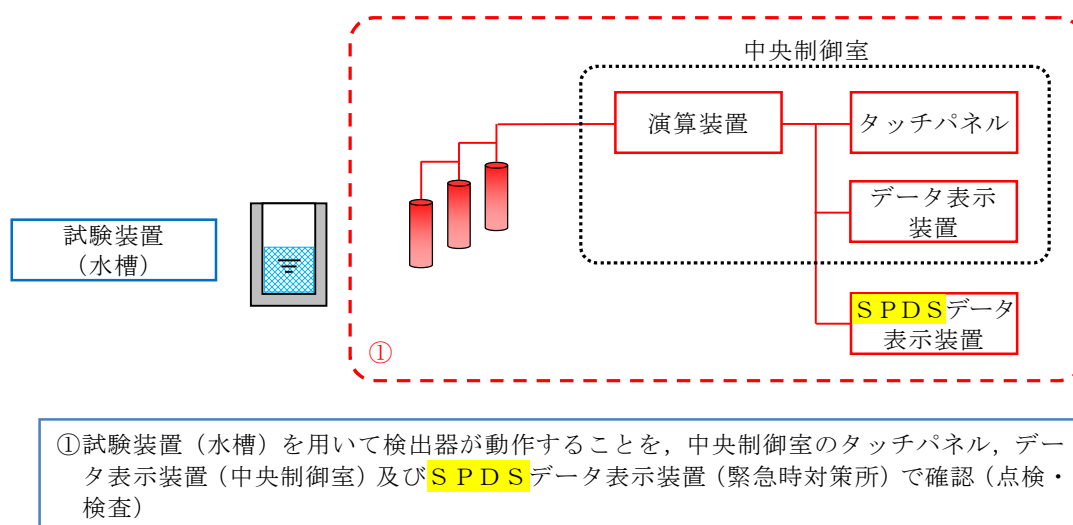
第 58-5-2 図 水位計の試験及び検査 (格納容器下部水位)
