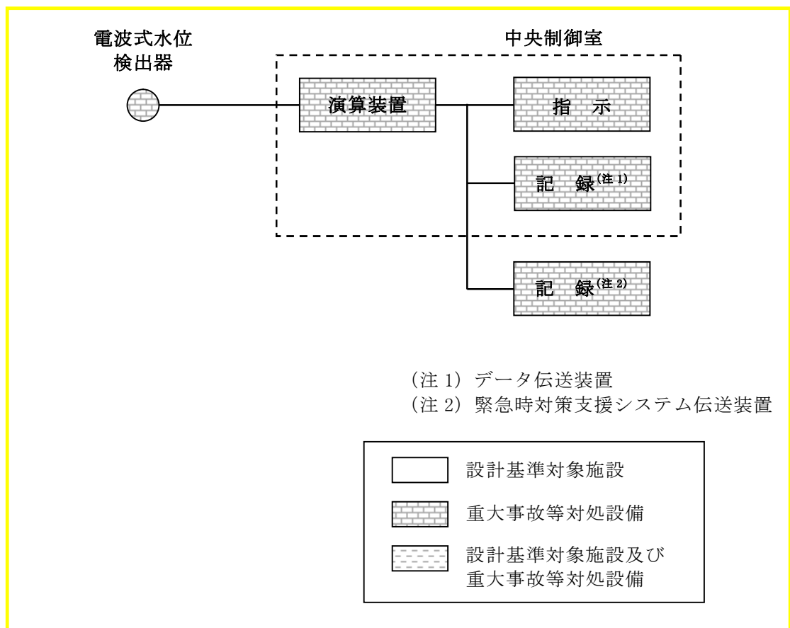
第 58-6-53 図 西側淡水貯水設備水位の概略構成図
