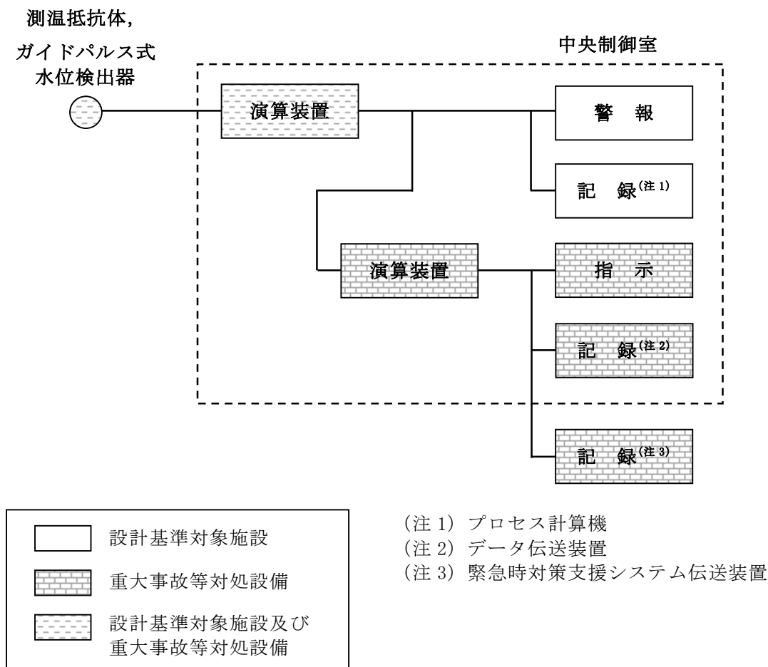
第 58-6-55 図 使用済燃料プール水位・温度（S A 広域）概略構成図
