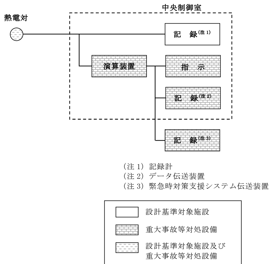
第 58-6-12 図 残留熱除去系熱交換器出口温度の概略構成図
