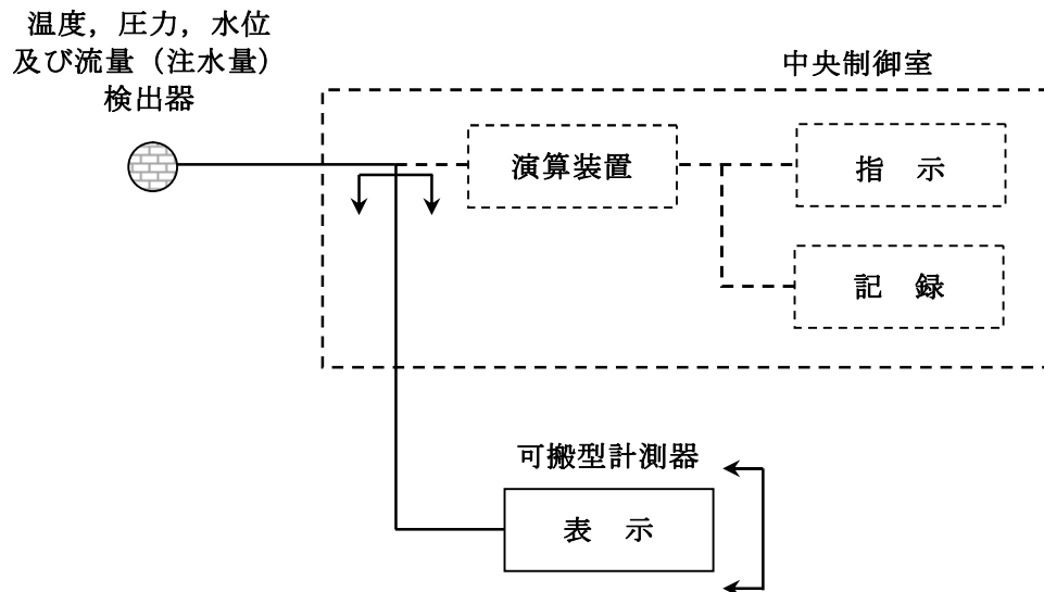
第 58-6-58 図 可搬型計測器の概略構成図
