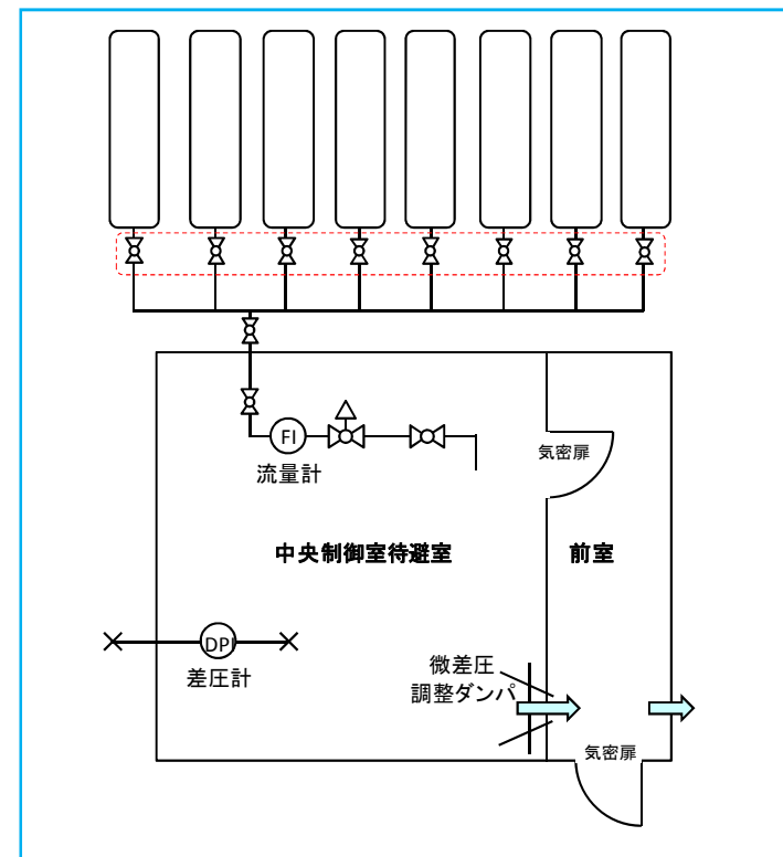
第59-4-2図 中央制御室待避室空気ポンプユニット 系統概要図
