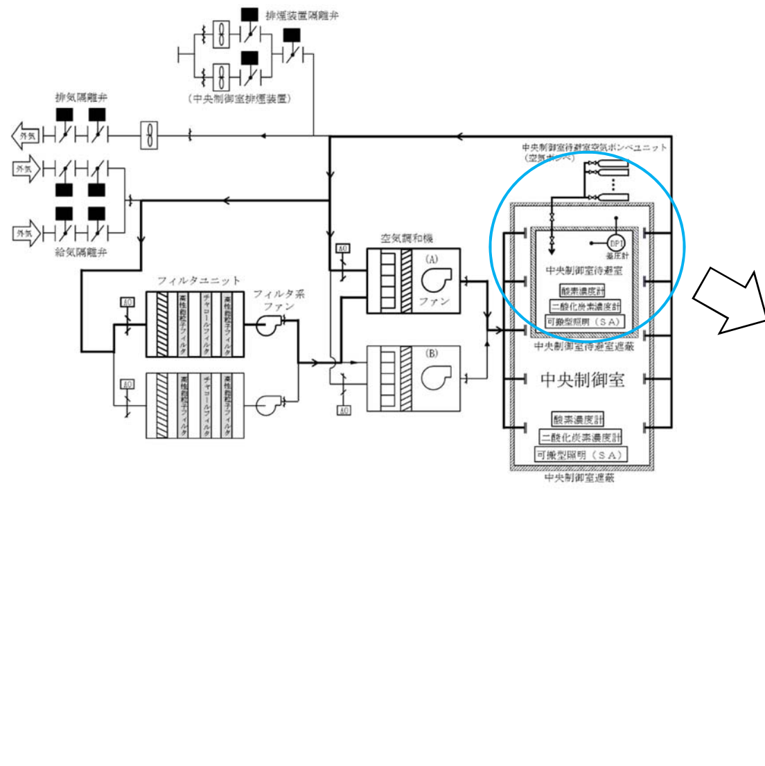
第59-4-2図 中央制御室待避室空気ポンプユニット 系統概要図
