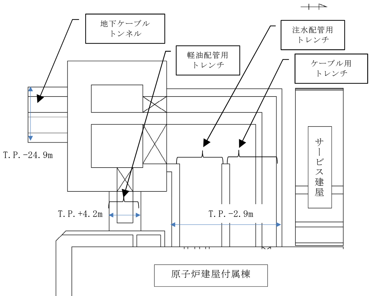
第57-11-9図 原子炉建屋西側接続口付近概要図
