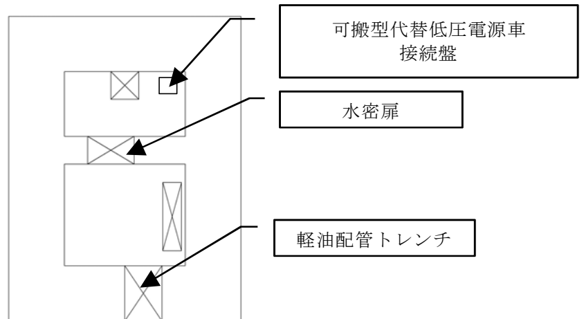
第57-11-8図 原子炉建屋西側立坑の配置 (T.P. +2.5m) (2/8)
