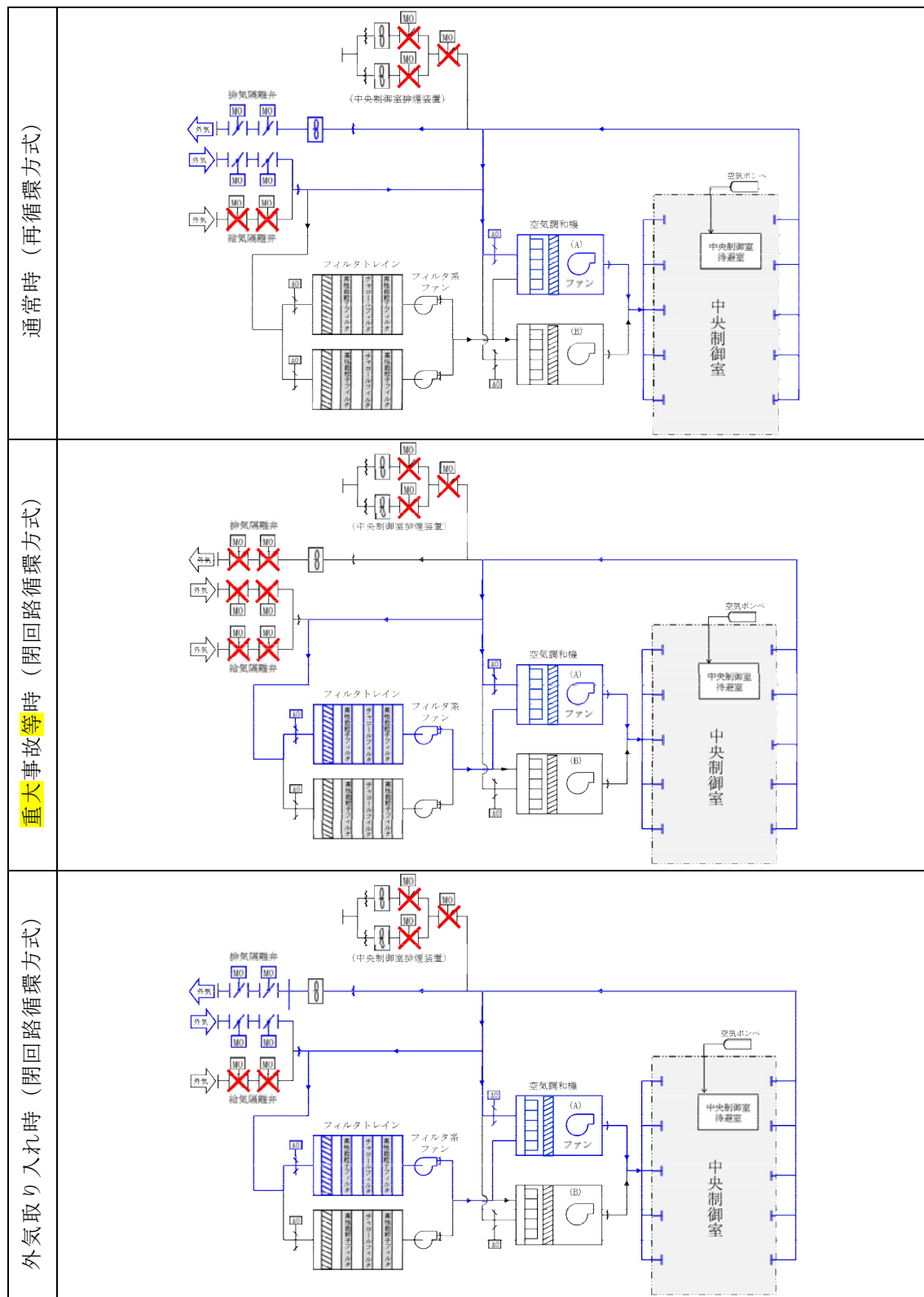
第 2.4-2 図 中央制御室換気系 概略図
