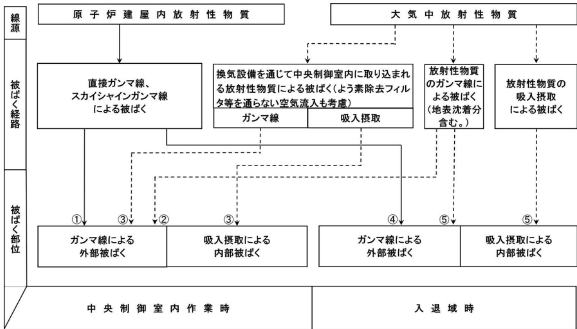
第 5-1 図 重大事故時の中央制御室居住性評価における想定被ばく経路
