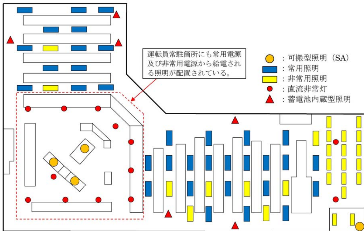
第59－3－1図 中央制御室照明配置図
