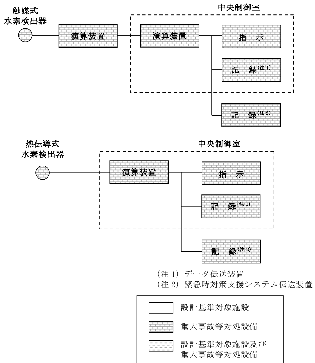
第 58-6-38 図 原子炉建屋水素濃度の概略構成図
