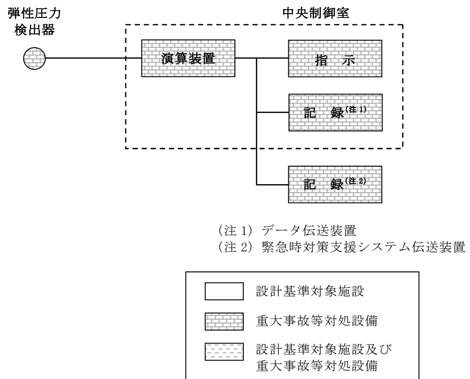
第 58-6-4 図 常設低圧代替注水系ポンプ吐出圧力の概略構成図
