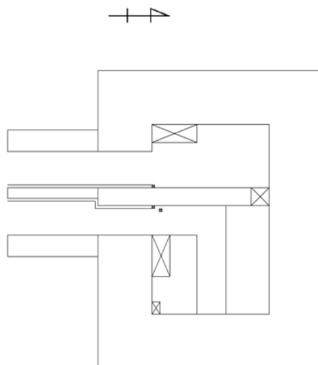
第57-11-8図 原子炉建屋西側立坑の配置 (T. P. -28.5) (8/8)
