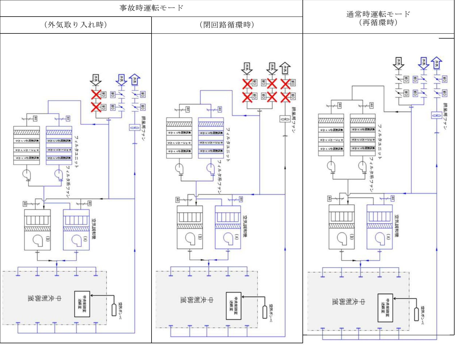
第5.1.3-2図 中央制御室換気系系統構成
