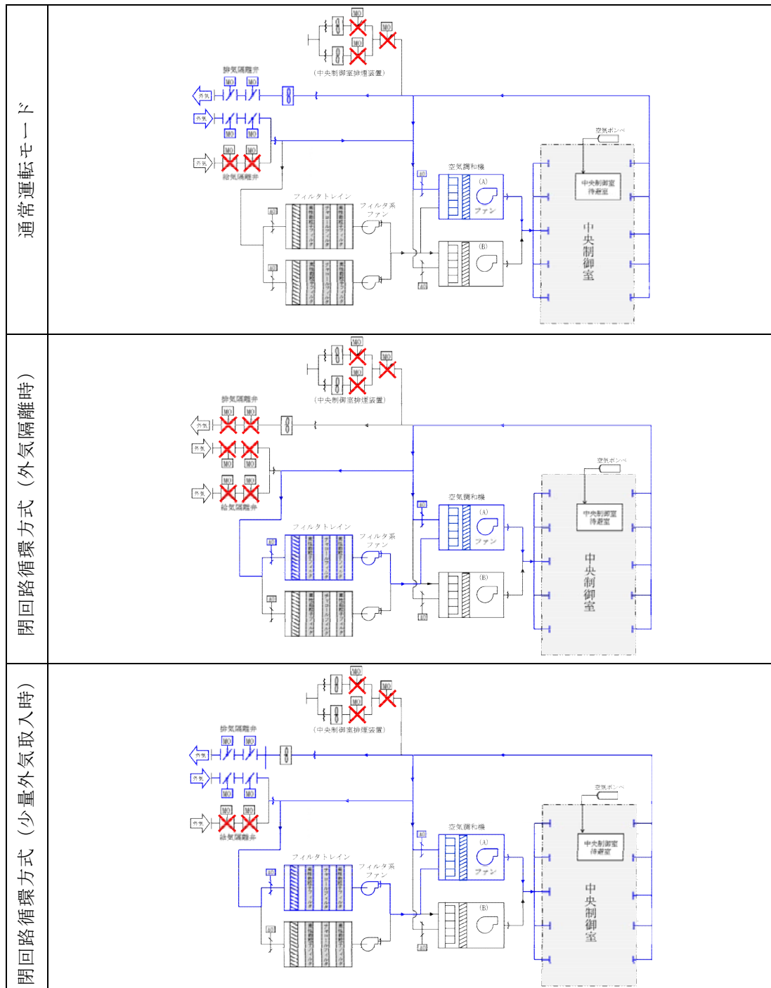
第2.4-8図 運転モードごとの中央制御室換気系系統概略図 (1/2)
