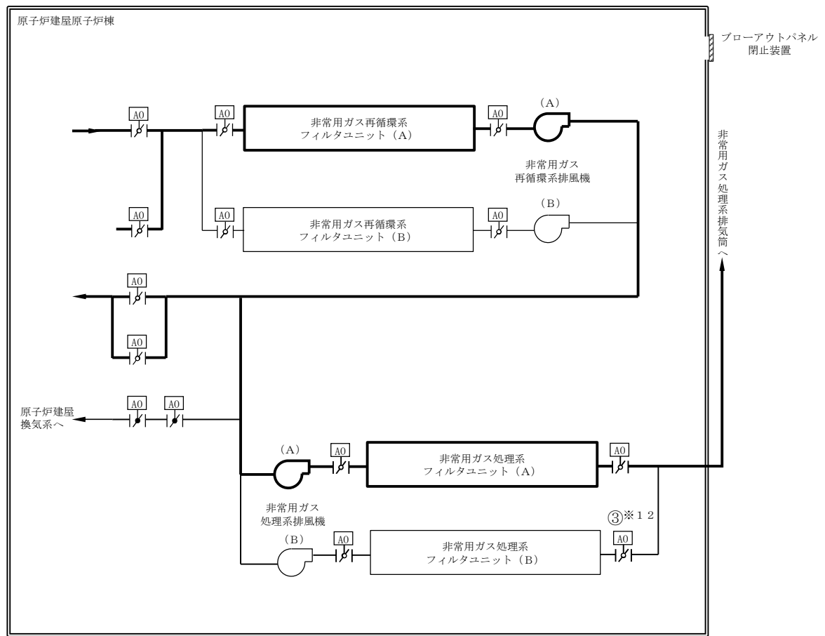
第 2.4-3 図 原子炉建屋ガス処理系 概略図
