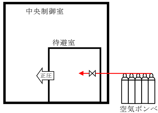
重大事故時【格納容器ベント実施中】 (空気ボンベ加圧)
