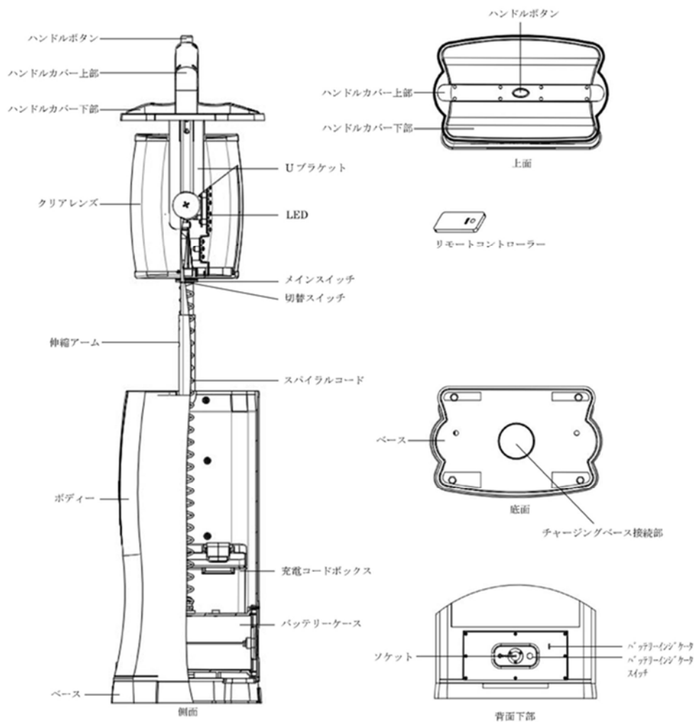
第59－5－1図 可搬型照明（S A）の概略構造図
