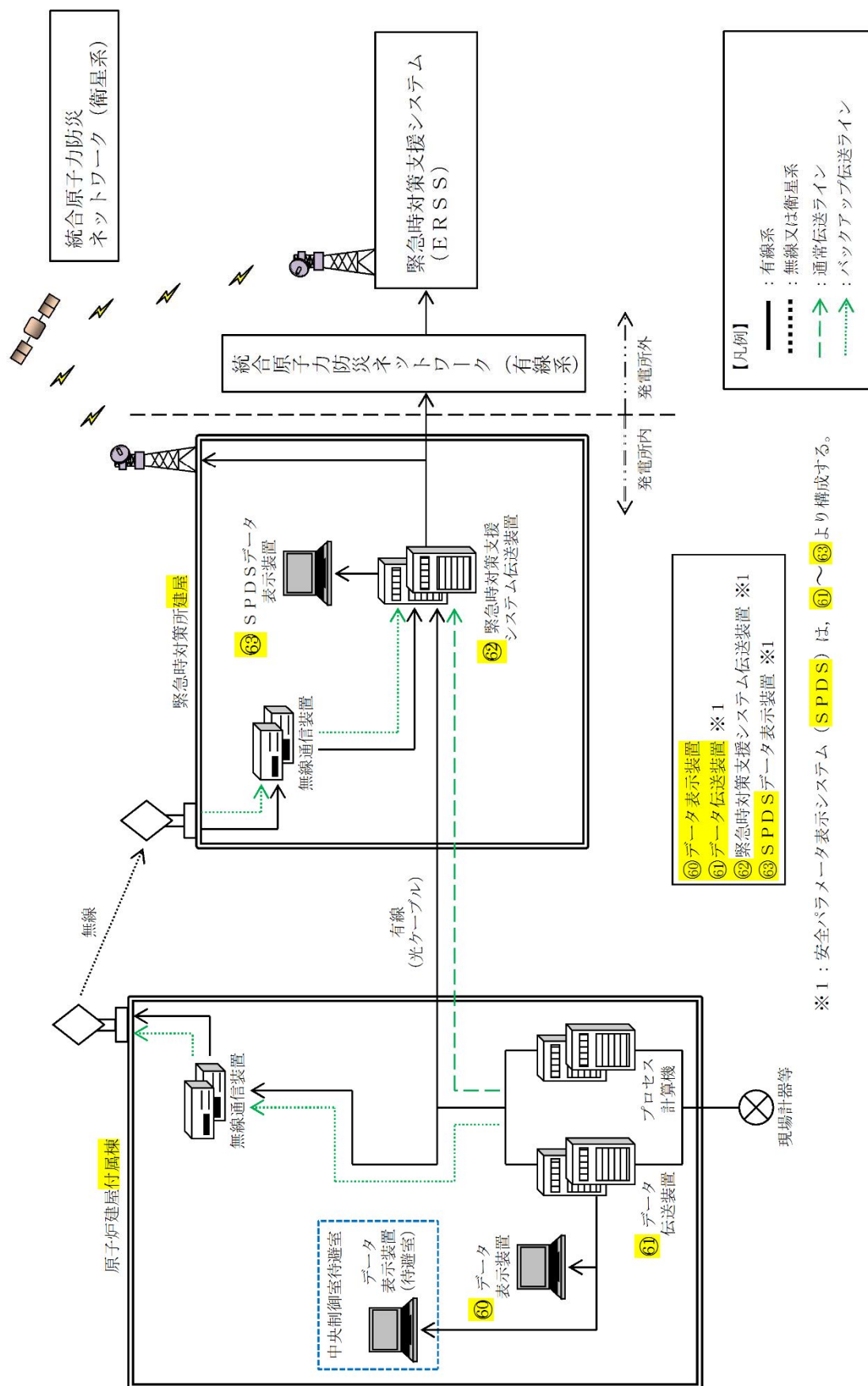
第 58-4-3 図 主要設備 系統概要図 (3/3)
