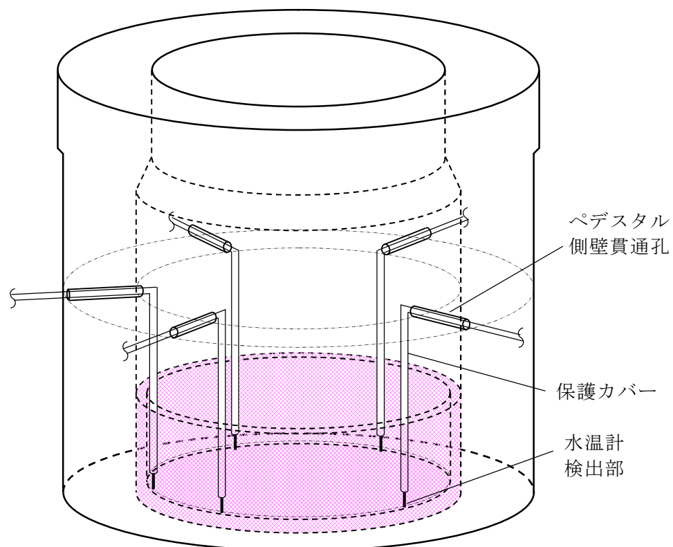
第5図 ペデスタル内検出器及びケーブル（MI ケーブル）設置概略図
