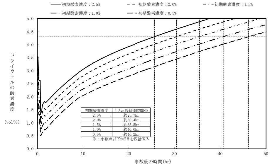
第 58-7-17 図 「雰囲気圧力・温度による静的負荷（格納容器過圧・過温破損）」 において代替循環冷却を使用する場合のドライウエルの酸素濃度変化 (格納容器内への窒素供給なし)
