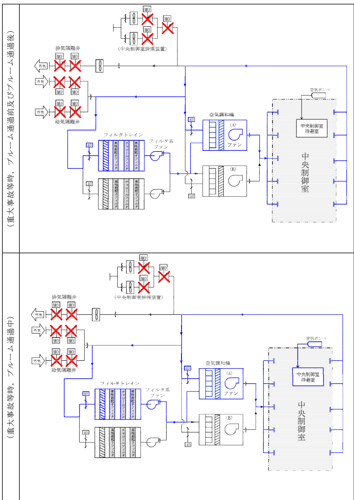
第 2.4-8 図 運転モードごとの中央制御室換気系系統概略図 (2/2)
