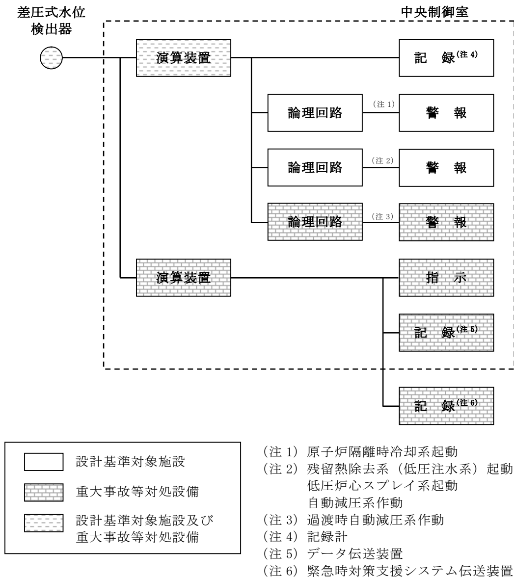
第 58-6-22 図 原子炉水位（広帯域）の概略構成図
