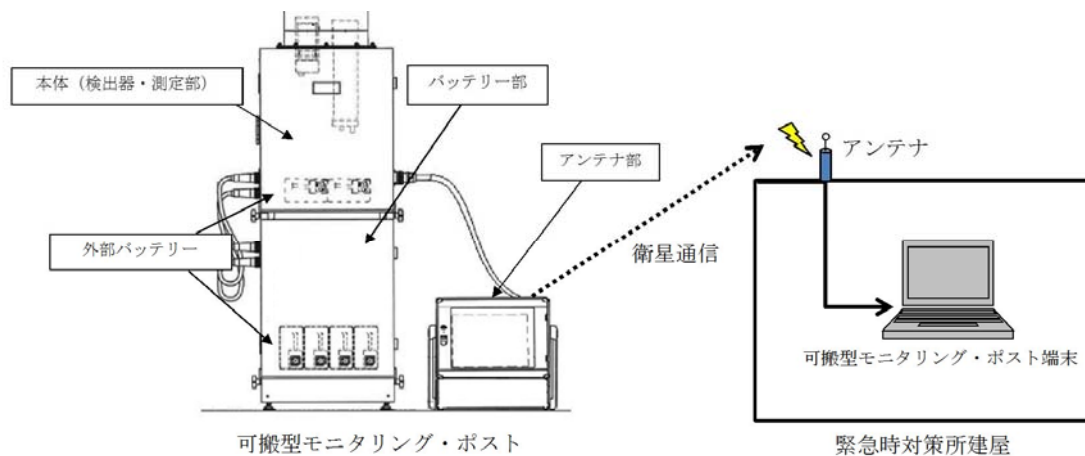
第 1.3-2 図 可搬型モニタリング・ポストの伝送概略図
