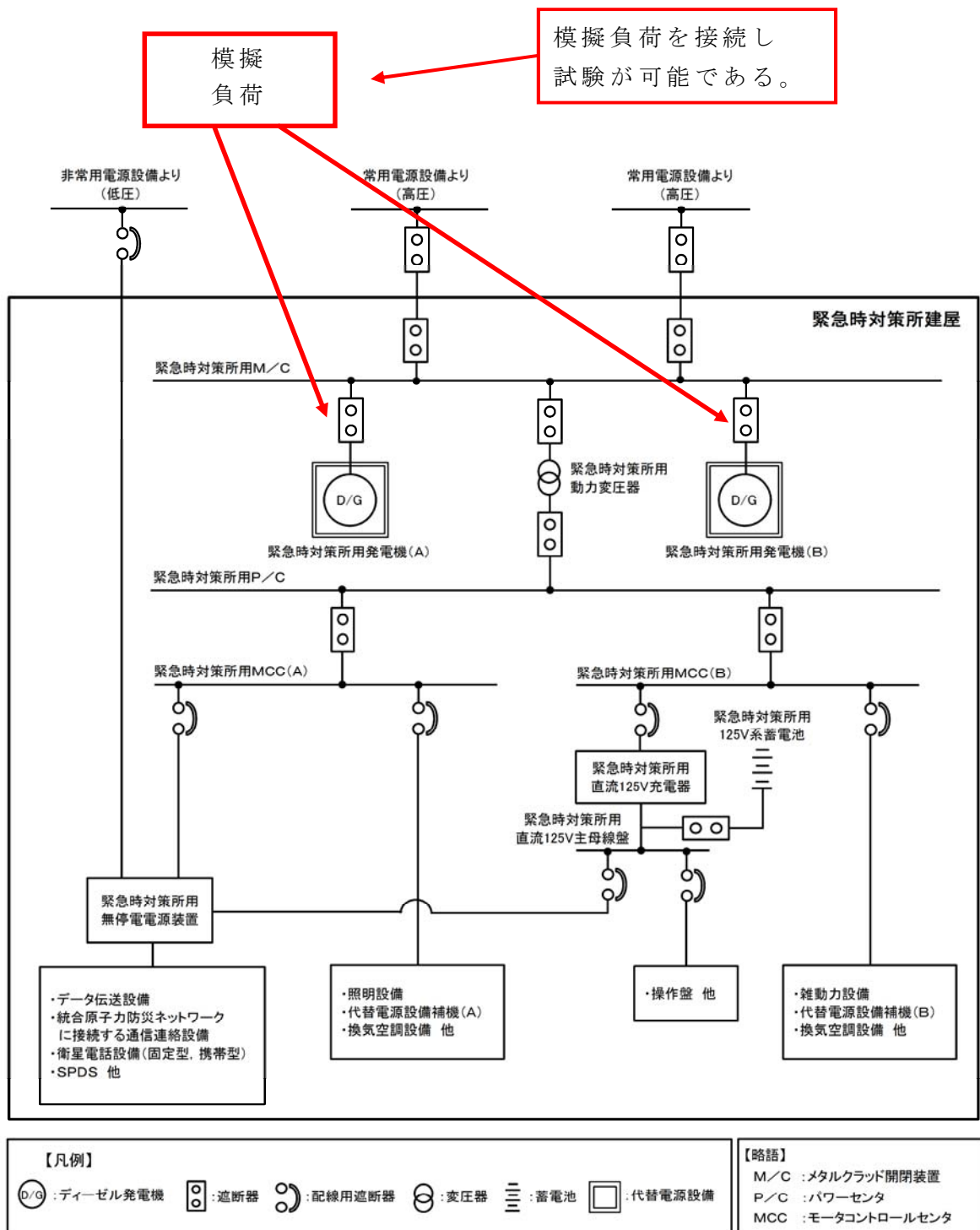
第61-5-5図 緊急時対策所用発電機 検査系統図
