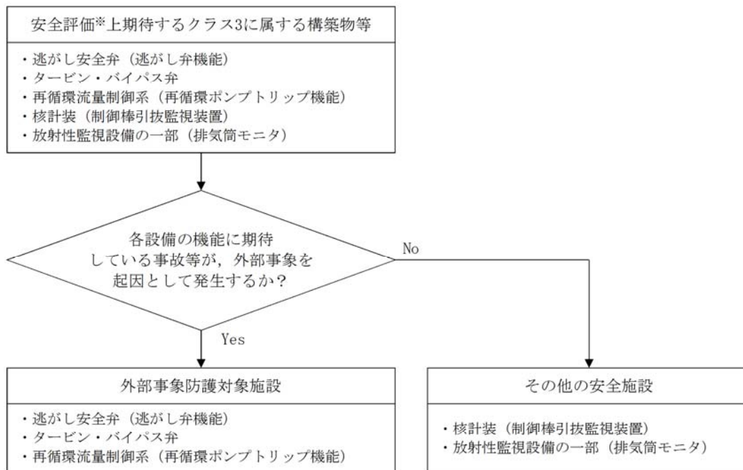
図2 外部事象防護対象施設選定フロー（クラス3に属する構築物等）
