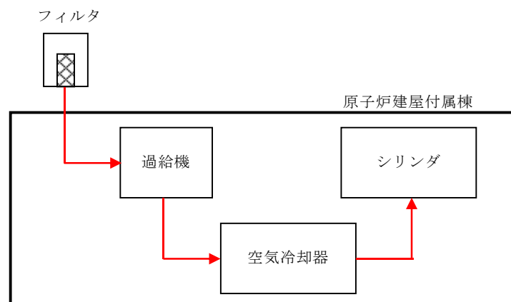
第 3.1-1 図 非常用ディーゼル発電機（高圧炉心スプレィ系ディーゼル発電機を含む。）吸気系統概略図
