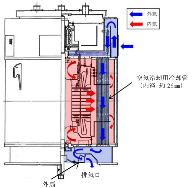
第2.4.2-6図 残留熱除去系海水ポンプ電動機 構造図
