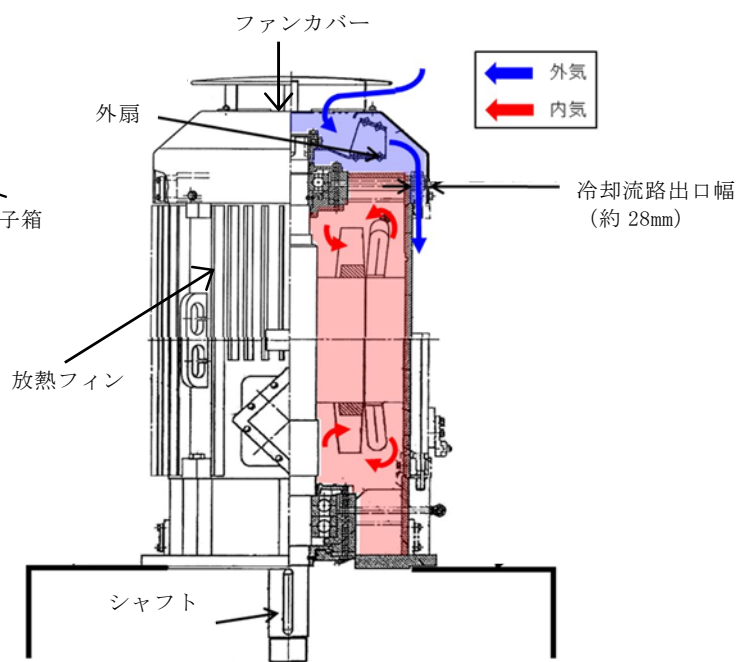
第 2.4.2-7 図 非常用ディーゼル発電機（高圧炉心スプレィ系ディーゼル発電機を含む。）用海水ポンプ電動機 構造図
