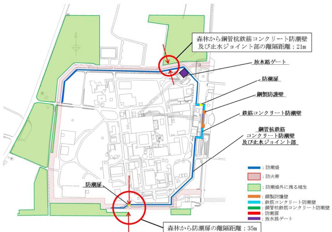
図 1 津波防護施設における森林火災の評価対象施設
