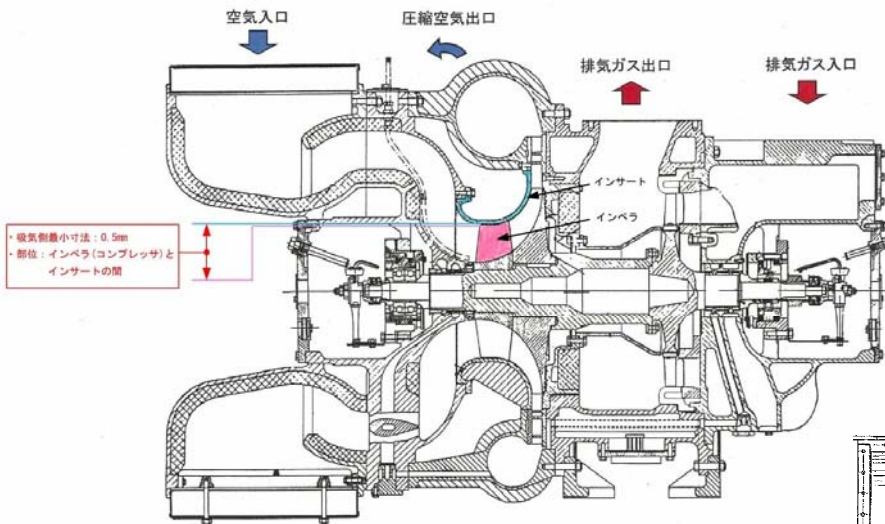
過給機断面
