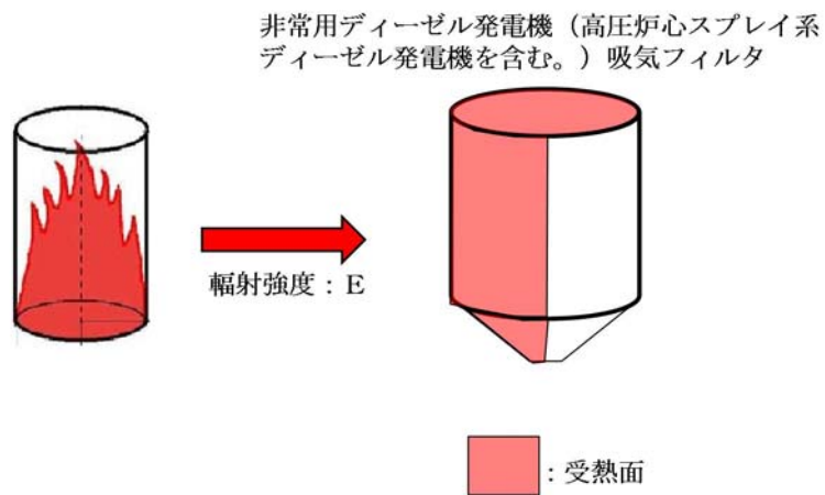
第 4.3.2.4-2 図 非常用ディーゼル発電機（高压炉心スプレイ系ディーゼル発電機を含む。）の評価概念図
