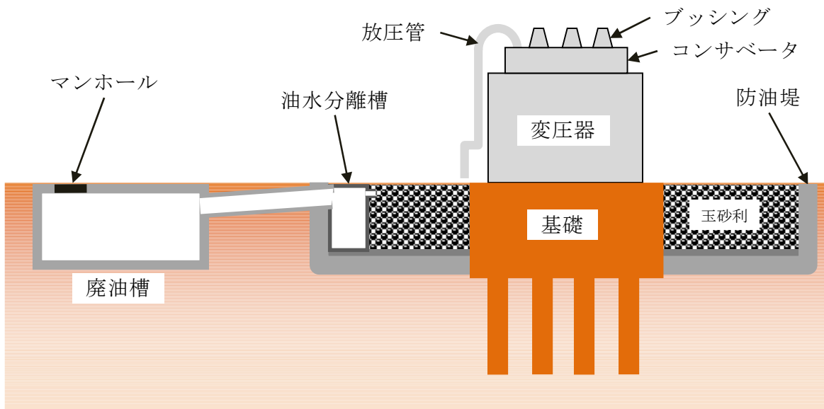
第1図 変圧器地下構造
