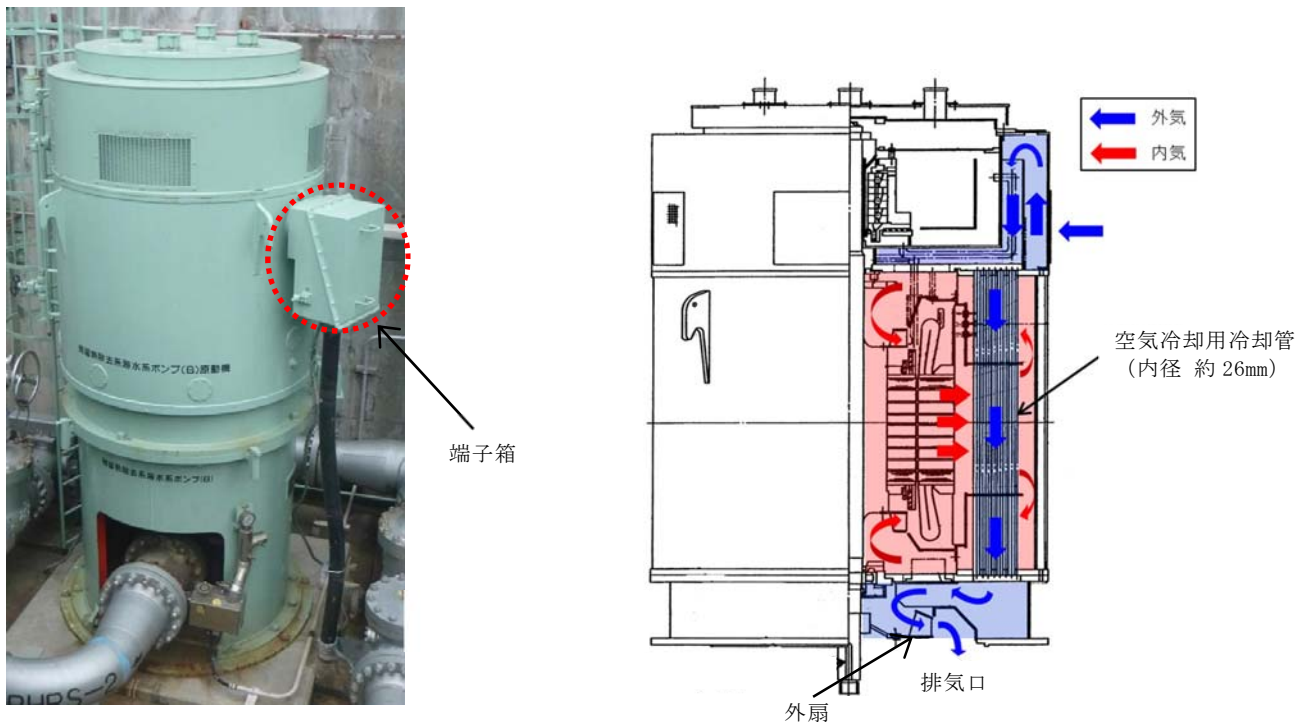
第 3.3-1 図 残留熱除去系海水ポンプ電動機 構造図
