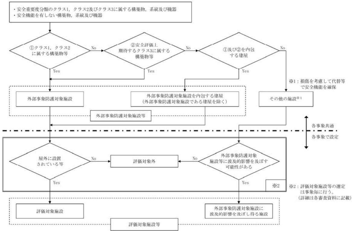
第1-1図 外部事象防護対象施設の抽出フロー
