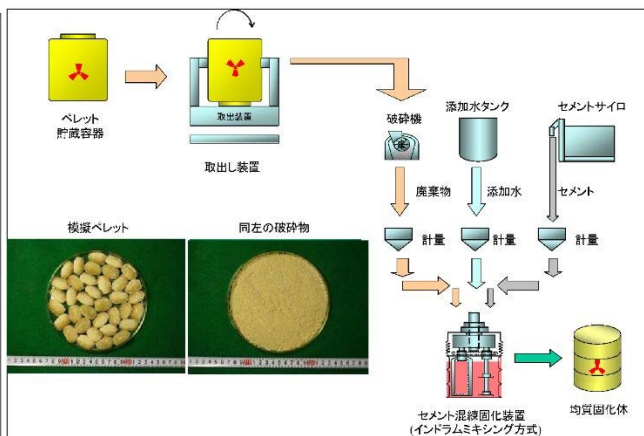
図 8 セメント混練固化装置の概要図
