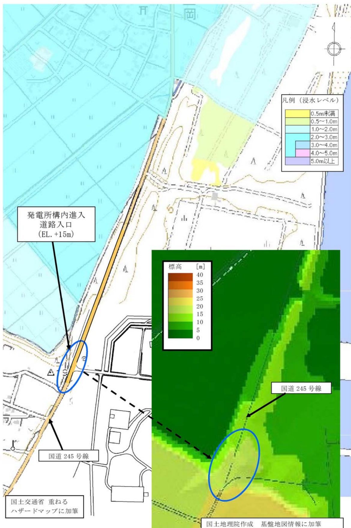
第 2-4 図 発電所敷地周辺の浸水想定図及び浸水ルート付近の標高
