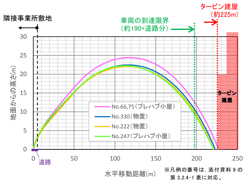
別図 7-1 北方の隣接事業所南端からタービン建屋への飛来物の飛跡
