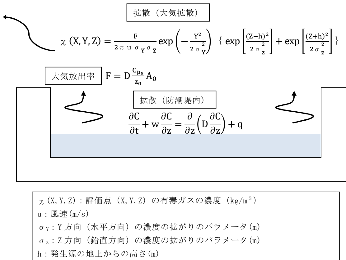
第 11-5 図 有毒ガス大気放出の考え方
