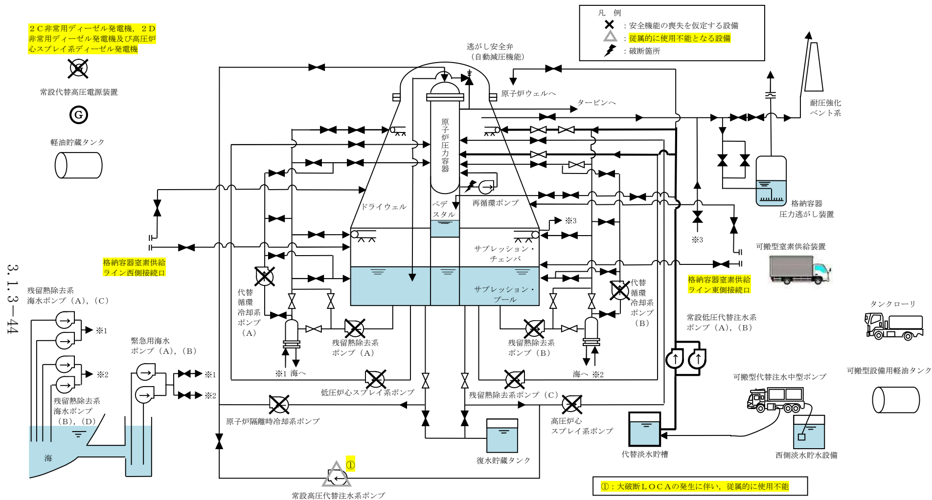
第 3.1.3-1 図 「雰囲気圧力・温度による静的負荷（格納容器過圧・過温破損）」の 重大事故等対策の概略系統図（代替循環冷却系を使用できない場合）（1/2） （低圧代替注水系（常設）による原子炉注水，代替格納容器スプレイス冷却系（常設）による格納容器冷却段階）
