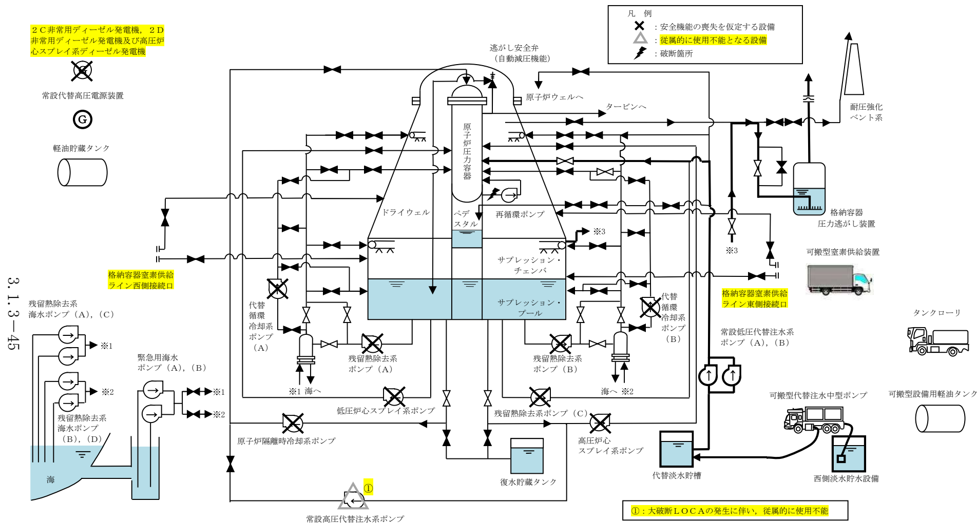
第 3.1.3-1 図 「雰囲気圧力・温度による静的負荷（格納容器過圧・過温破損）」の 重大事故等対策の概略系統図（代替循環冷却系を使用できない場合）（2/2） （低圧代替注水系（常設）による原子炉注水，格納容器圧力逃がし装置による格納容器減圧及び除熱段階）
