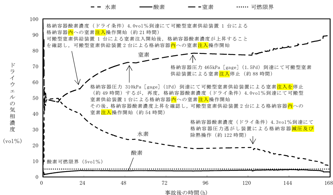
第 3 図 ドライウエルの気相濃度の推移 (ドライ条件)
