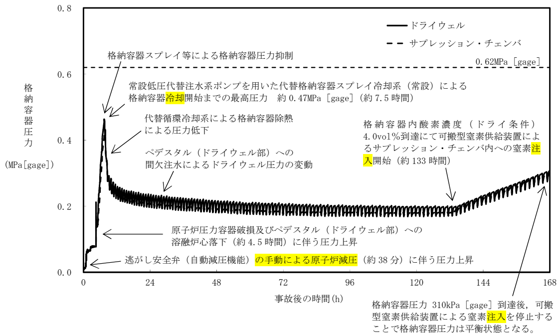
第 3.2-28 図 原子炉圧力容器破損後に原子炉注水しない場合の 格納容器圧力の推移
