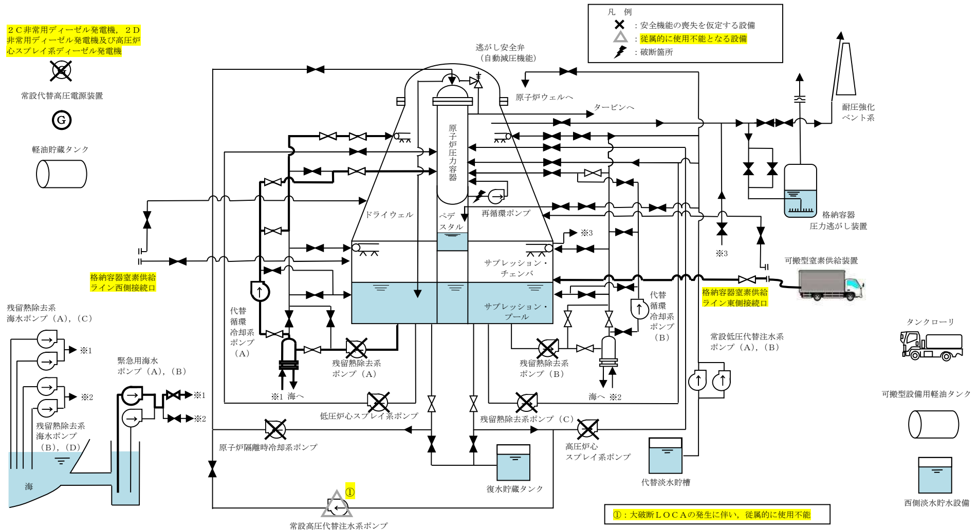
第 3.1.2-1 図 「雰囲気圧力・温度による静的負荷（格納容器過圧・過温破損）」の 重大事故等対策の概略系統図（代替循環冷却系を使用する場合）（3/3） （代替循環冷却系による原子炉注水及び格納容器除熱並びに可搬型室素供給装置による格納容器内への室素注入段階）
