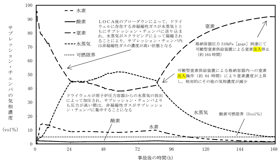
第 3.4-4 図 サブプレッション・チェンバの気相濃度の推移 (ウェット条件)
