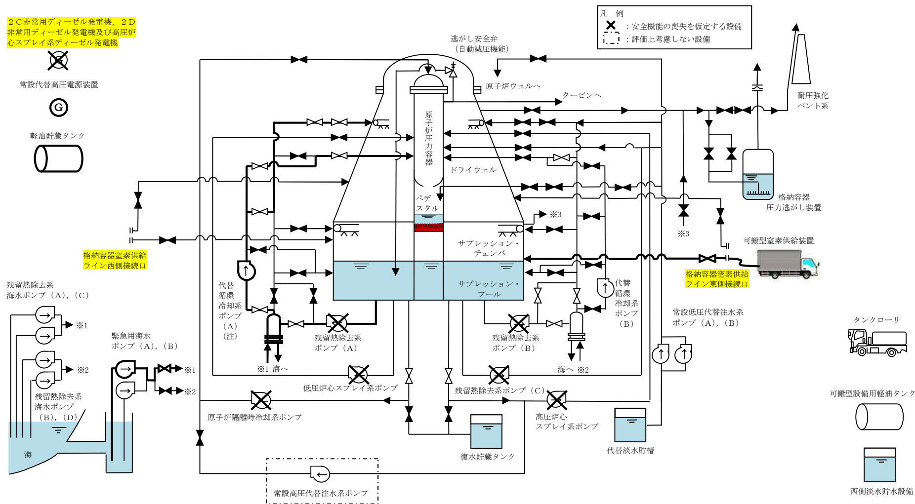
第 3.2-1 図 高压溶融物放出／格納容器雰囲気直接加熱時の重大事故等対処設備の概略系統図 (5/5) (原子炉圧力容器破損後の代替循環冷却系による原子炉注水及び格納容器除熱、 可搬型室素供給装置による格納容器内への室素注入段階)
