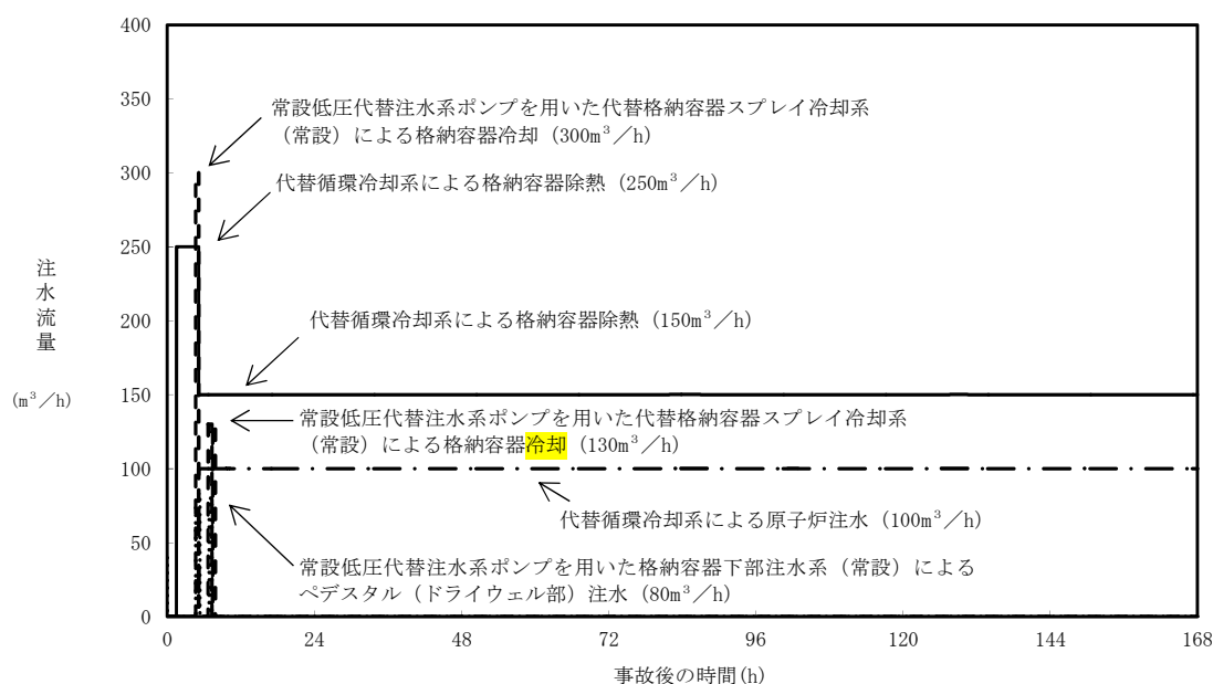
第 3.2-15 図 注水流量の推移
