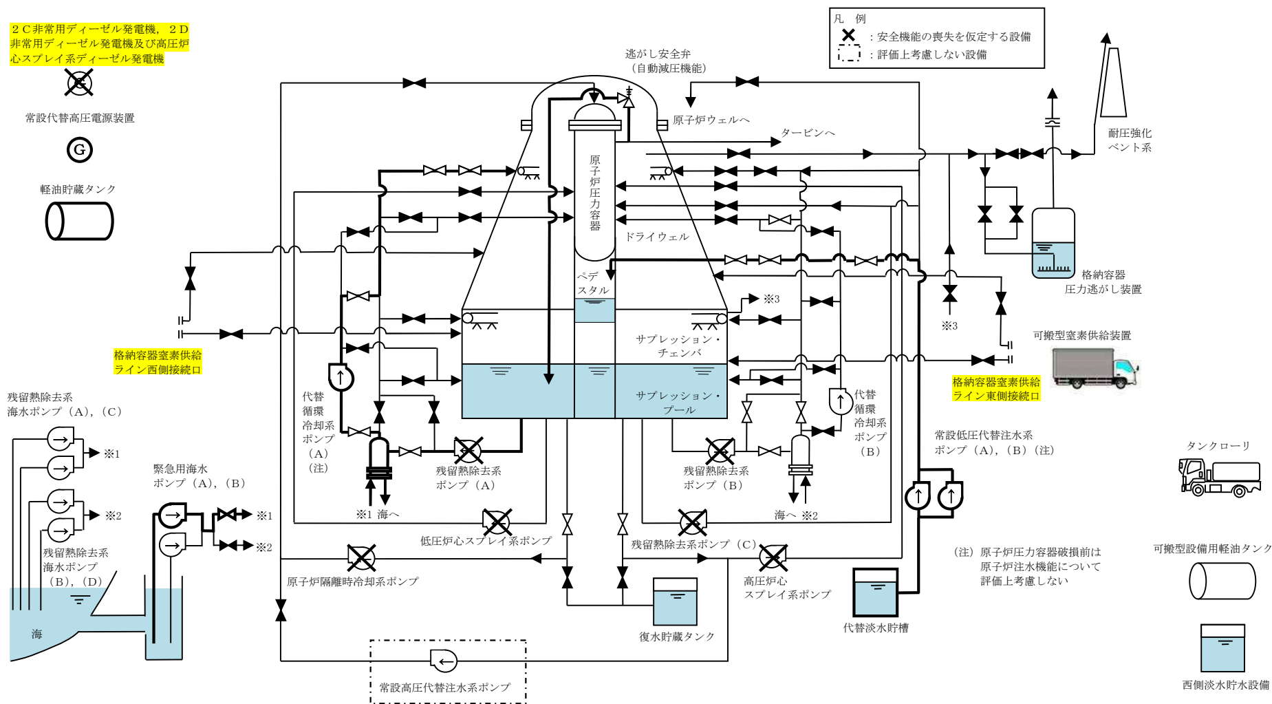
第 3.2-1 図 高压熔融物放出／格納容器雰囲気直接加熱時の重大事故等対処設備の概略系統図 (2/5) (原子炉压力容器破損前の代替循環冷却系による格納容器除熱及び 格納容器下部注水系 (常設) による ペデスタル (ドライウェル部) 水位の確保段階 )
