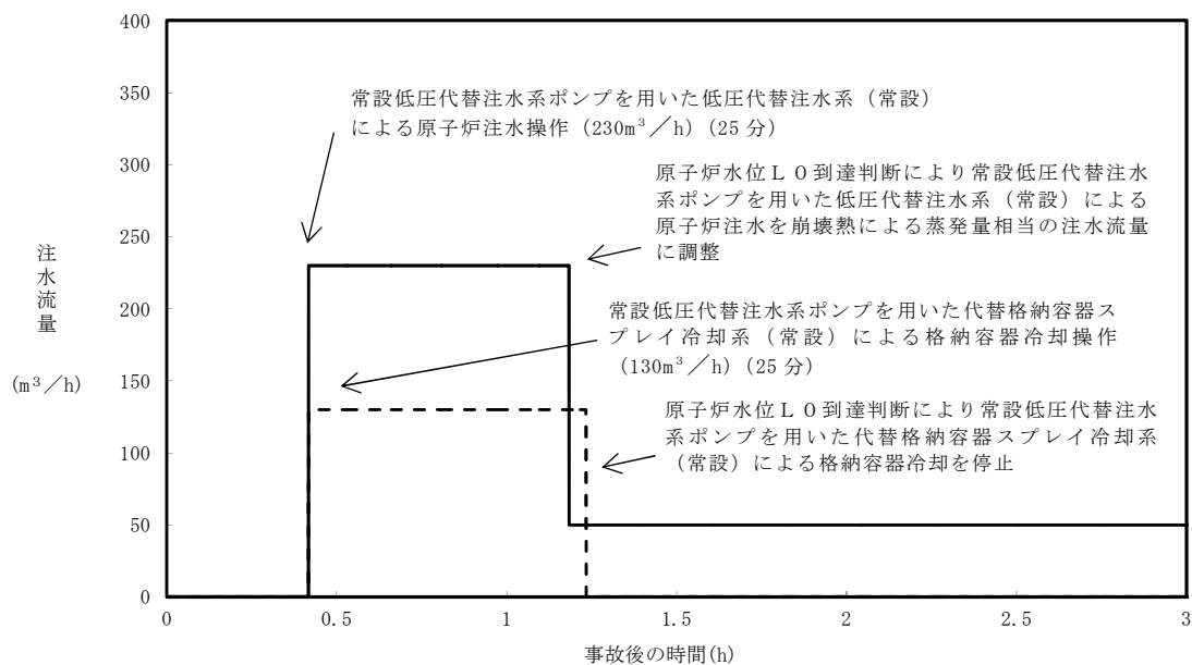
第 3.1.3-7 図 注水流量の推移 (～3 時間)
