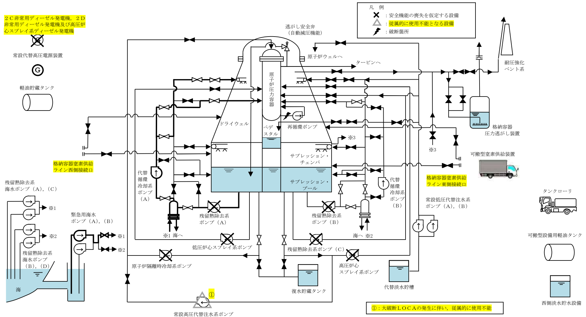
第 3.1.2-1 図 「雰囲気圧力・温度による静的負荷（格納容器過圧・過温破損）」の 重大事故等対策の概略系統図（代替循環冷却系を使用する場合）（2/3） （代替循環冷却系による原子炉注水及び格納容器除熱段階）
