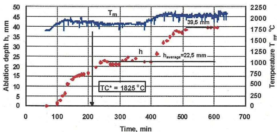
第 4 図 CIT-11 における模擬溶融炉心表面温度と耐熱材侵食深さの推移
