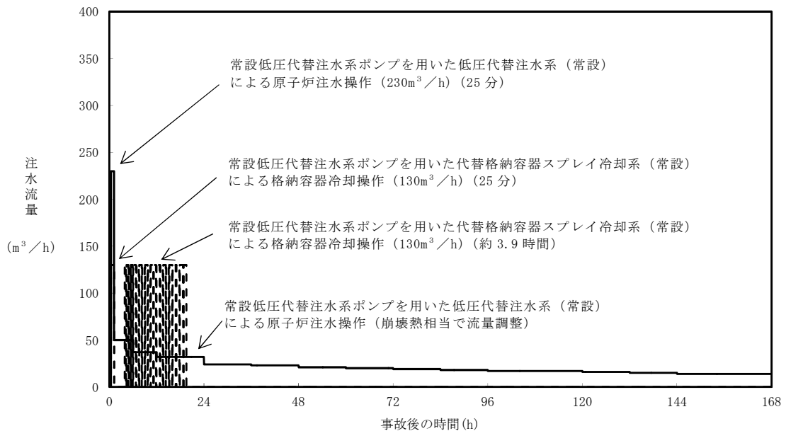
第 3. 2. 1. 3－5 図 注水流量の推移
