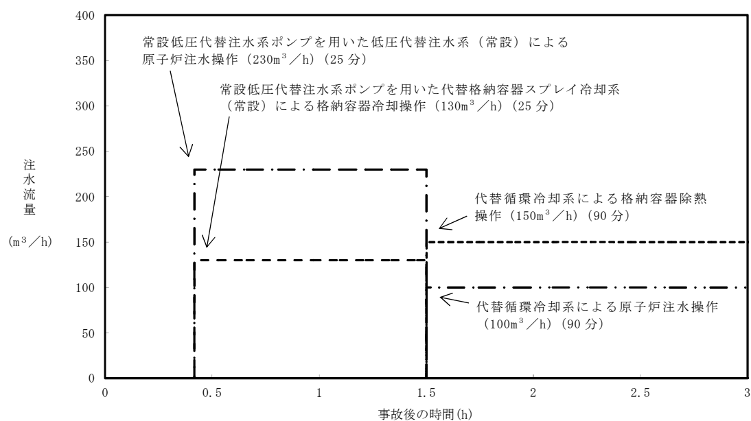
第 3. 1. 2－7 図 注水流量の推移（～3 時間）
