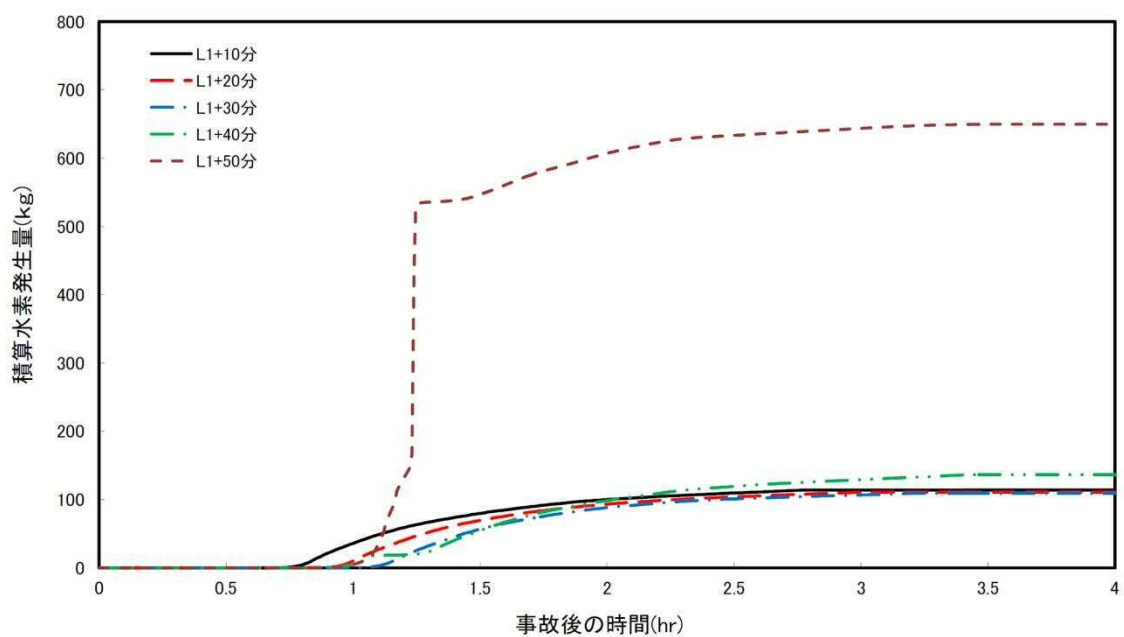
第 2 図 積算水素発生量の時間変化（逃がし安全弁（自動減圧機能）7 弁）
