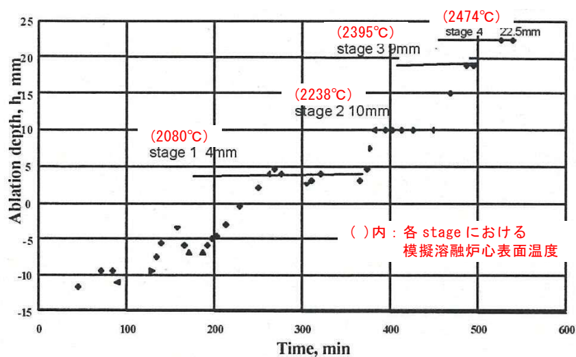
第 3 図 CIT-9 における模擬溶融炉心表面温度と耐熱材侵食深さの推移
