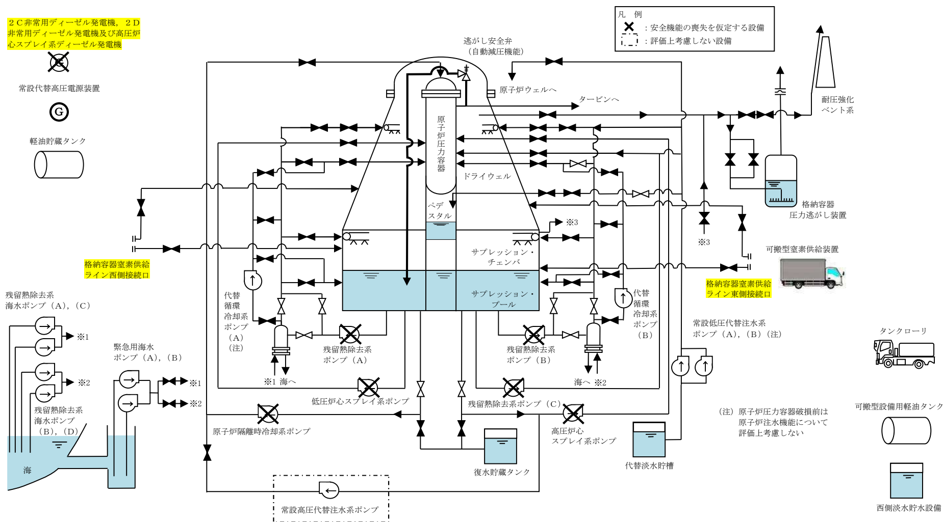
第 3.2-1 図 高压溶融物放出／格納容器雰囲気直接加熱時の重大事故等対処設備の概略系統図 (1/5) (原子炉圧力容器破損前の逃がし安全弁 (自動減圧機能) による原子炉減圧段階)
