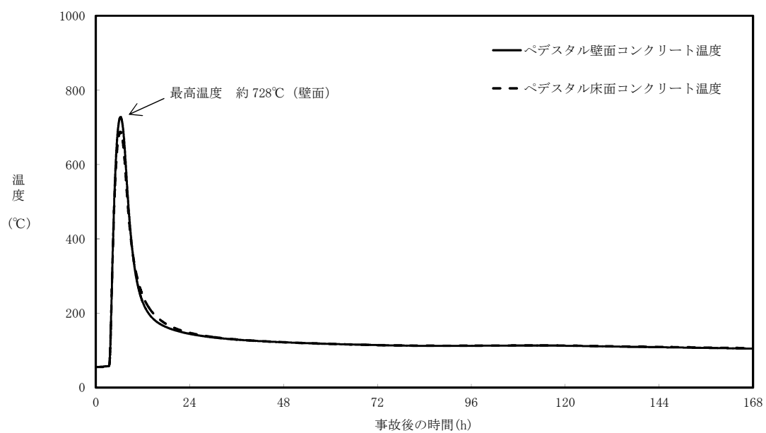
第 7.2.5-3 図 コリウムシールドの侵食及び伝熱物性値の温度依存性を 考慮した場合のペデスタル（ドライウェル部）の 壁面及び床面のコンクリート温度の推移
