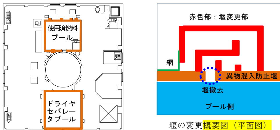
第8図 プール堰の変更概要
