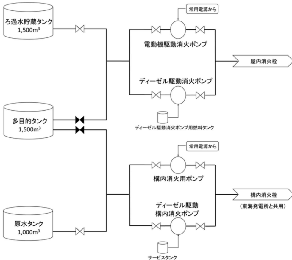
第41-1-22図 屋内消火用水供給系の概要
