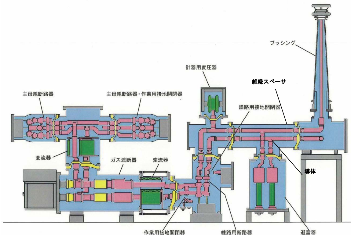
第 16 図 接地された管体内等に導体が収納された構造の例（GIS）
