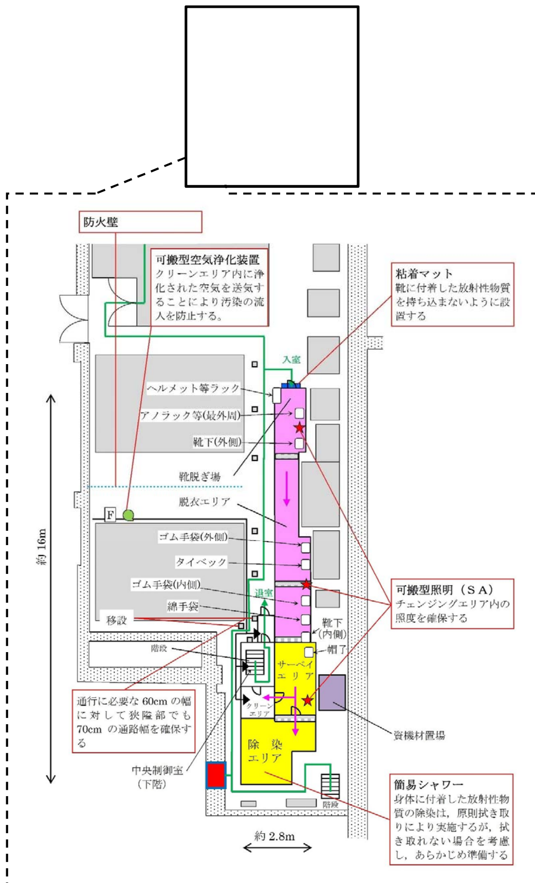
図 1-1-5 中央制御室チェン징エリア
