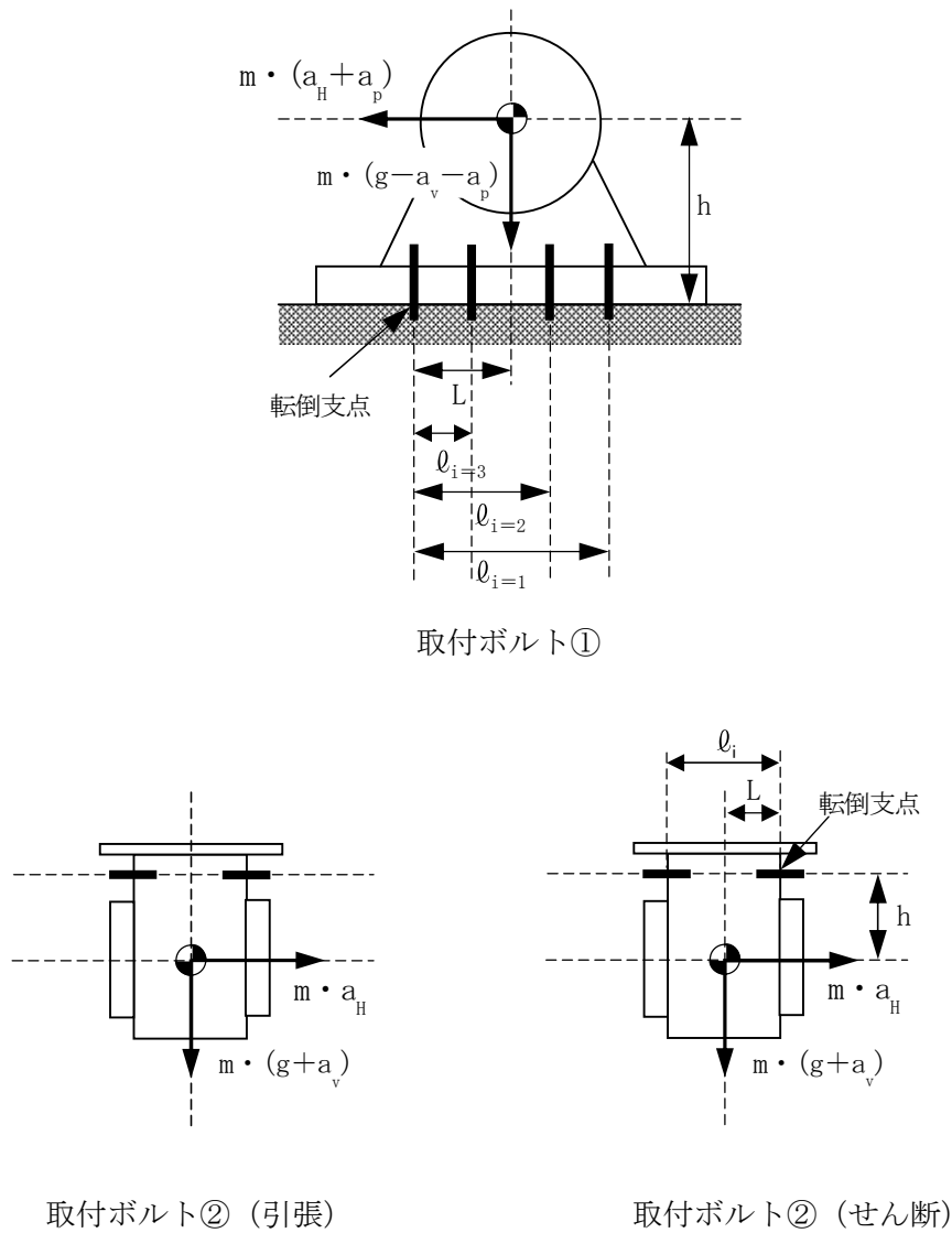
図4-1 直接支持構造物の計算モデル例
