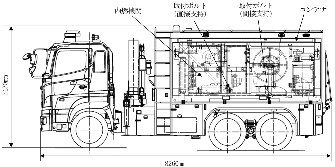
図2-3 可搬型代替注水中型ポンプの構造図 (外観図)
