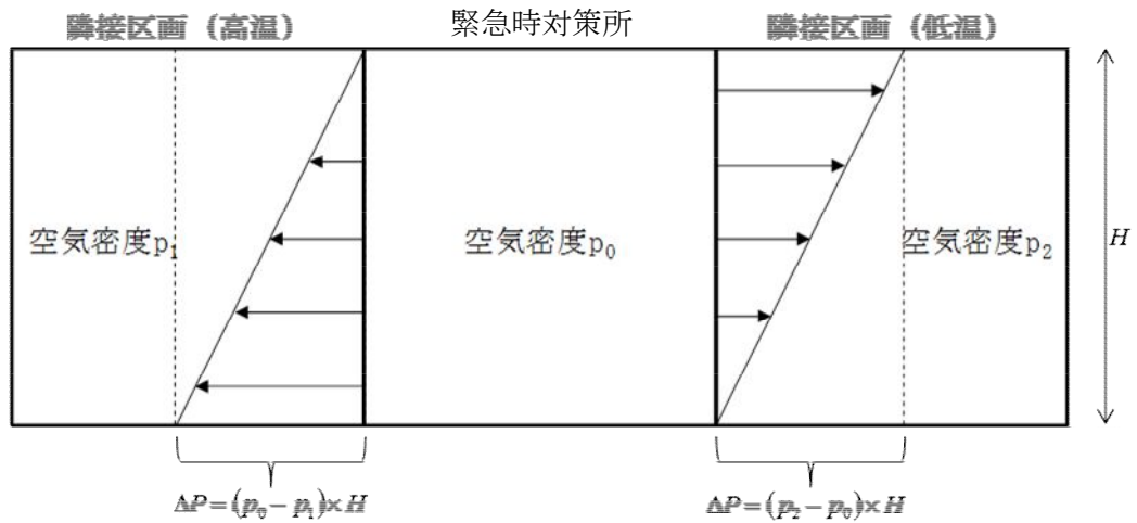
図4-9 温度差のある区画の圧力分布
