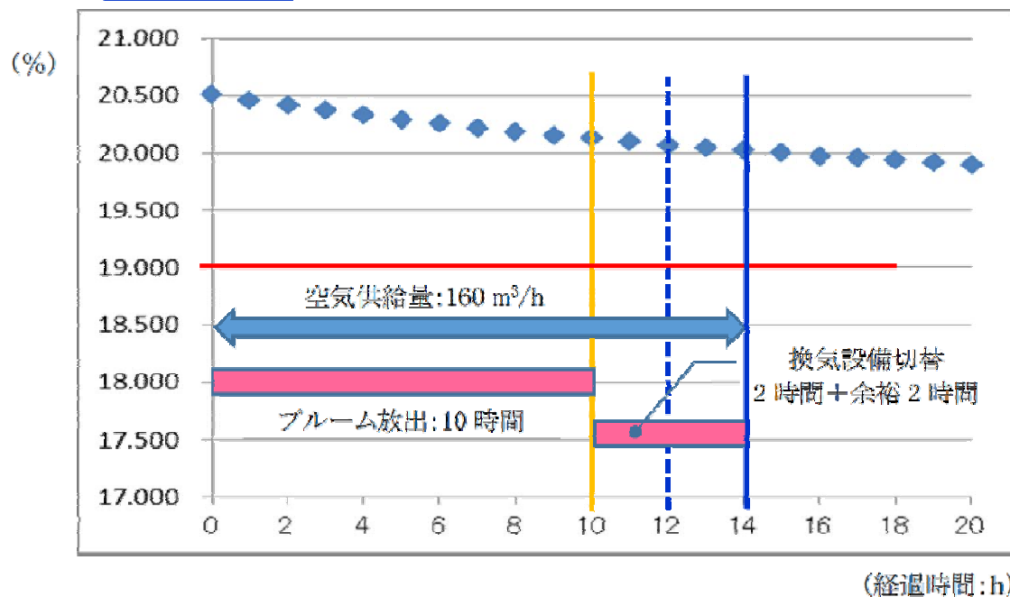
図4-13 緊急時対策所内酸素濃度及び二酸化炭素濃度推移
