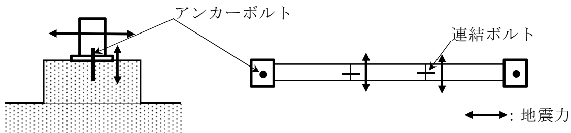
第8図(2/2) 耐震評価概要図
