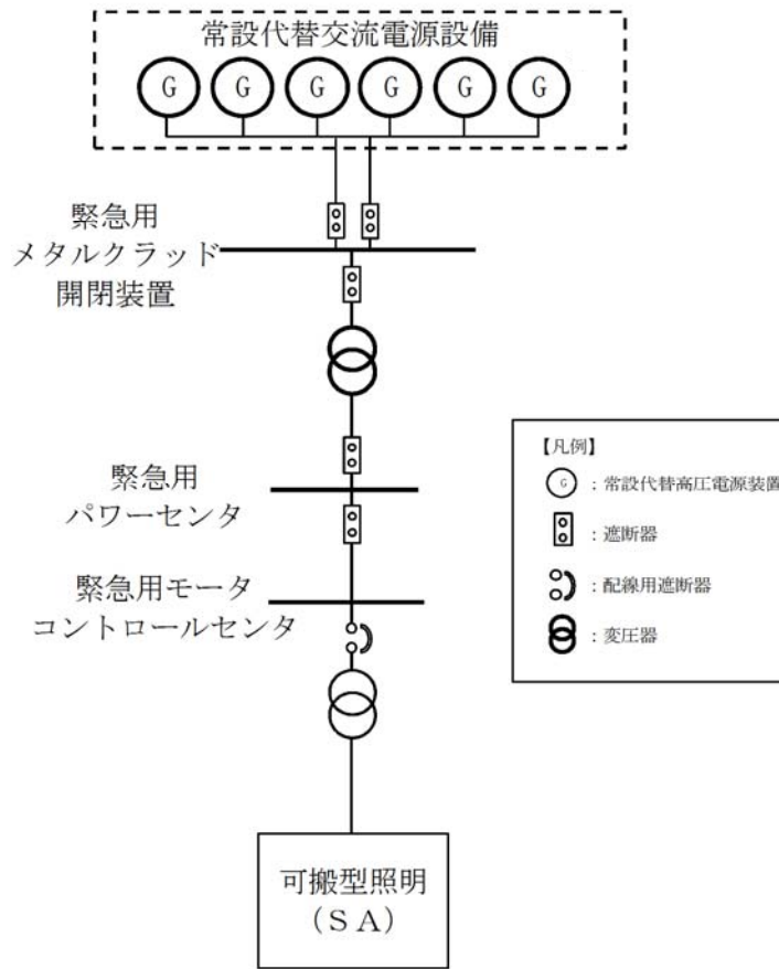
図 2 可搬型照明 (S A) 電源系統図
