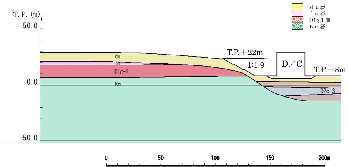
第 13-2 図 D/Cの西側斜面の影響評価断面図
