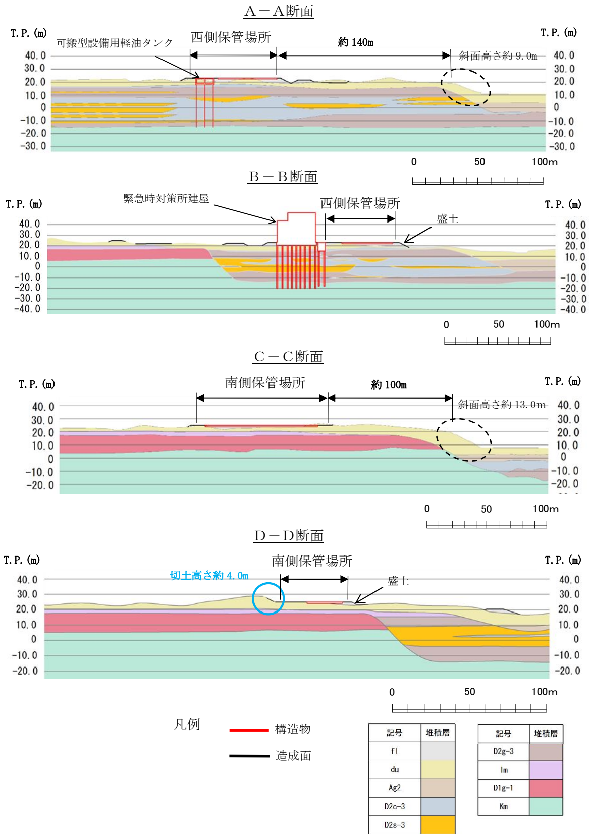
第2-4図 保管場所の周辺斜面の崩壊及び敷地内斜面のすべりに対する影響評価断面図 (1/2)
