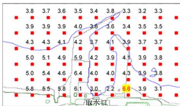
【防波堤なし】
