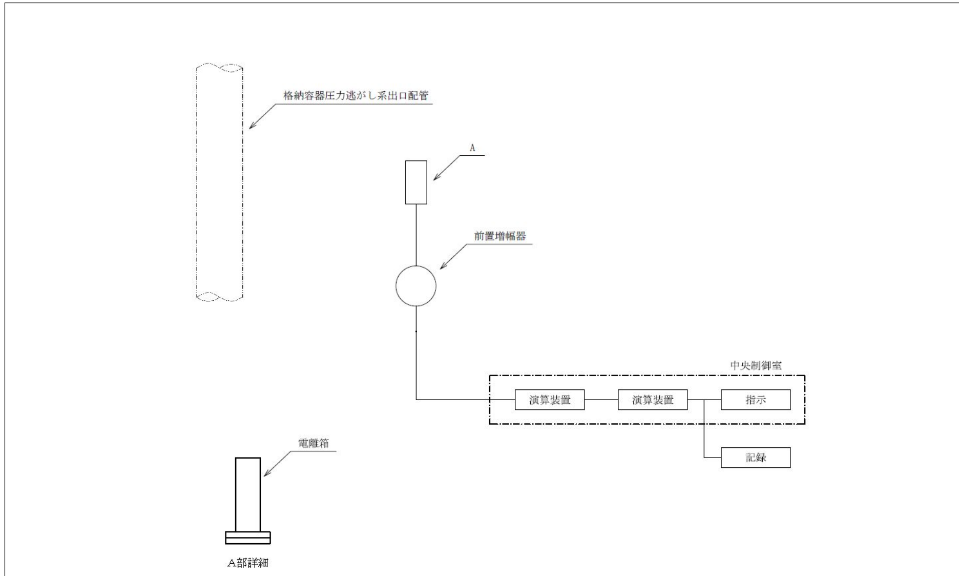
図 3-1-2-4 検出器の構造図 (フィルタ装置出口放射線モニタ (高レンジ)) (1/2)
