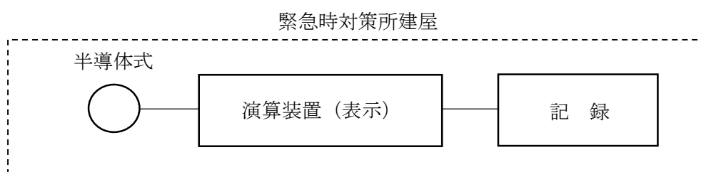
図 3-2-1-1 緊急時対策所エリアモニタの概略構成図
