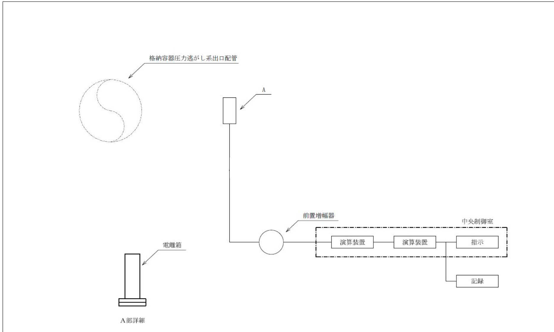
図 3-1-2-5 検出器の構造図 (フィルタ装置出口放射線モニタ (高レンジ)) (2/2)
