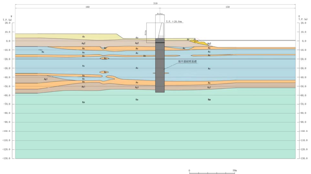
第3-2 図 (2) 鉄筋コンクリート防潮壁 評価対象断面図 (②-②断面)
