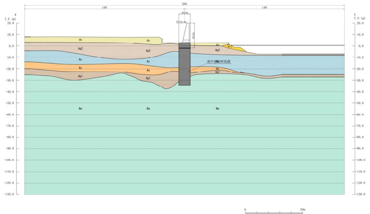
第3-2 図 (6) 鉄筋コンクリート防潮壁 評価対象断面図 (⑥-⑥断面)
