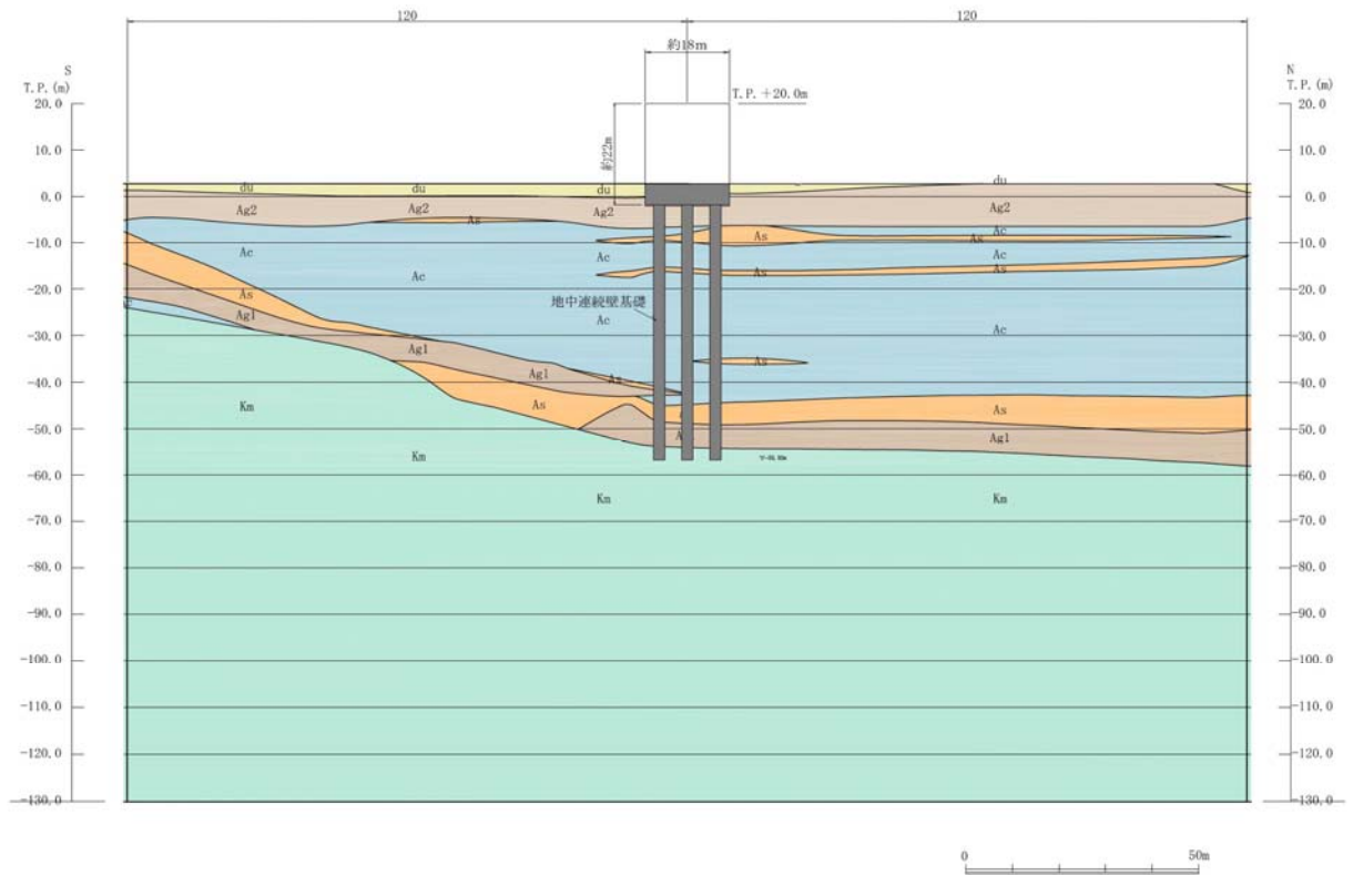
第3-2 図 (1) 鉄筋コンクリート防潮壁 評価対象断面図 (①-①断面)
