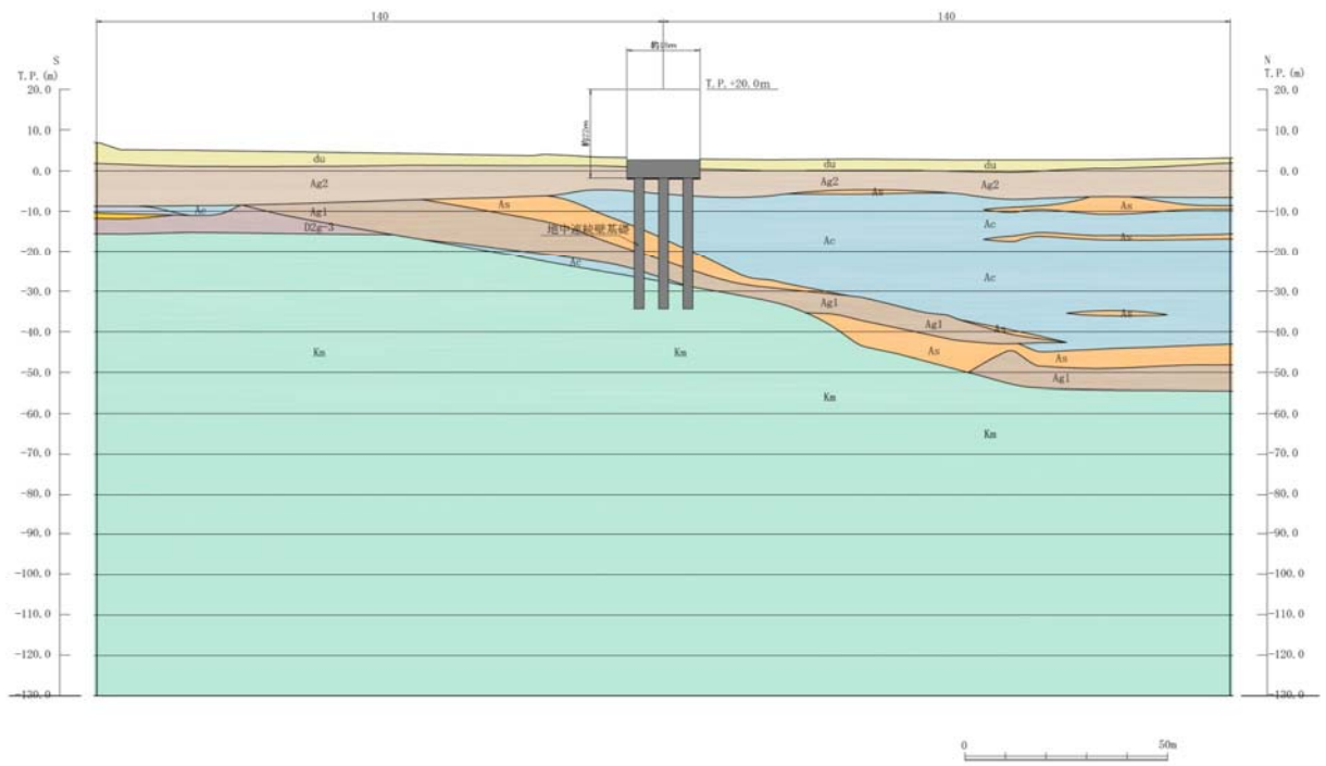
第3-2 図 (5) 鉄筋コンクリート防潮壁 評価対象断面図 (⑤-⑤断面)
