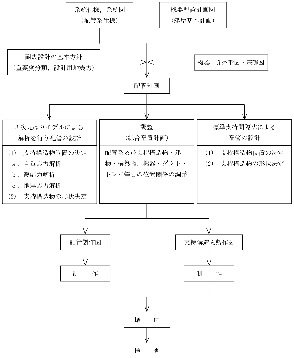
図 2-1 配管系及び支持構造物の設計作業手順
