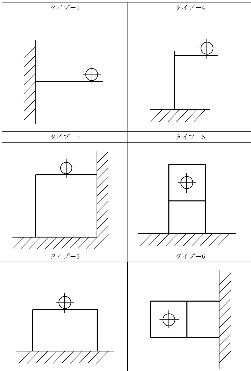
図 4-2 支持架構の代表構造例
