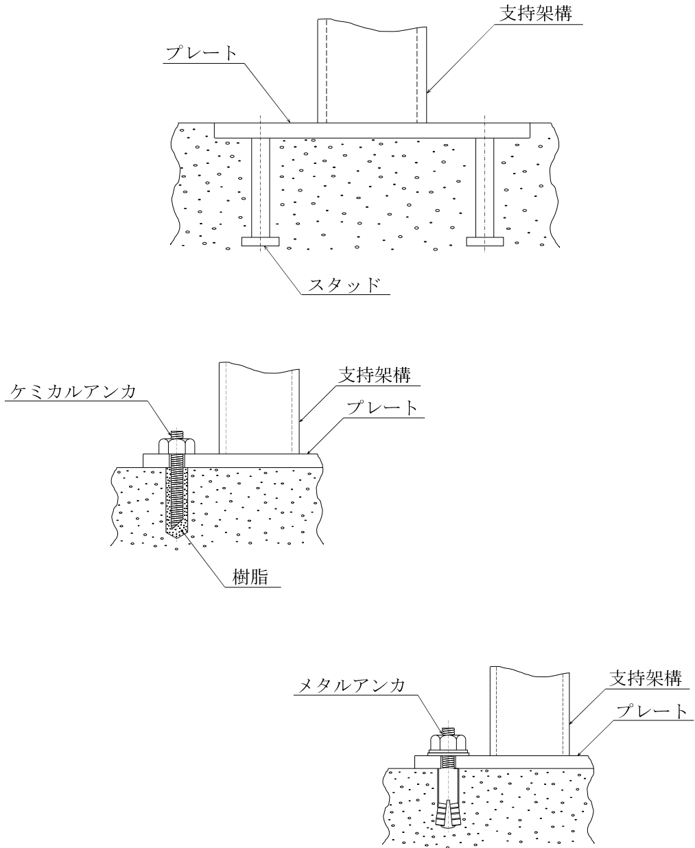
図 4-3 埋込金物の概略図
