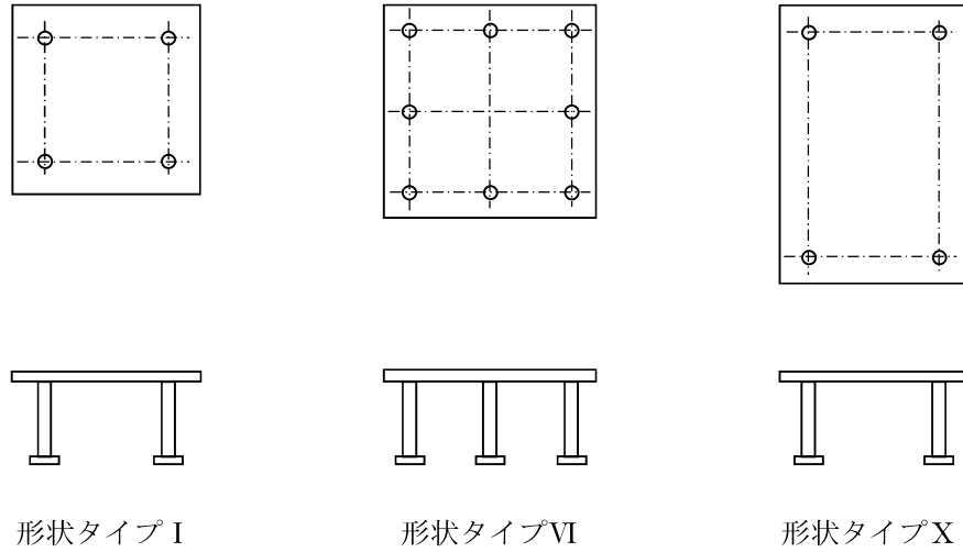
図 4-4 埋込金物の形状例
