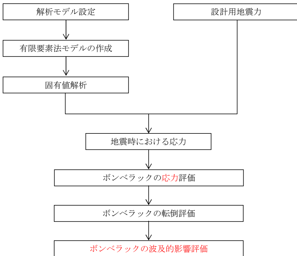
図 2-1 ボンベ設備の耐震評価フロー
