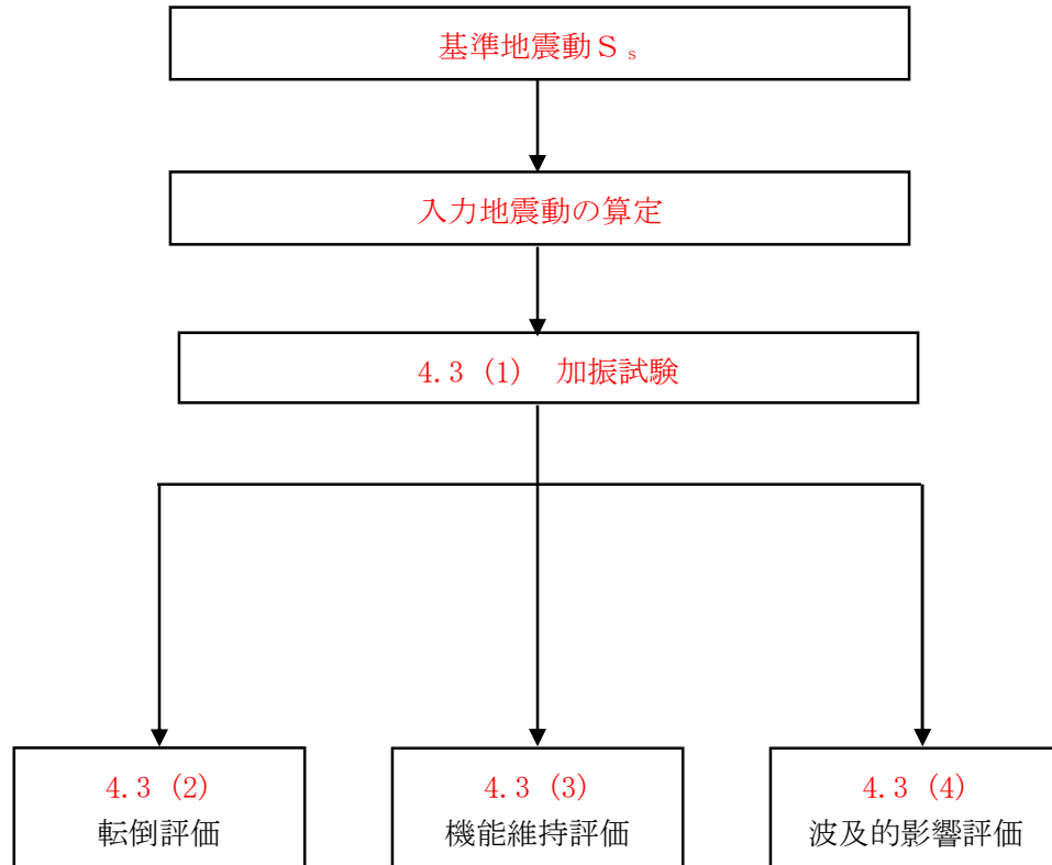
図4-5 その他設備の評価フロー
