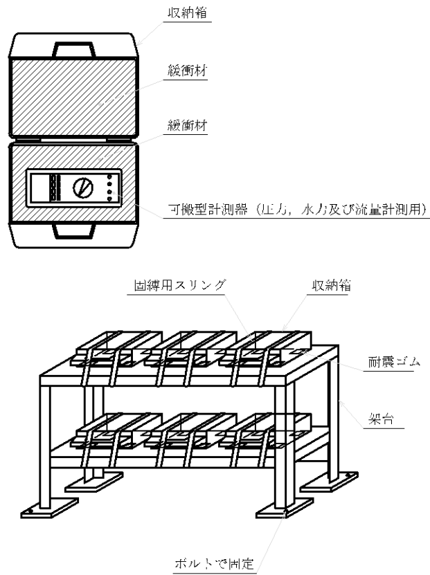
図2-6 その他設備（収納箱固縛）
