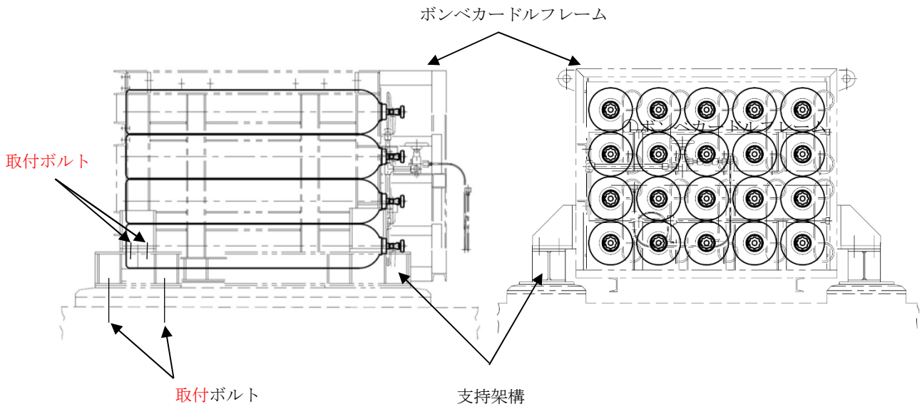
図2-4 ポンベ設備 (緊急時対策所加圧設備)
