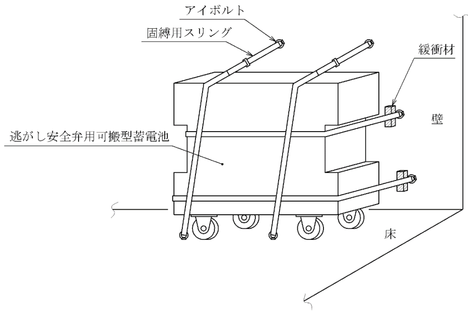
図2-7 その他設備（本体固縛）
