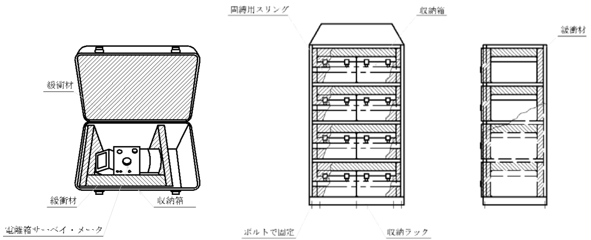
図2-5 その他設備（収納ラック固縛）
