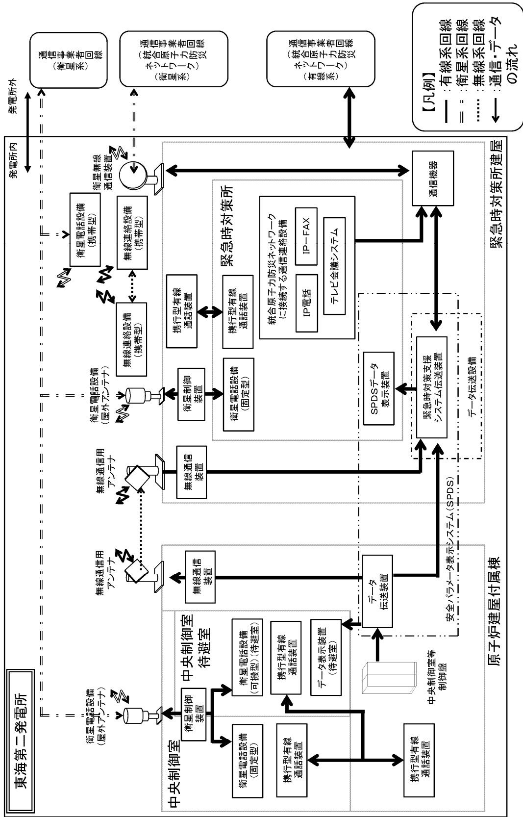
第7図 緊急時対策所情報収集設備
