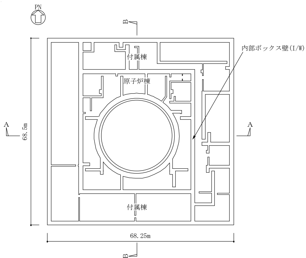
図 2-2 (2/2) 原子炉棟を含む原子炉建屋の概略平面図 (EL. -4.0 m)
