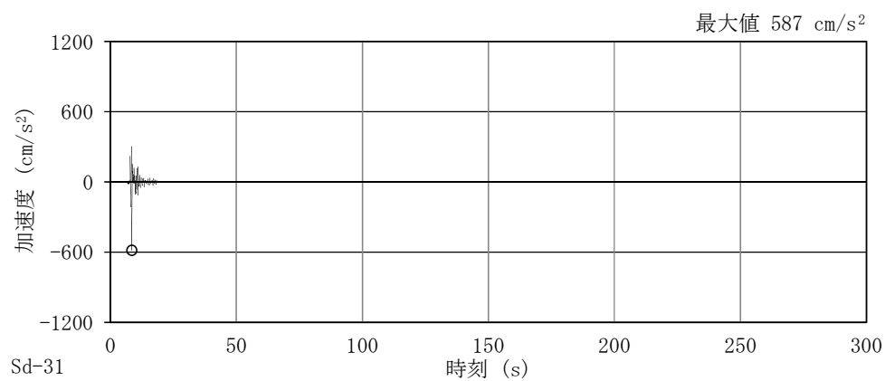
図4-19 加速度時刻歴波形
