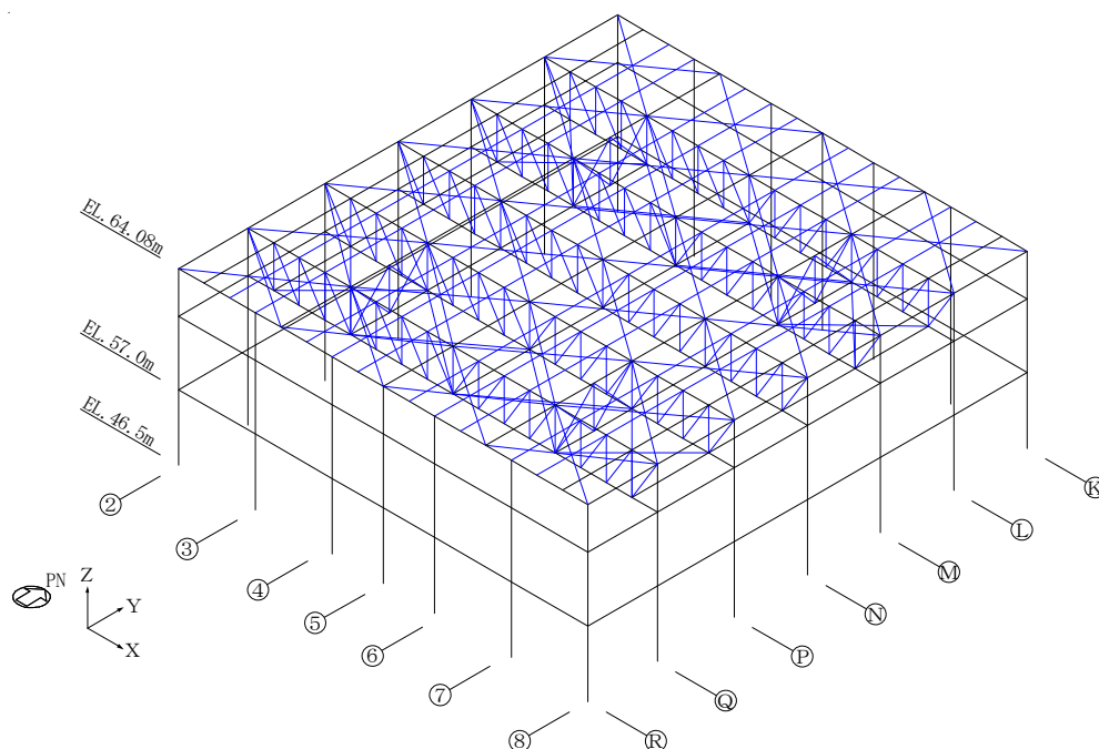
図4-66 解析モデル（屋根トラス）
