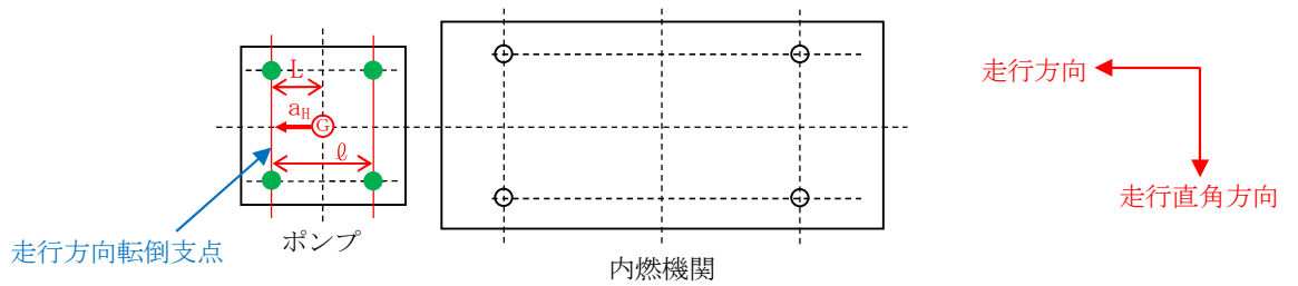
平面図
