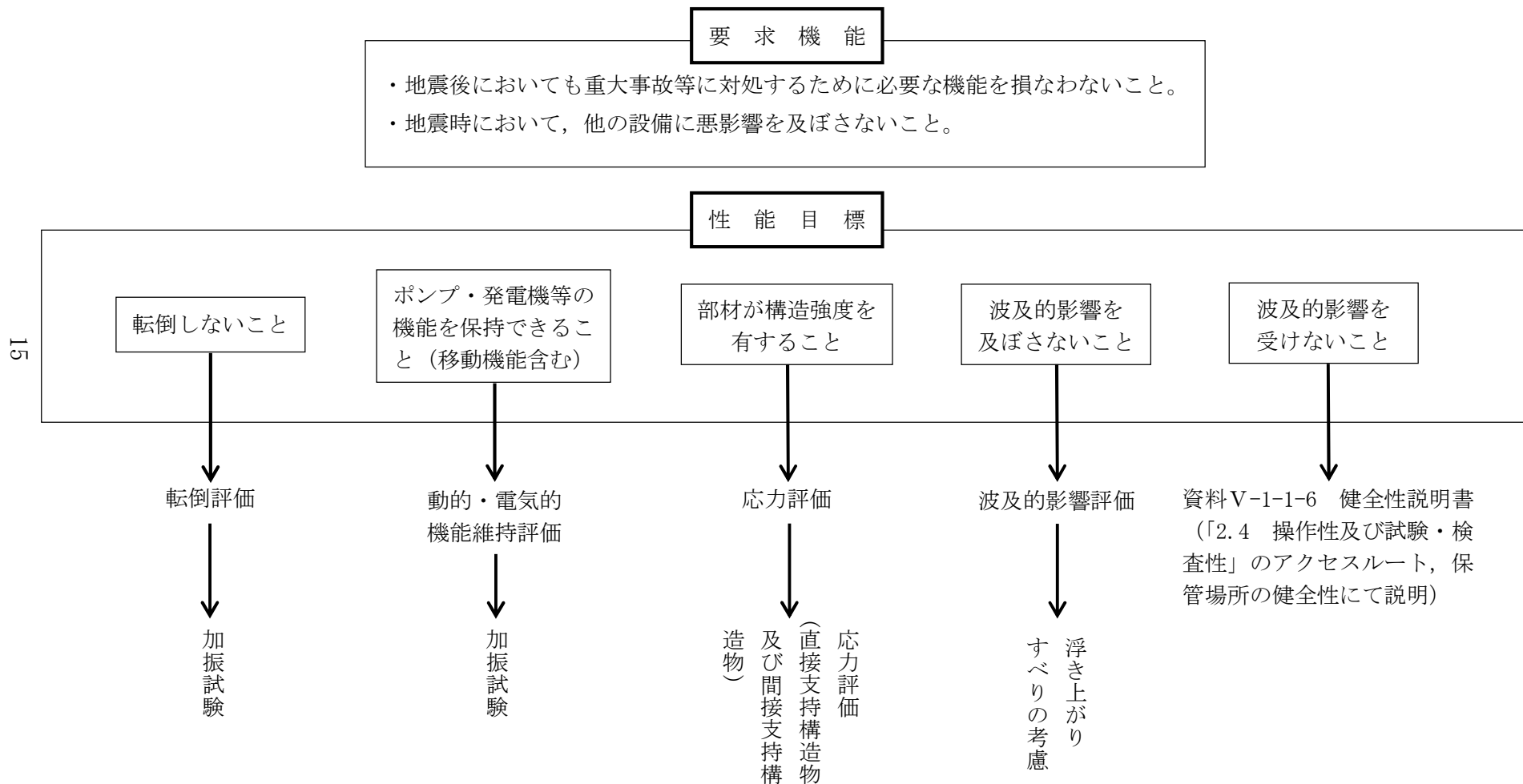
図 3-2-1 評価ツリー
