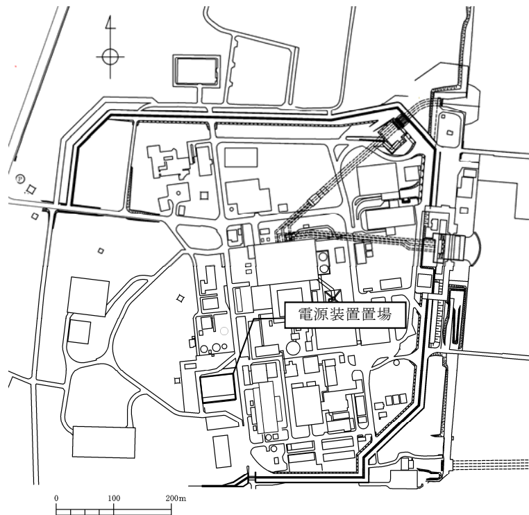
第2-1図 (1) 電源装置置場の平面配置図 (全体平面図)
