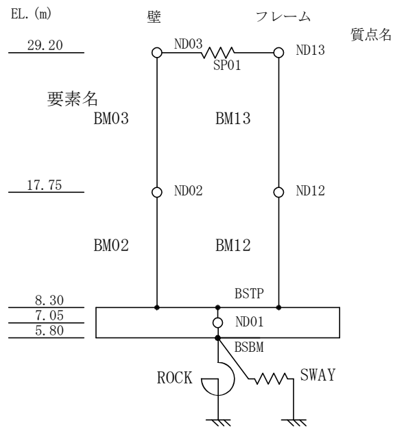
図 3-6 使用済燃料乾式貯蔵建屋地震応答解析モデル (E W 方向)
