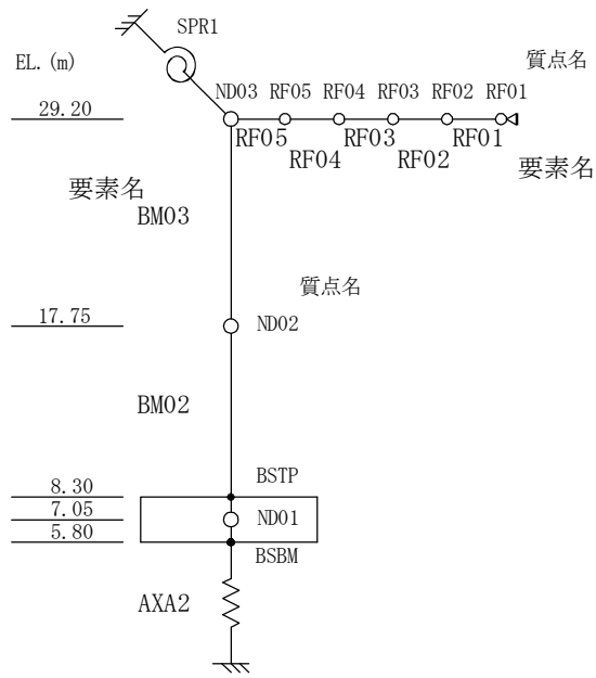
図 3-7 使用済燃料乾式貯蔵建屋地震応答解析モデル (鉛直方向)
