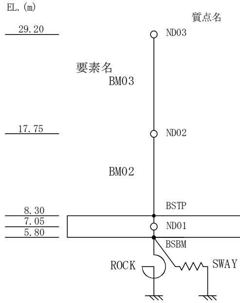
図 3-5 使用済燃料乾式貯蔵建屋地震応答解析モデル (N S 方向)
