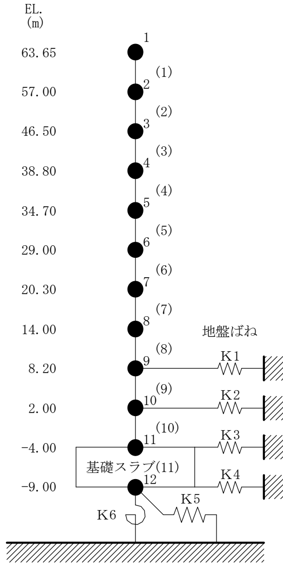
図 3-3 原子炉建屋地震応答解析モデル (水平方向)
