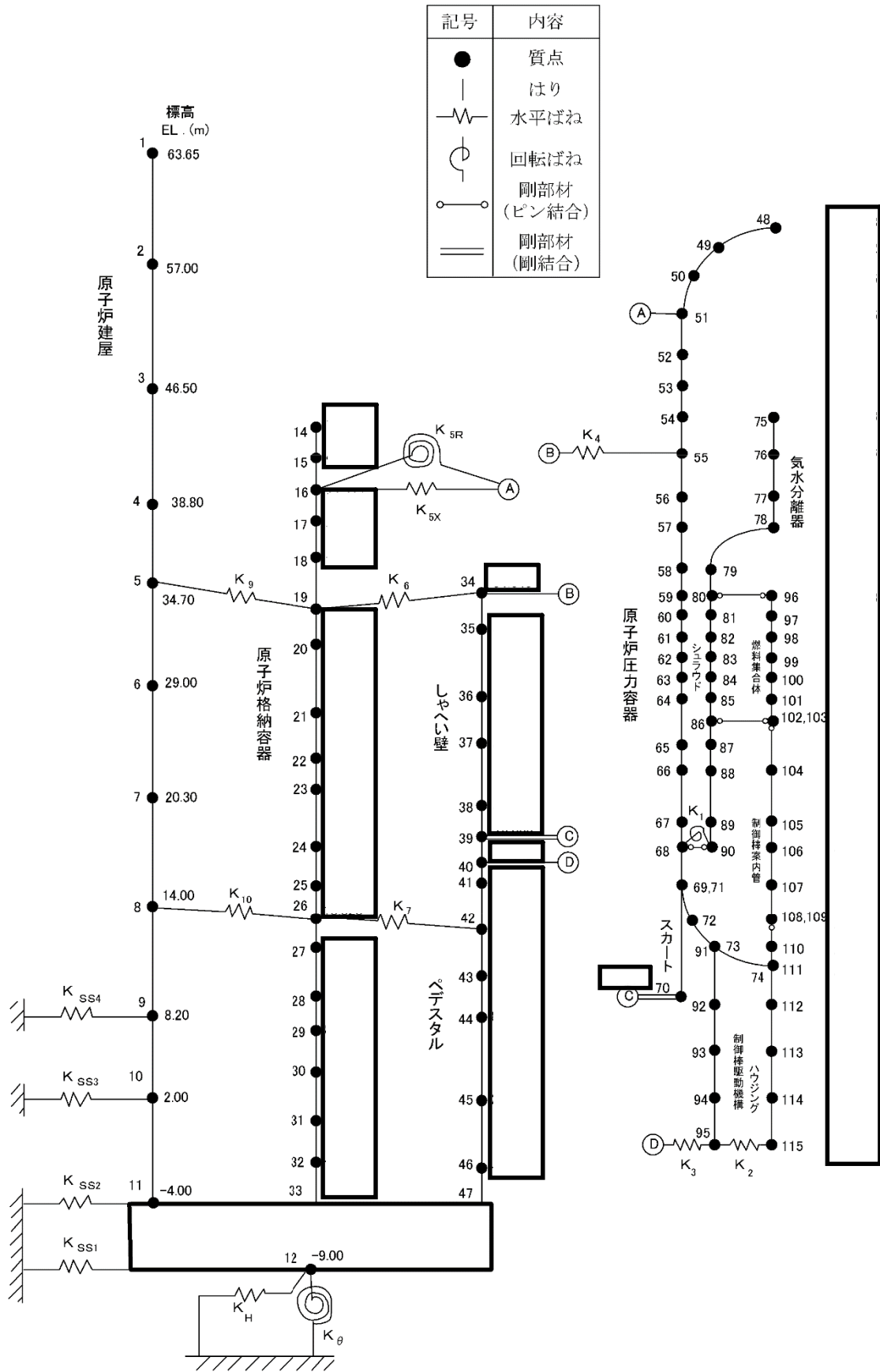
図 3-1 原子炉本体地震応答解析モデル (水平方向)
