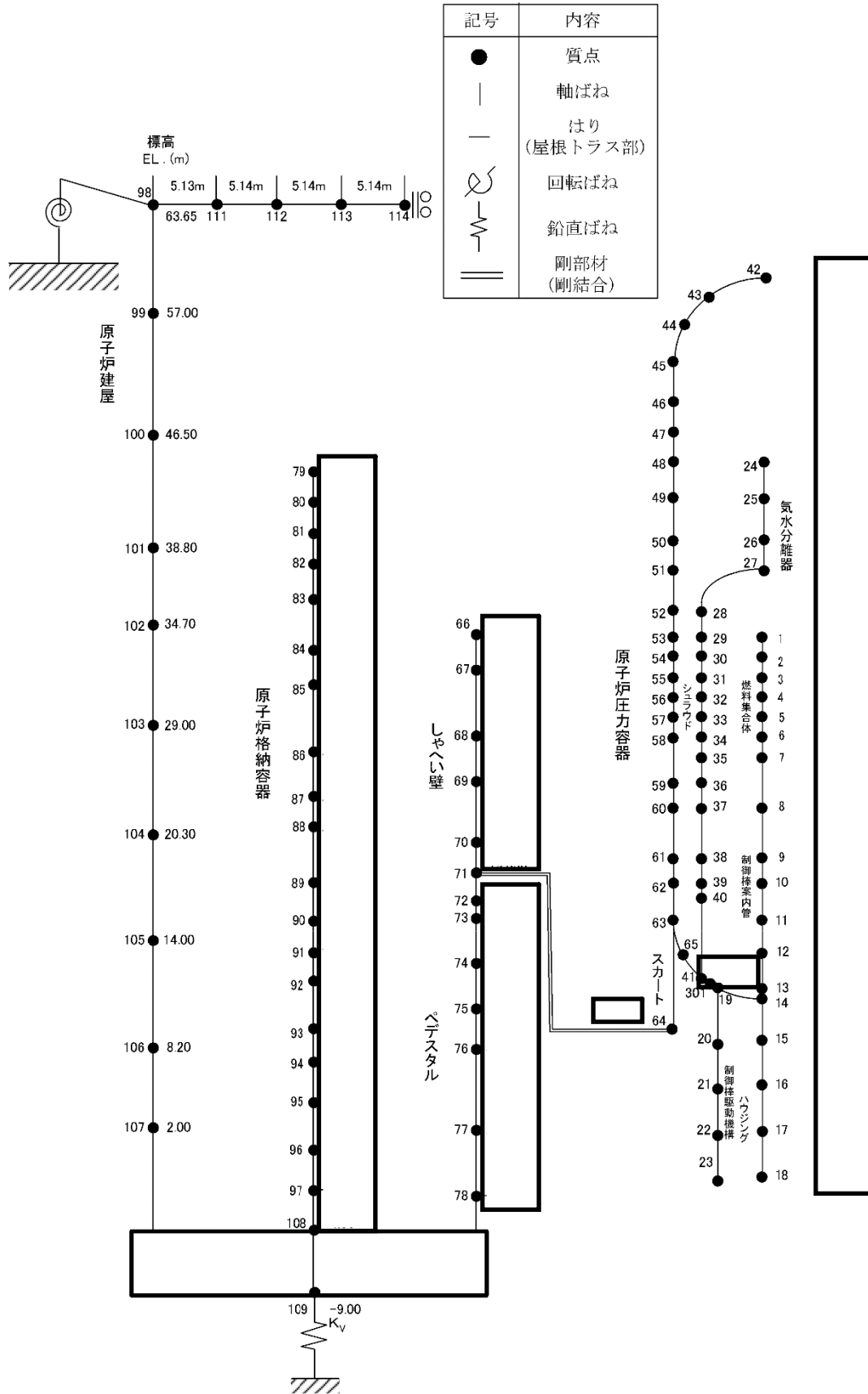
図 3-2 原子炉本体地震応答解析モデル (鉛直方向)
