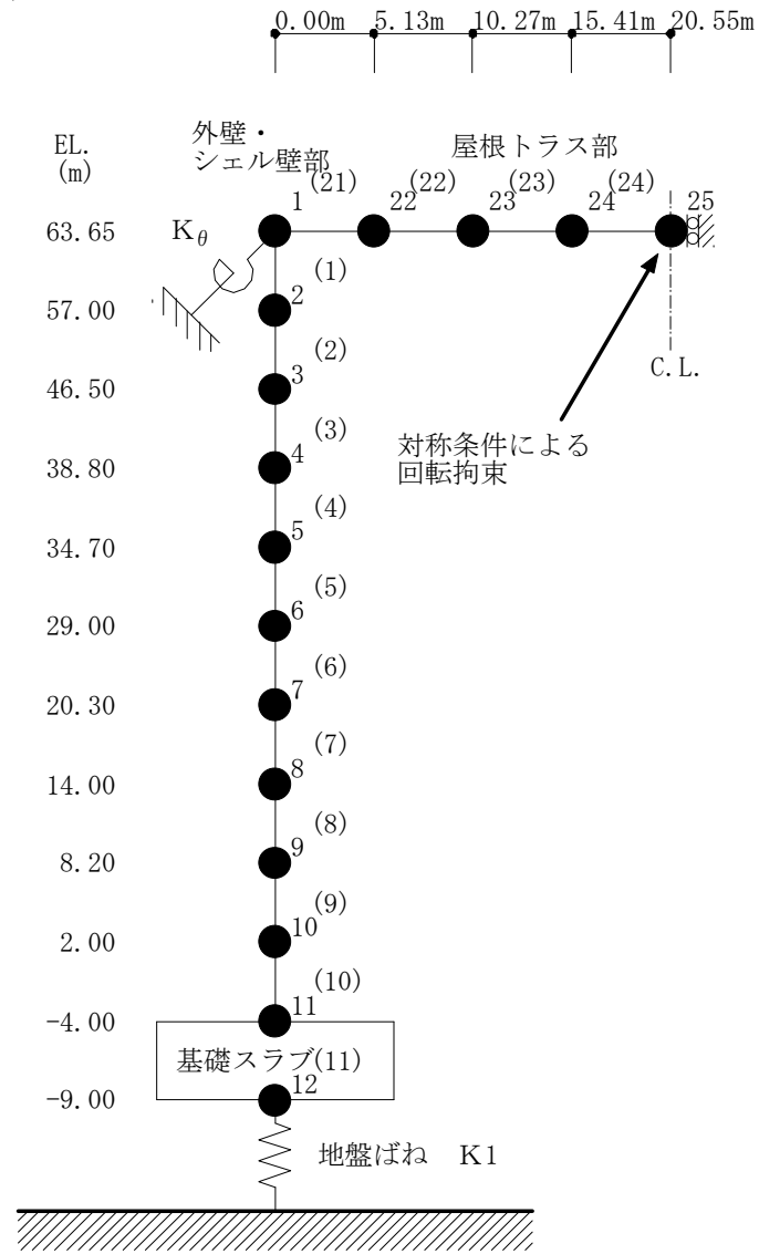
図 3-4 原子炉建屋地震応答解析モデル（鉛直方向）
